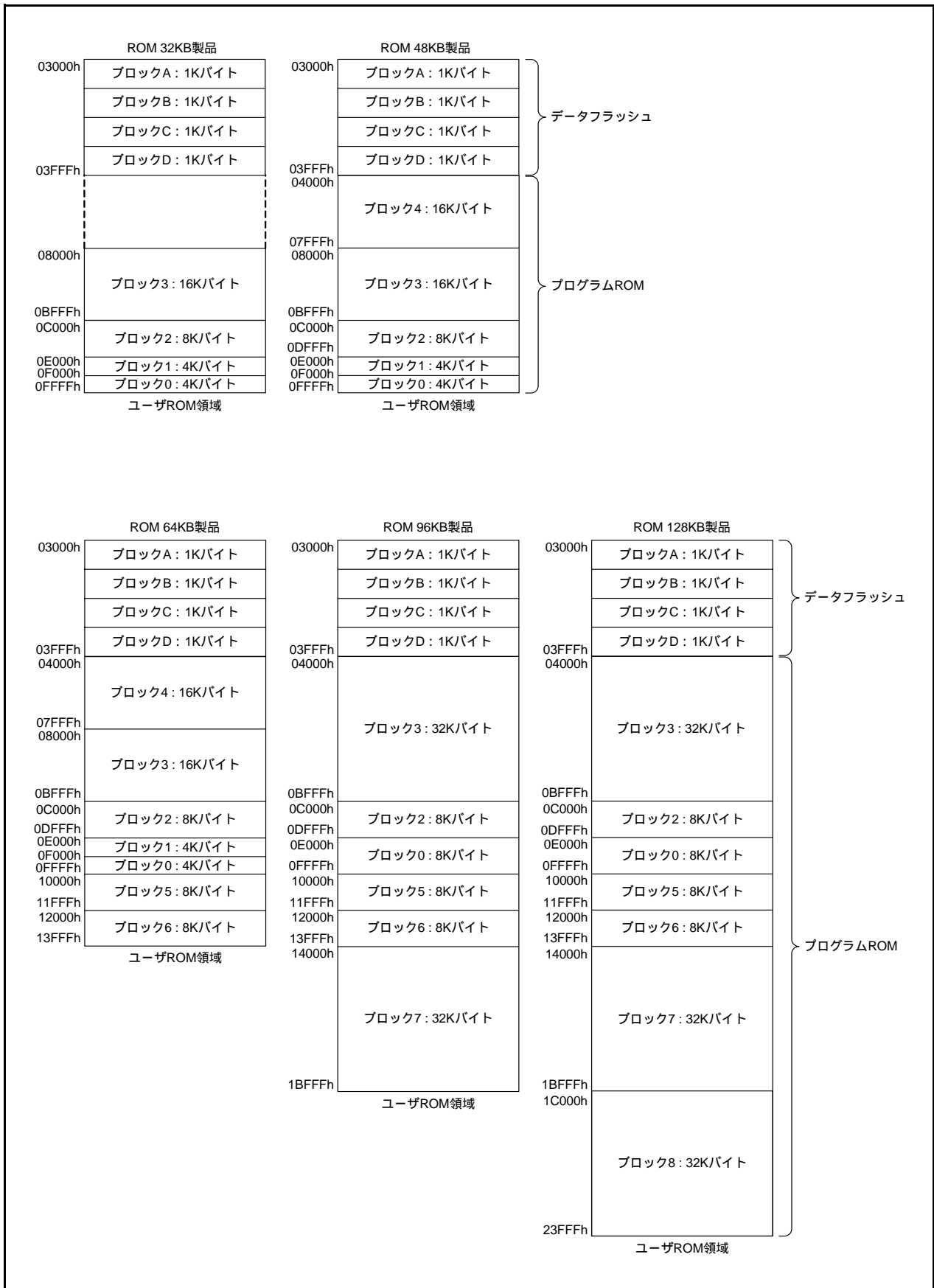
図 33.2 R8C/36C グループのフラッシュメモリのブロック図 (2)
