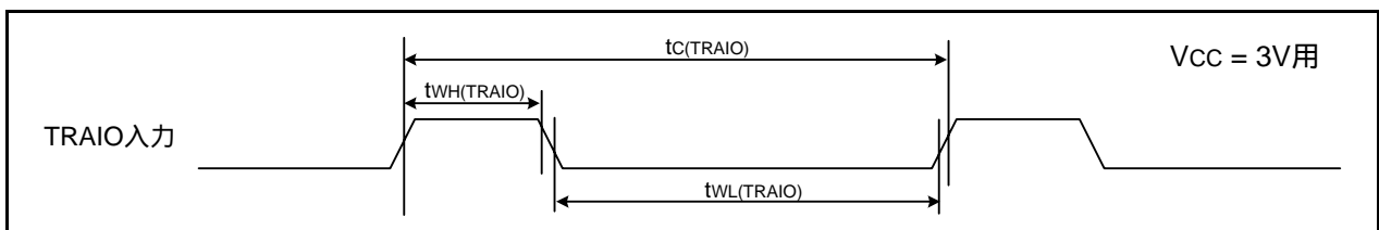
図35.14 VCC = 3V時のTRAI0入力タイミング
