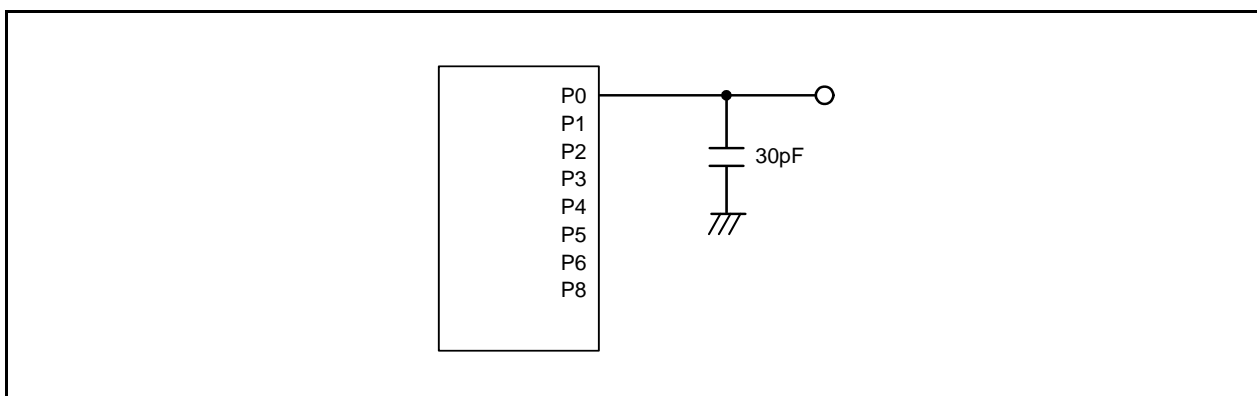
図35.1 ポートP0～P6、P8のタイミング測定回路
