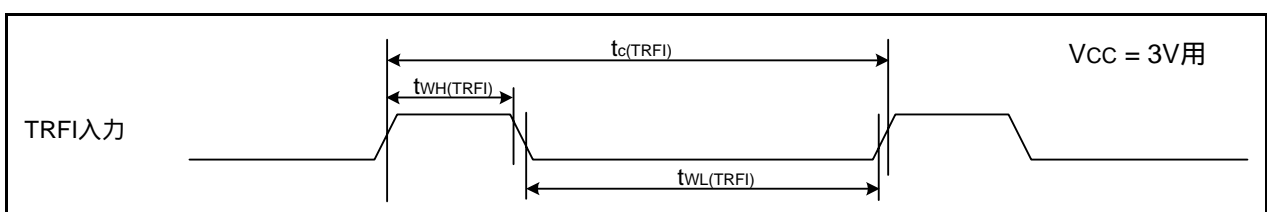
図35.15 VCC = 3V時のTRFI入力タイミング
