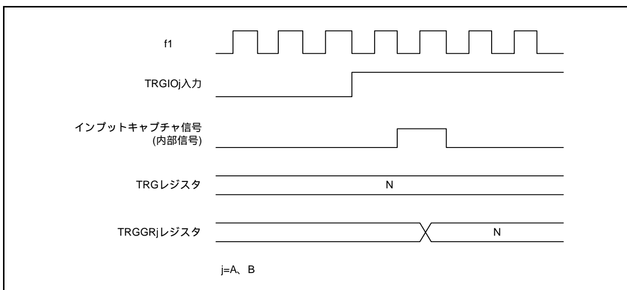
図23.7 インットキャプチャ入力信号タイミング
