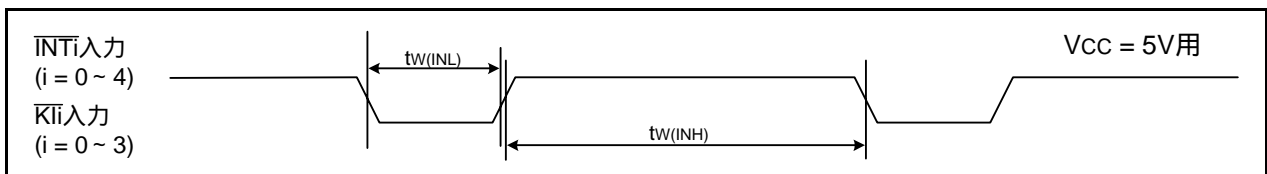
図35.12 Vcc = 5V時の外部割り込み \overline{INTi} およびキー入力割り込み \overline{Kli} 入力タイミング
