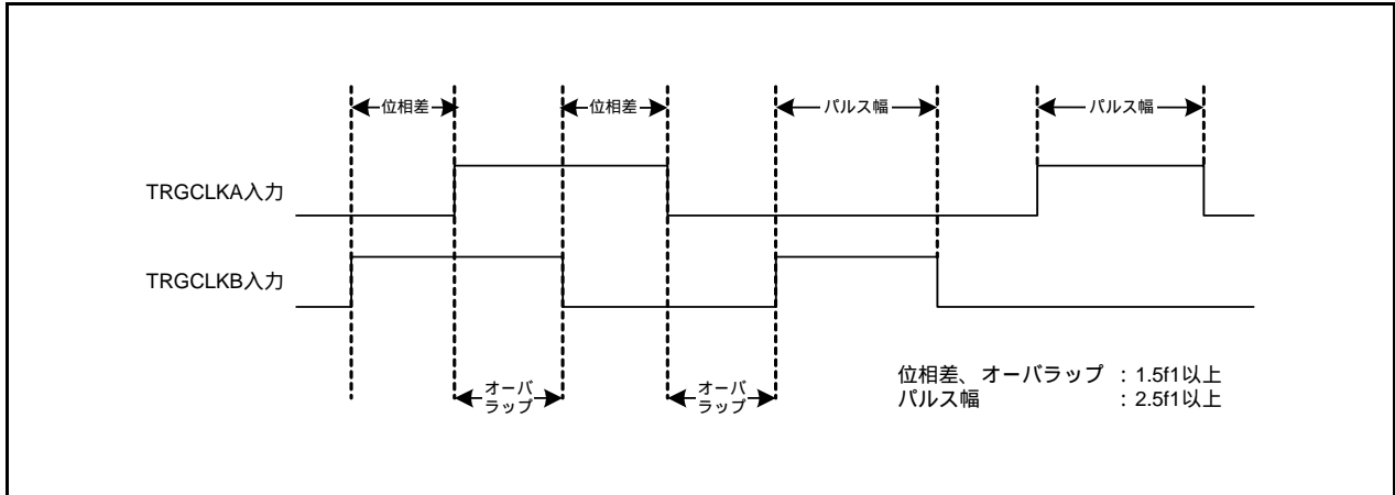
図 36.7 位相計数モード時の位相差、オーバーラップおよびパルス幅
