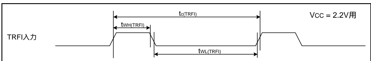
図35.20 VCC = 2.2V時のTRFI入力タイミング
