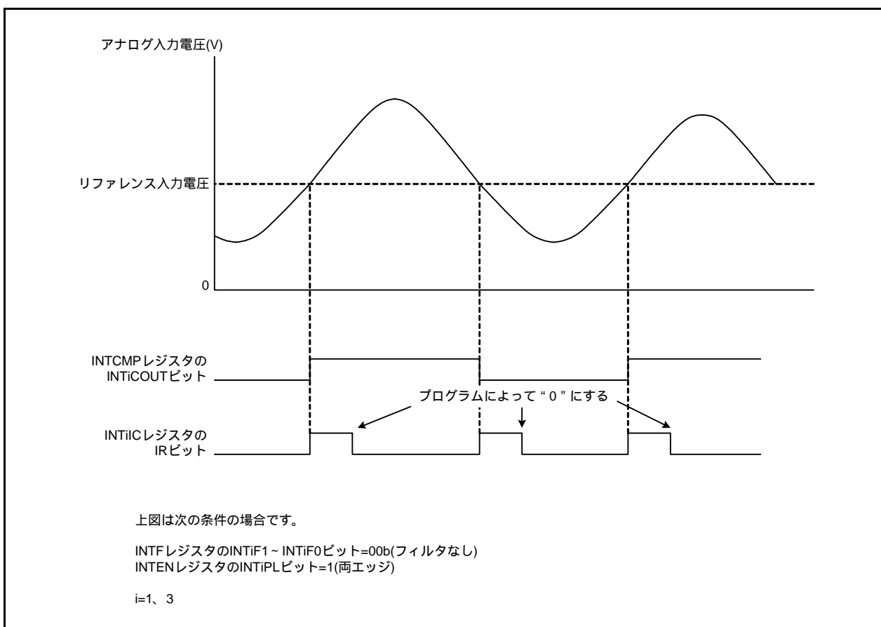
図32.2 コンパレータBi (i=1、3)の動作例
