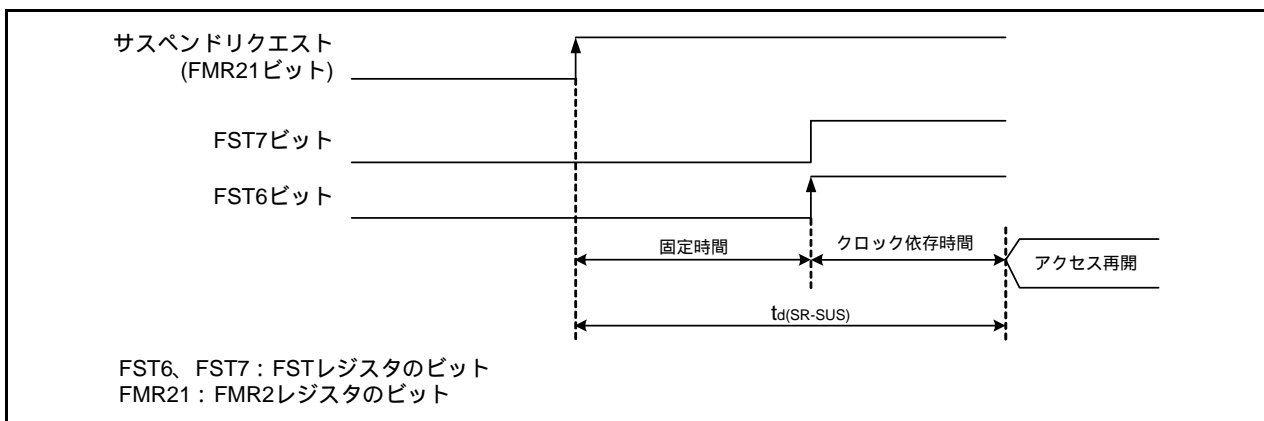
図35.2 サスペンドへの遷移時間
