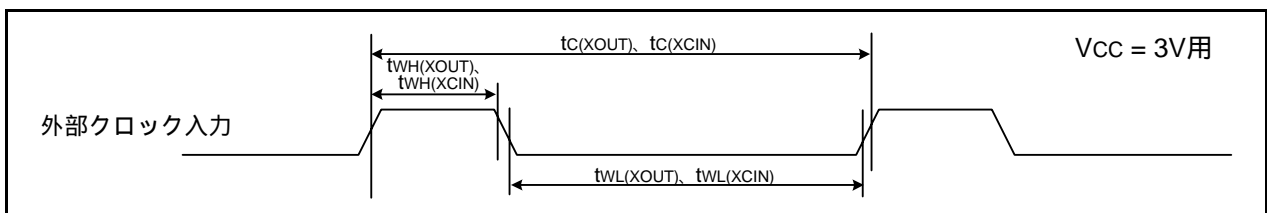
図35.13 VCC = 3V時の外部クロック入力タイミング
