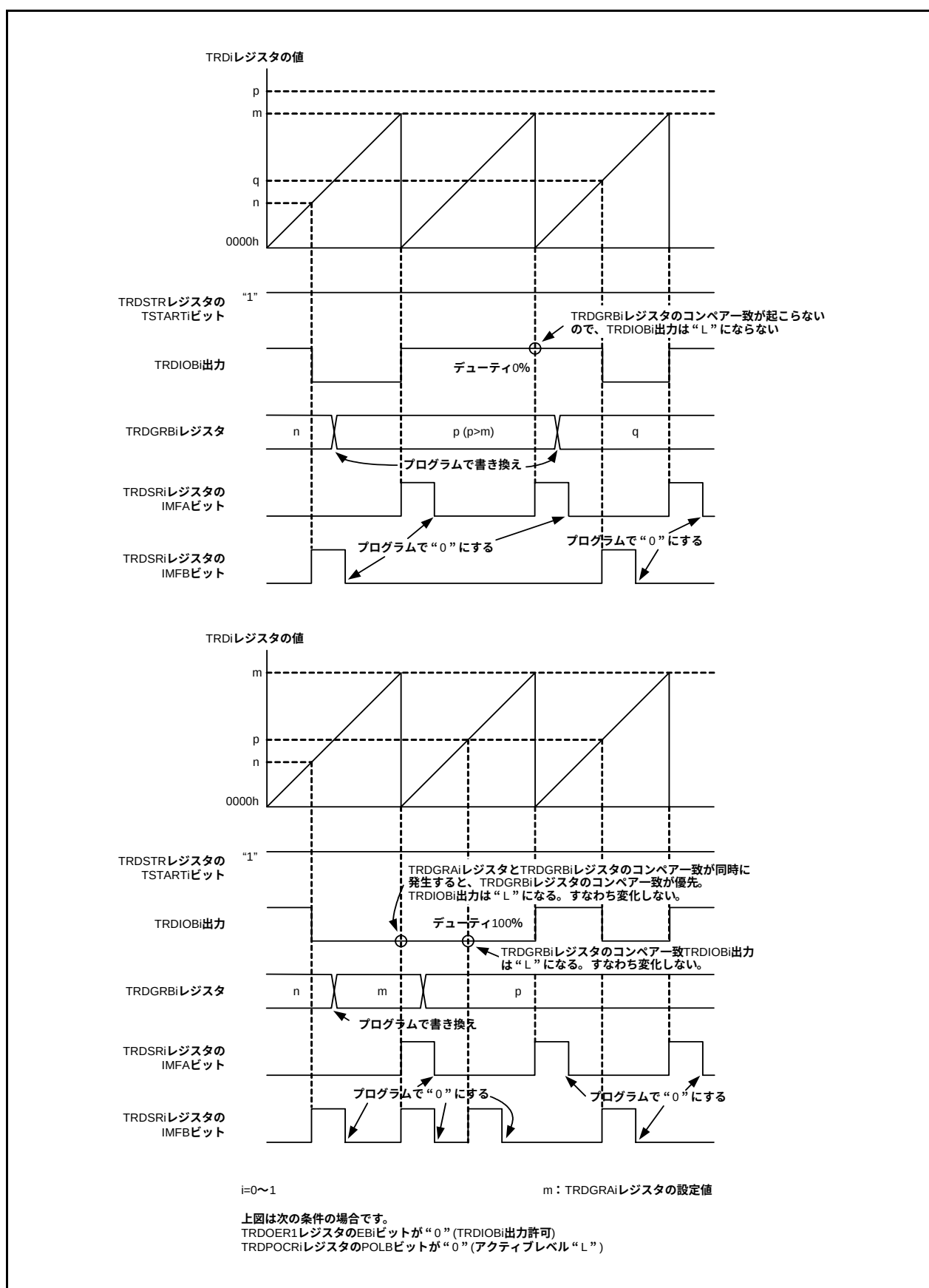
図 20.16 PWM モードの動作例 (デューティ 0%、デューティ 100%)
