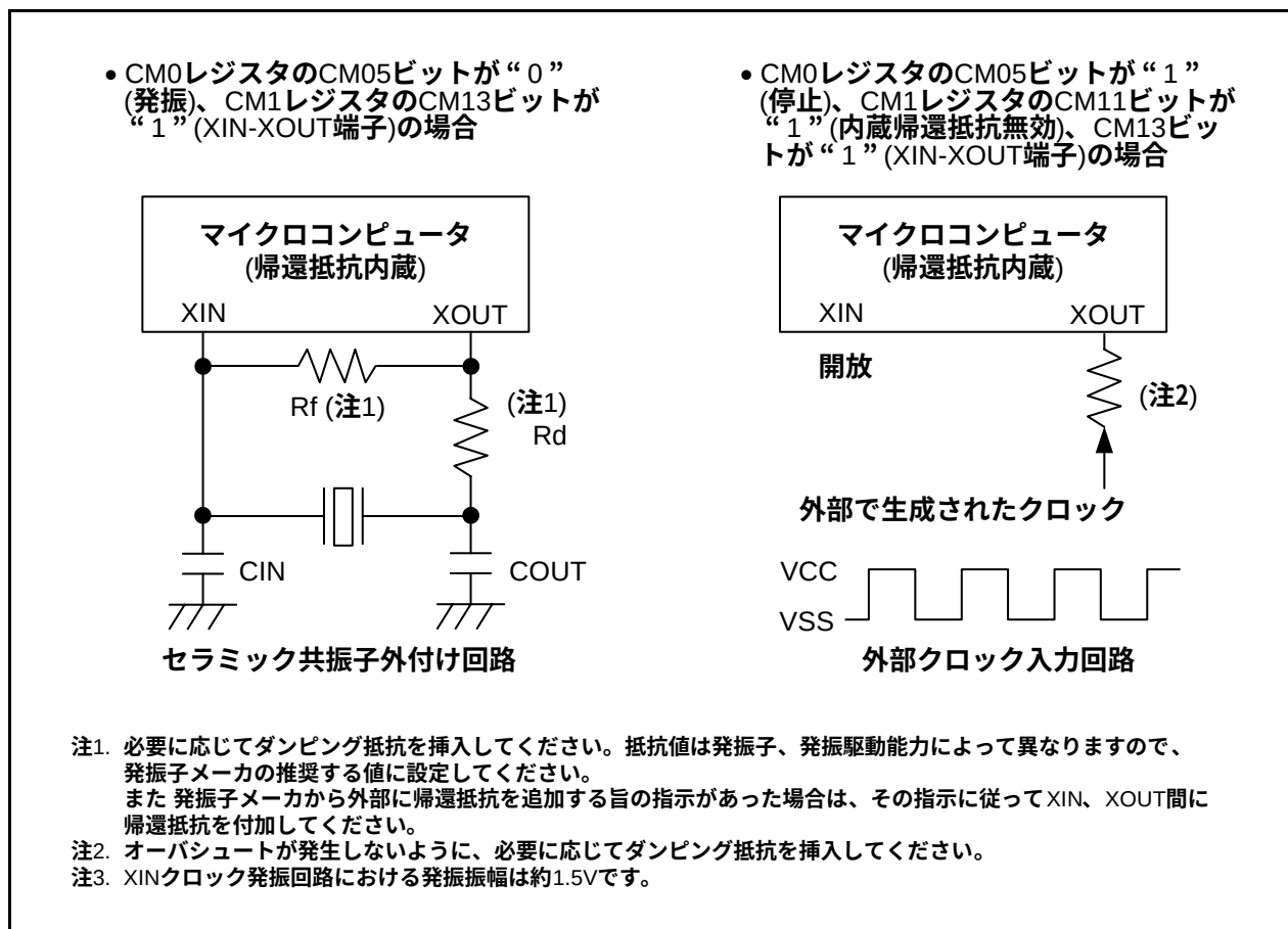
図9.3 XINクロックの接続回路例
