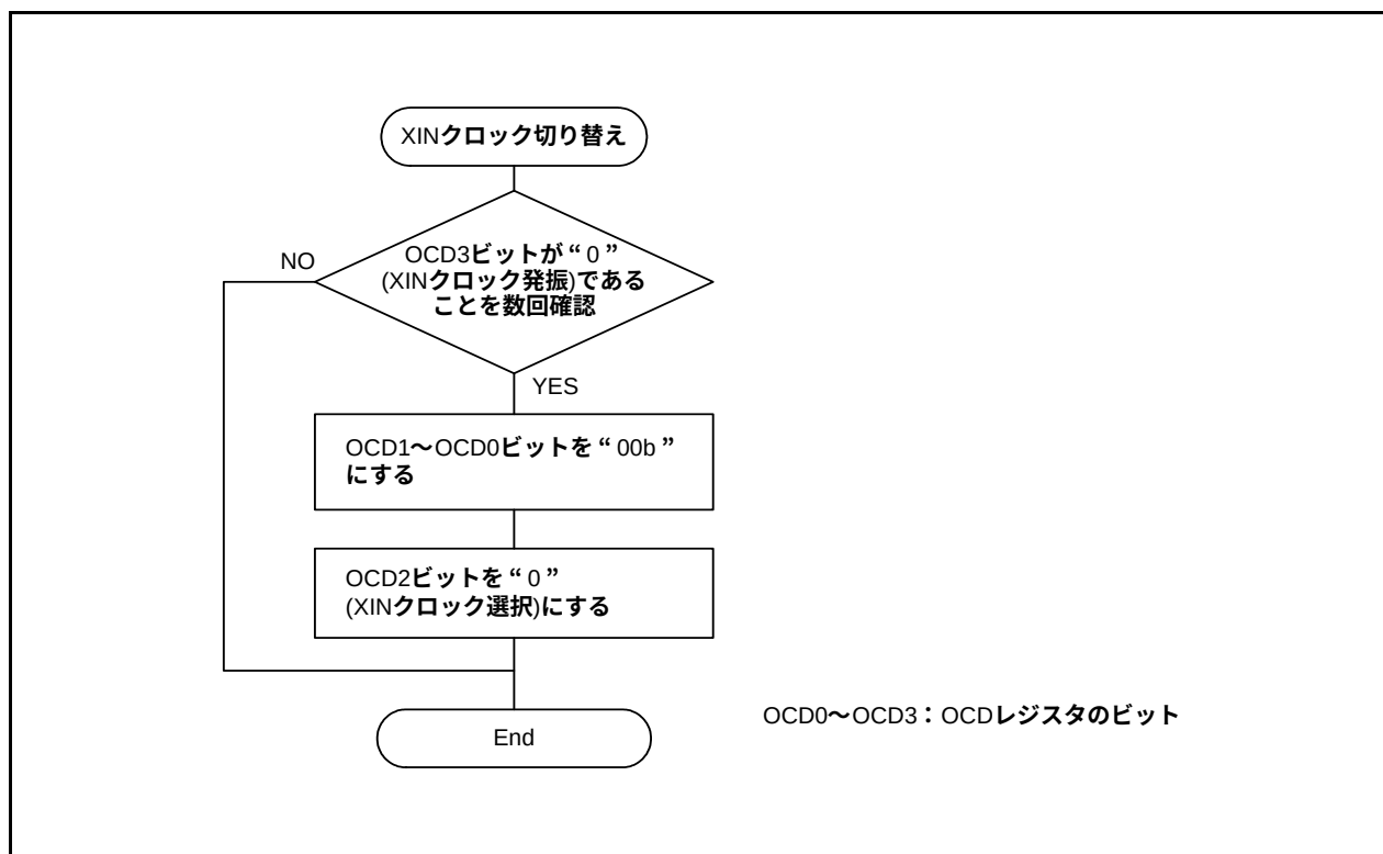
図9.8 発振停止検出後、XIN クロックが再発振した場合のXIN クロックへの切り替え手順
