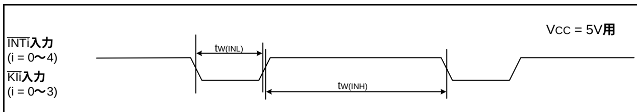
図 30.10 Vcc = 5V時の外部割り込み \overline{\text{INTi}} およびキー入力割り込み \overline{\text{Kli}} 入力タイミング
