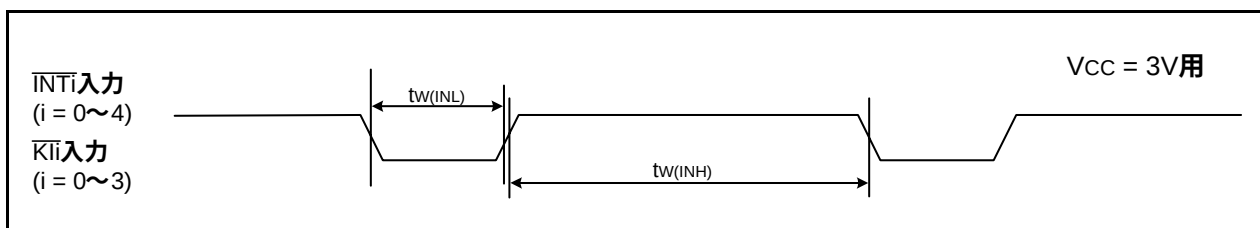
図 30.14 V_{CC} = 3V 時の外部割り込み \overline{INTi} およびキー入力割り込み \overline{Kli} 入力タイミング
