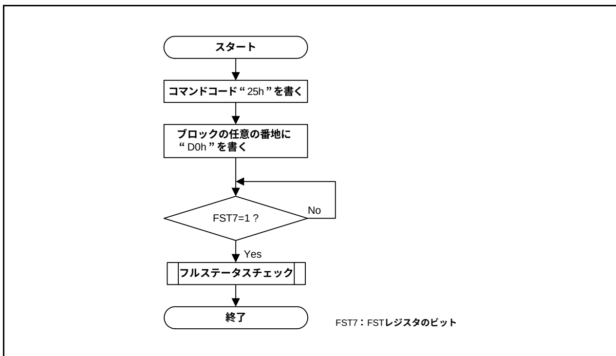
図 28.16 ブロックブランクチェックフローチャート
