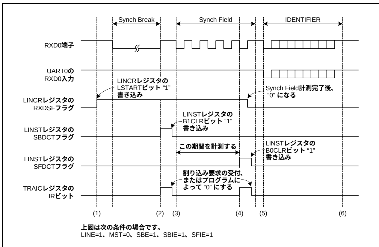
図 24.5 ヘッダフィールドの受信時の動作例
