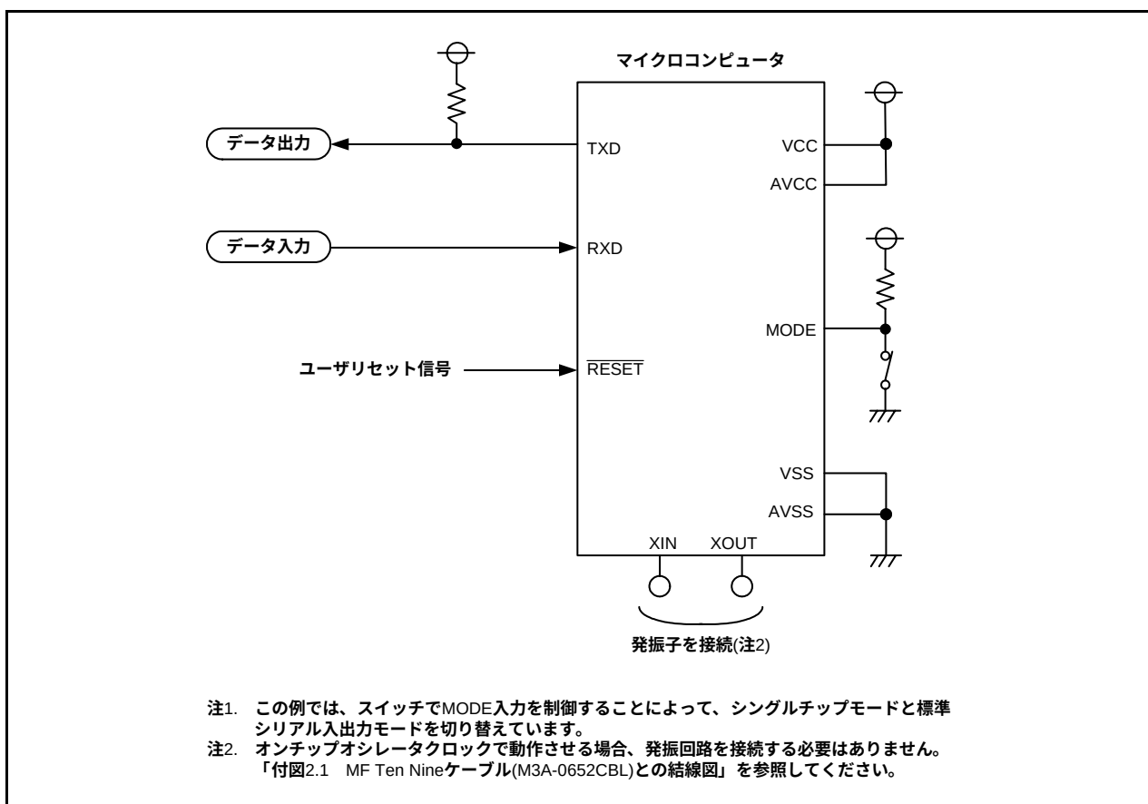
図 28.18 標準シリアル入出力モード2を使用する場合の端子処理例
