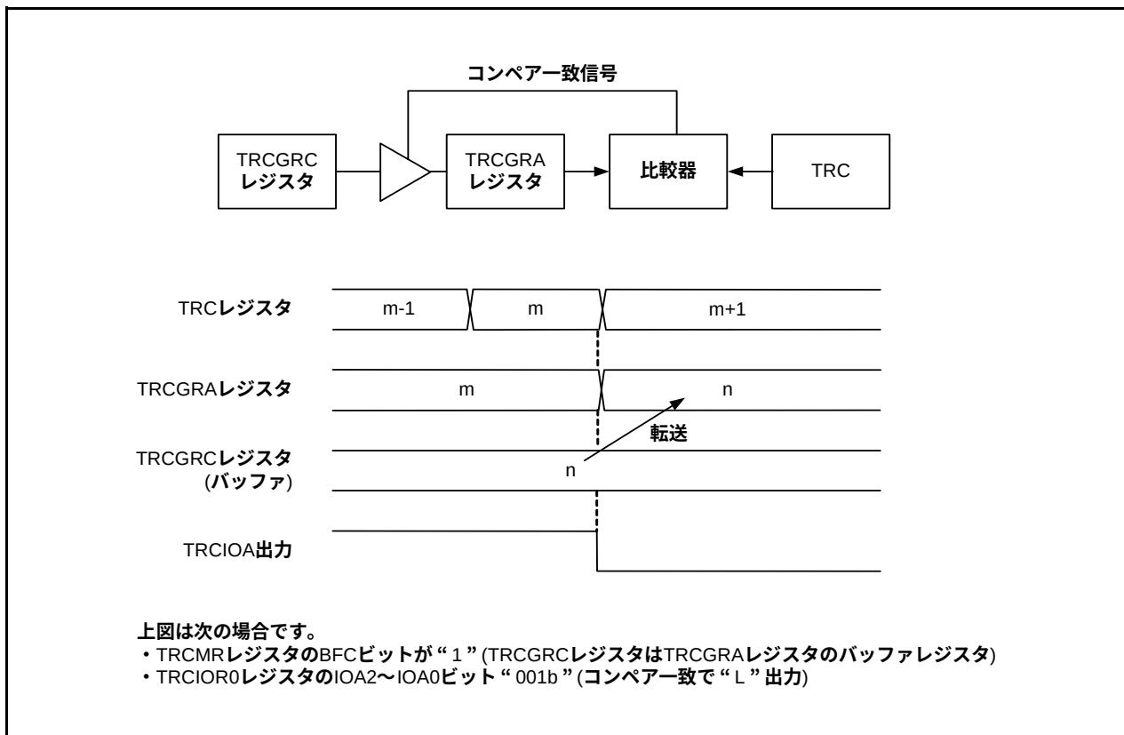
図19.4 アウトプットコンペア機能のバッファ動作
