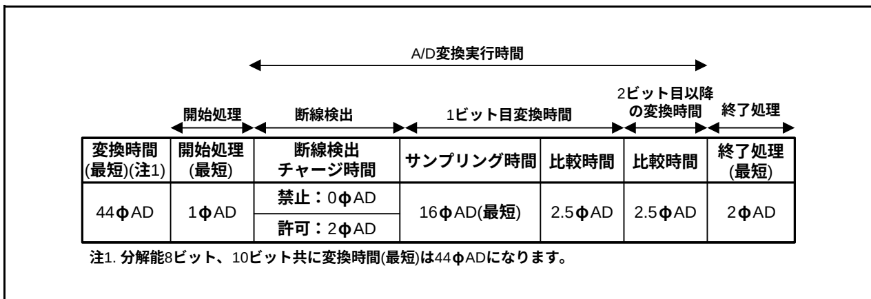
図25.3 A/D変換サイクル数( \phi_{AD} = f_{AD} のとき)
