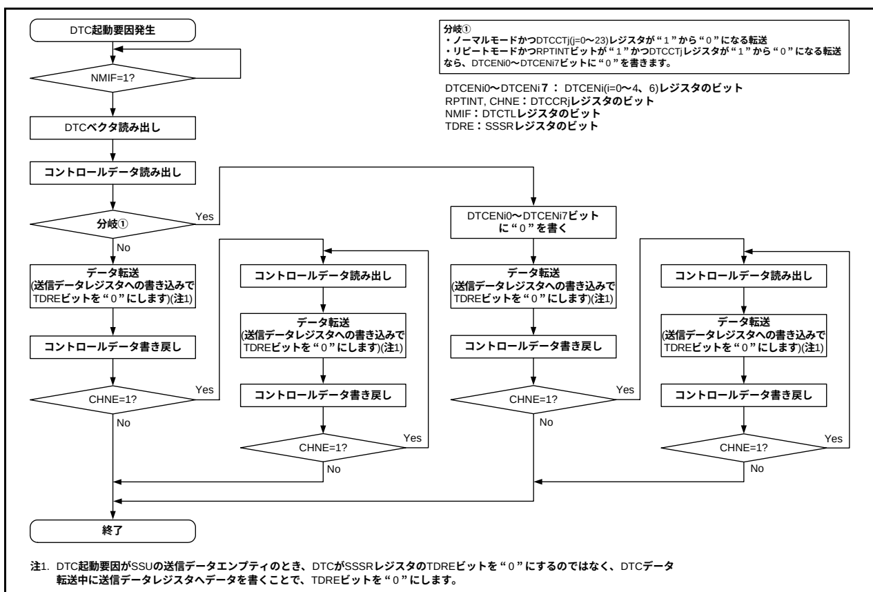
図 15.6 DTC起動要因がSSUの送信データエンプティであるときのDTC内部動作フローチャート
