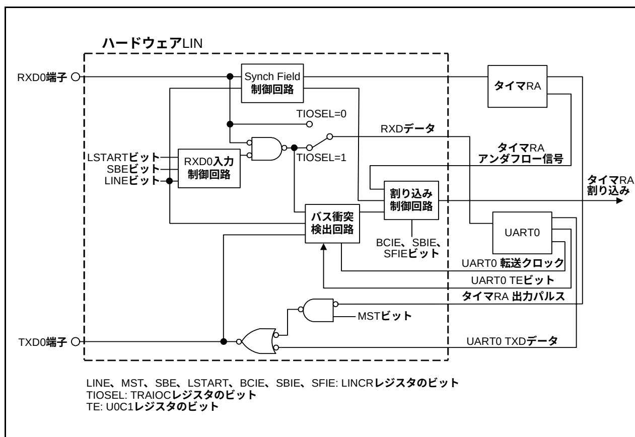
図 24.1 ハードウェア LIN のブロック図
