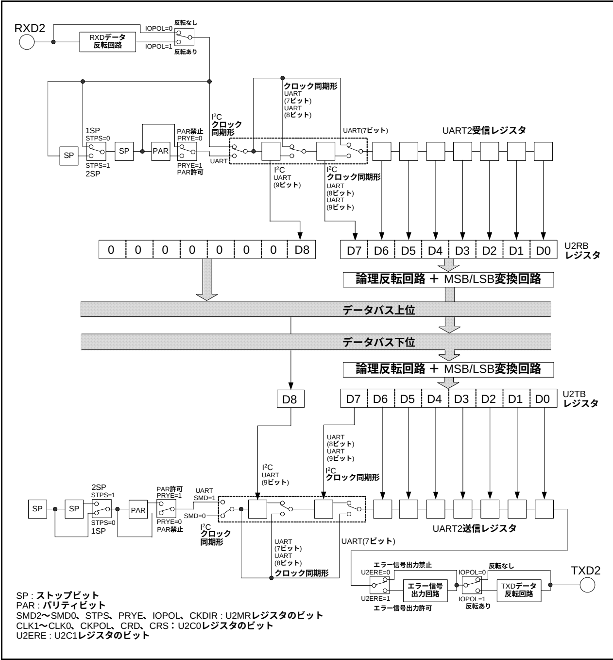
図 22.2 UART2受信部のブロック図
