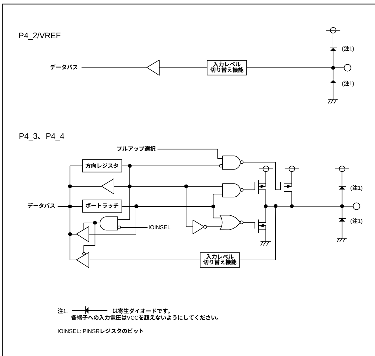
図7.9 I/Oポートの構成(9)
