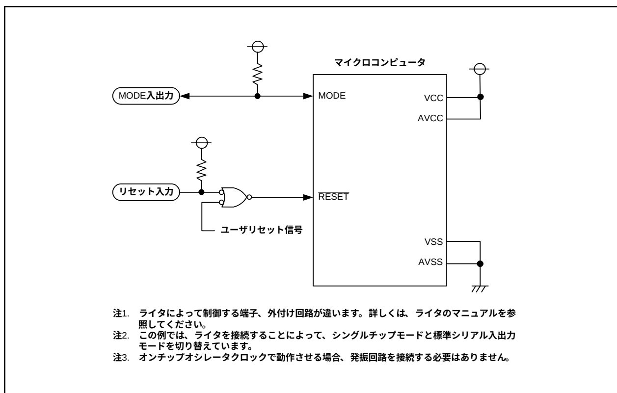
図 28.19 標準シリアル入出力モード3を使用する場合の端子処理例
