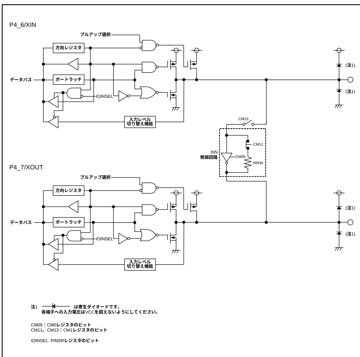
図7.11 I/Oポートの構成(11)
