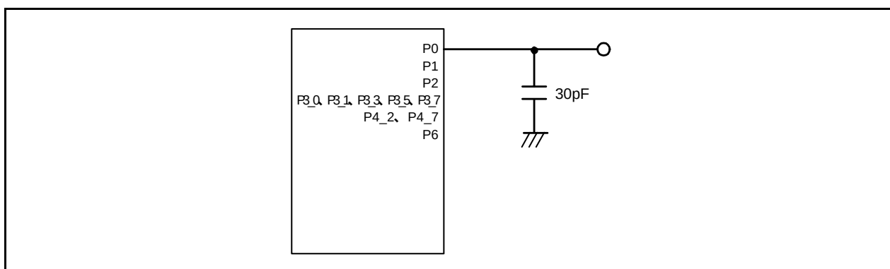
図 30.1 ポート P0～P2、P3_0、P3_1、P3_3～P3_5、P3_7、P4_2～P4_7、P6 のタイミング測定回路
