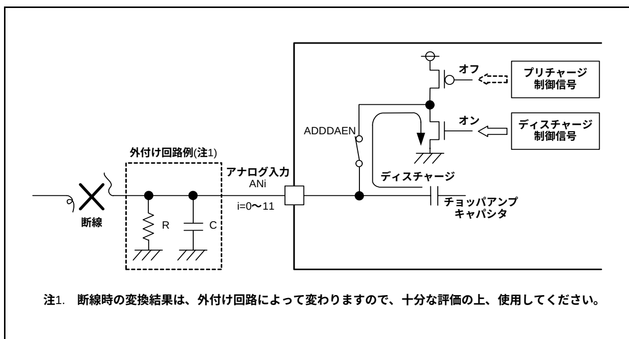
図 25.6 AVSS側でのA/D断線検出例(変換前デイスチャージを選択)
