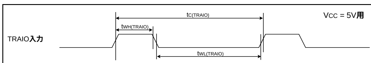
図 30.8 V_{CC} = 5V 時のTRAIO入力タイミング
