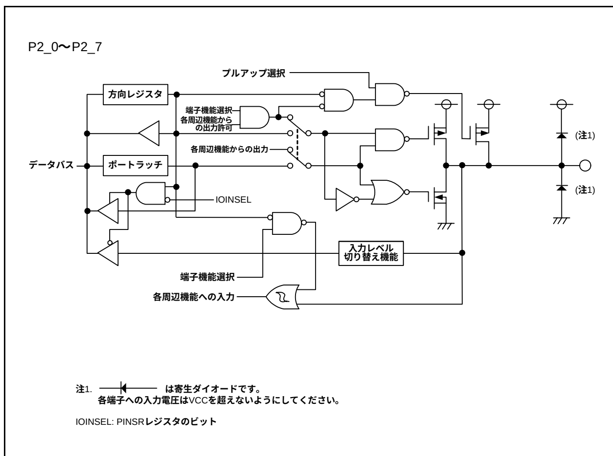
図7.6 I/Oポートの構成(6)
