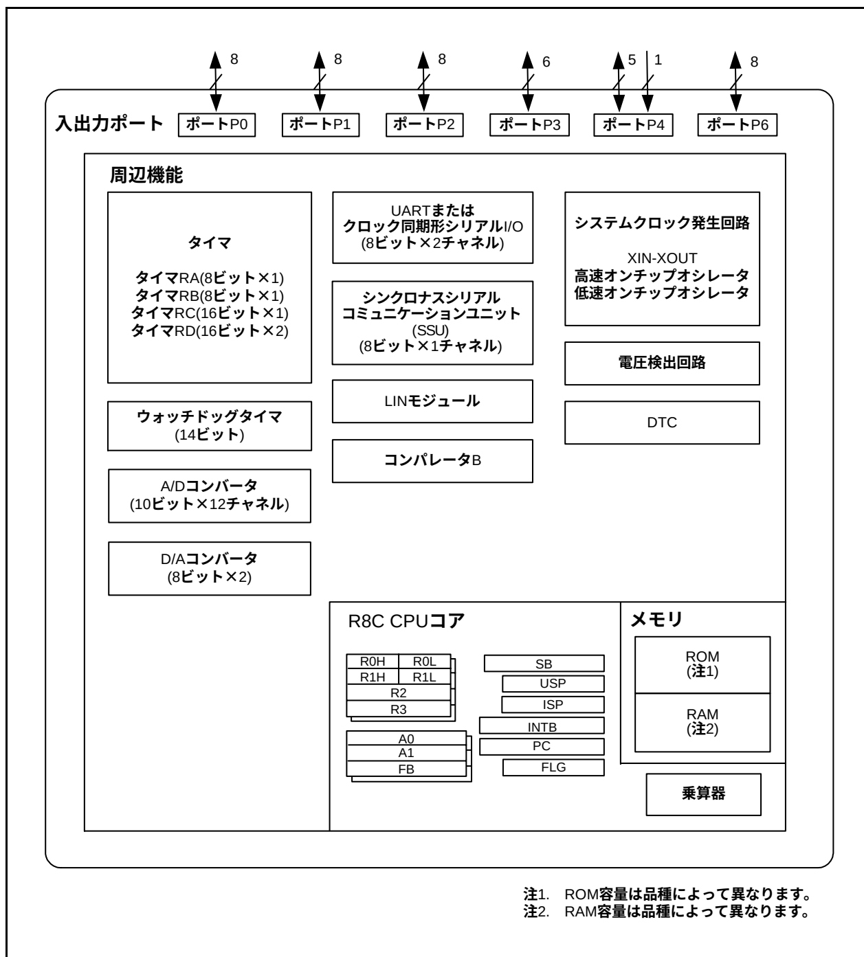
図1.3 ブロック図
