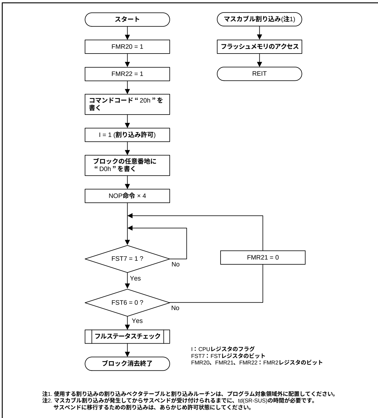
図 28.13 EW1モードのブロックイレーズフローチャート(フラッシュレディステータス割り込み禁止かつサスペンド許可)
