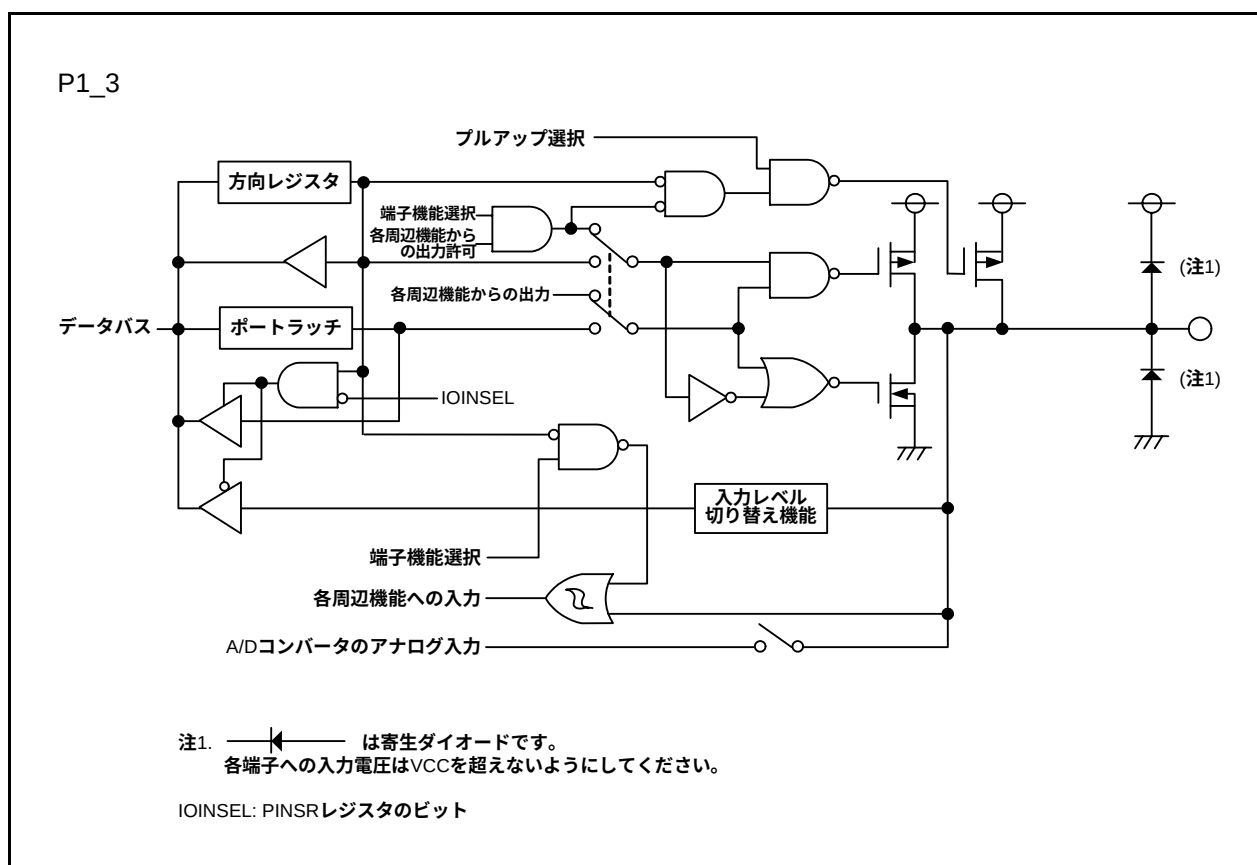
図7.3 I/Oポートの構成(3)
