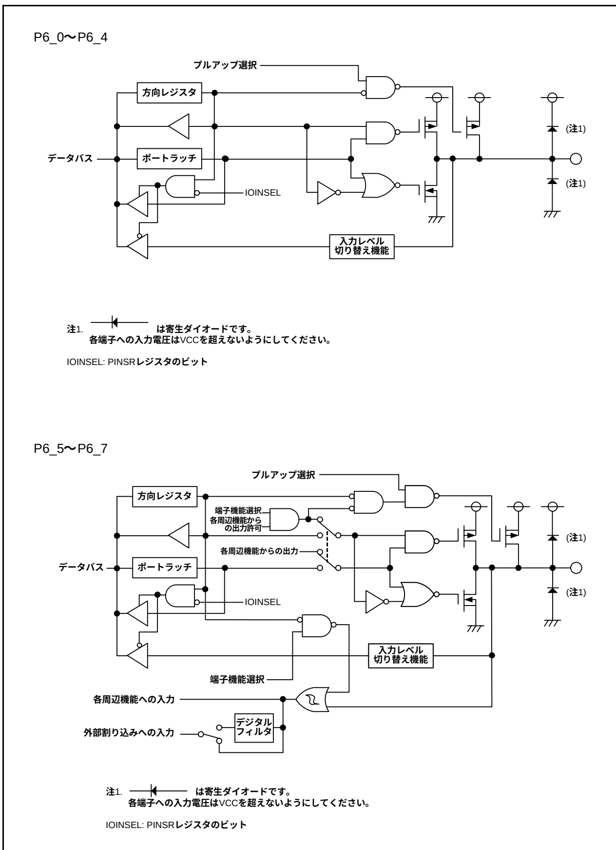
図7.12 I/Oポートの構成(12)
