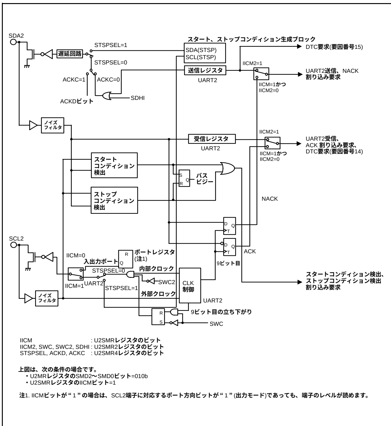
図 22.13 I²Cモードのブロック図
