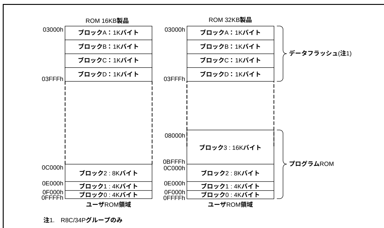
図 28.1 R8C/34Pグループ、R8C/34Rグループのフラッシュメモリのブロック図
