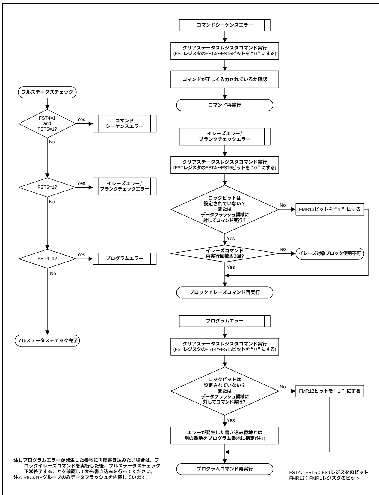
図 28.17 フルステータスチェックフローチャート、各エラー発生時の対処方法
