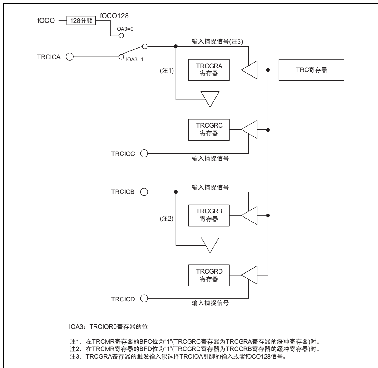
图 15.42 输入捕捉功能的框图
