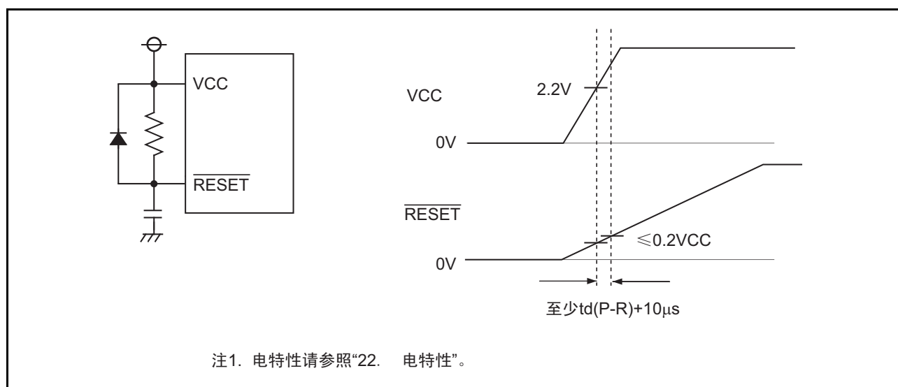
图 6.5 硬件复位的电路例子和运行
