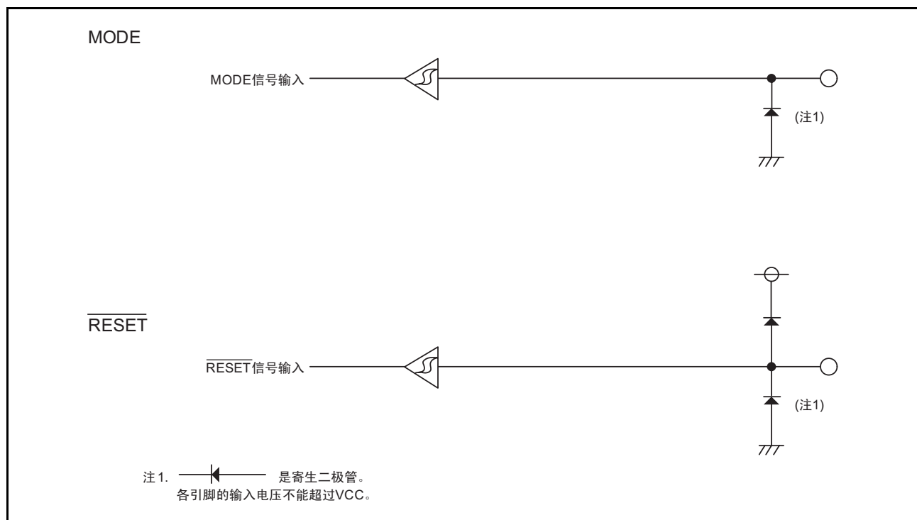
图 8.6 引脚的结构
