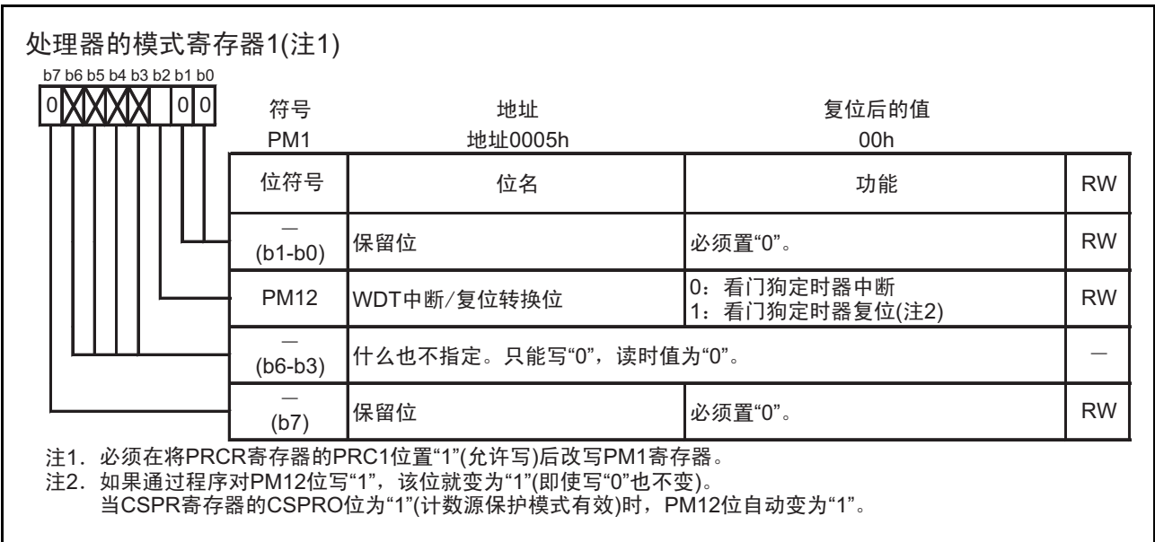
图 9.2 PM1 寄存器
