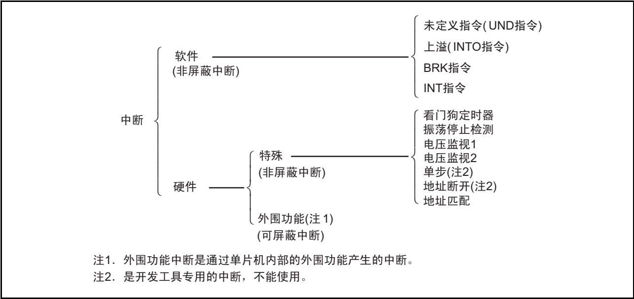
图 13.1 中断分类
