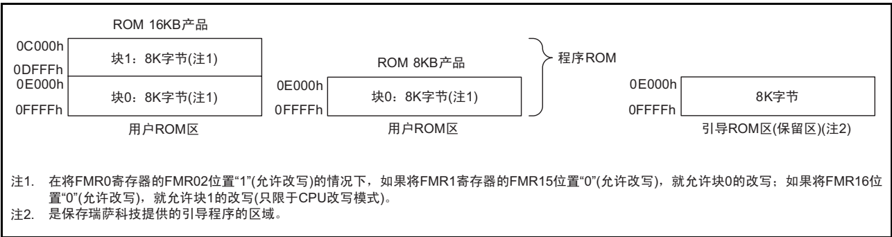
图 21.1 R8C/2E 群的闪存框图
