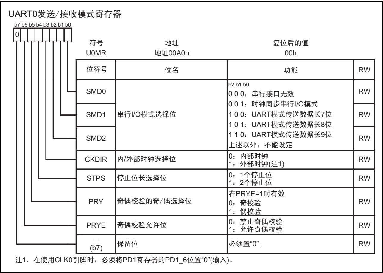
图 16.4 U0MR 寄存器
