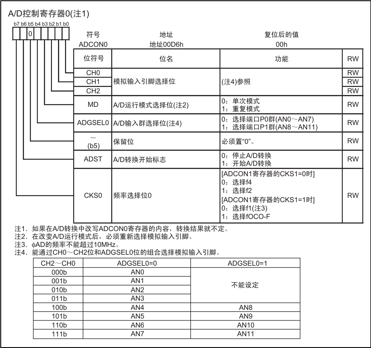
图 18.2 ADCON0 寄存器
