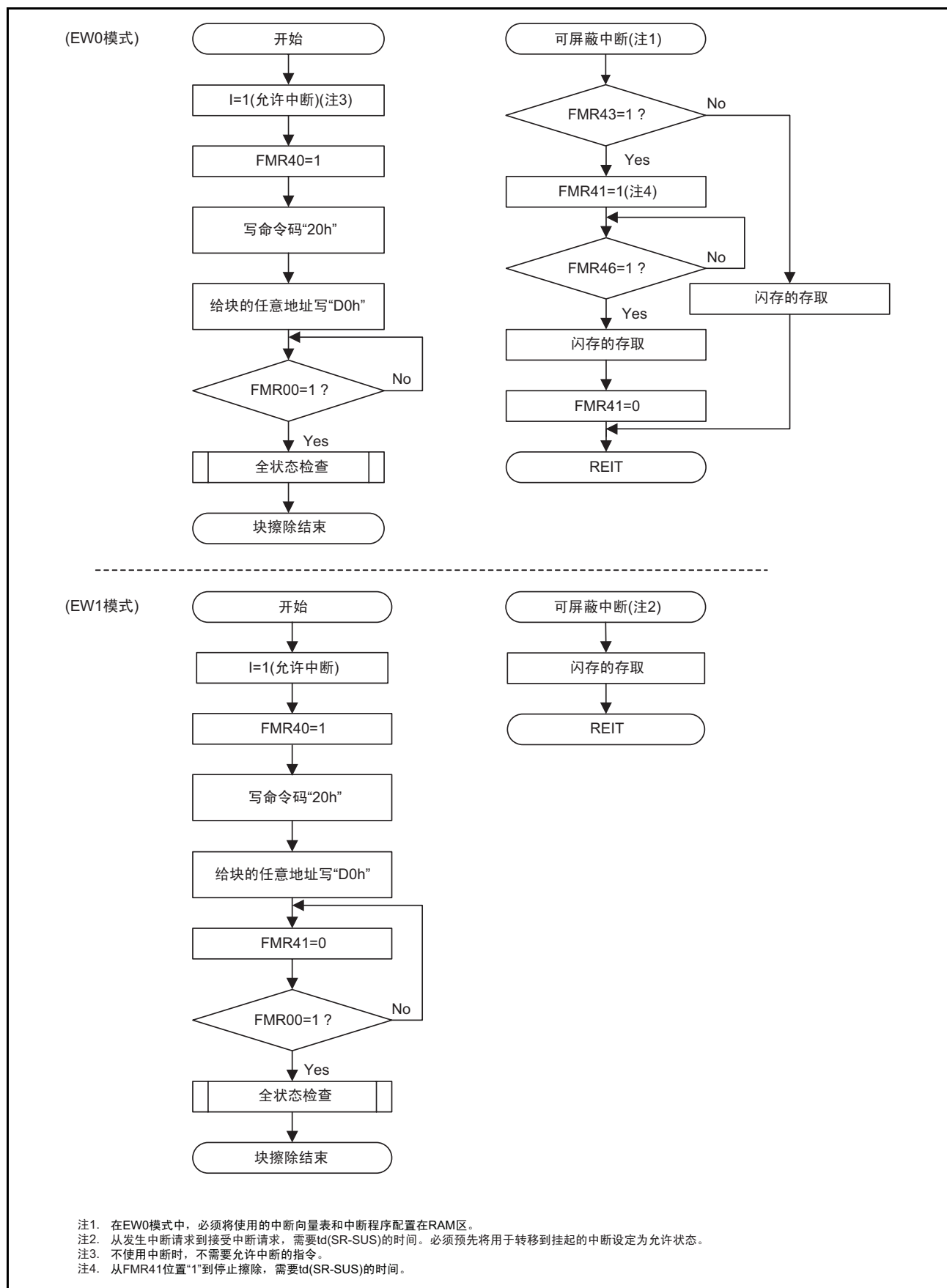
图 21.15 块擦除流程图（允许擦除挂起功能时）
