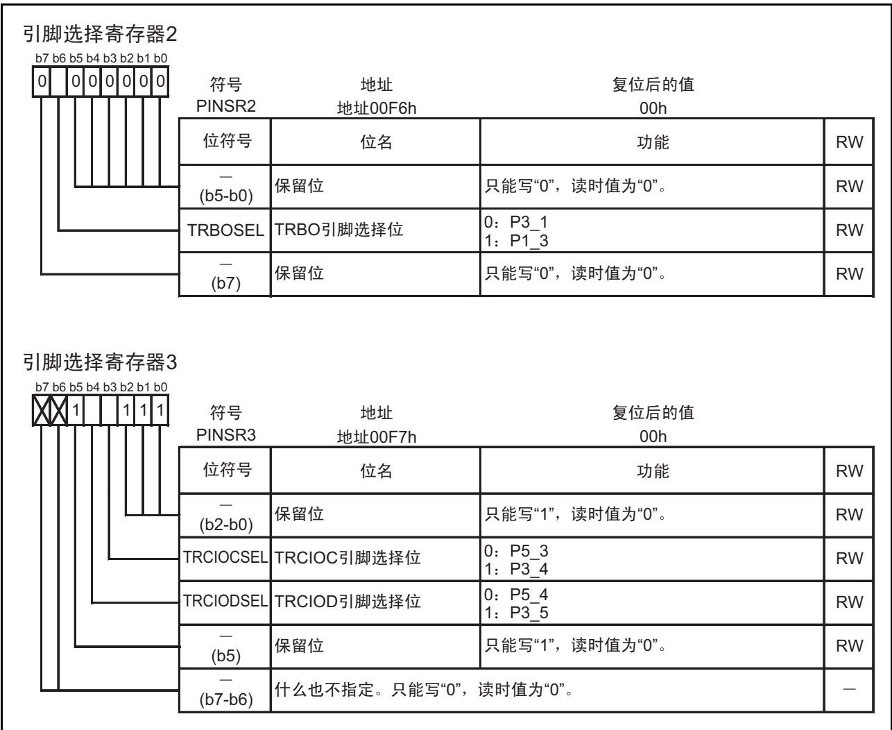
图 8.9 PINSR2 和 PINSR3 寄存器
