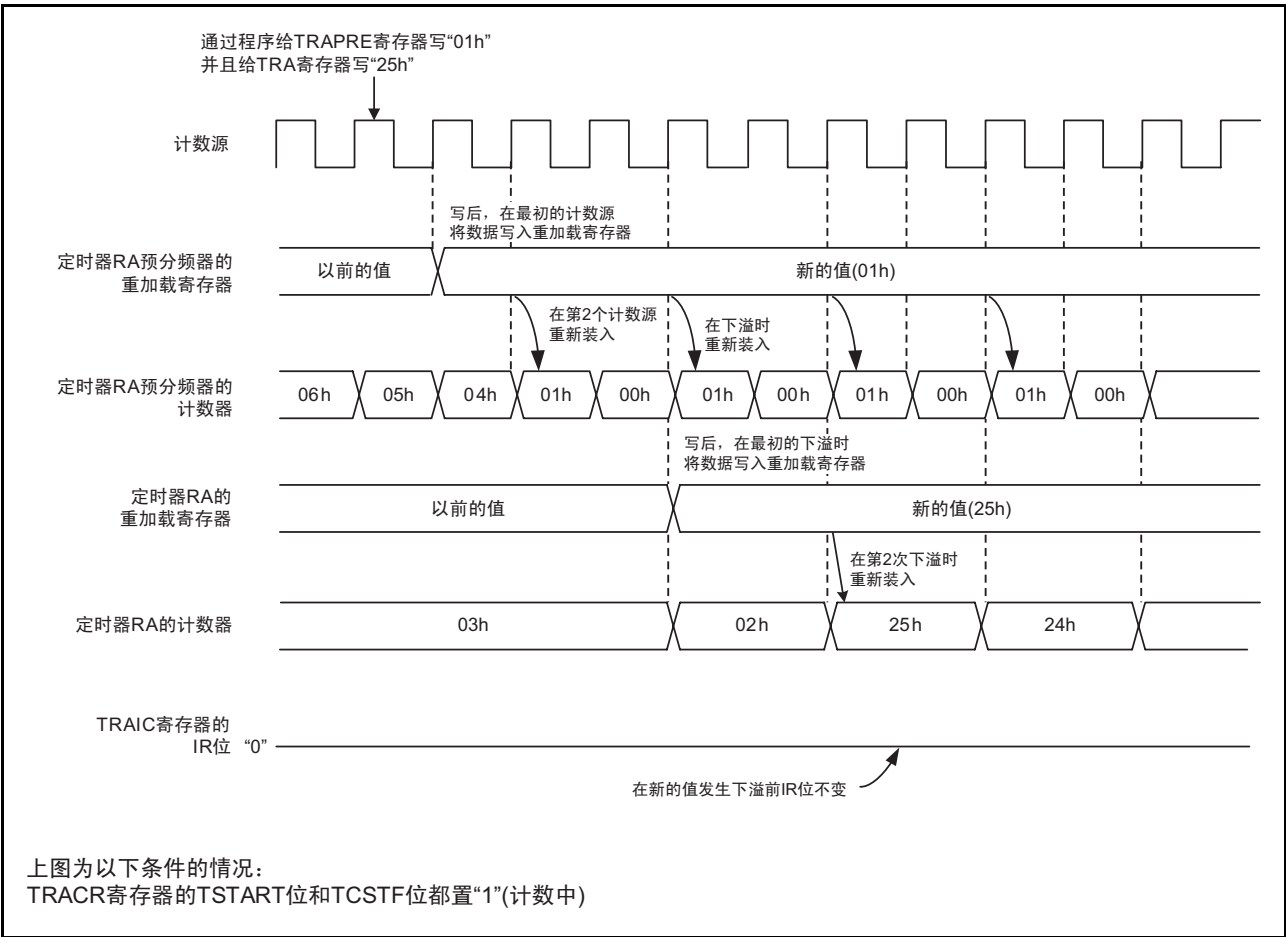
图 15.5 在定时器 RA 计数中改写计数值的运行例子
