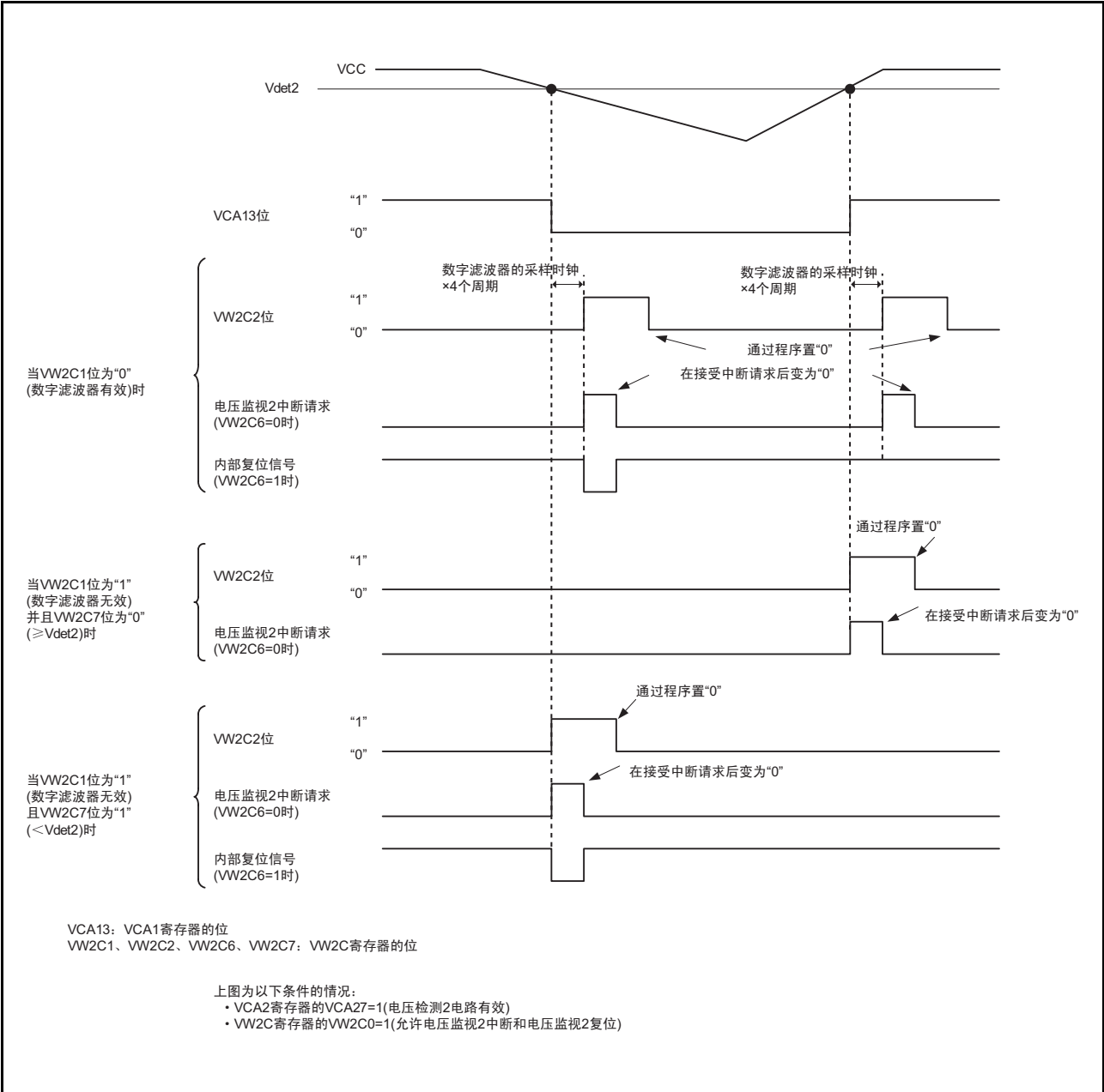
图 7.8 电压监视 2 中断和电压监视 2 复位的运行例子
