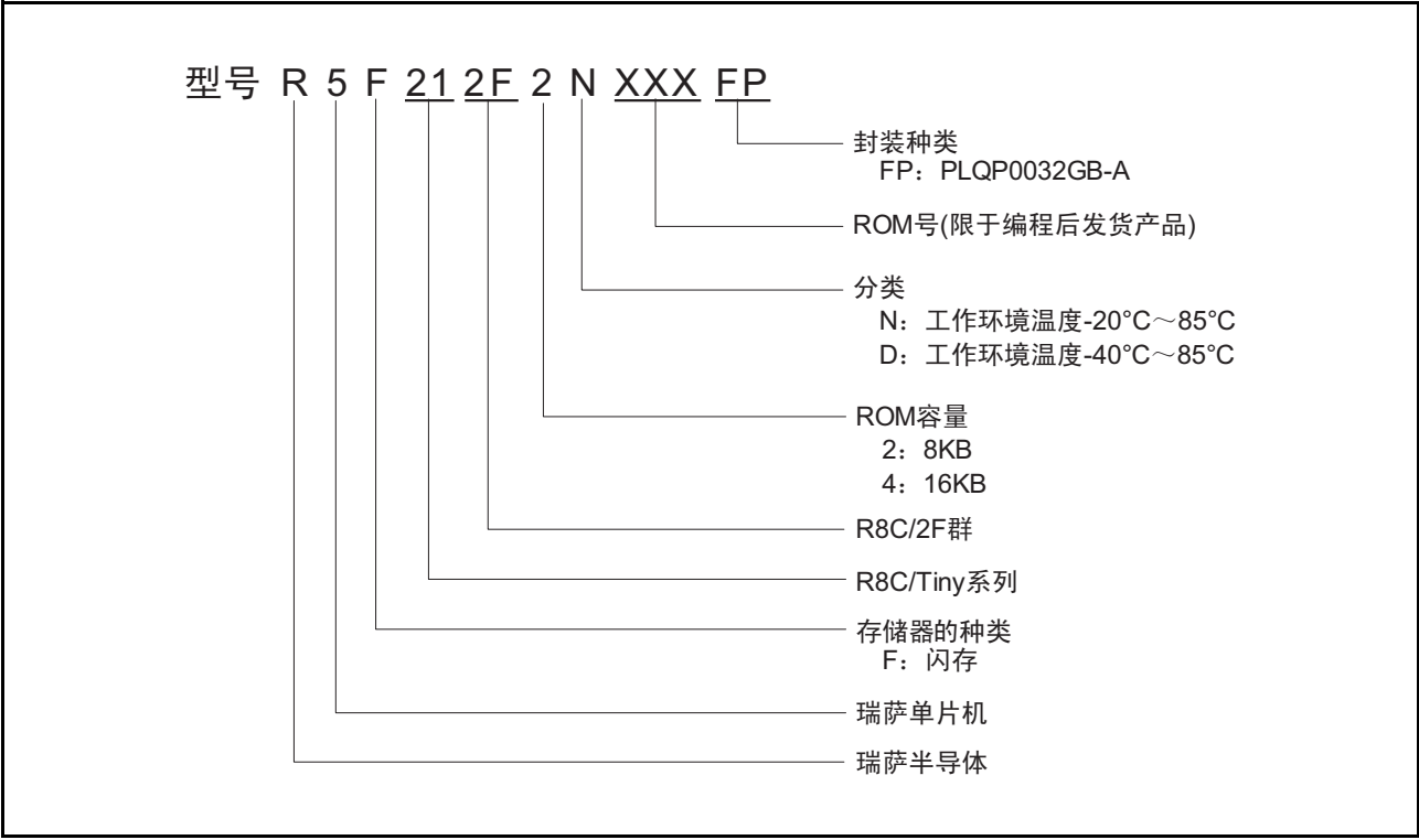
图 1.2 R8C/2F 群的型号和存储器容量及封装
