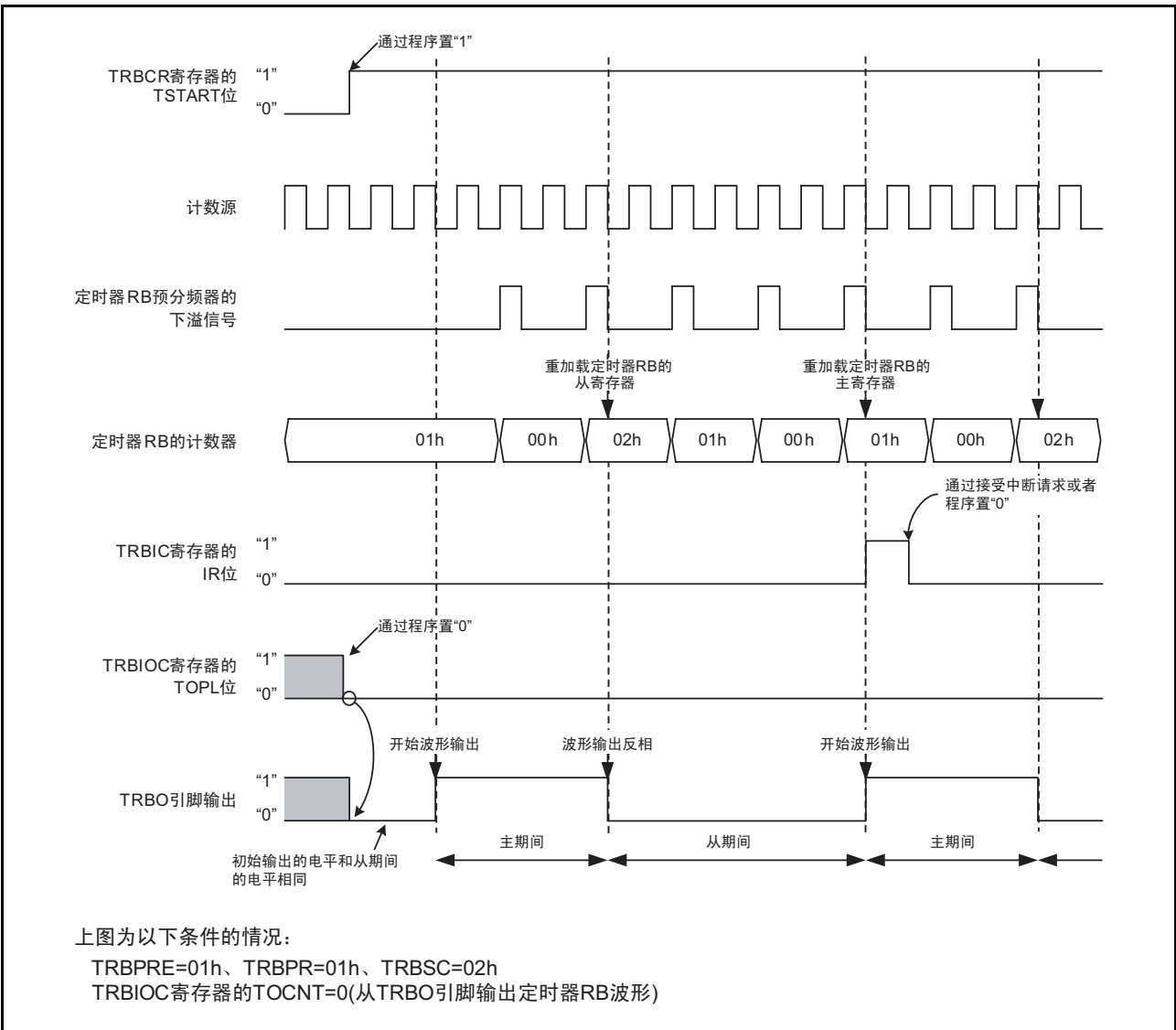
图 15.19 可编程波形发生模式时的定时器 RB 的运行例子
