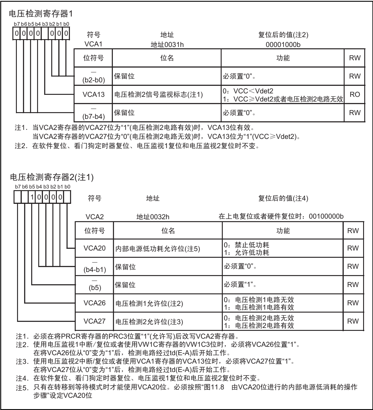
图 7.4 VCA1 和 VCA2 寄存器
