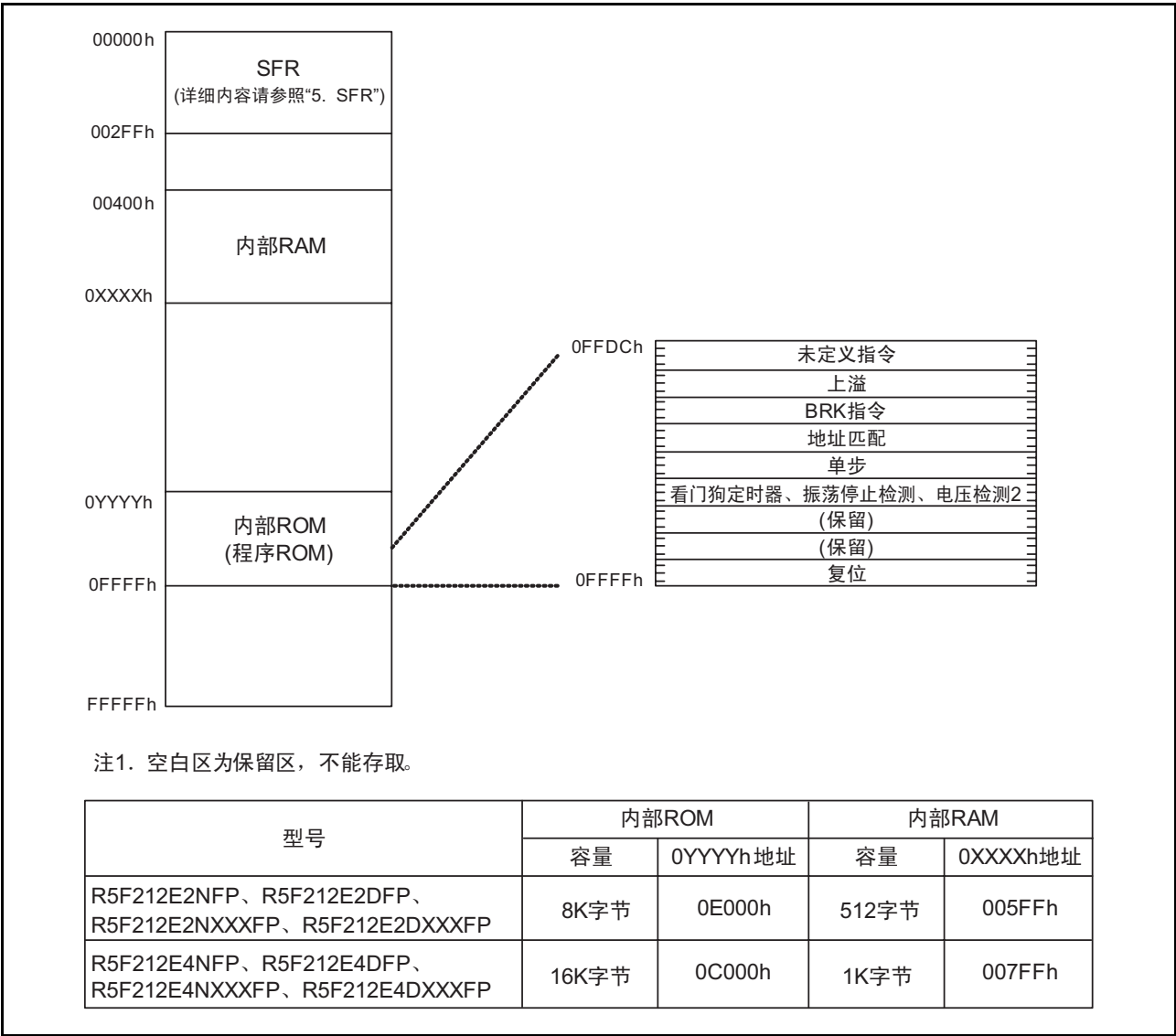
图 4.1 R8C/2E 群的存储器分配图
