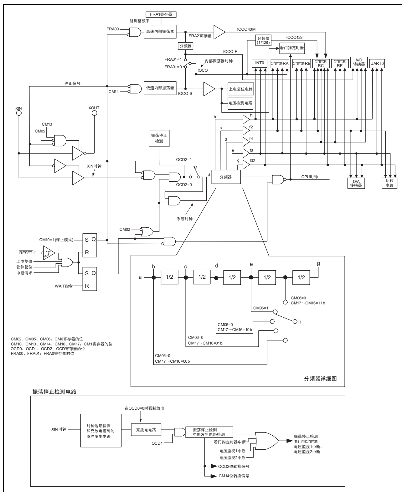
图 11.1 时钟发生电路
