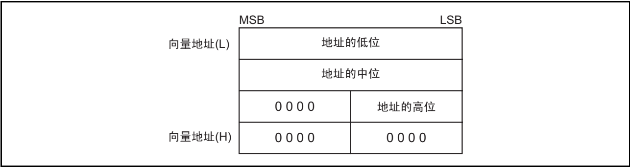
图 13.2 中断向量
