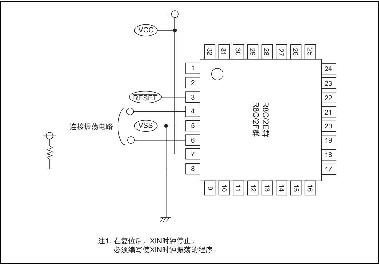
附图 3.1 振荡评价电路例子
