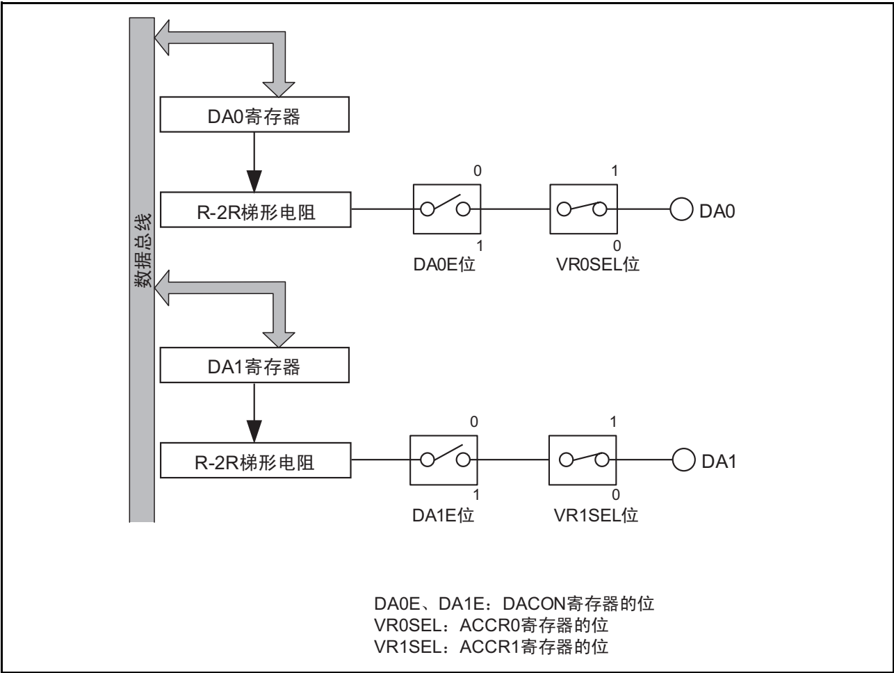
图 19.1 D/A 转换器的框图
