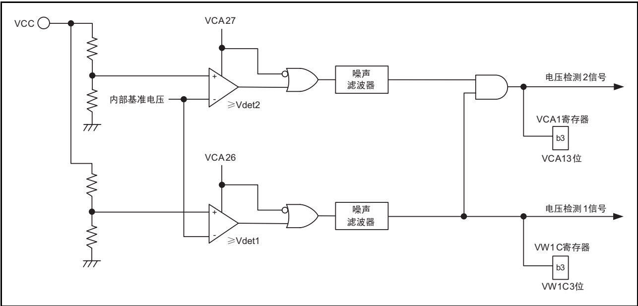
图 7.1 电压检测电路的框图
