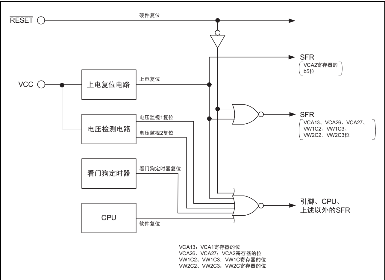
图 6.1 复位电路的框图
