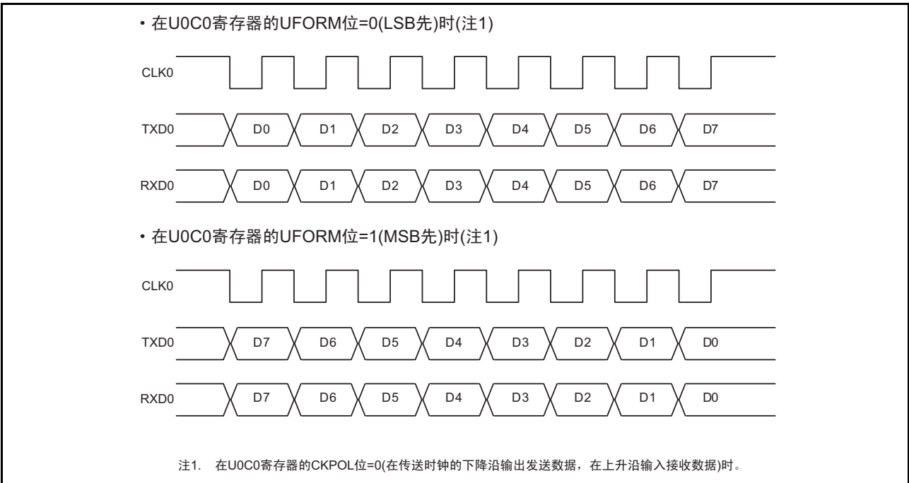
图 16.10 传送格式
