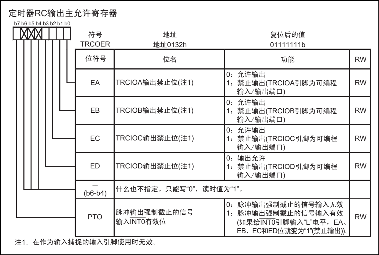
图 15.35 TRCOER 寄存器
