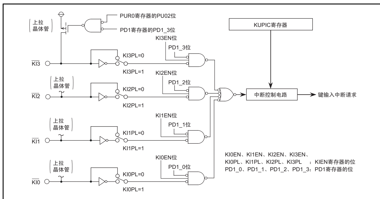
图 13.16 键输入中断的框图
