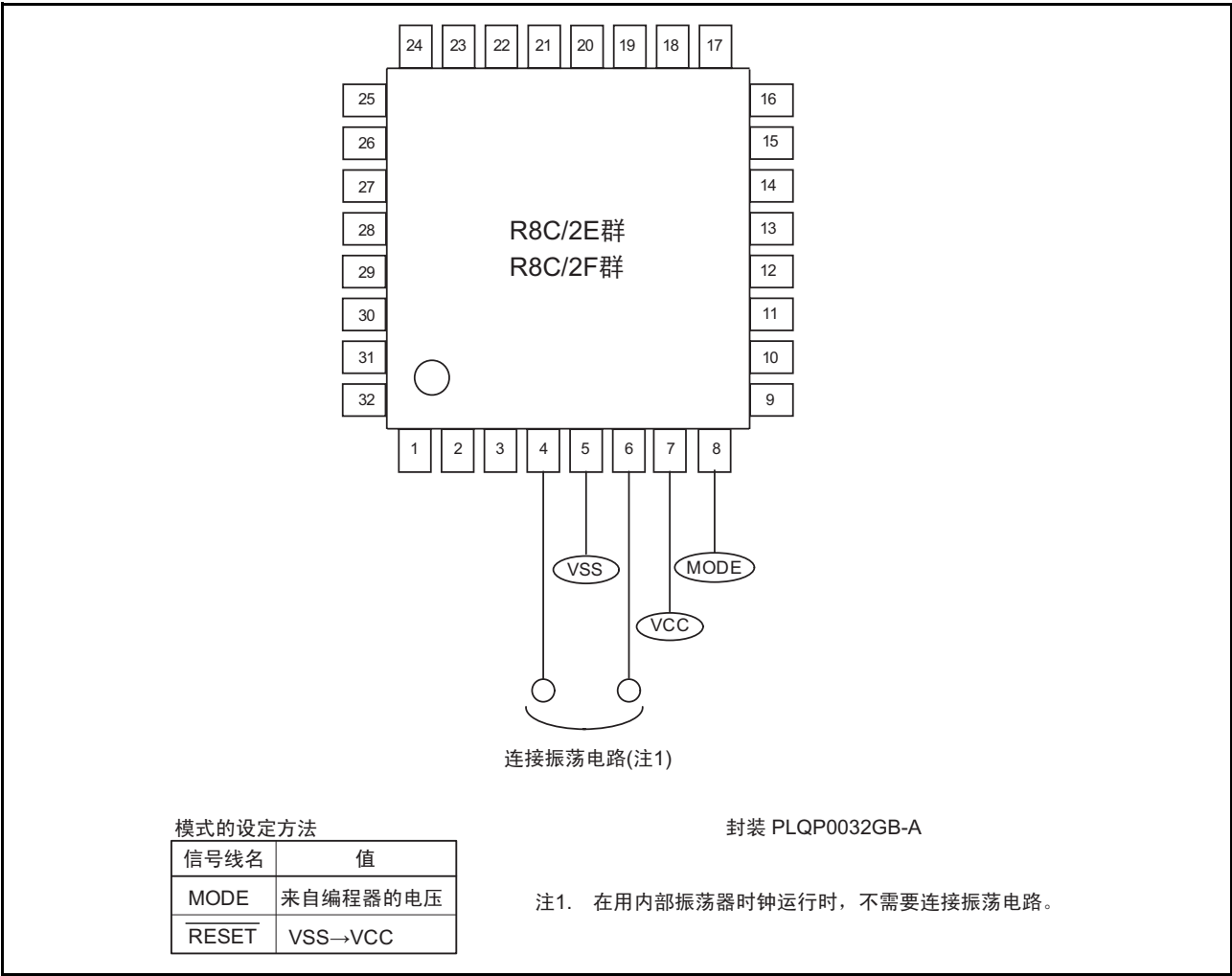
图 21.17 标准串行输入 / 输出模式 3 时的引脚接线图
