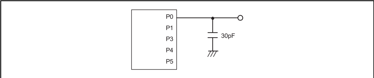
图 22.1 端口 P0、P1、P3 ~ P5 的时序测量电路
