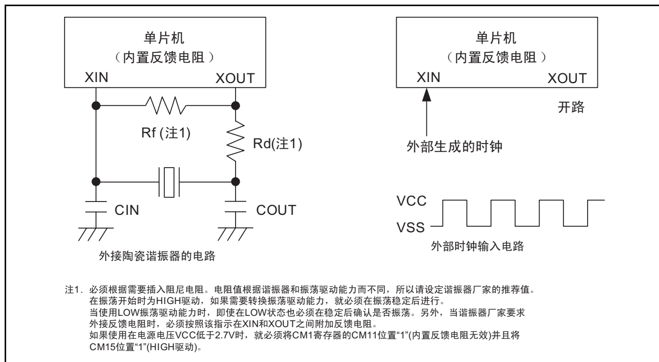
图 11.9 XIN 时钟的连接电路例子
