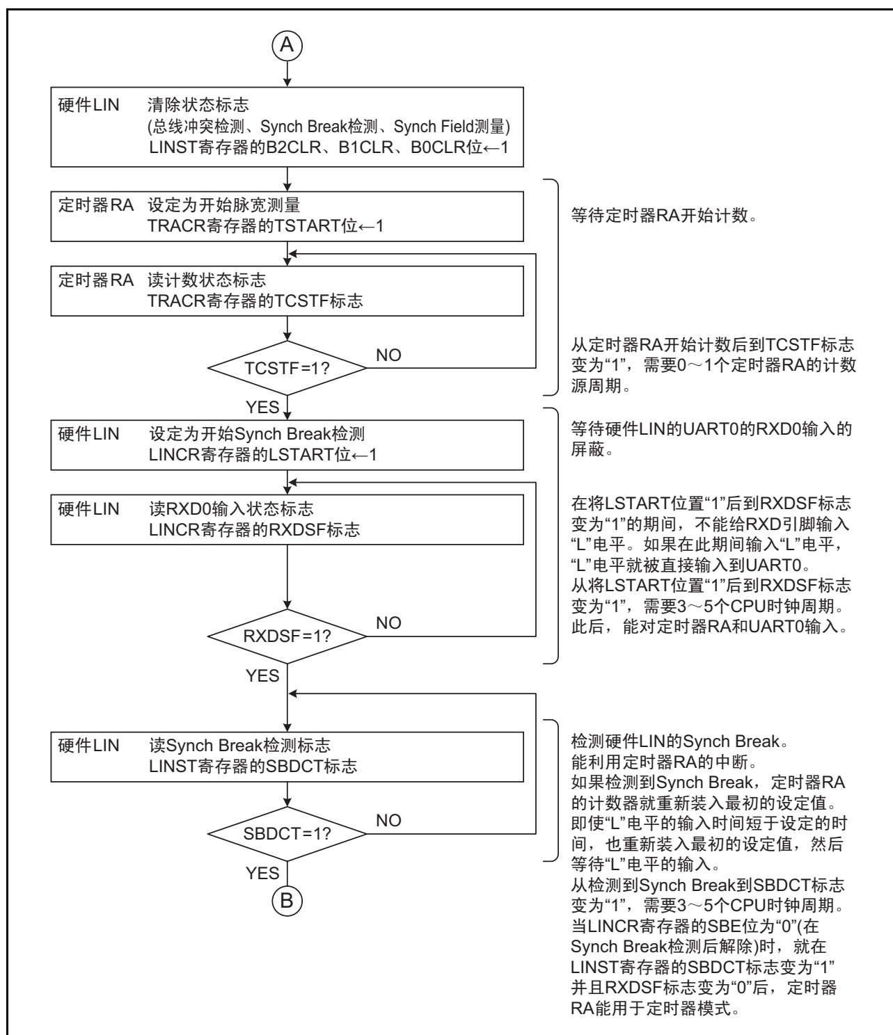
图 17.9 标题段的接收流程图例子 (2)
