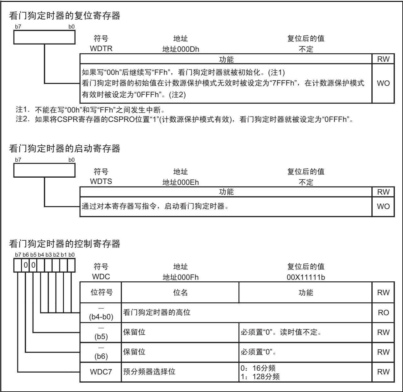
图 14.2 WDTR、WDTS 和 WDC 寄存器
