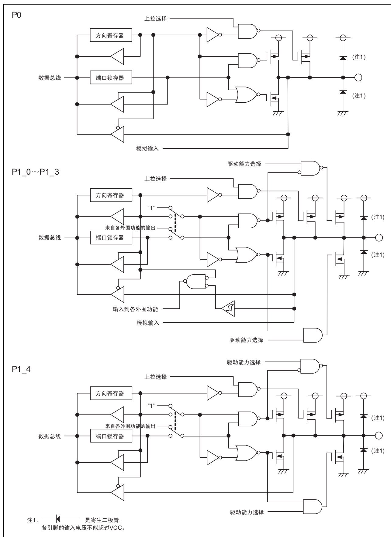
图 8.1 可编程输入 / 输出端口的结构 (1)
