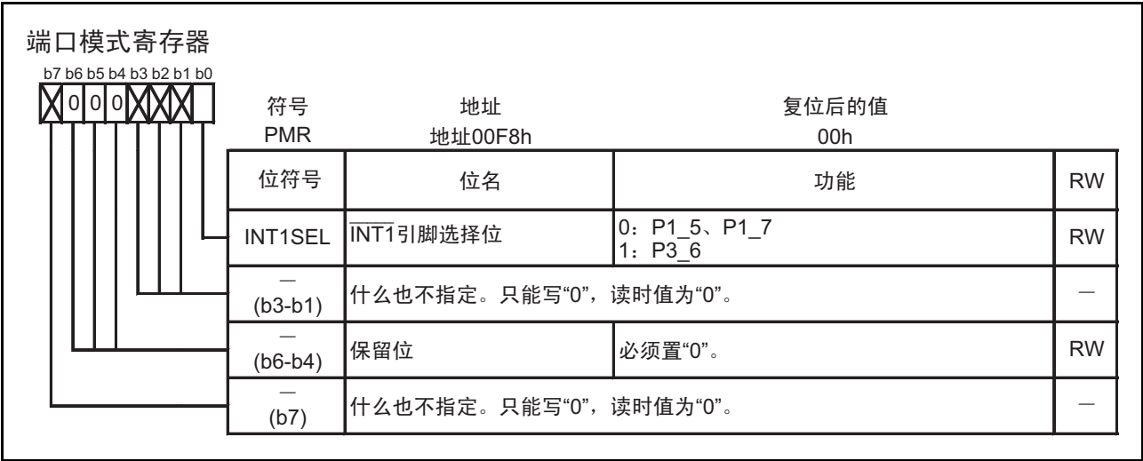
图 16.7 PMR 寄存器
