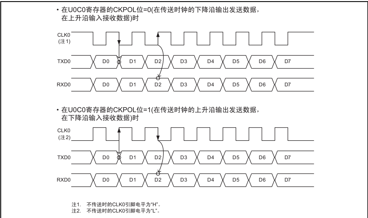
图 16.9 传送时钟的极性
