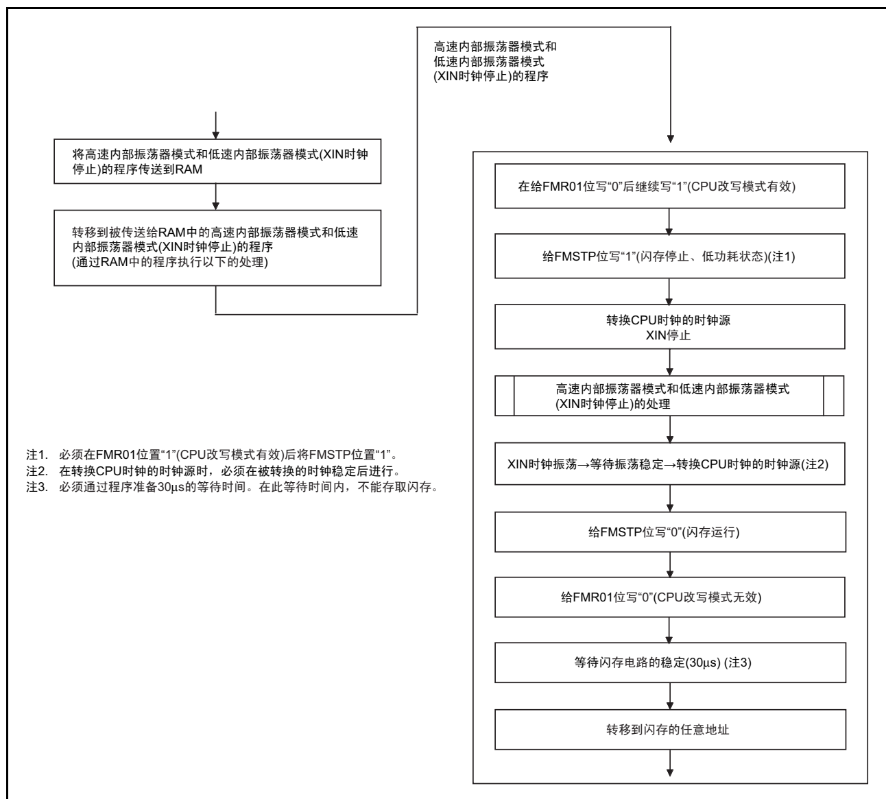
图 21.11 在高速内部振荡器模式和低速内部振荡器模式（XIN 时钟停止）中设定为低功耗的处理
