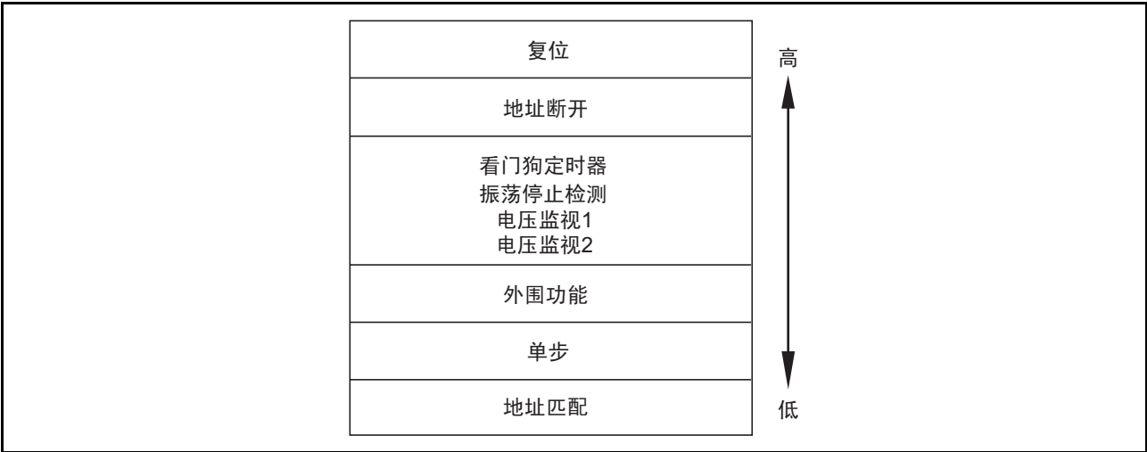
图 13.10 硬件中断的中断优先权
