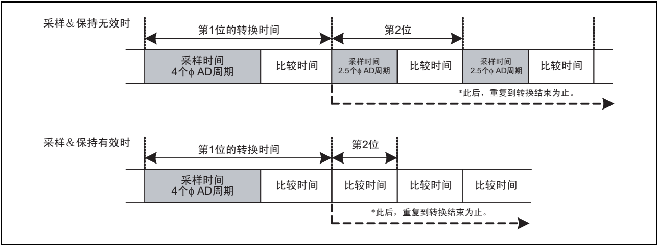
图 18.8 A/D 转换时序图
