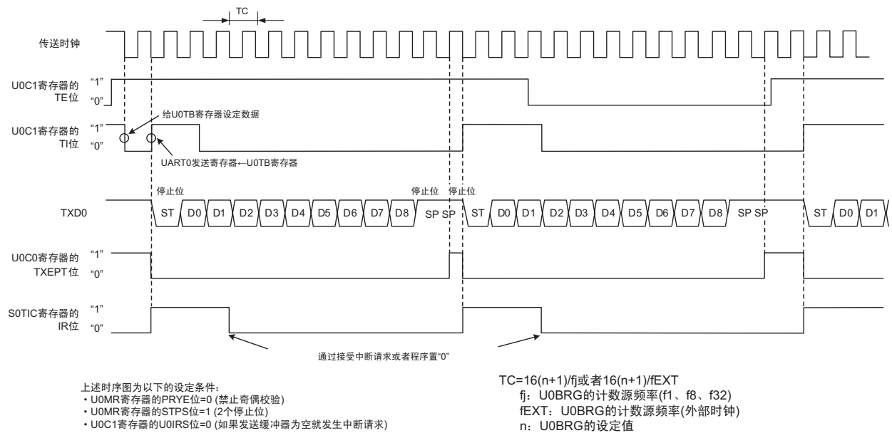
图 16.11 UART 模式时的发送时序例子
