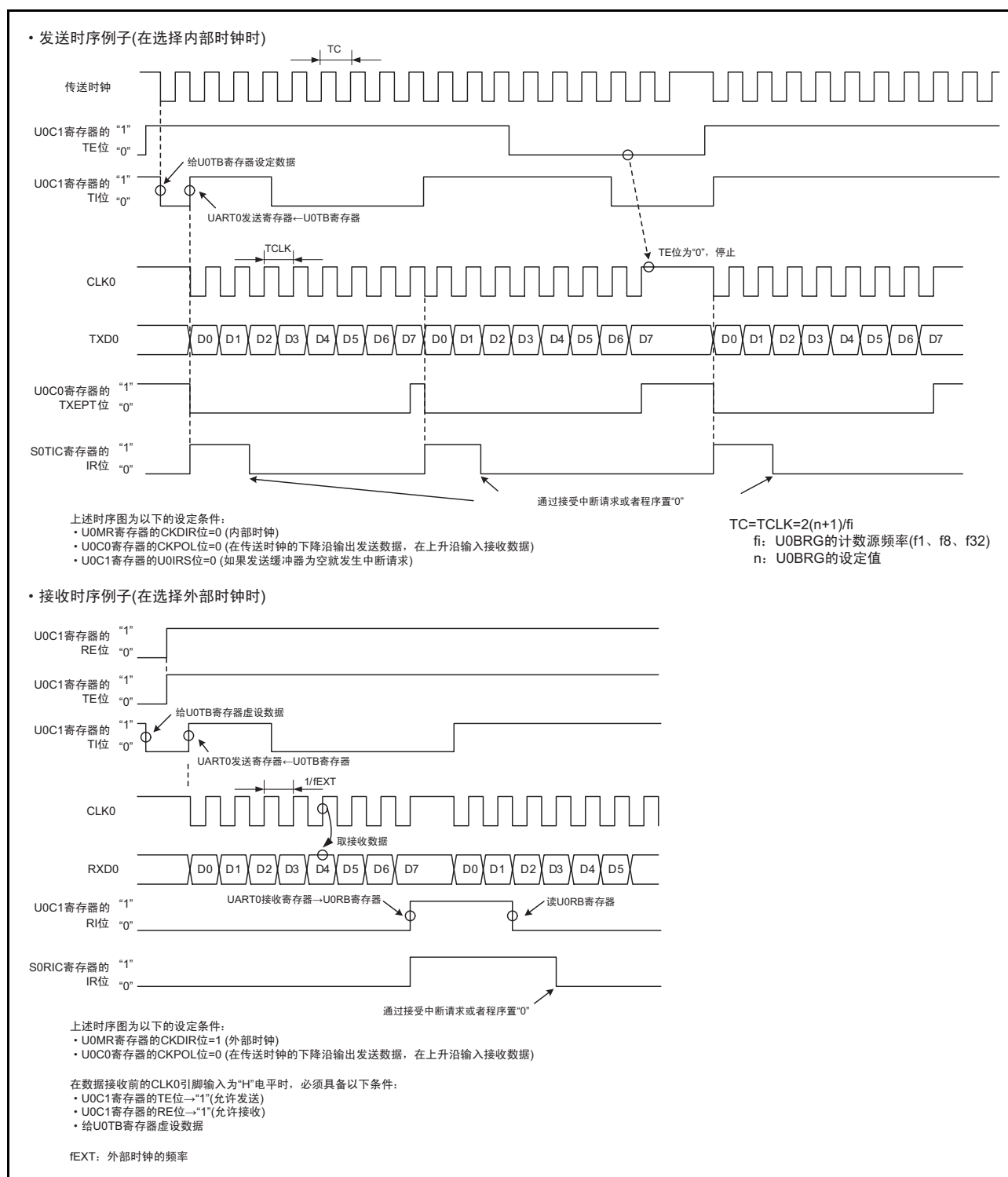
图 16.8 时钟同步串行 I/O 模式时的发送 / 接收时序例子
