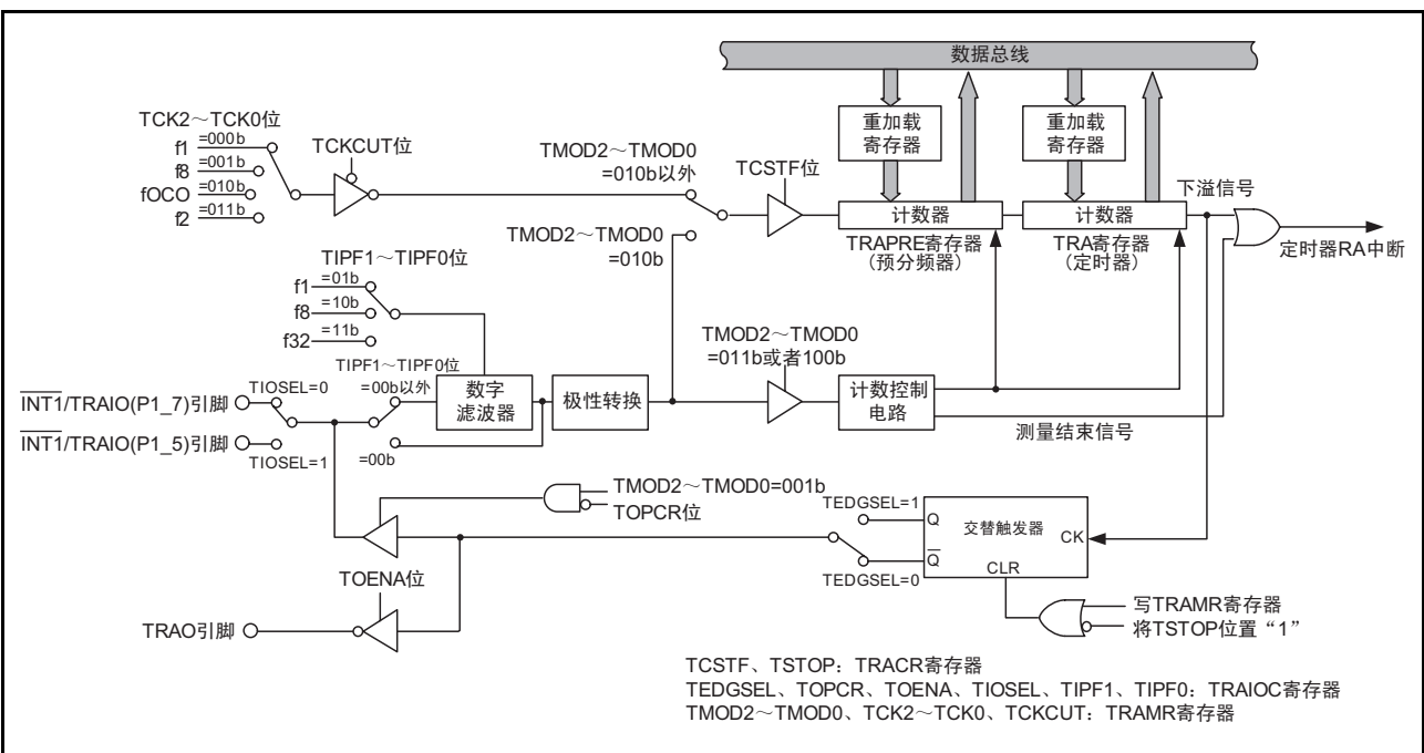
图 15.1 定时器 RA 的框图
