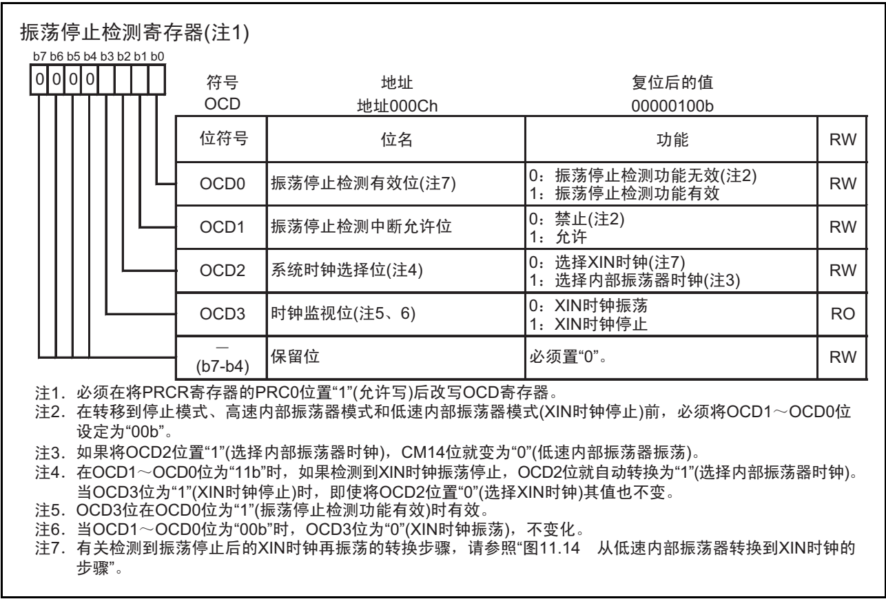
图 11.4 OCD 寄存器
