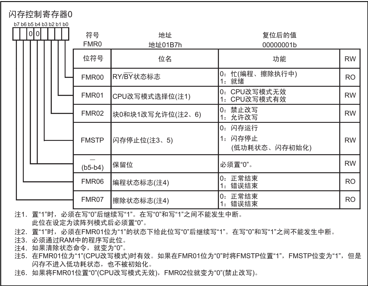
图 21.5 FMR0 寄存器
