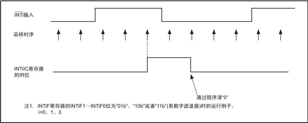
图 13.15 \overline{\text{INT}}i 输入滤波器的运行例子
