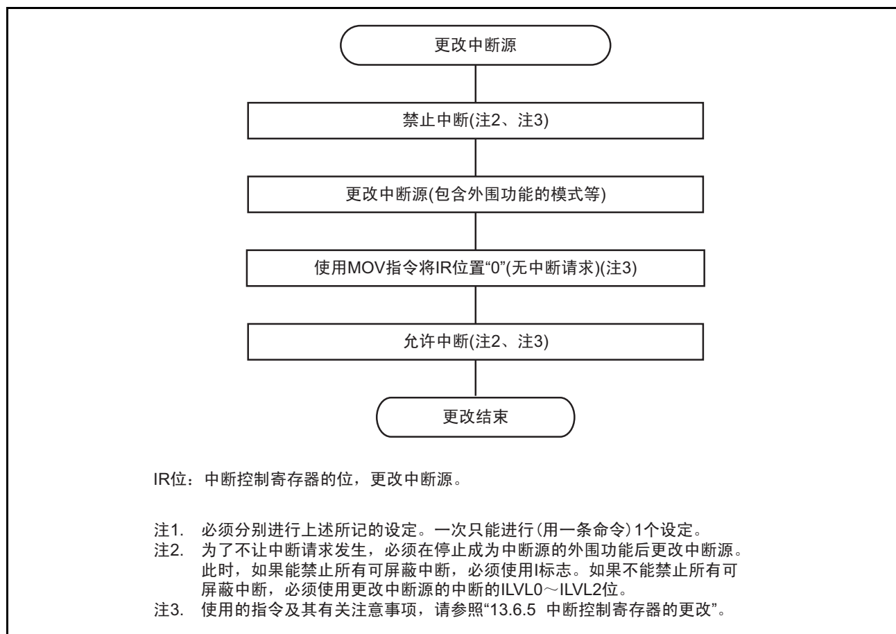
图 13.19 中断源更改步骤的例子
