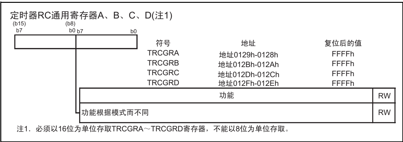
图 15.32 TRCGRA、TRCGRB、TRCGRC 和 TRCGRD 寄存器
