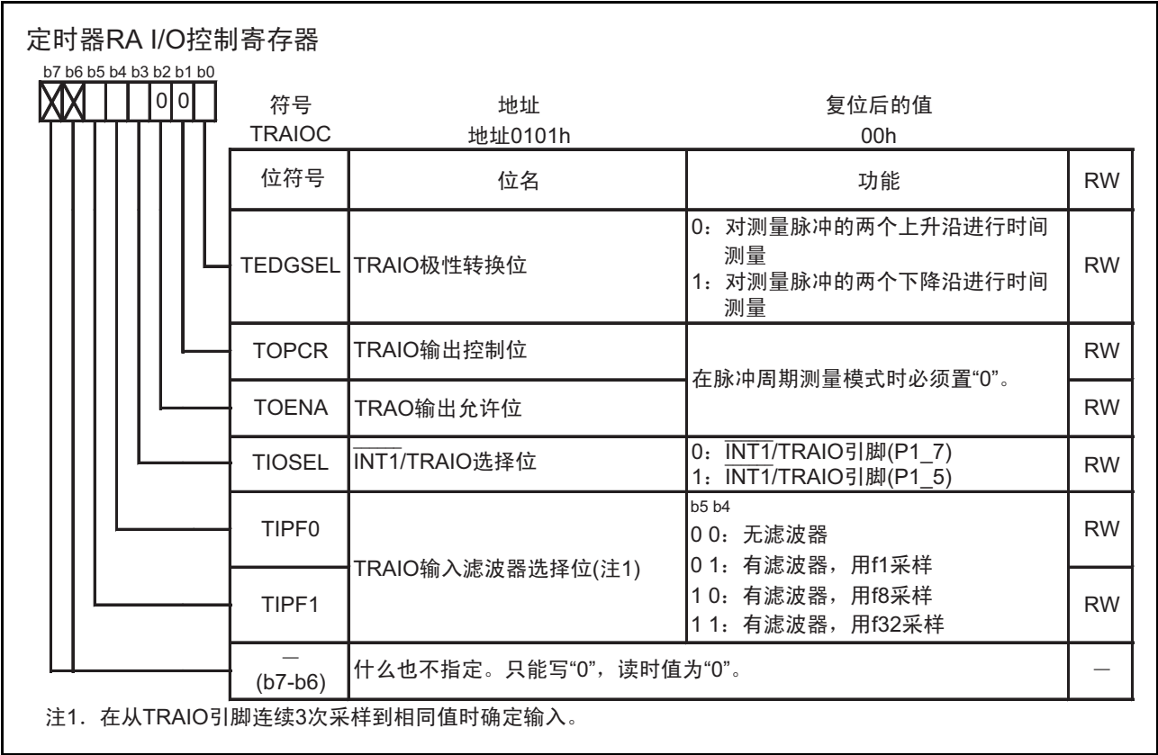
图 15.10 脉冲周期测量模式时的 TRAIOC 寄存器
