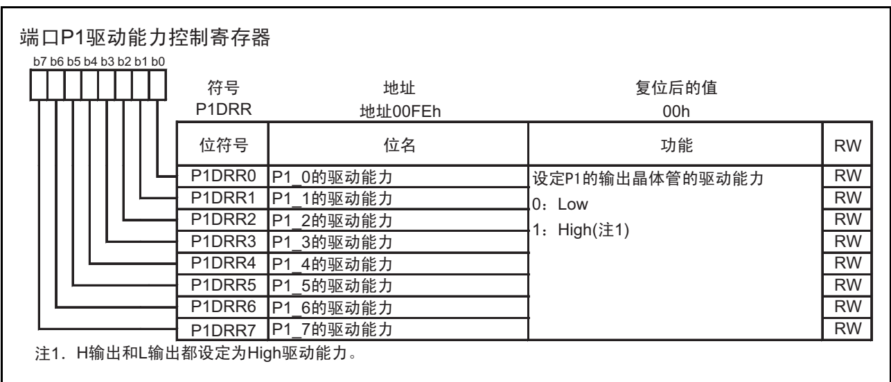
图 8.12 P1DRR 寄存器
