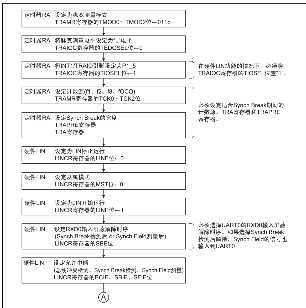
图 17.8 标题段的接收流程图例子 (1)
