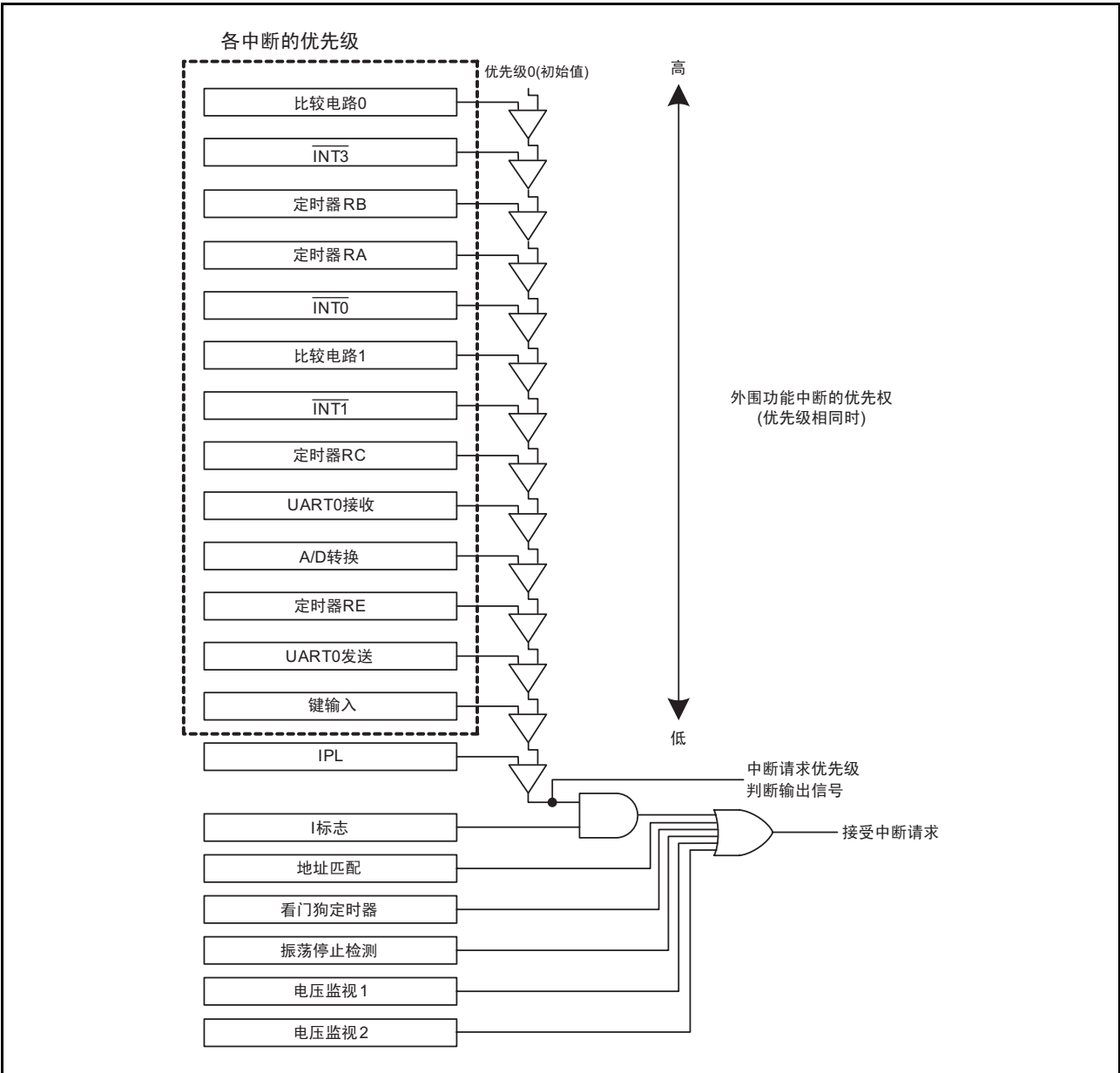
图 13.11 中断优先级判断电路
