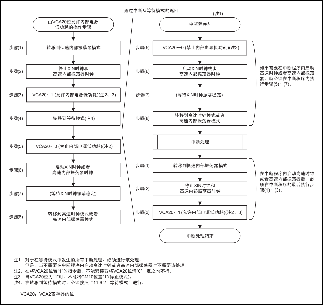
图 11.8 由 VCA20 位进行的内部电源低功耗的操作步骤
