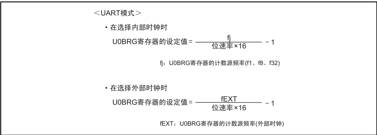
图 16.13 U0BRG 寄存器的设定值的计算式
