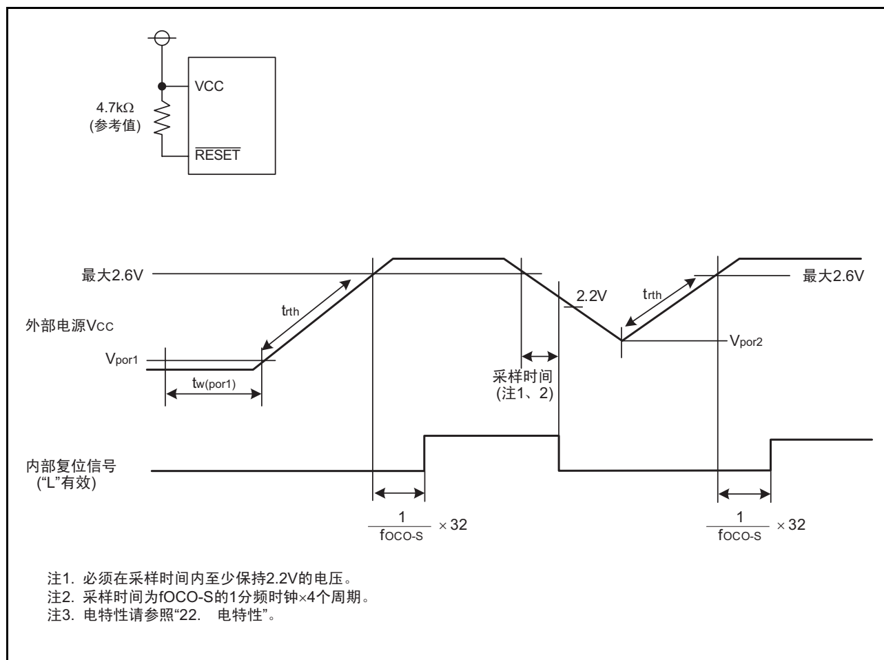
图 6.7 上电复位的电路例子和运行
