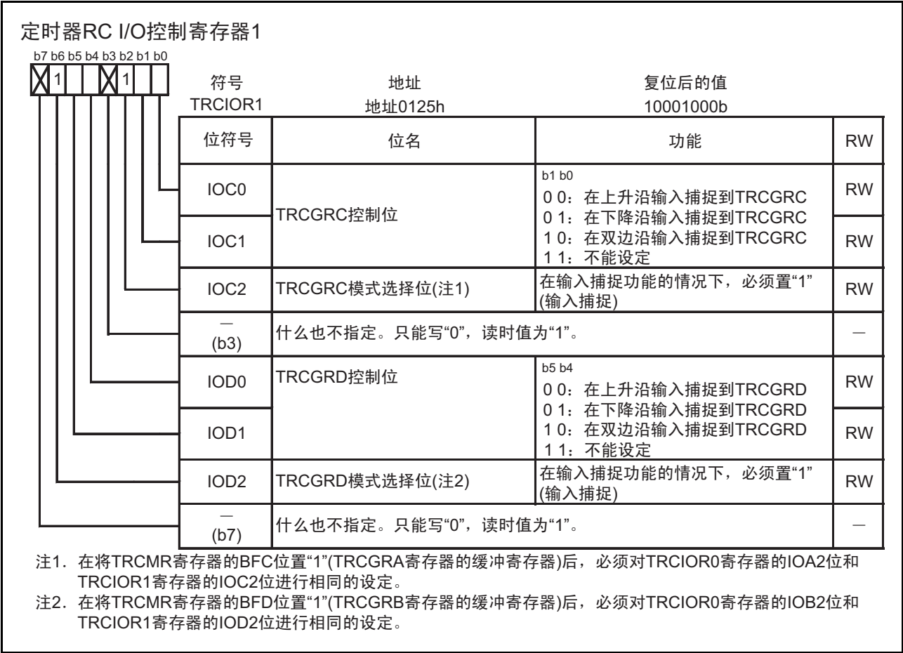
图 15.44 输入捕捉功能时的 TRCIOR1 寄存器
