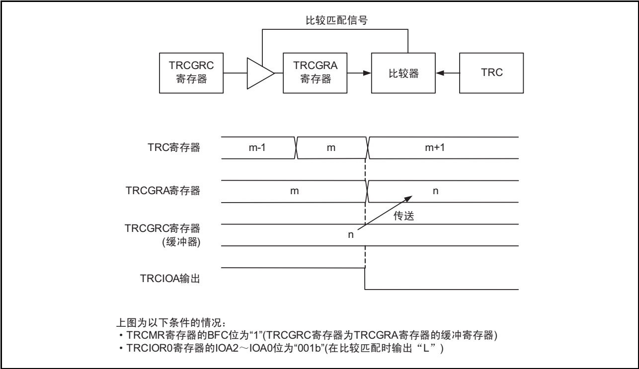
图 15.39 输出比较功能的缓冲器运行
