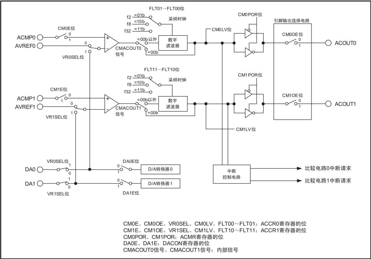
图 20.1 比较电路的框图
