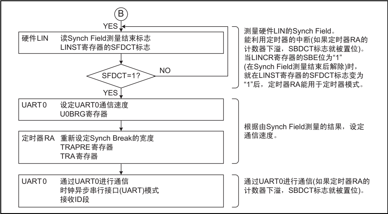
图 17.10 标题段的接收流程图例子 (3)
