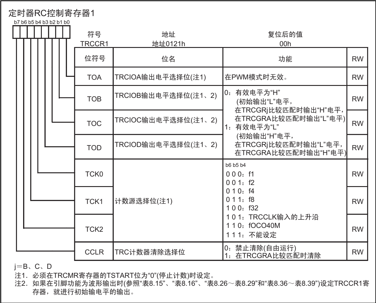
图 15.52 PWM 模式时的 TRCCR1 寄存器
