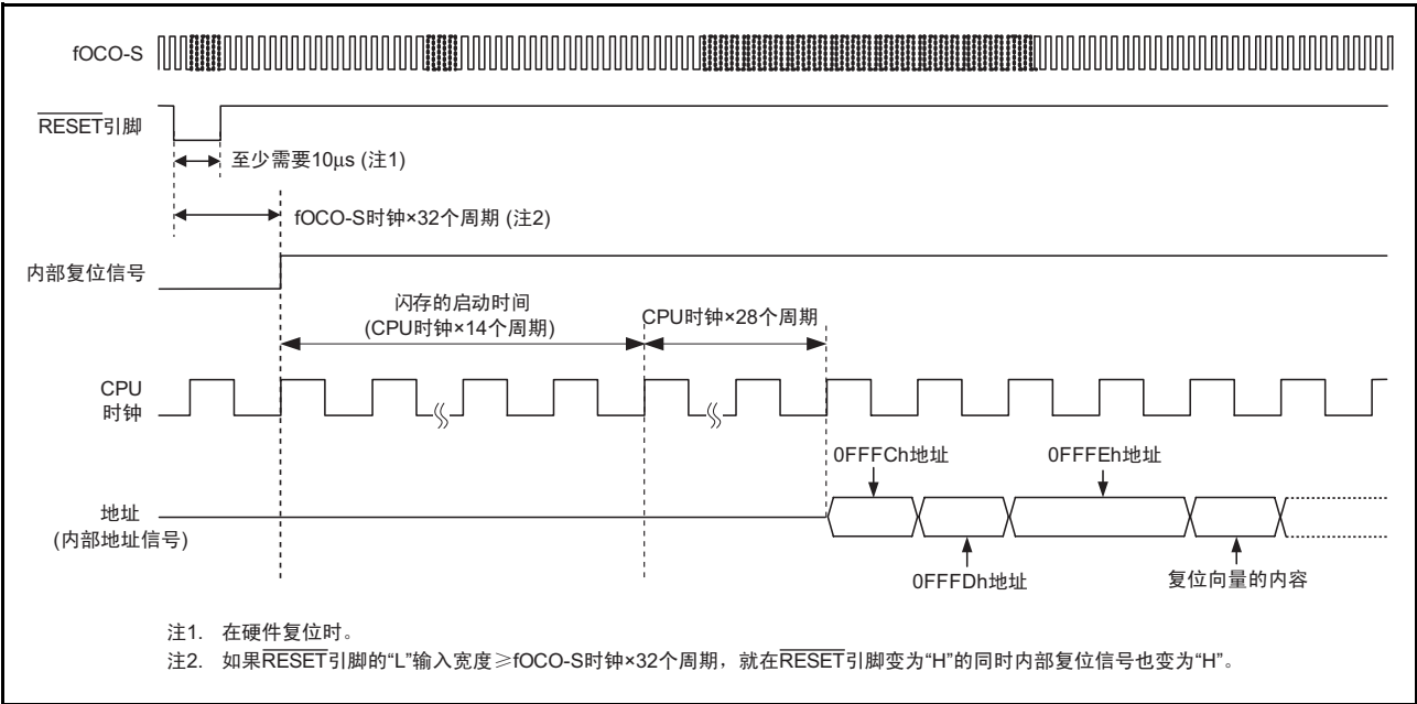
图 6.3 复位顺序
