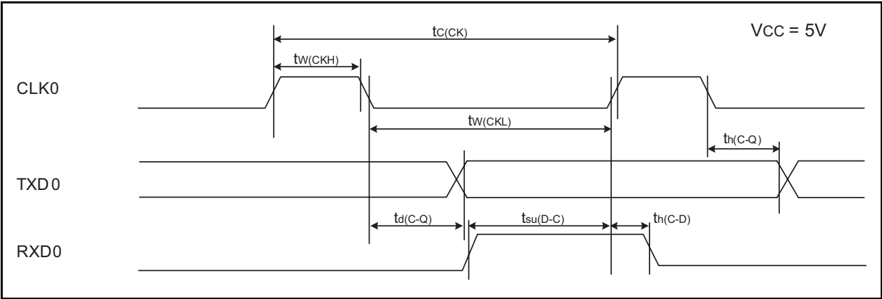
图 22.6 V_{CC}=5V 时的串行接口时序
