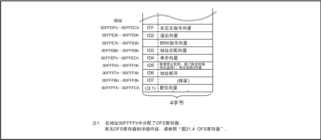
图 21.3 ID 码的保存地址
