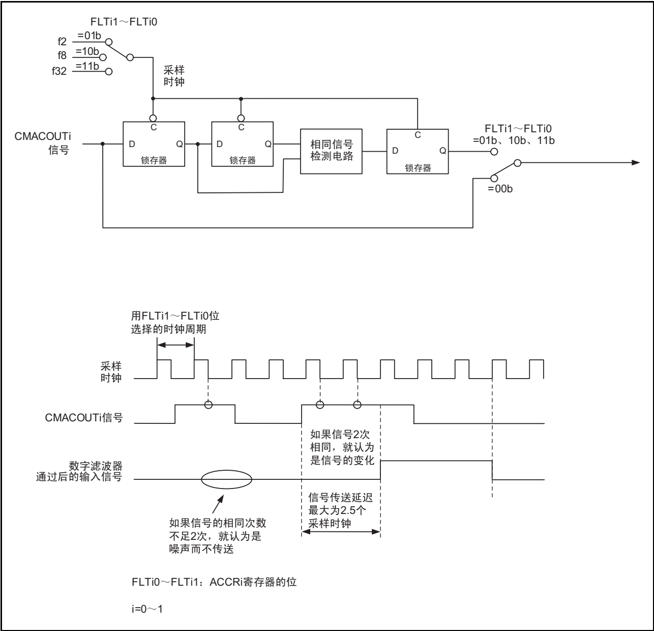
图 20.5 数字滤波器的框图
