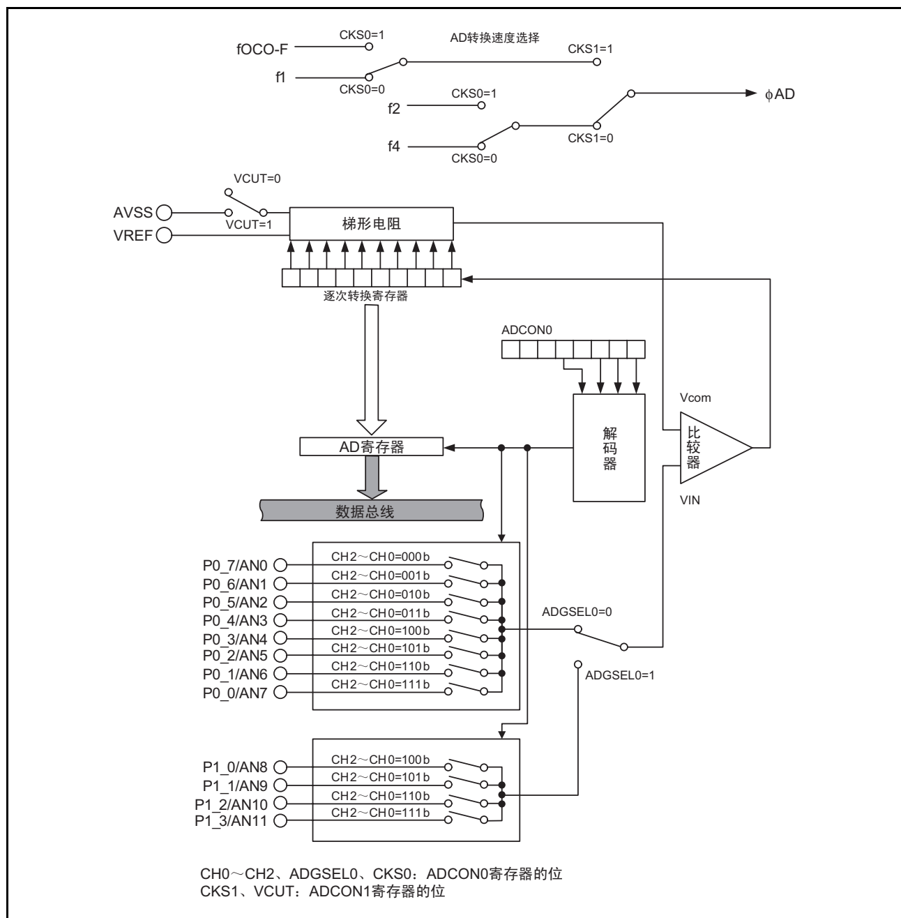
图 18.1 A/D 转换器的框图
