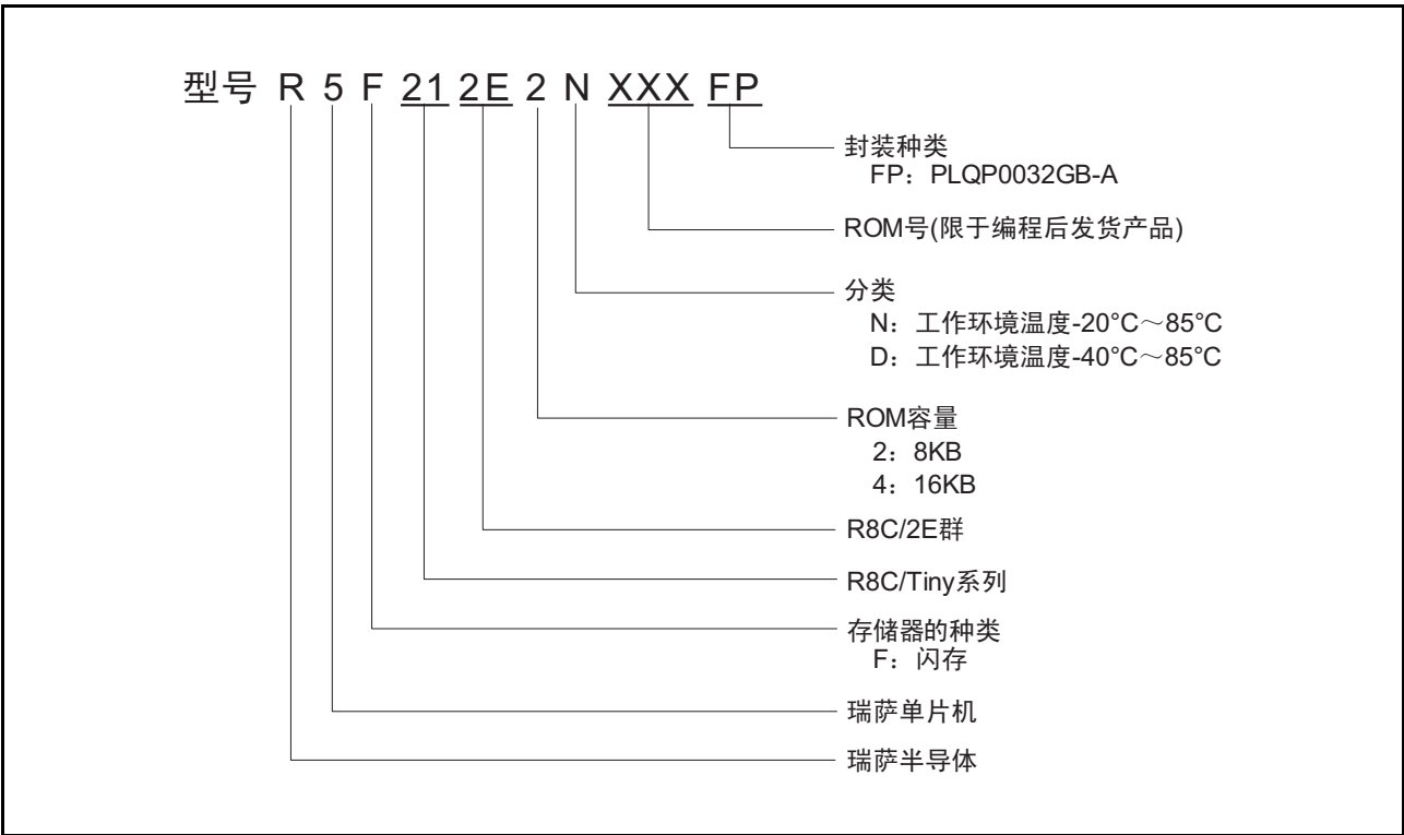
图 1.1 R8C/2E 群的型号和存储器容量及封装
