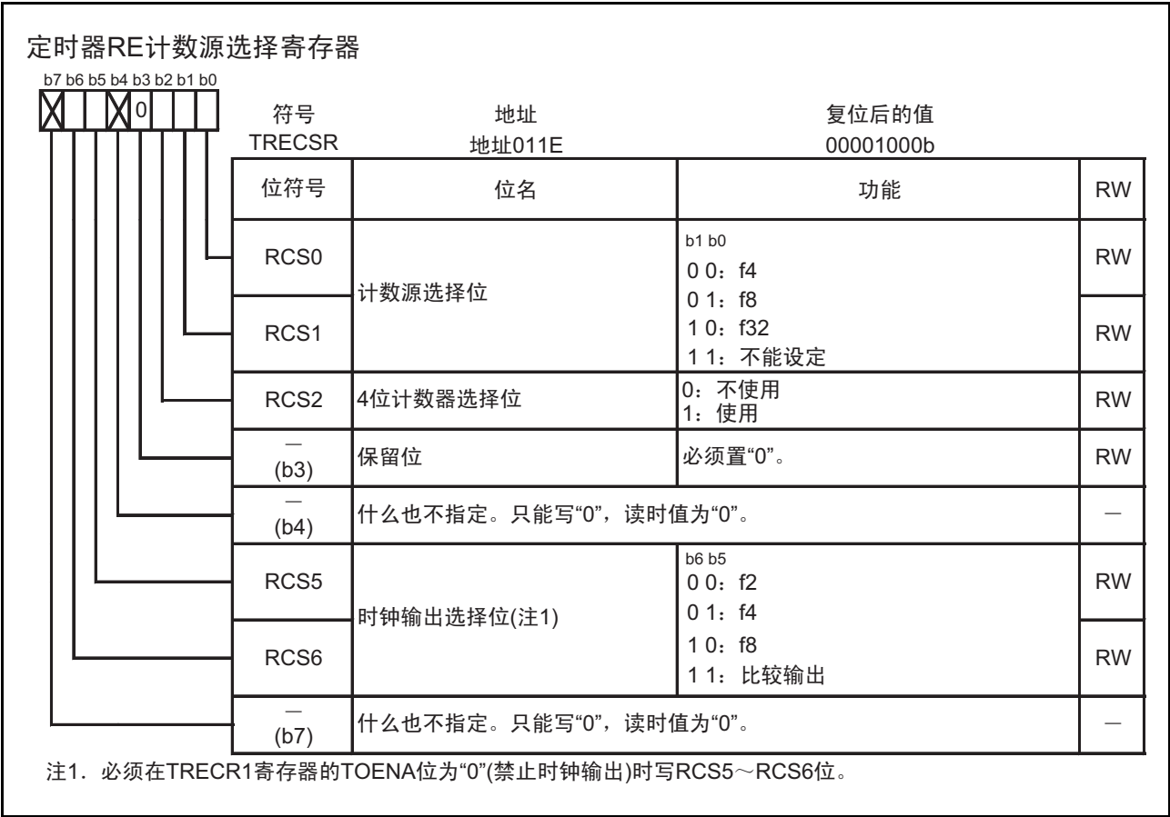
图 15.66 输出比较模式时的 TRECSR 寄存器
