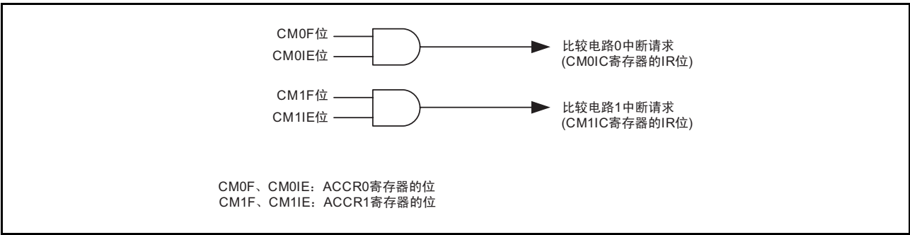
图 20.6 比较电路中断的框图
