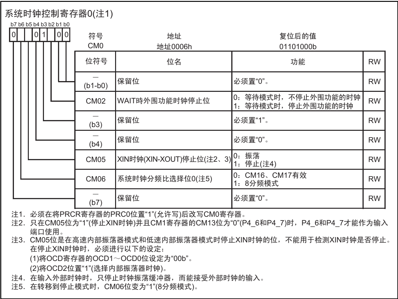
图 11.2 CM0 寄存器
