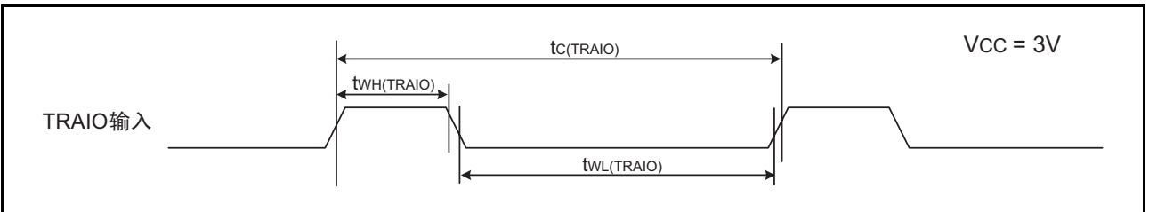
图 22.9 V_{CC}=3V 时的 TRAIO 输入时序
