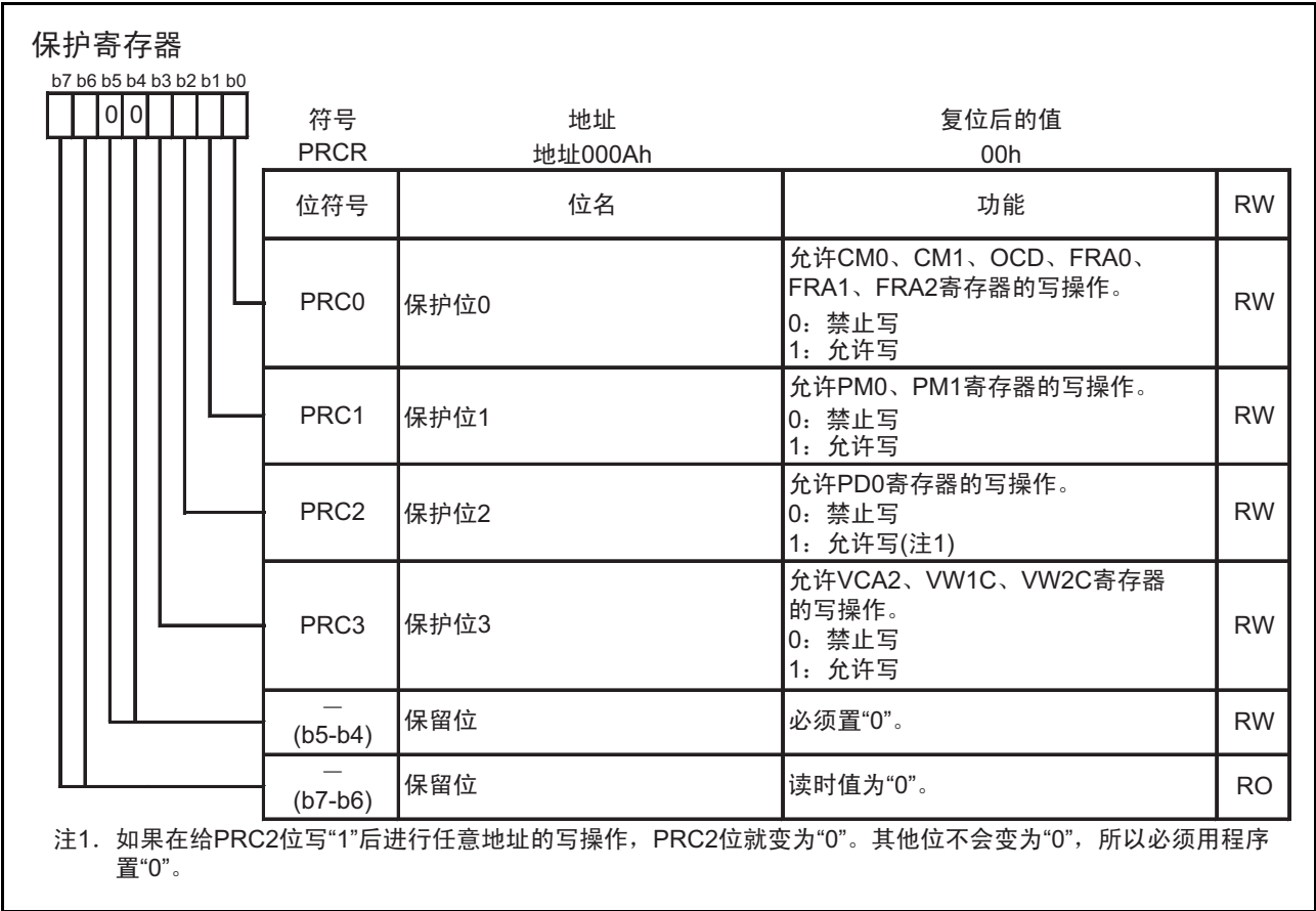
图 12.1 PRCR 寄存器
