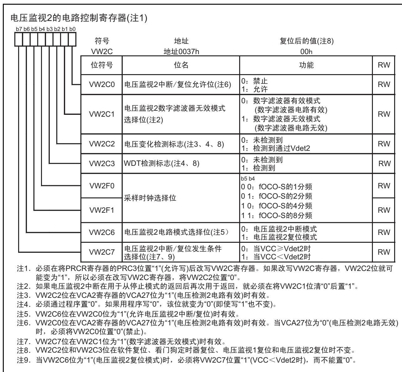
图 7.6 VW2C 寄存器
