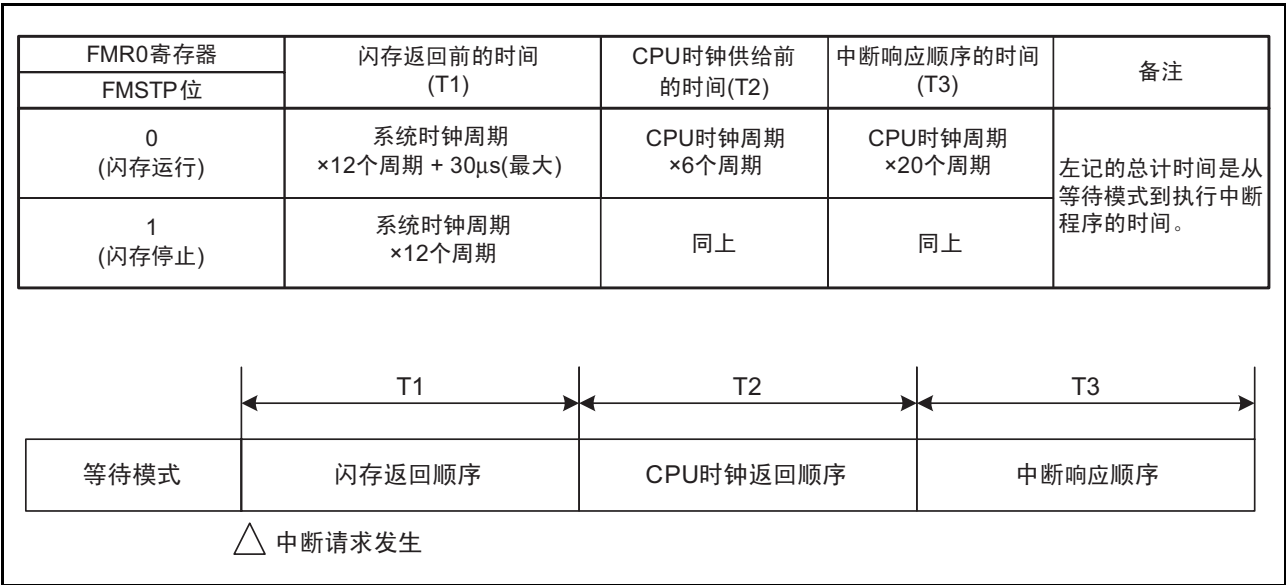
图 11.10 从等待模式到执行中断程序的时间
