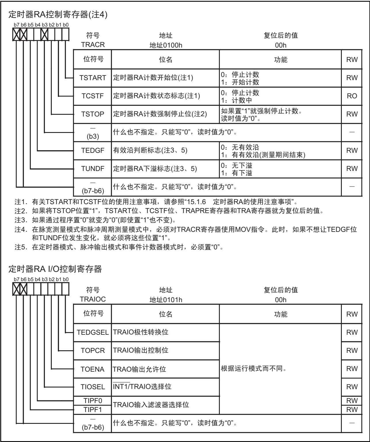
图 15.2 TRACR 和 TRAIOC 寄存器
