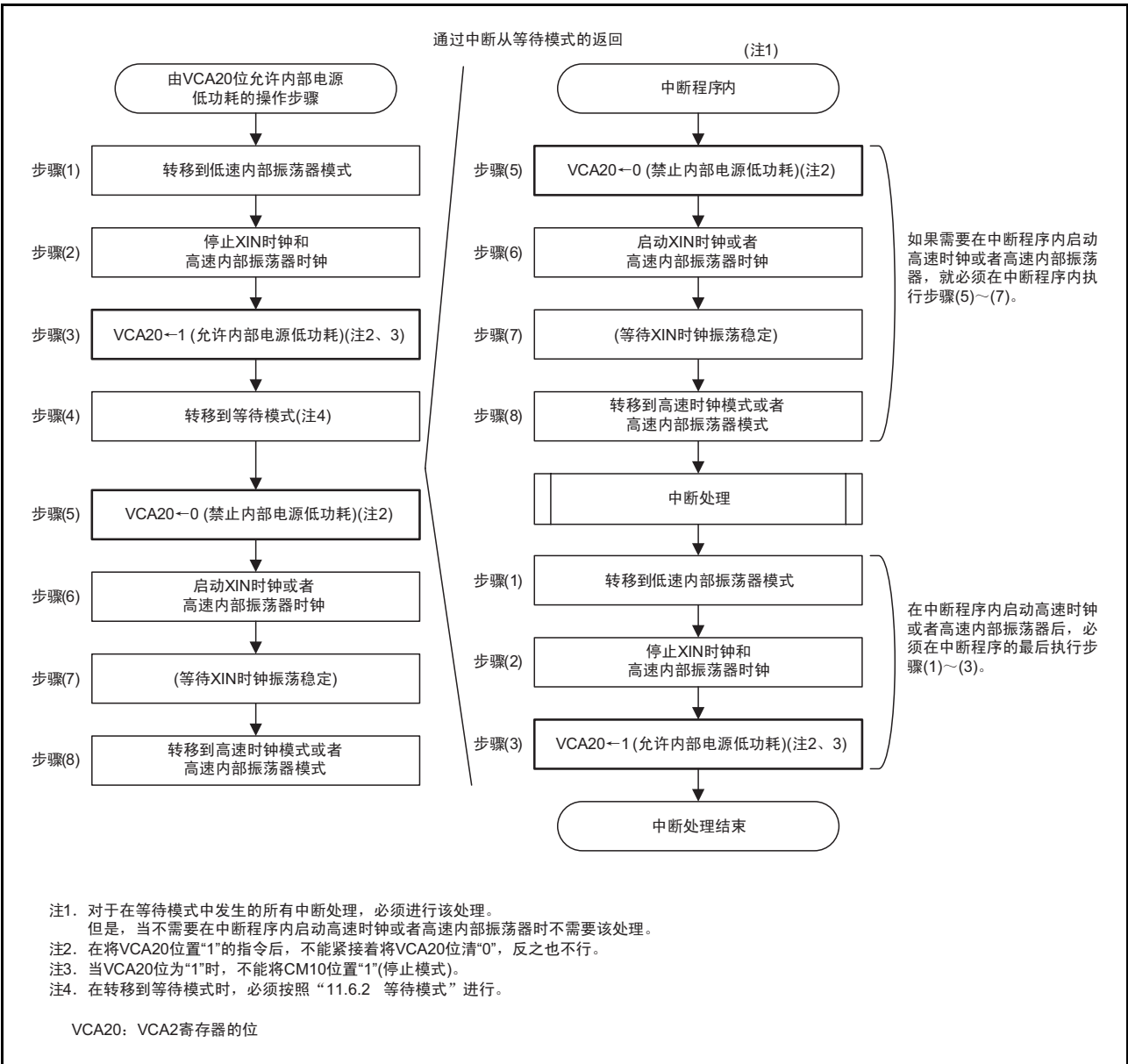
图 11.11 由 VCA20 位进行的内部电源低功耗的操作步骤
