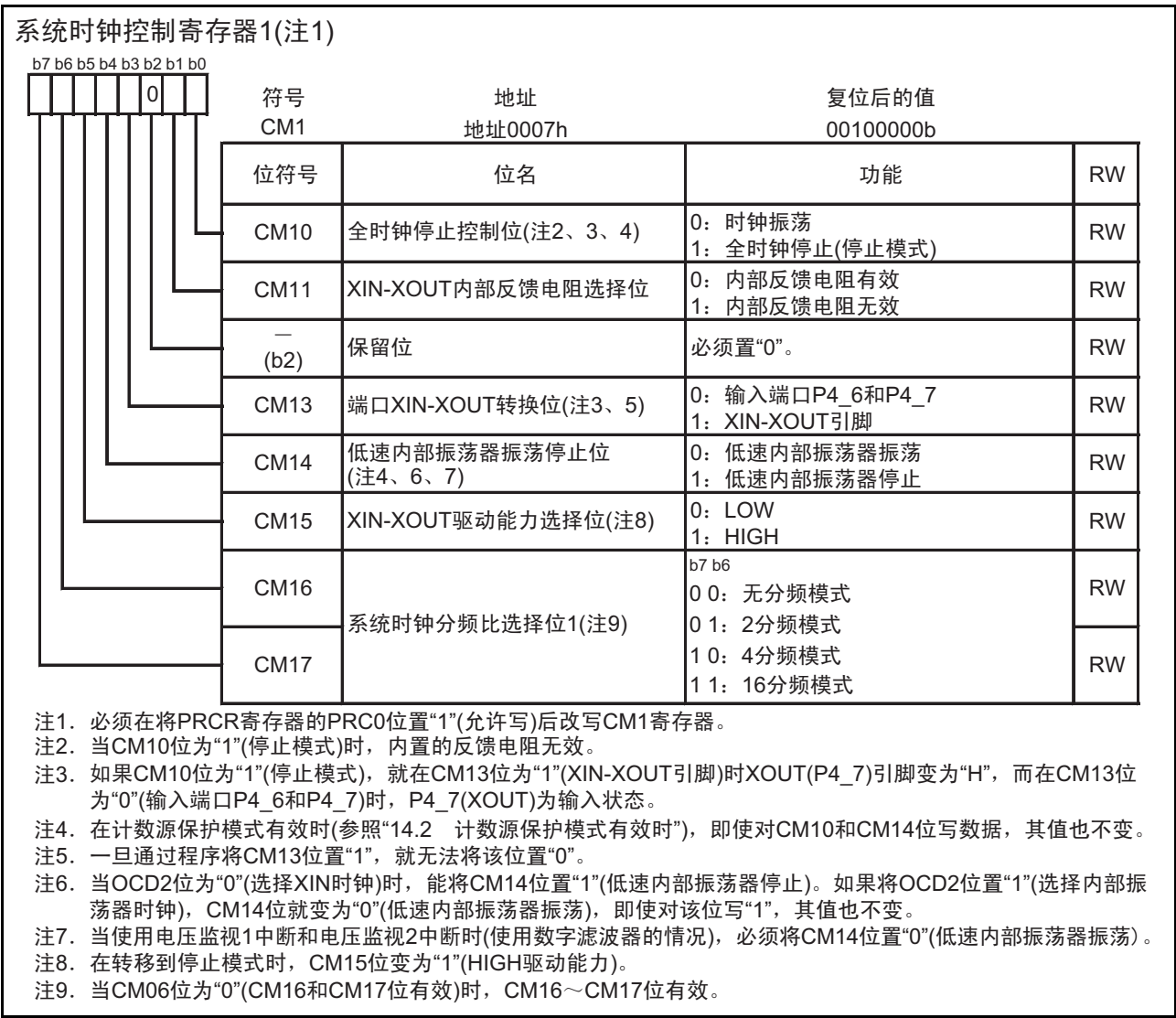
图 11.3 CM1 寄存器
