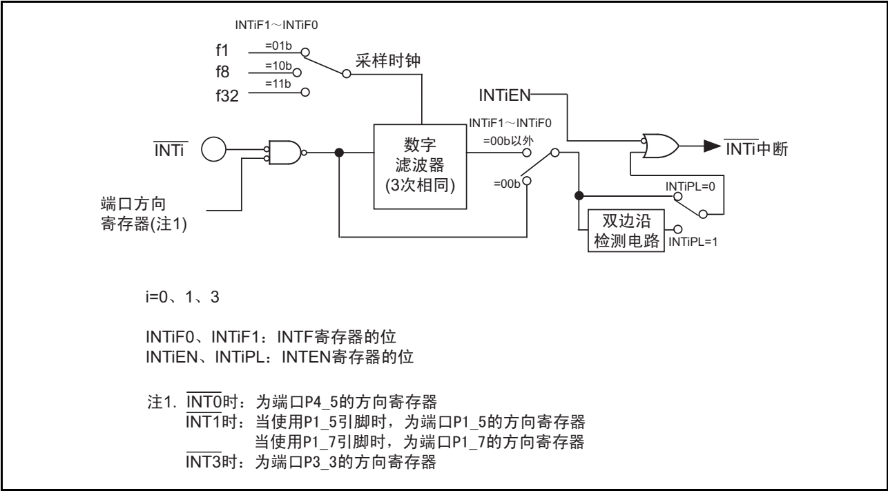
图 13.14 \overline{\text{INT}}i 输入滤波器的结构
