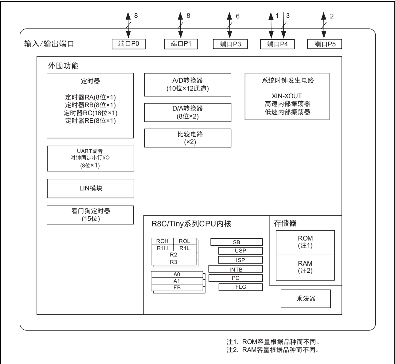
图 1.3 框图
