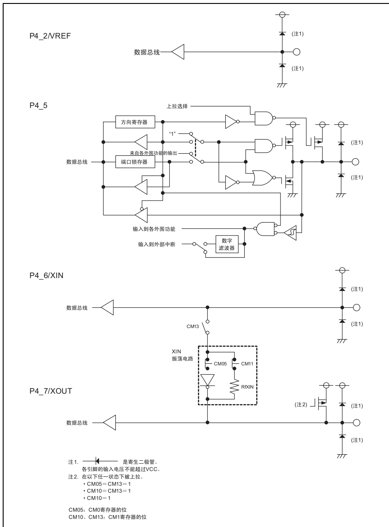
图 8.4 可编程输入 / 输出端口的结构 (4)
