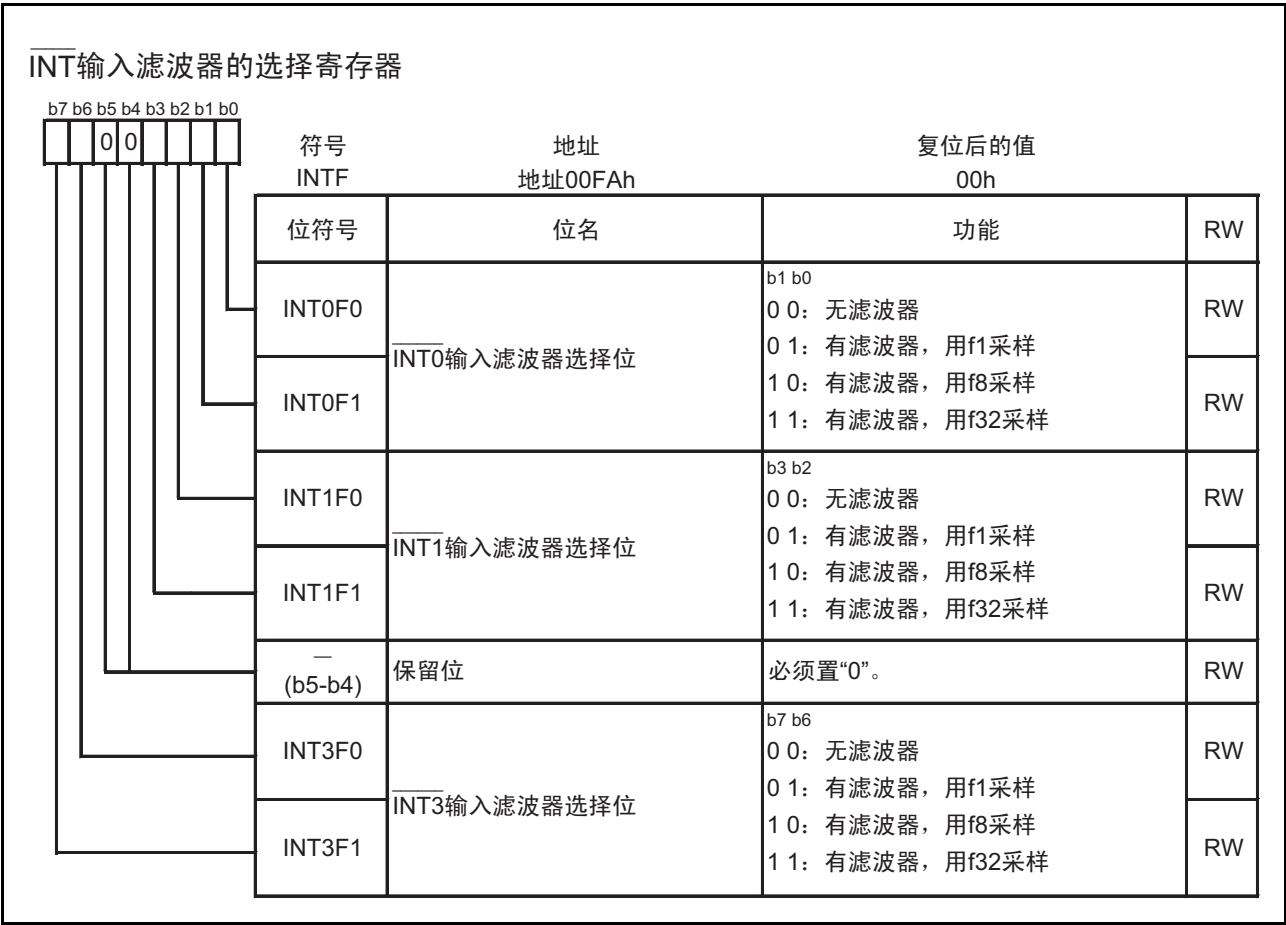
图 13.13 INTF 寄存器
