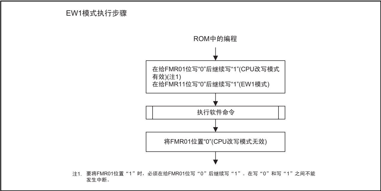
图 21.10 EW1 模式的设定和解除方法
