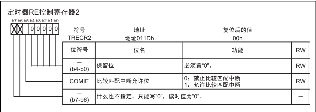
图 15.65 输出比较模式时的 TRECR2 寄存器
