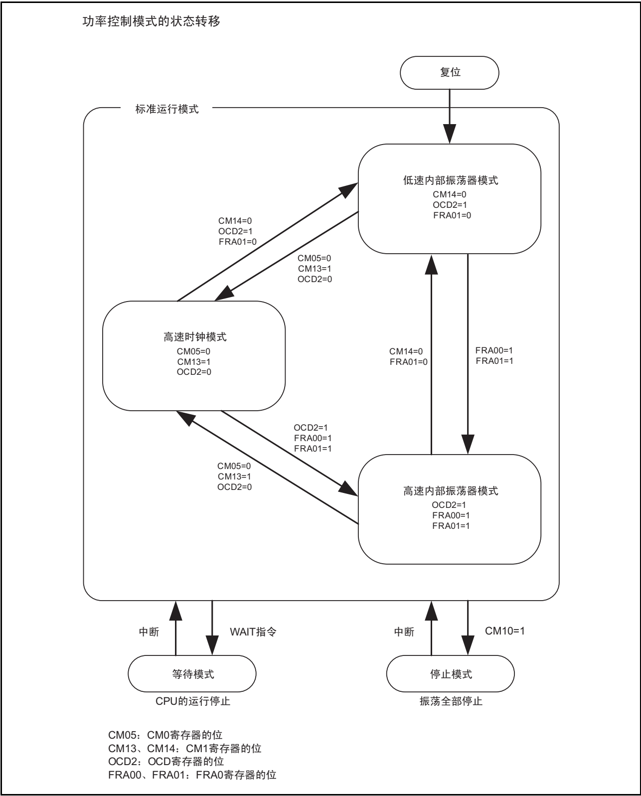
图 11.13 功率控制的状态转移
