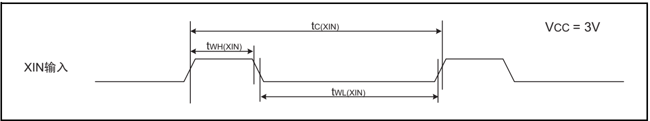
图 22.8 V_{CC}=3V 时的 XIN 输入时序
