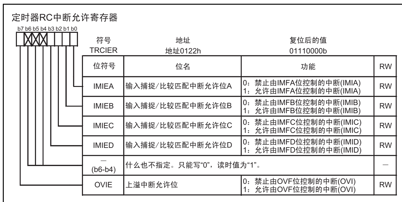
图 15.29 TRCIER 寄存器
