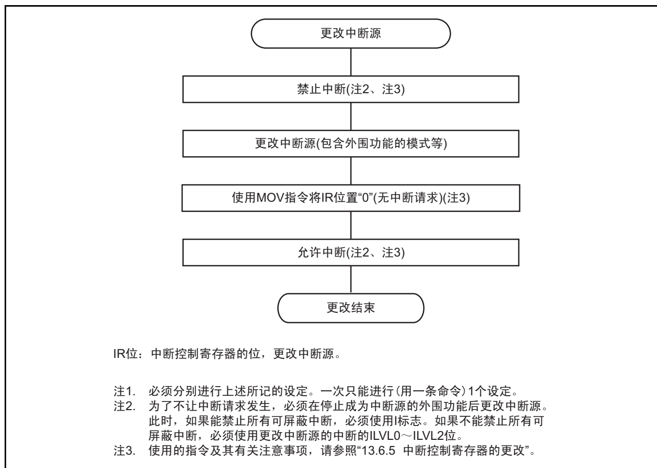
图 2.1 中断源更改步骤的例子
