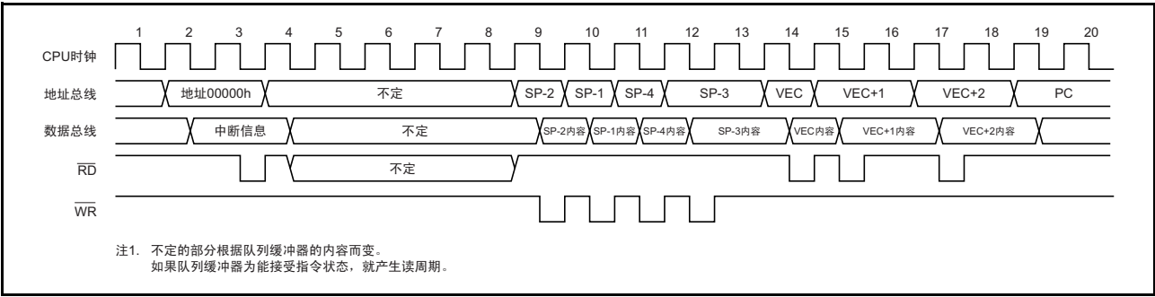
图 13.6 中断响应顺序的执行时间
