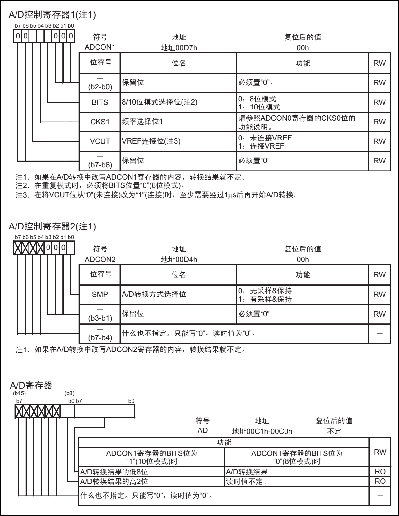
图 18.3 ADCON1、ADCON2 和 AD 寄存器
