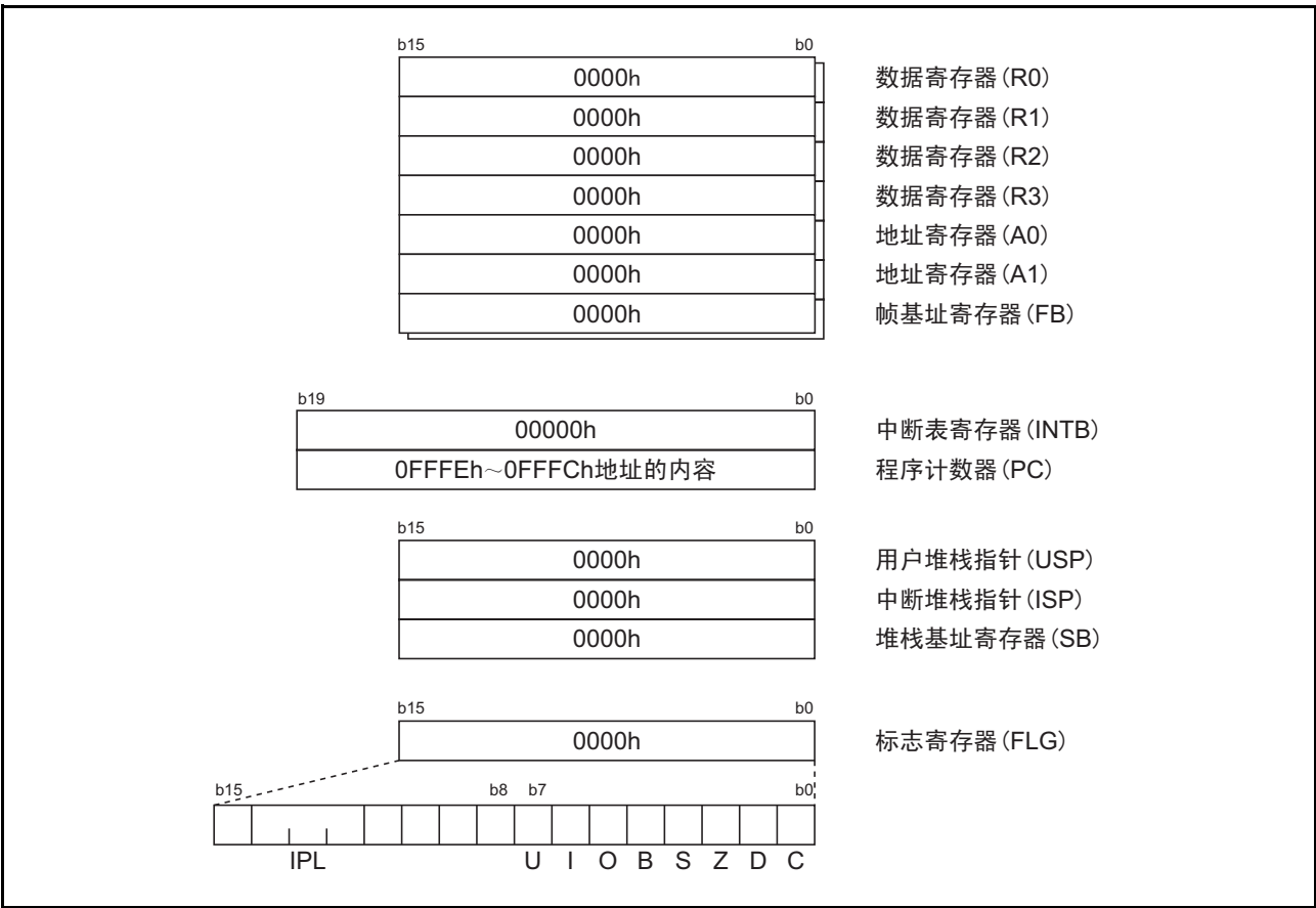
图 6.2 复位后的 CPU 寄存器状态
