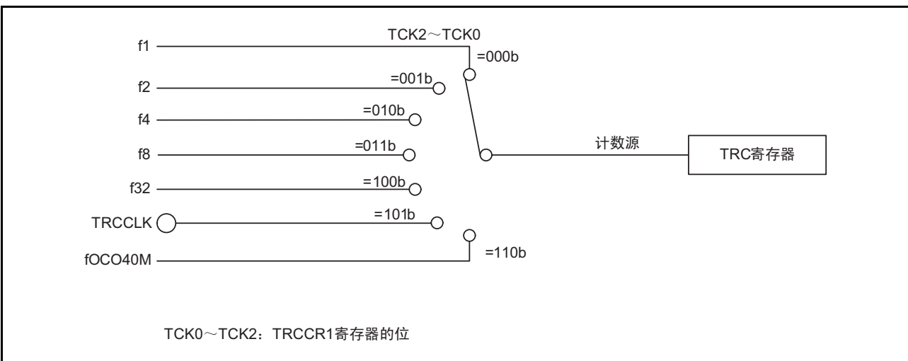
图 15.37 计数源的框图
