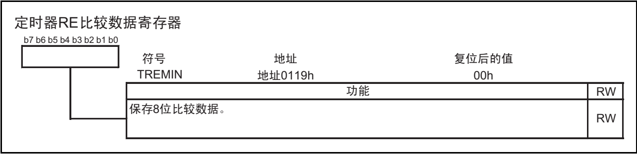
图 15.63 输出比较模式时的 TREMIN 寄存器
