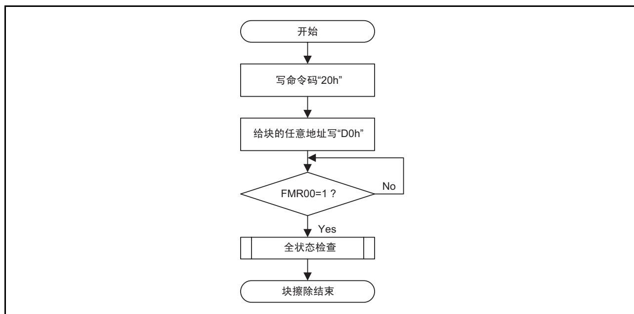
图 21.14 块擦除流程图（禁止擦除挂起功能时）
