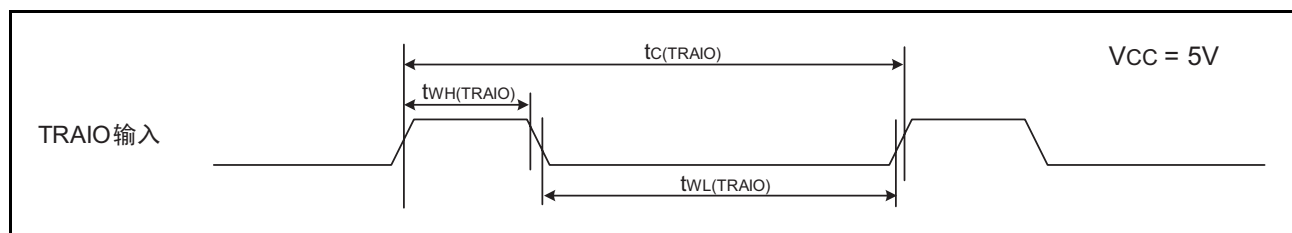
图 22.5 V_{CC}=5V 时的 TRAIO 输入时序
