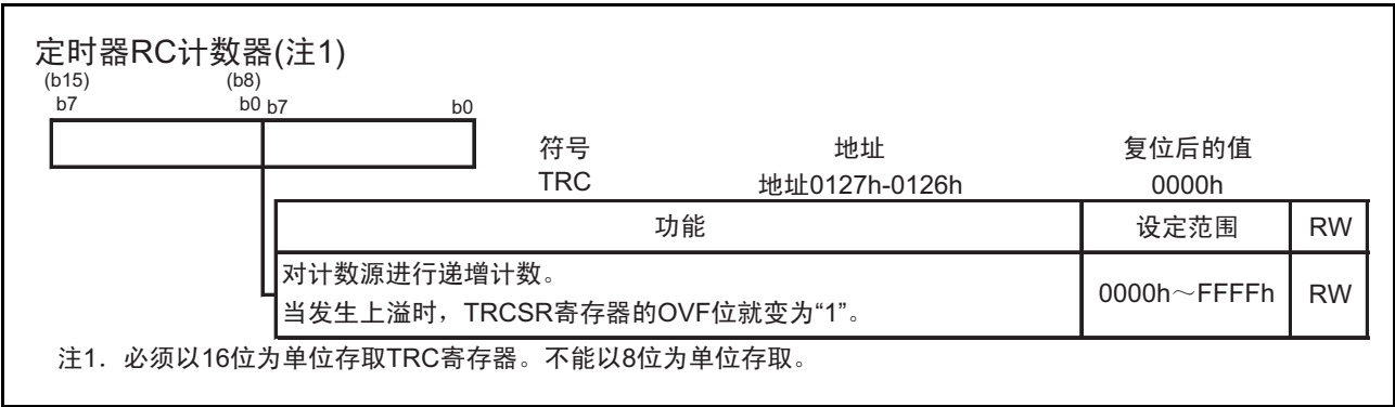
图 15.31 TRC 寄存器
