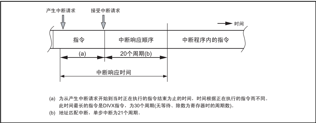
图 13.7 中断响应时间
