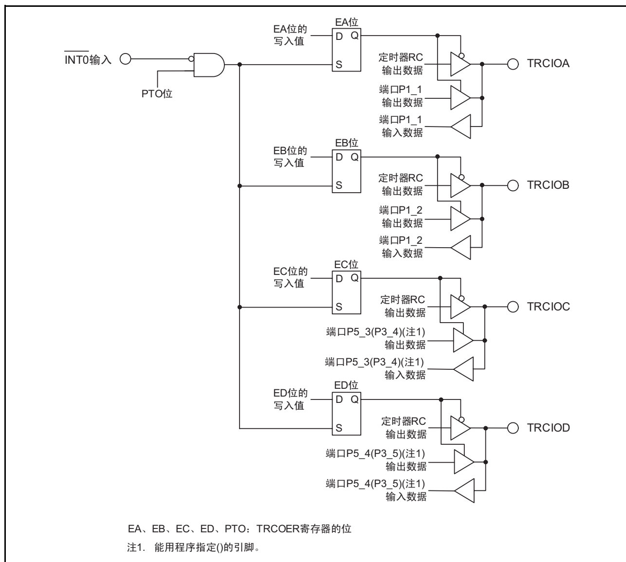
图 15.41 脉冲输出的强制截止
