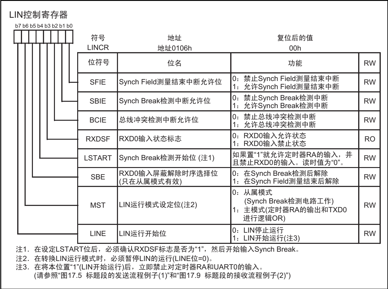
图 17.2 LINCRC 寄存器
