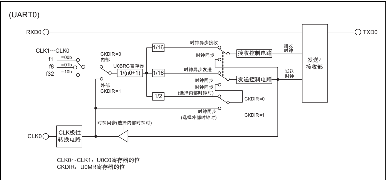
图 16.1 UART0 的框图
