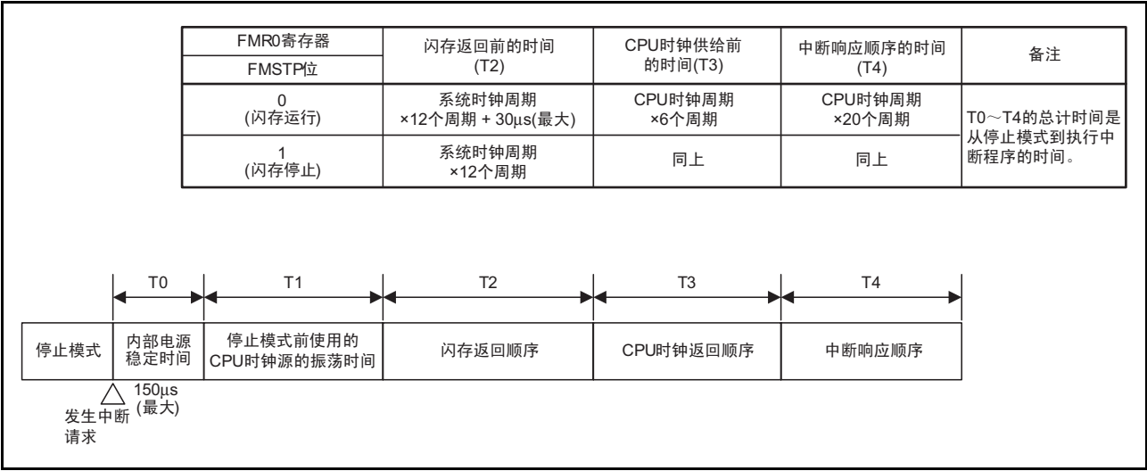
图 11.12 从停止模式到执行中断程序的时间
