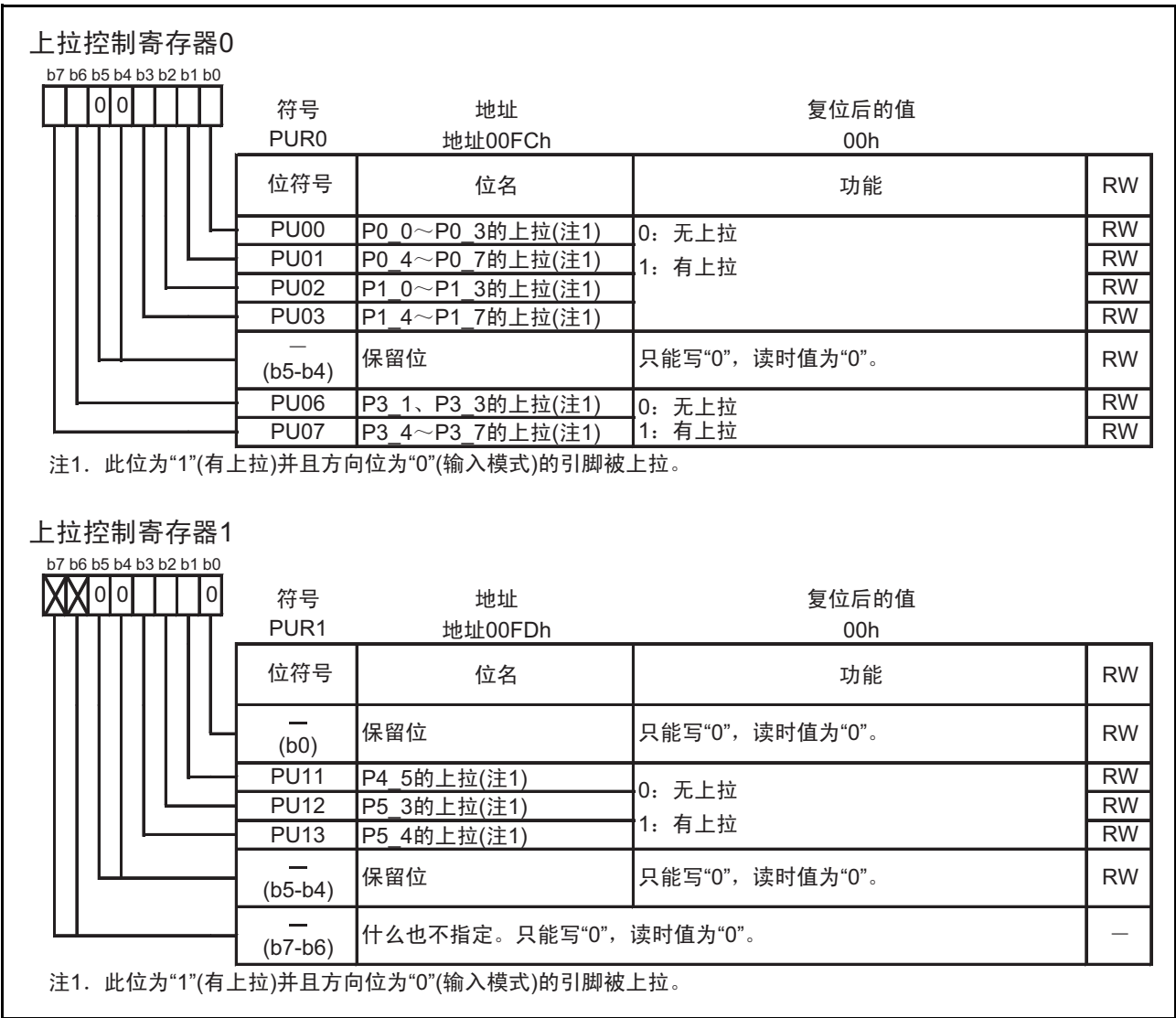
图 8.11 PUR0 和 PUR1 寄存器
