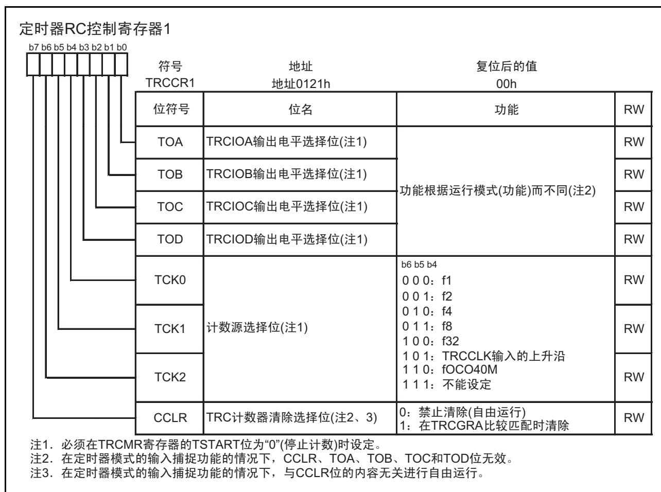
图 15.28 TRCCR1 寄存器
