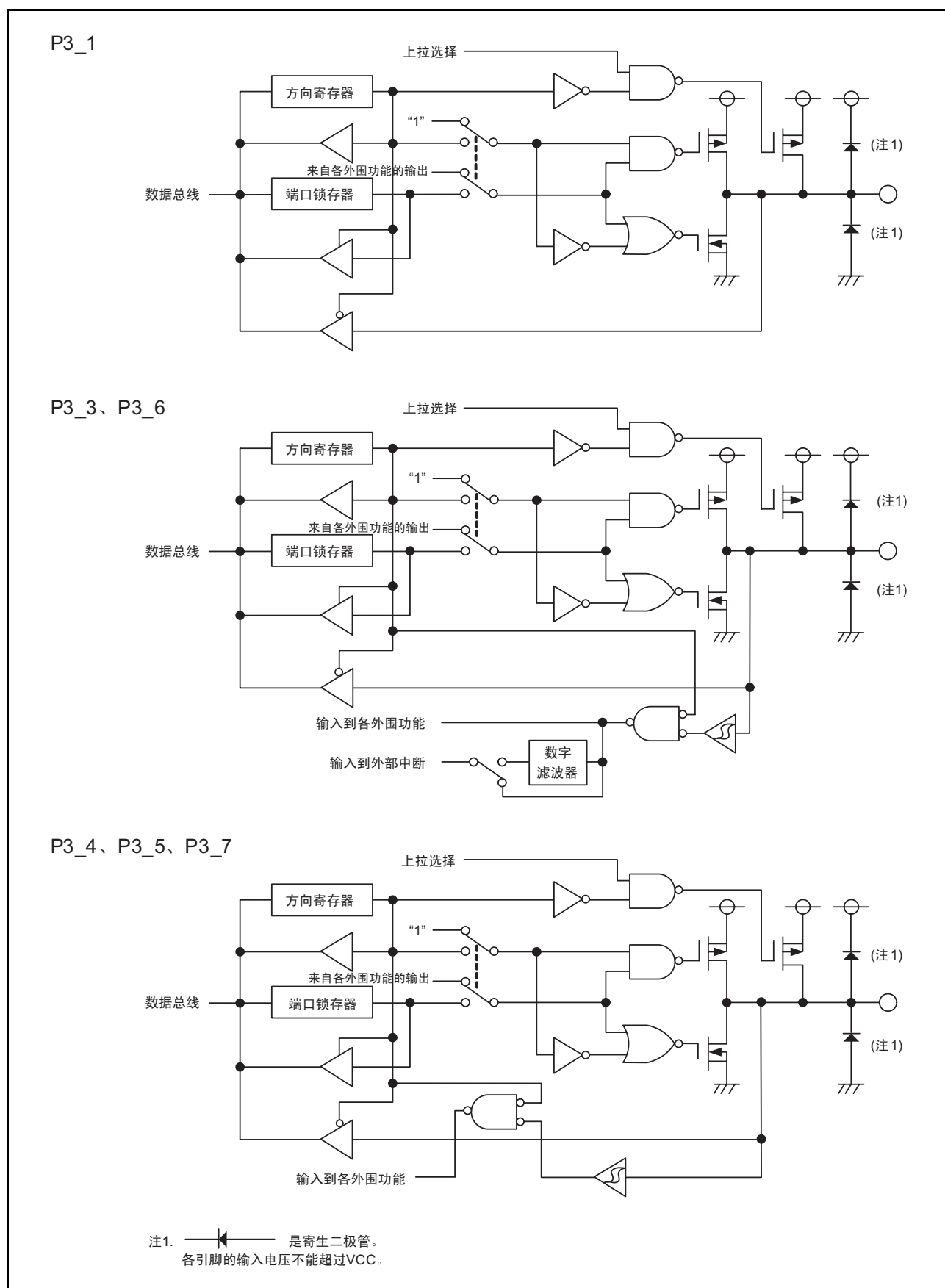
图 8.3 可编程输入 / 输出端口的结构 (3)
