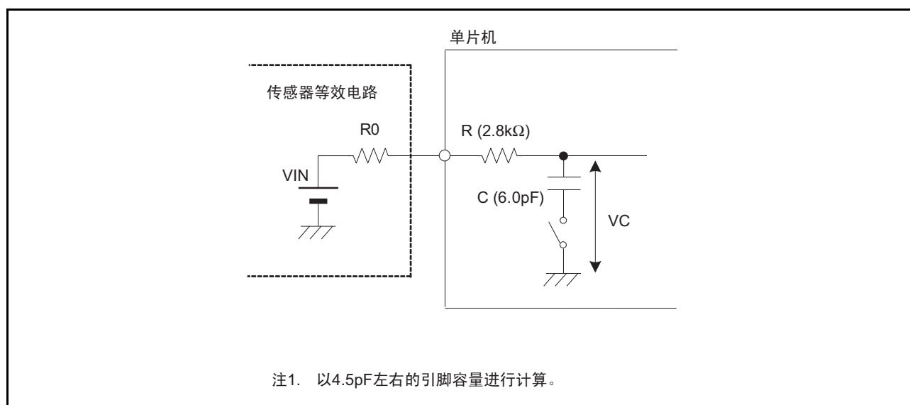
图 18.11 模拟输入引脚和外部传感器的等效电路例子
