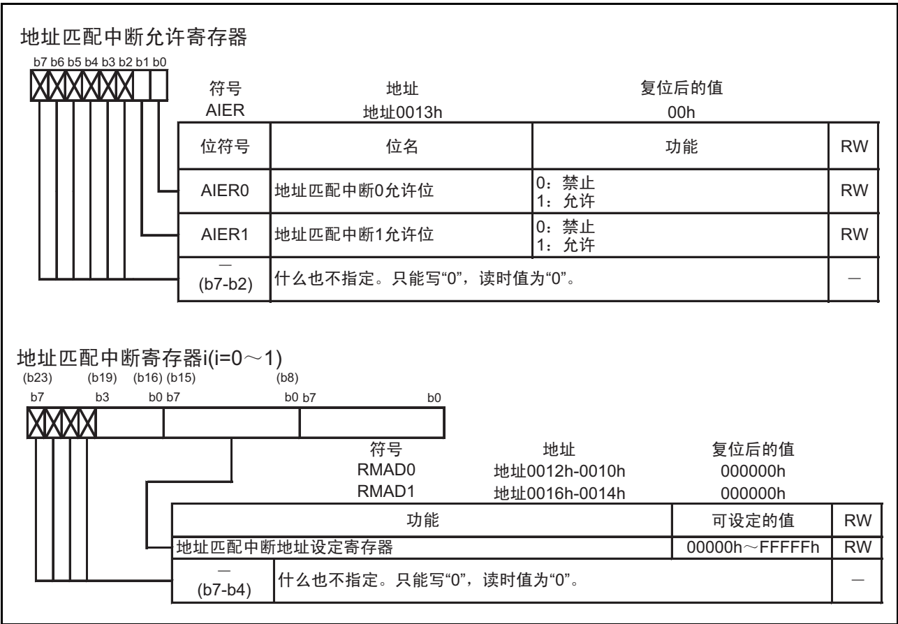
图 13.18 AIER 和 RMAD0 ~ RMAD1 寄存器
