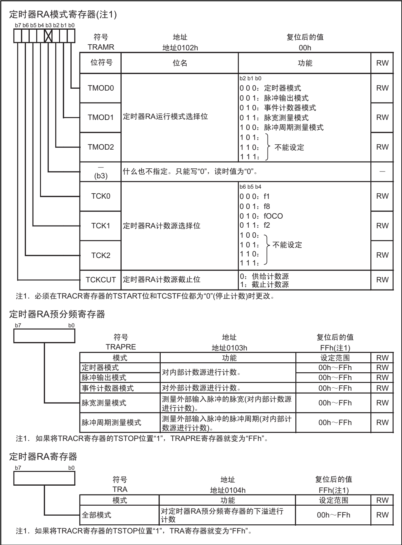
图 15.3 TRAMR、TRAPRE 和 TRA 寄存器
