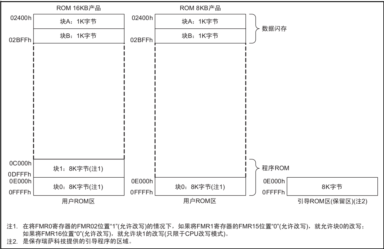
图 21.2 R8C/2F 群的闪存框图
