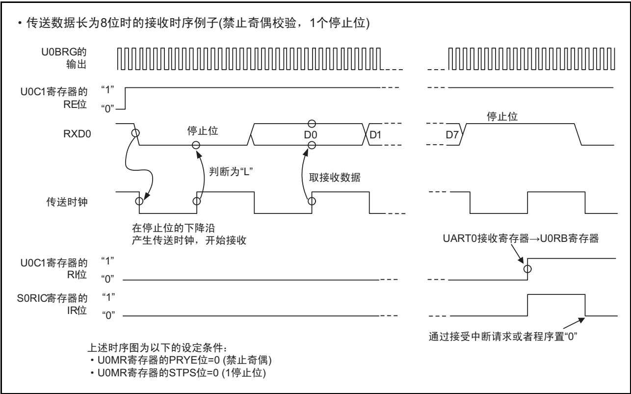
图 16.12 UART 模式时的接收时序例子
