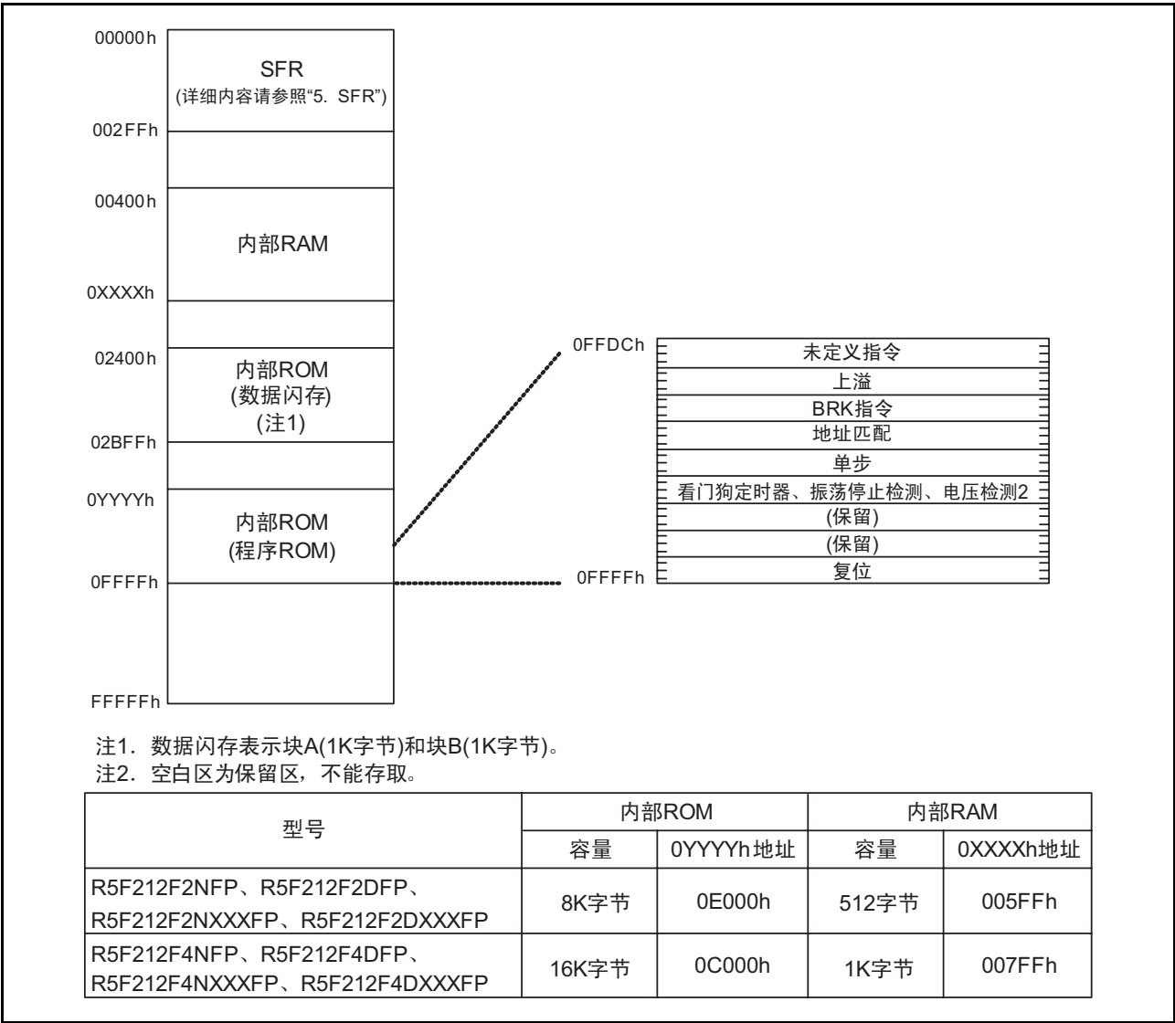
图 4.2 R8C/2F 群的存储器分配图
