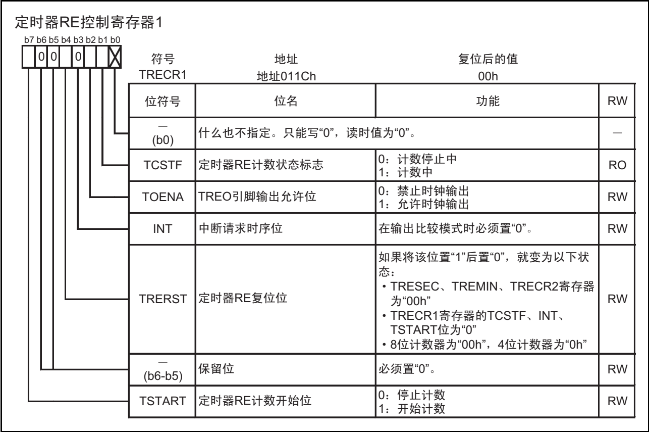
图 15.64 输出比较模式时的 TRECR1 寄存器
