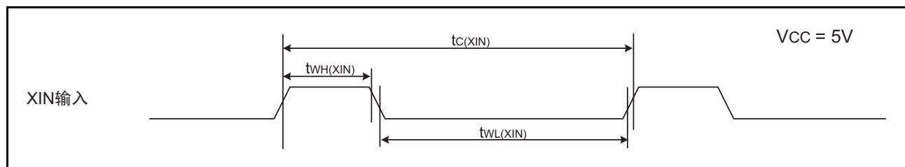
图 22.4 V_{CC}=5V 时的 XIN 输入时序
