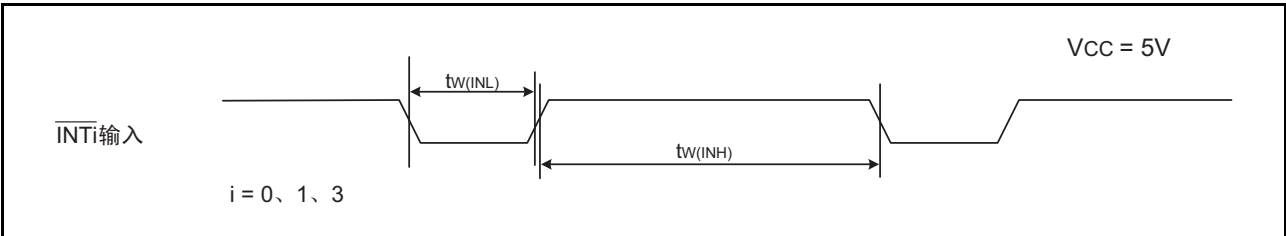
图 22.7 V_{CC}=5V 时的外部中断 \overline{INTi} 输入时序
