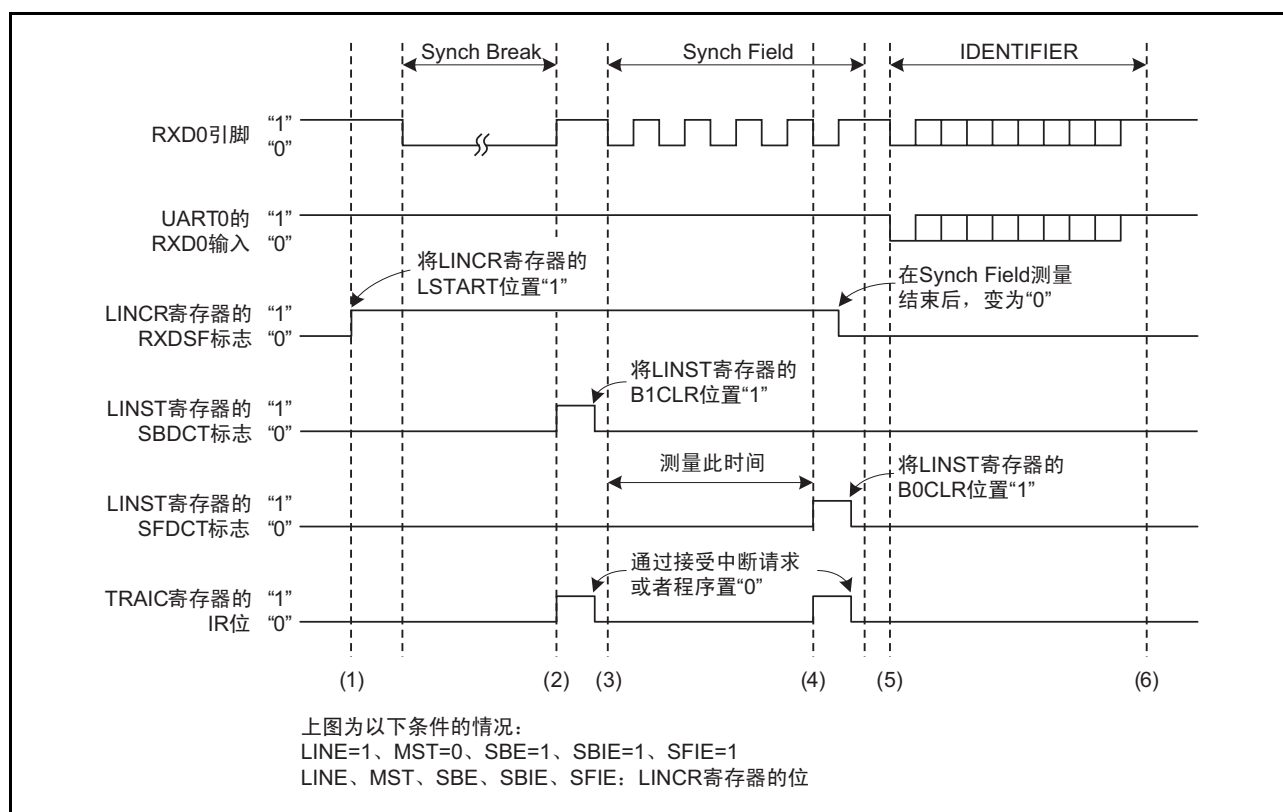
图 17.7 标题段的接收运行例子
