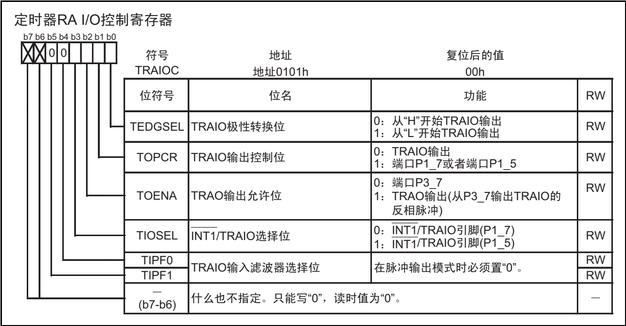
图 15.6 脉冲输出模式时的 TRAIOC 寄存器
