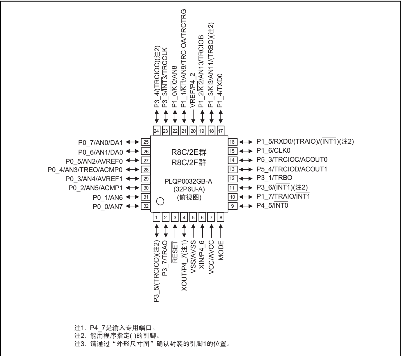
图 1.4 引脚配置图（俯视图）
