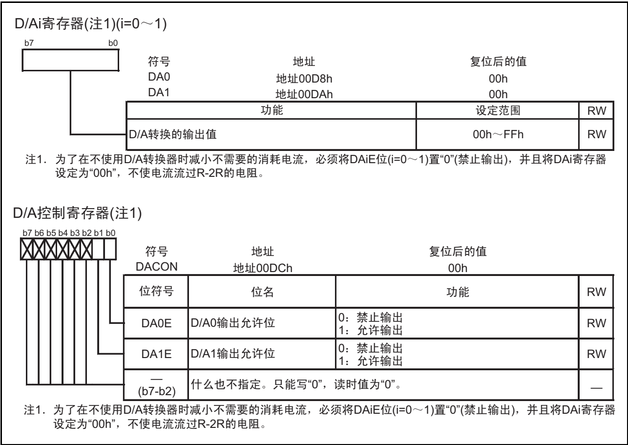
图 19.2 DA0 ~ DA1 和 DACON 寄存器
