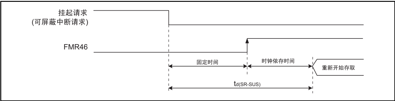
图 22.2 挂起的转移时间
