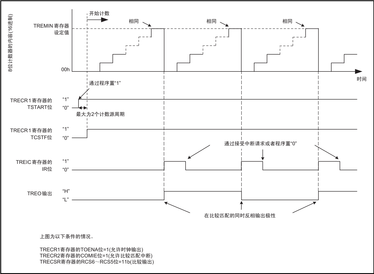
图 15.67 输出比较模式的运行例子
