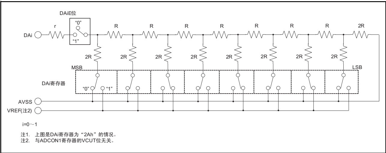
图 19.4 D/A 转换器的等效电路
