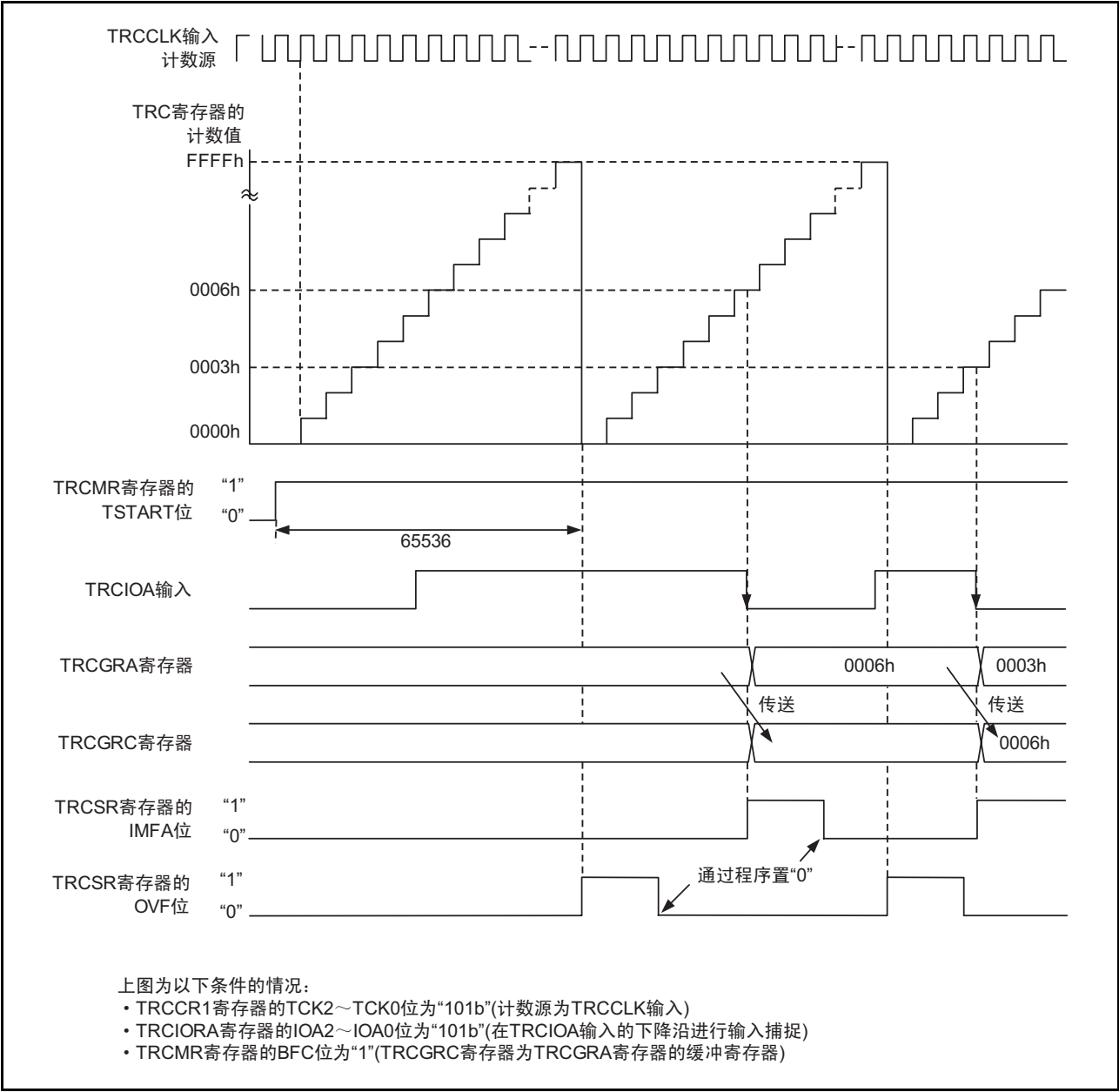
图 15.45 输入捕捉功能的运行例子
