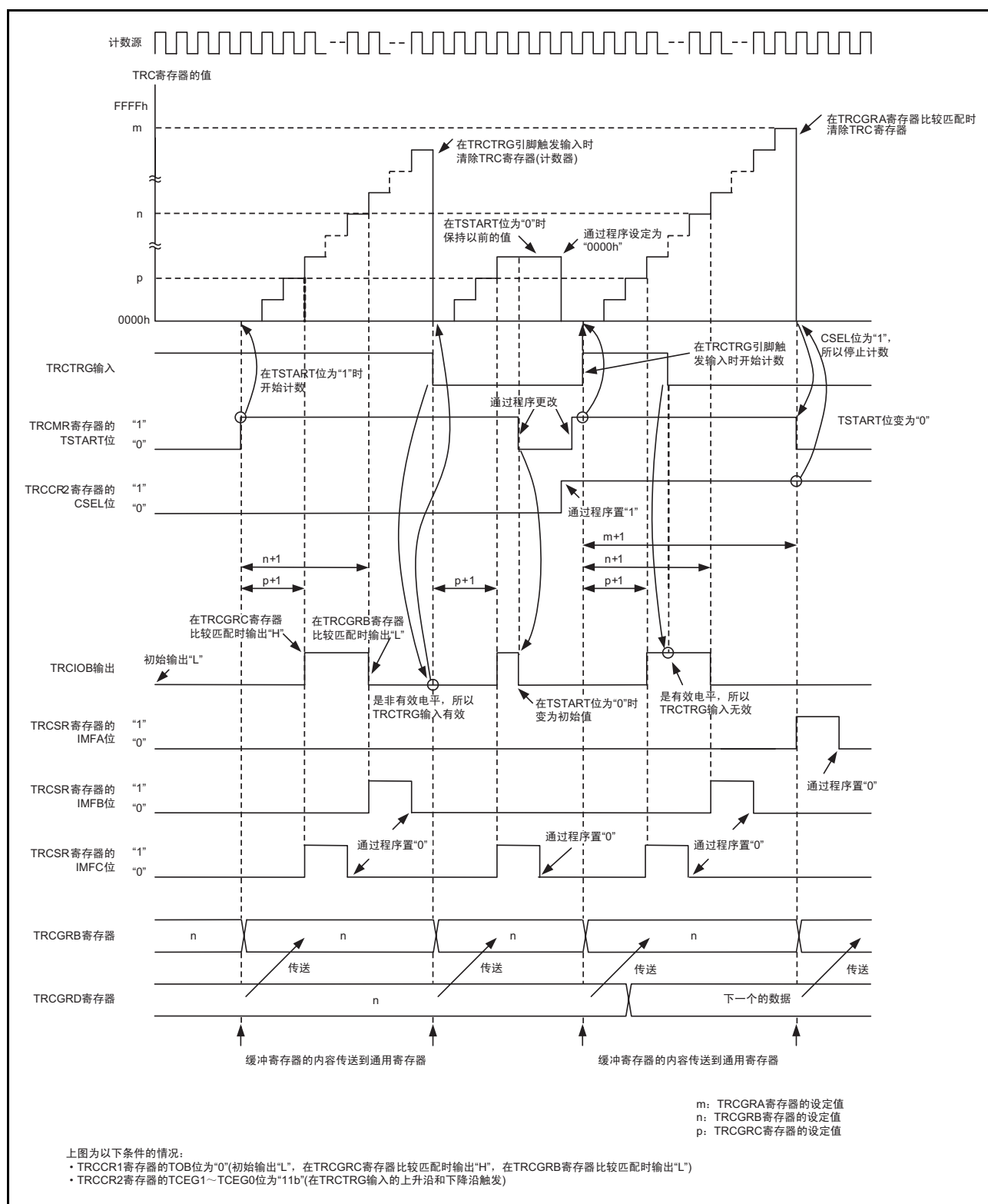
图 15.58 PWM2 模式的运行例子（允许 TRCTRIG 触发输入）
