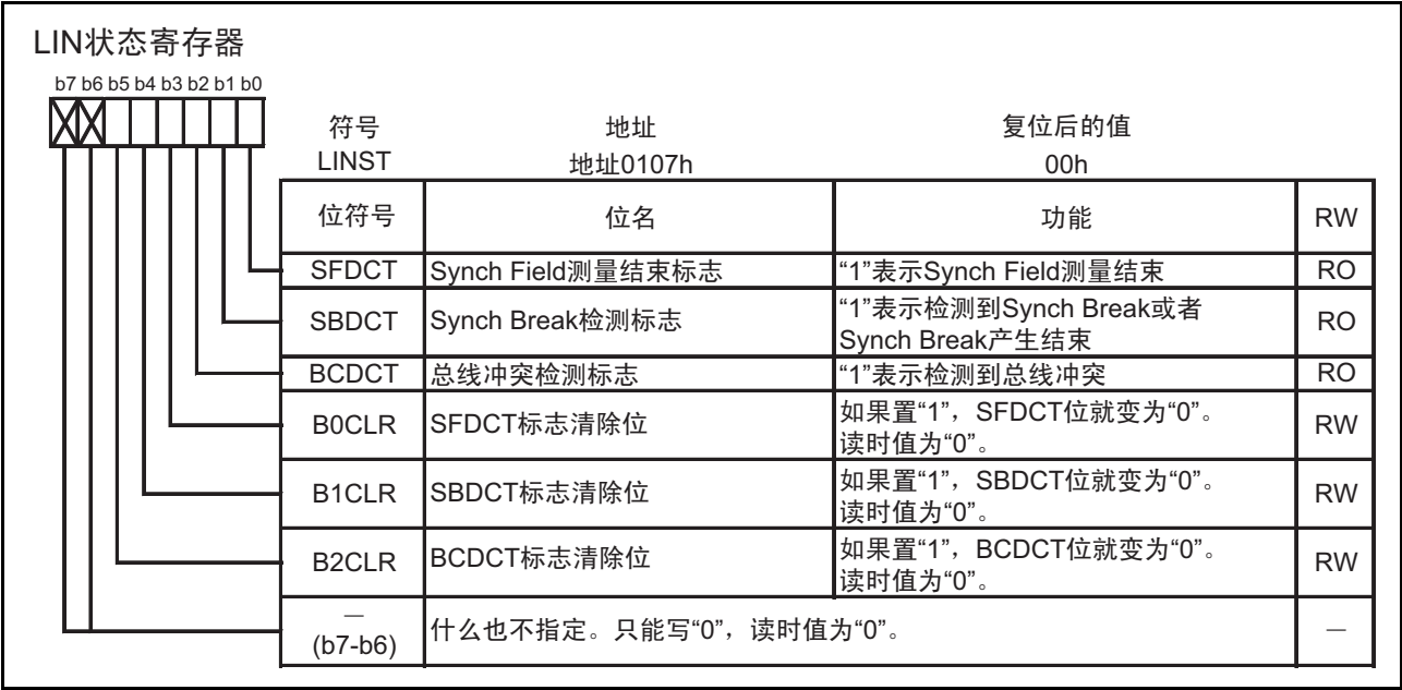
图 17.3 LINST 寄存器
