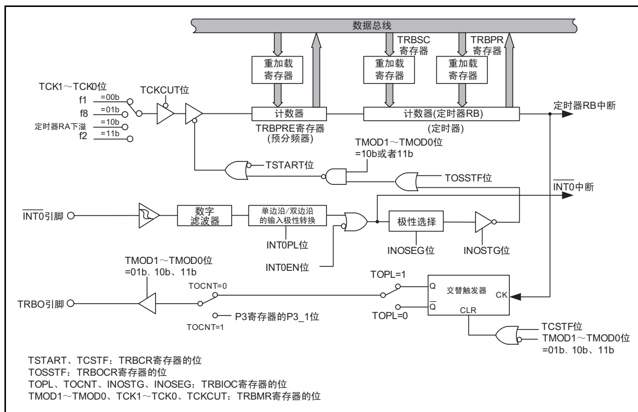
图 15.12 定时器 RB 的框图
