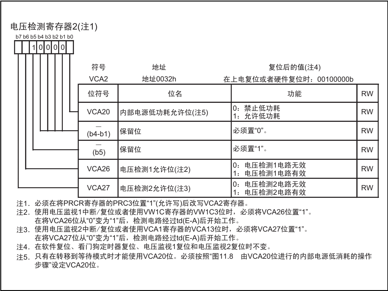
图 11.7 VCA2 寄存器
