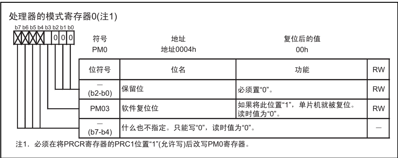
图 9.1 PM0 寄存器
