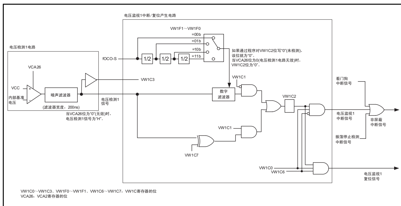
图 7.2 电压监视 1 中断 / 复位产生电路的框图
