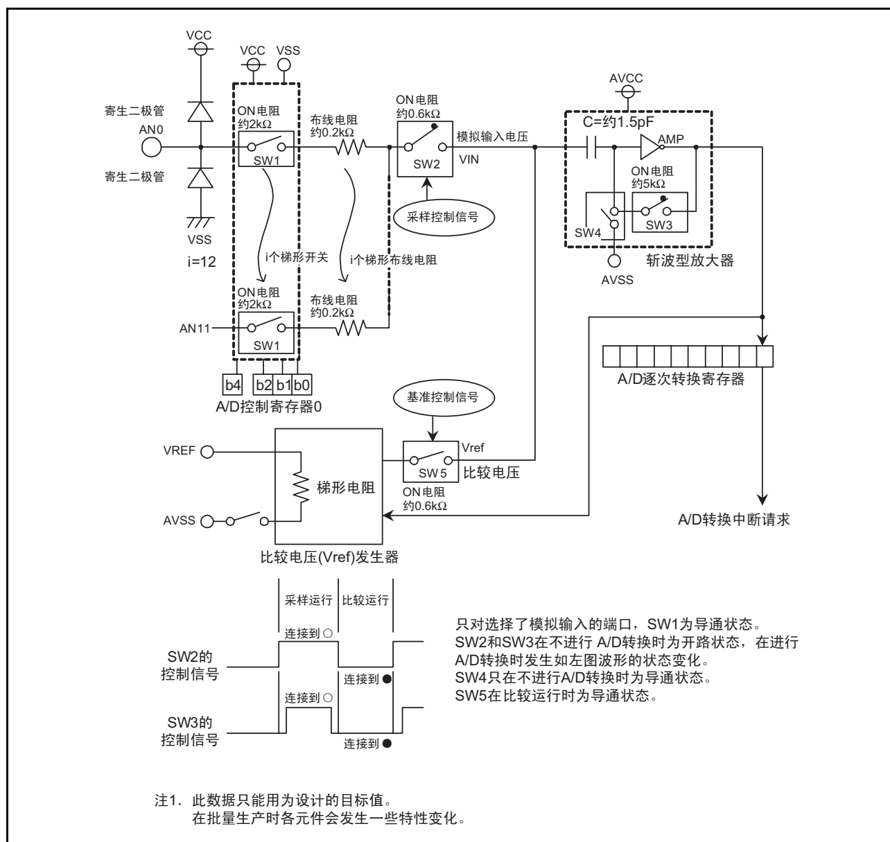
图 18.10 模拟输入内部等效电路
