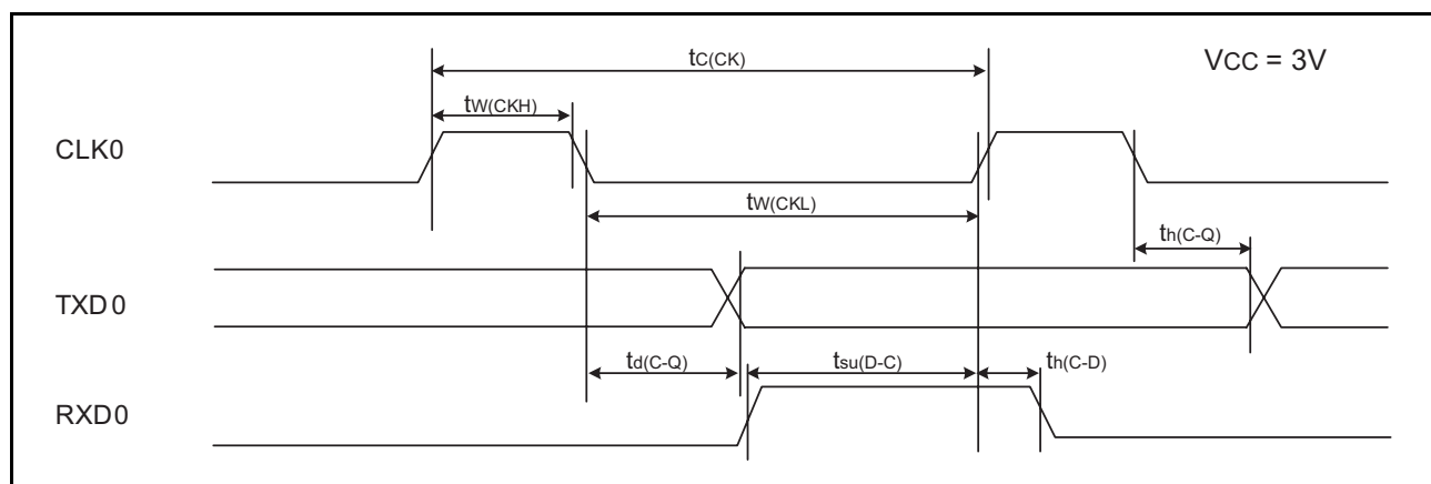
图 22.10 V_{CC}=3V 时的串行接口时序
