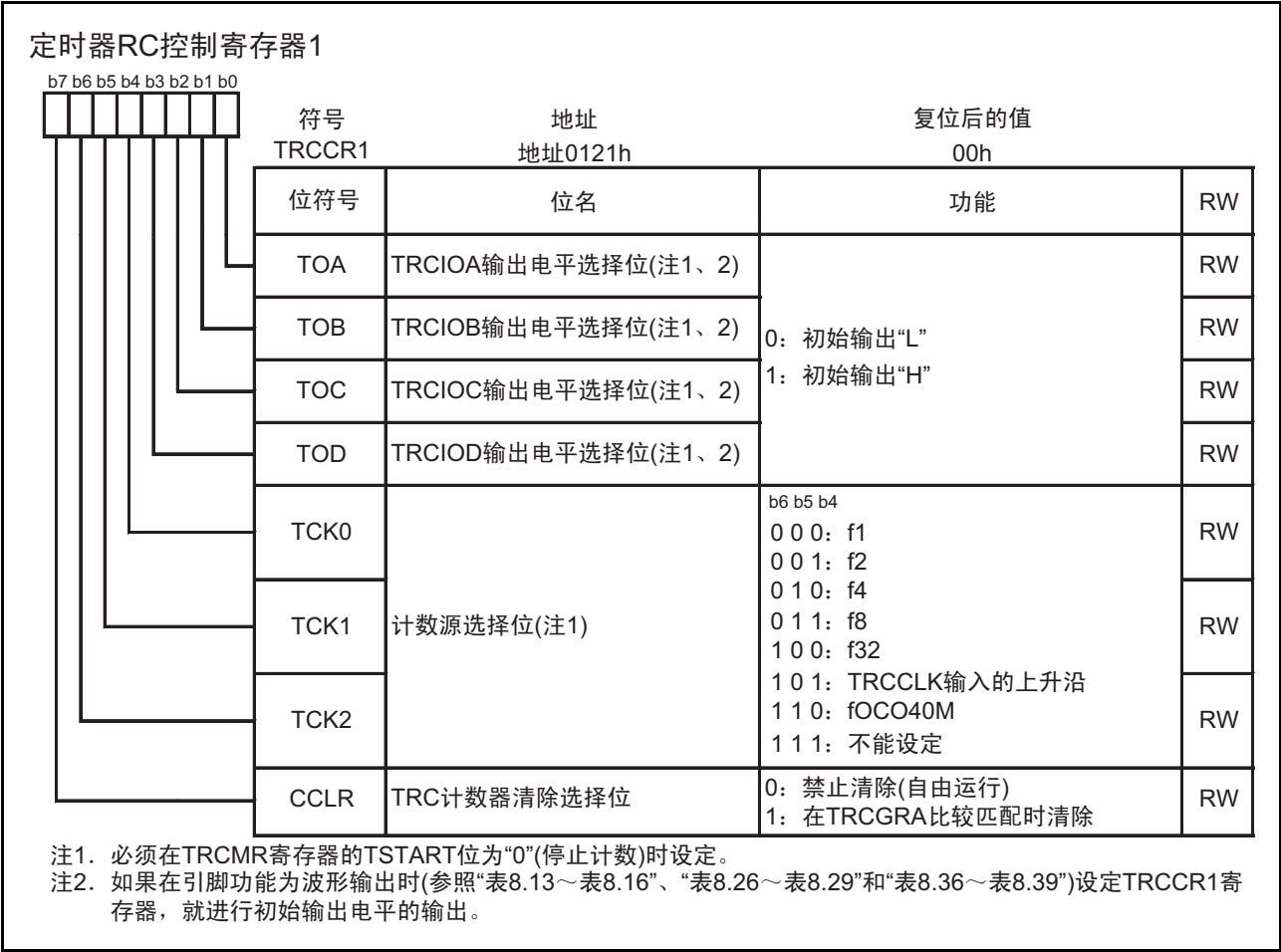
图 15.49 输出比较功能时的 TRCCR1 寄存器
