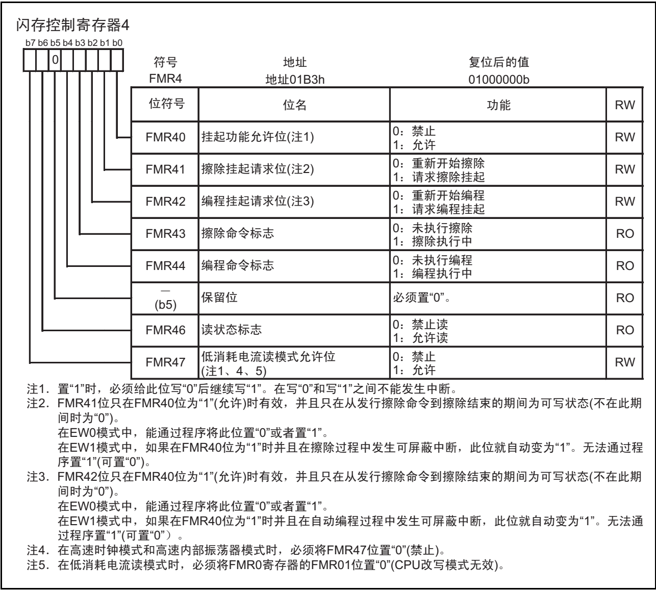
图 21.7 FMR4 寄存器
