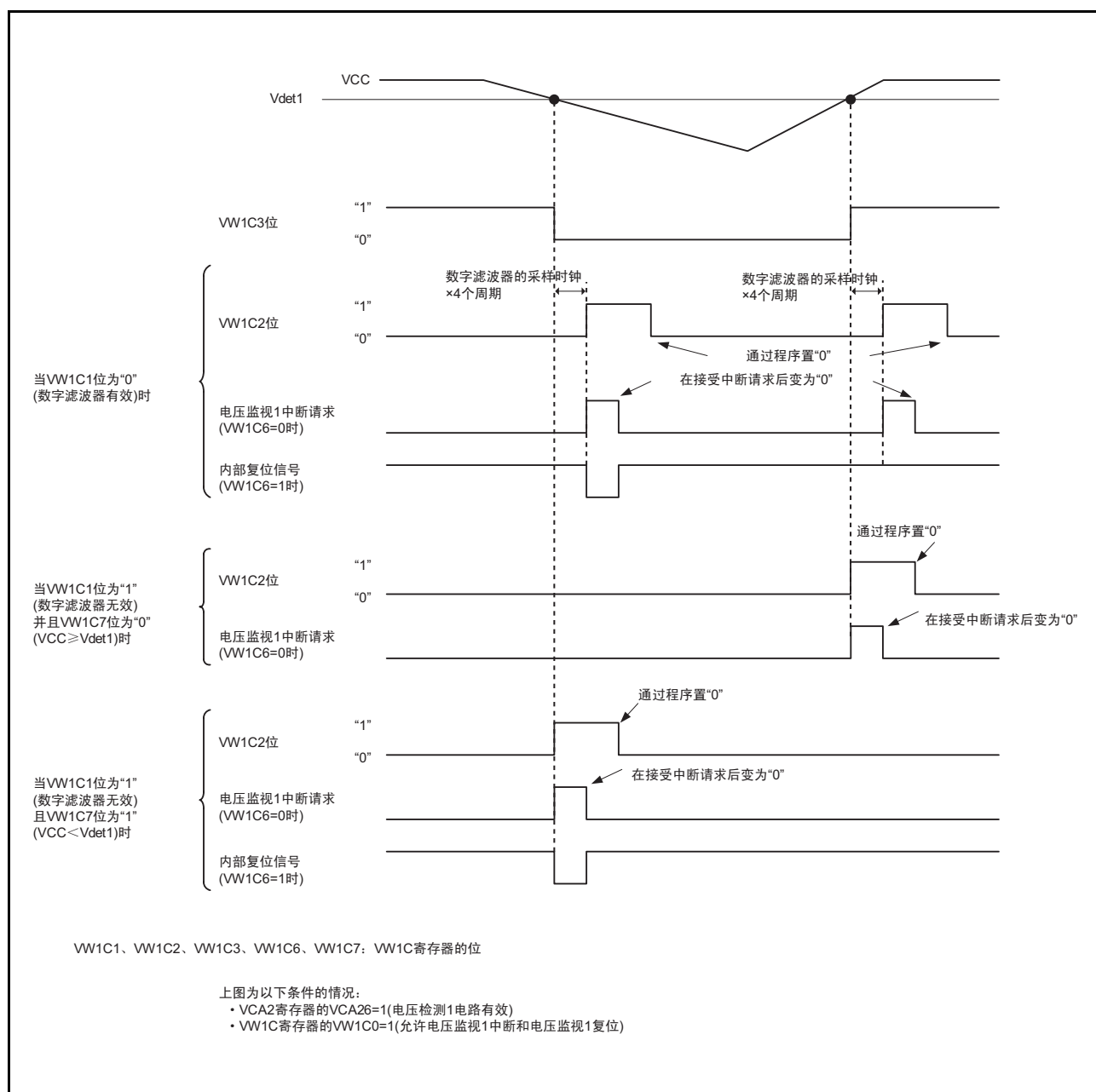
图 7.7 电压监视 1 中断和电压监视 1 复位的运行例子
