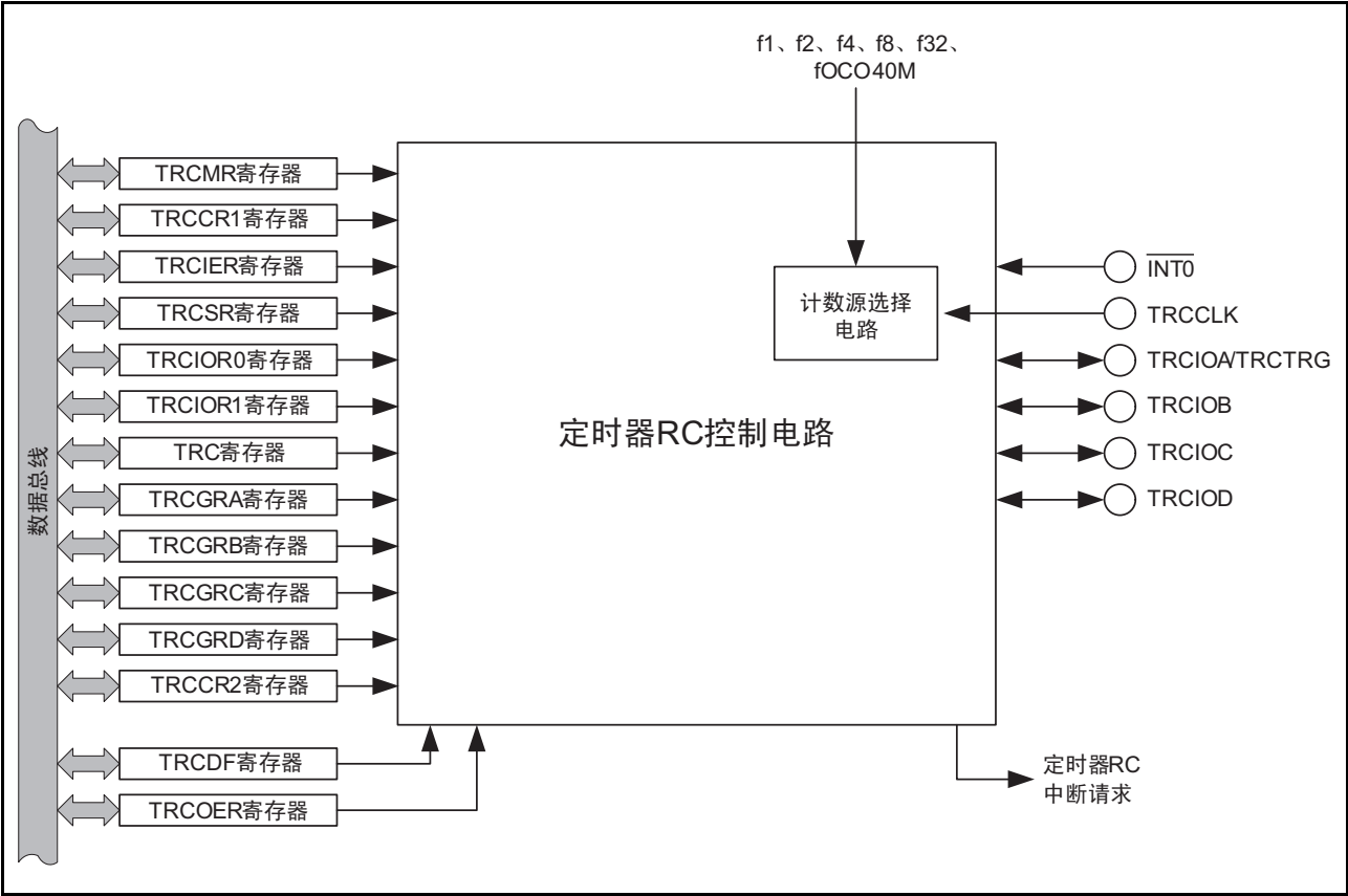
图 15.26 定时器 RC 的框图
