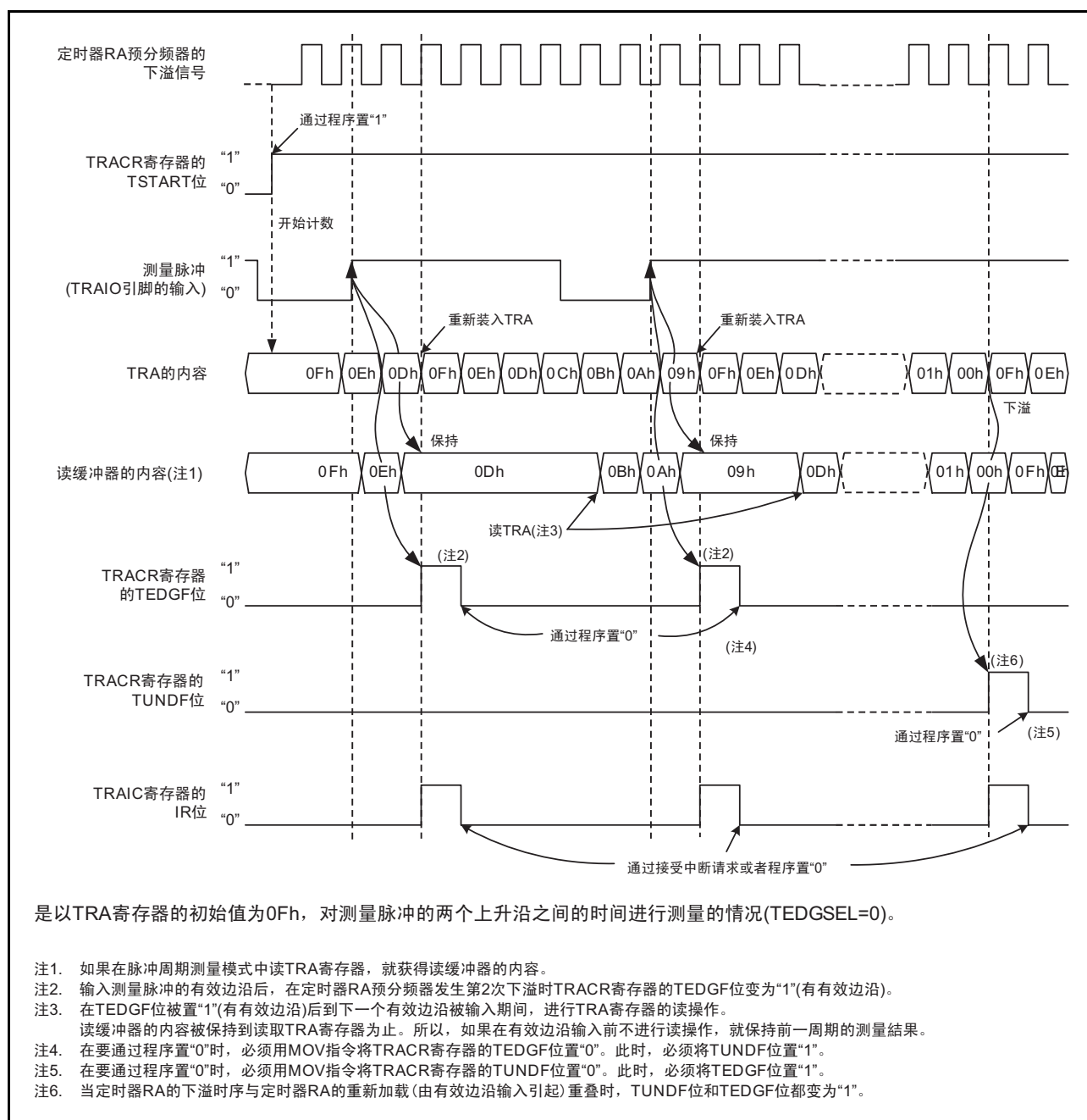
图 15.11 脉冲周期测量模式时的运行例子
