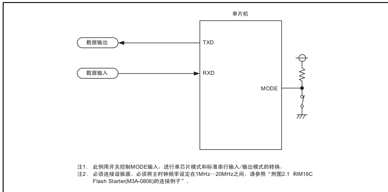
图 21.18 使用标准串行输入 / 输出模式 2 时的引脚处理例子
