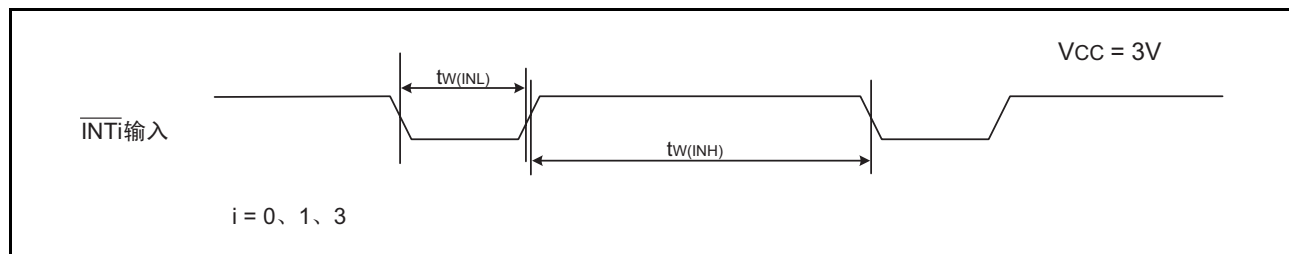
图 22.11 V_{CC}=3V 时的外部中断 \overline{INTi} 输入时序
