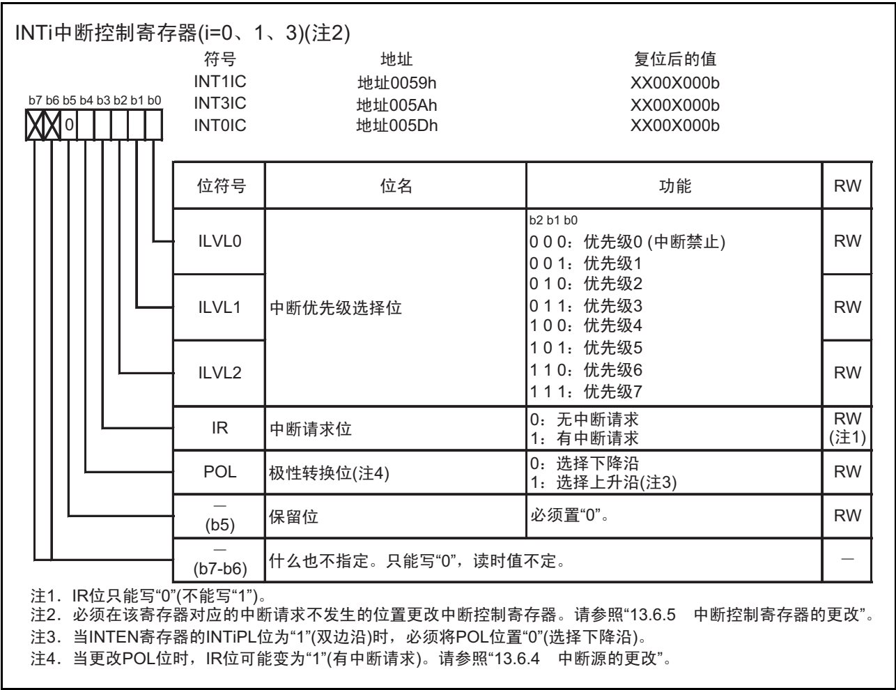
图 13.5 INT0IC、INT1IC 和 INT3IC 寄存器
