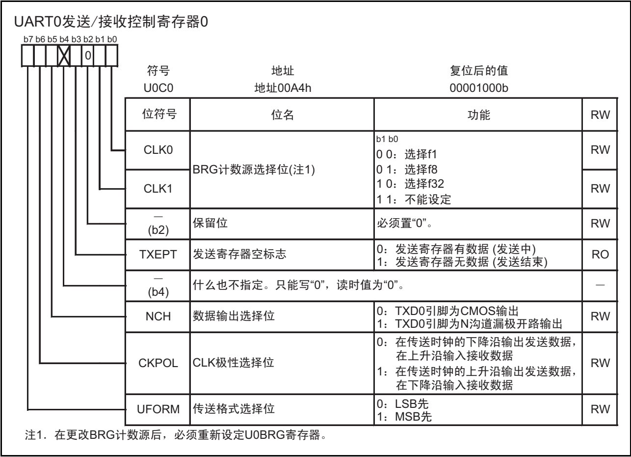
图 16.5 U0C0 寄存器
