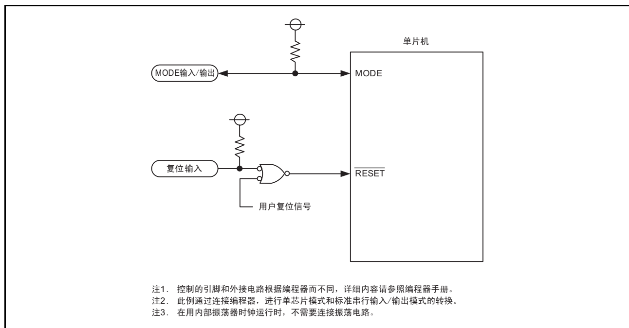
图 21.19 使用标准串行输入 / 输出模式 3 时的引脚处理例子
