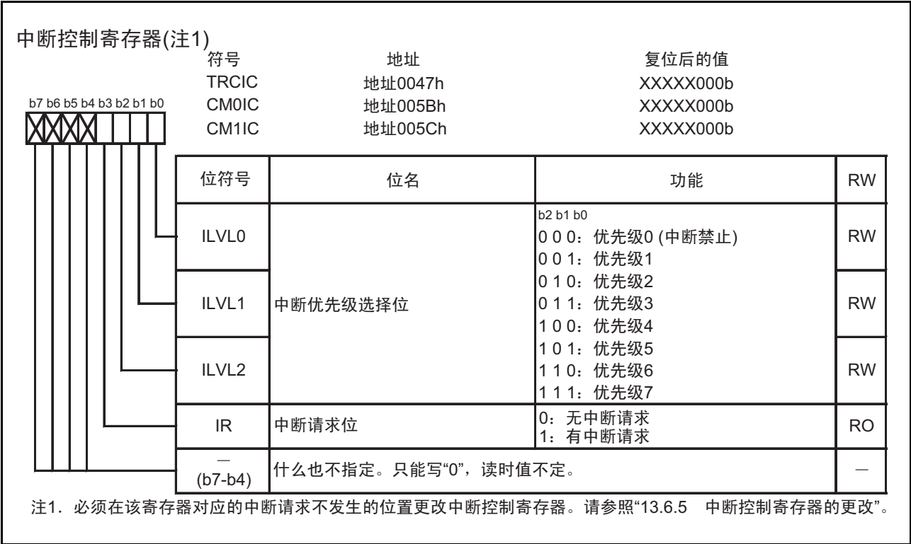
图 13.4 TRCIC、CM0IC 和 CM1IC 寄存器
