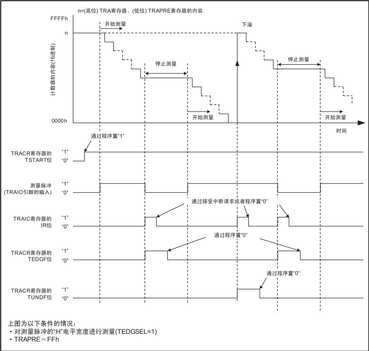
图 15.9 脉宽测量模式时的运行例子
