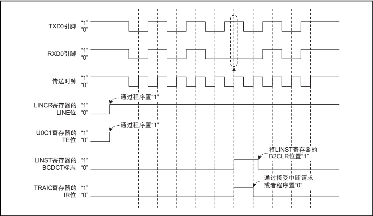
图 17.11 检测总线冲突时的运行例子
