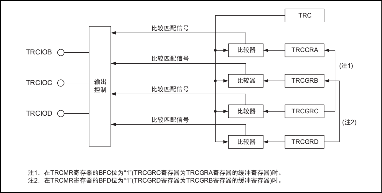
图 15.51 PWM 模式的框图
