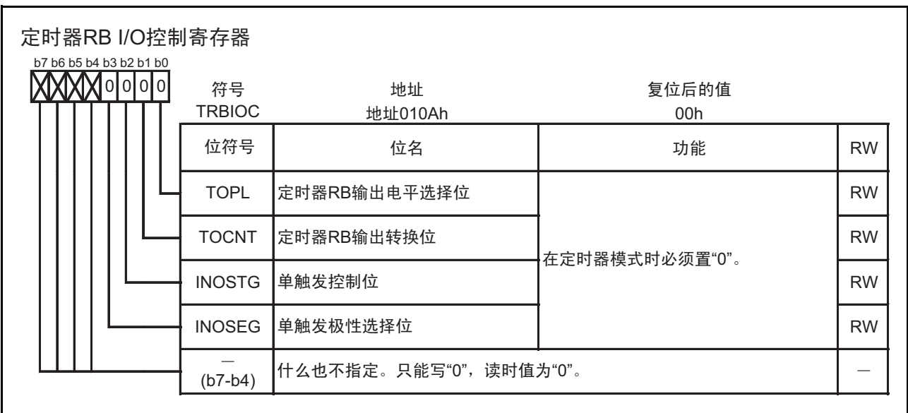
图 15.16 定时器模式时的 TRBIOC 寄存器
