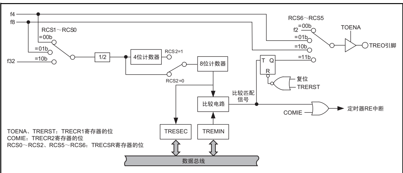
图 15.61 输出比较模式的框图
