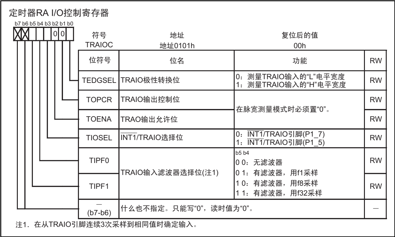
图 15.8 脉宽测量模式时的 TRAIOC 寄存器
