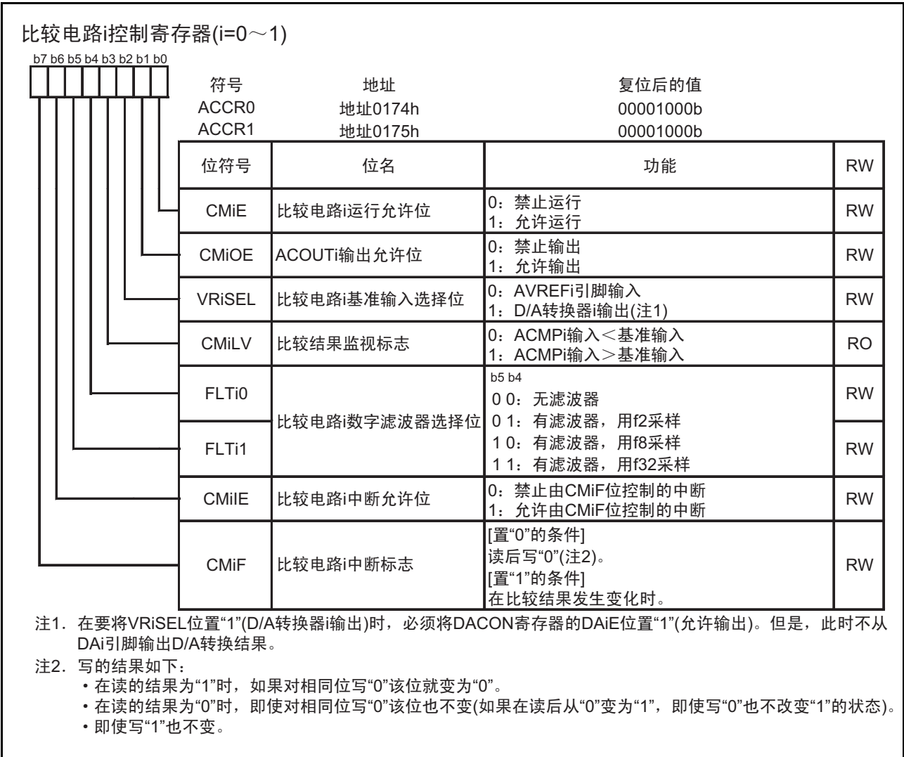
图 19.3 ACCR0 ~ ACCR1 寄存器
