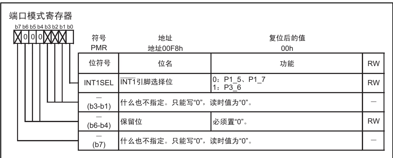
图 8.10 PMR 寄存器
