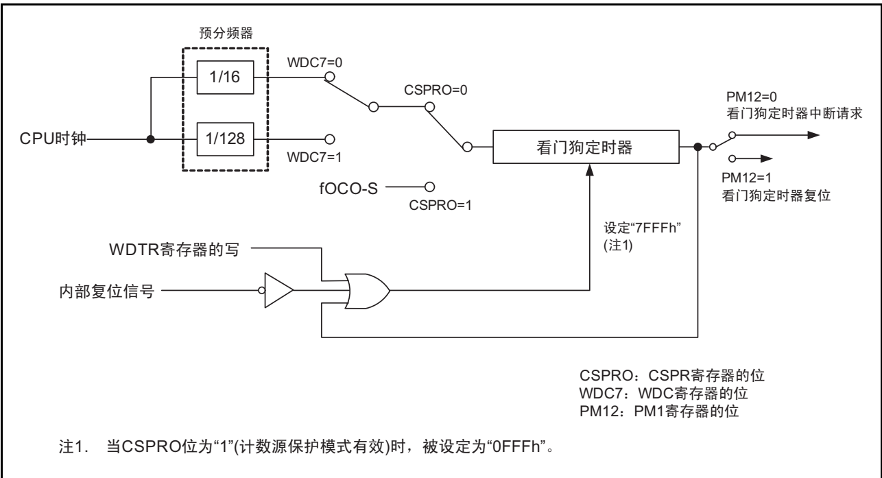
图 14.1 看门狗定时器的框图
