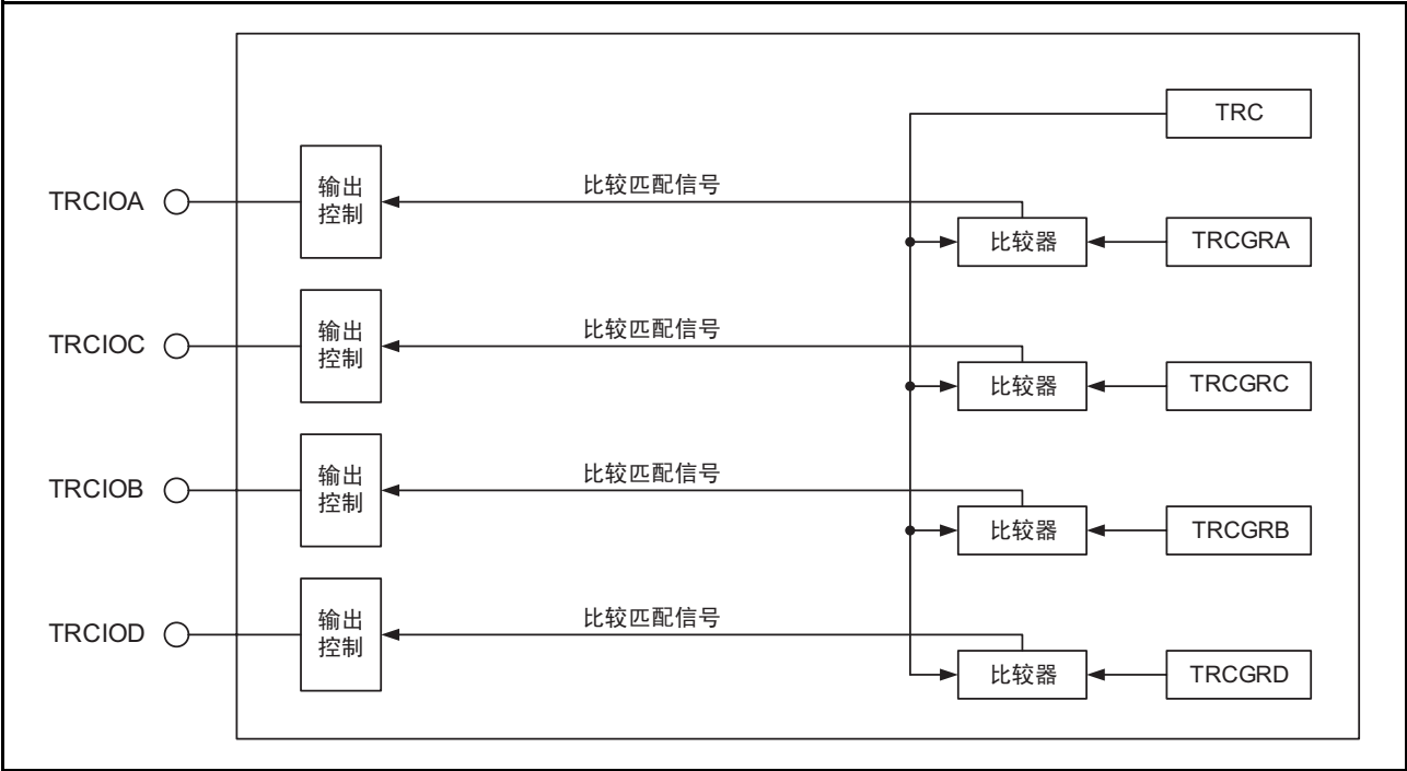
图 15.46 输出比较功能的框图
