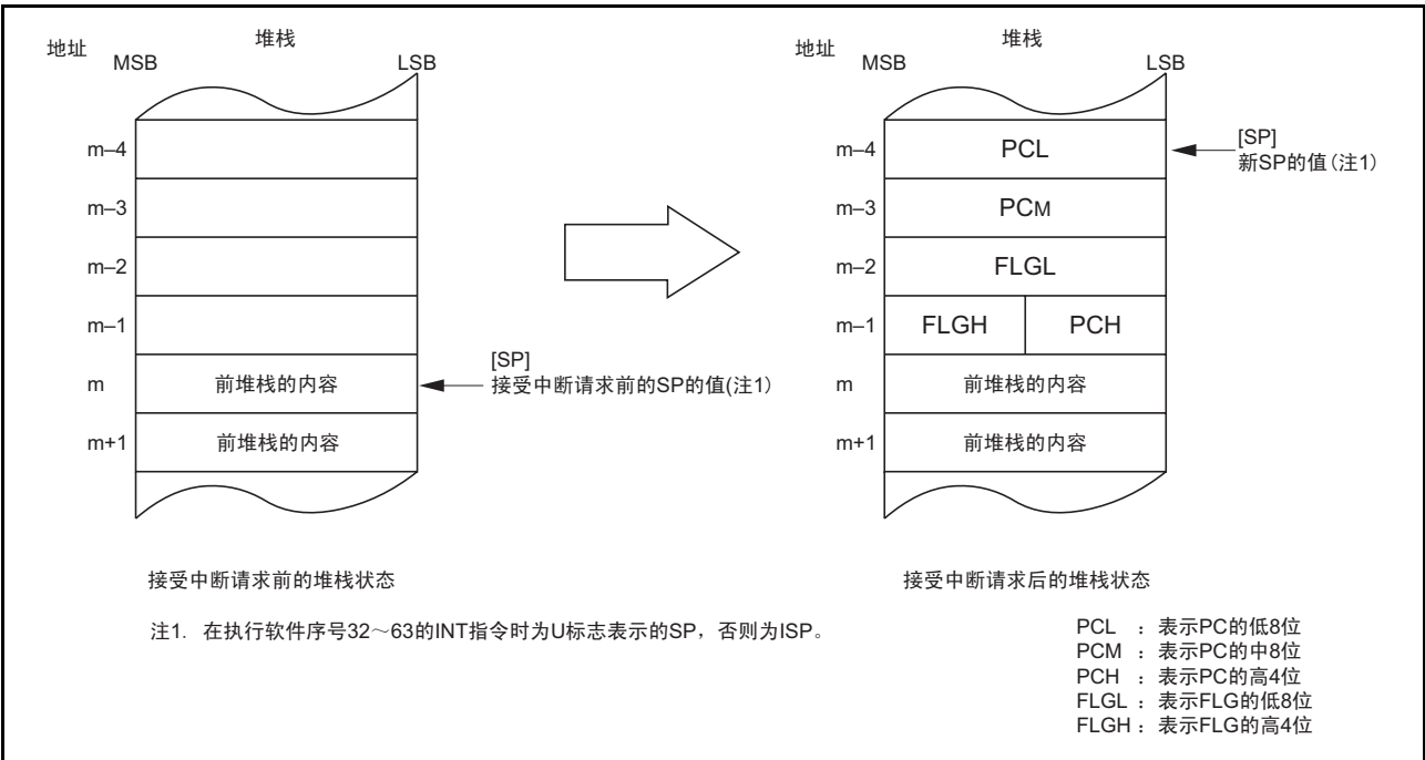
图 13.8 中断请求接受前后的堆栈状态
