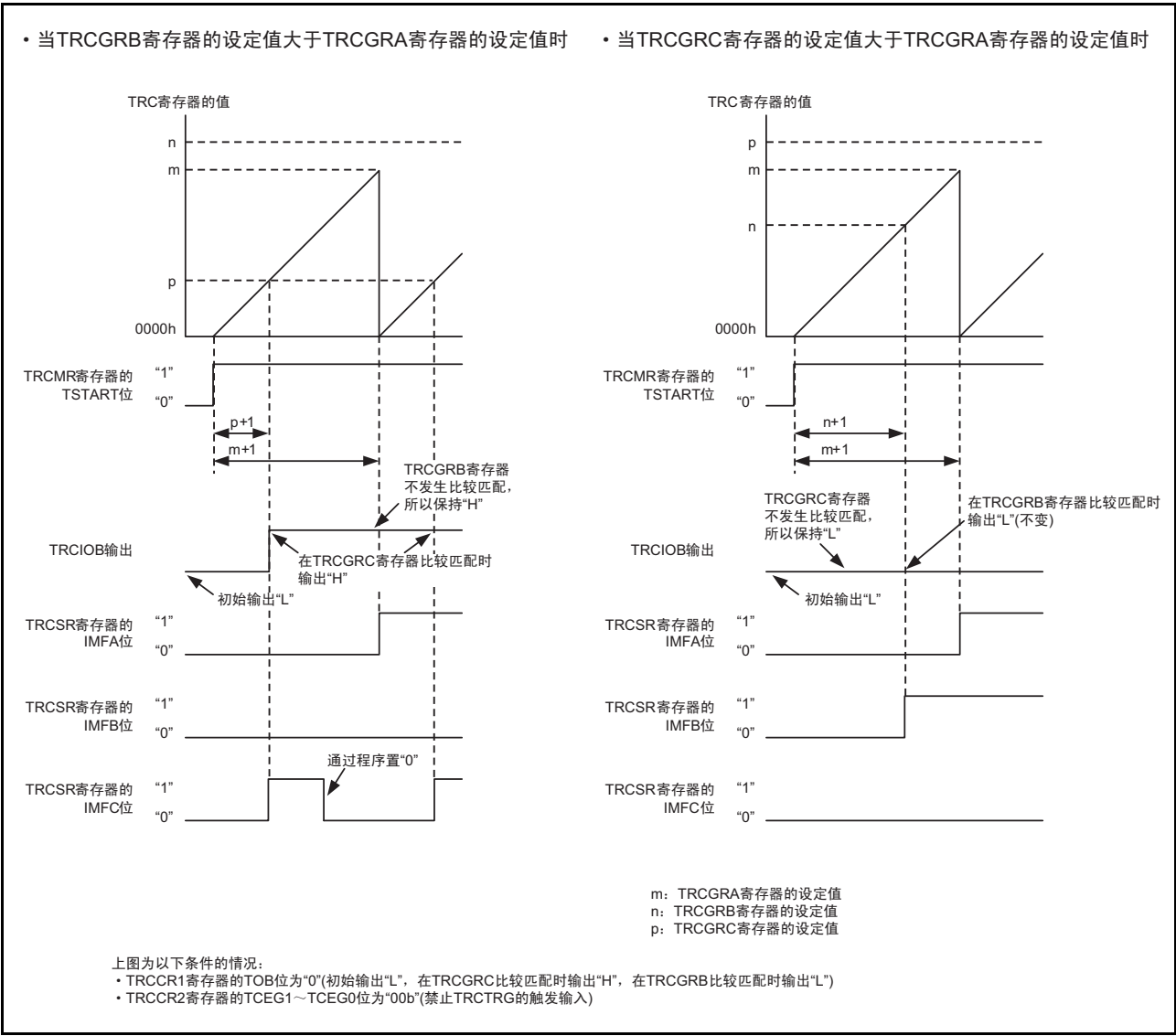
图 15.59 PWM2 模式的运行例子（占空比 0% 和占空比 100%）
