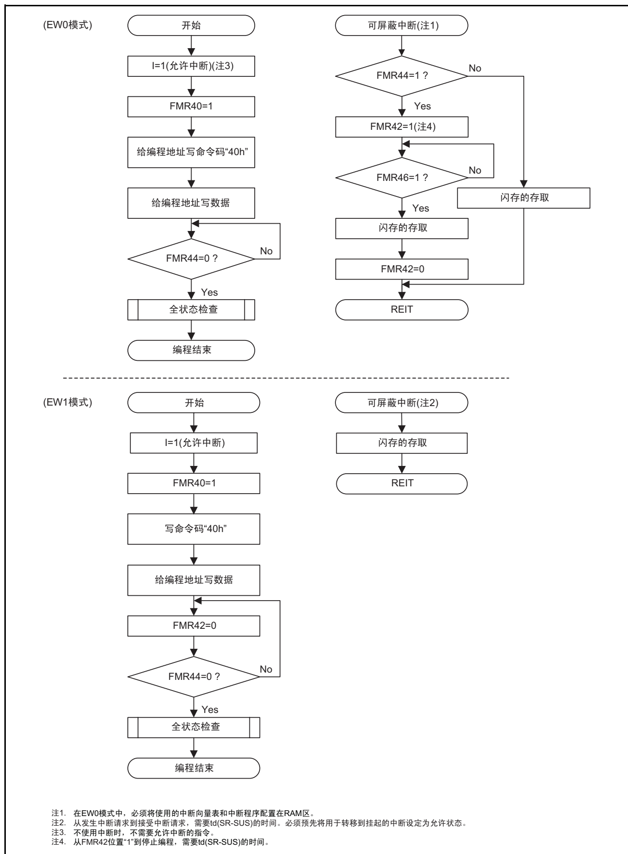
图 21.13 编程流程图 (允许挂起功能时)
