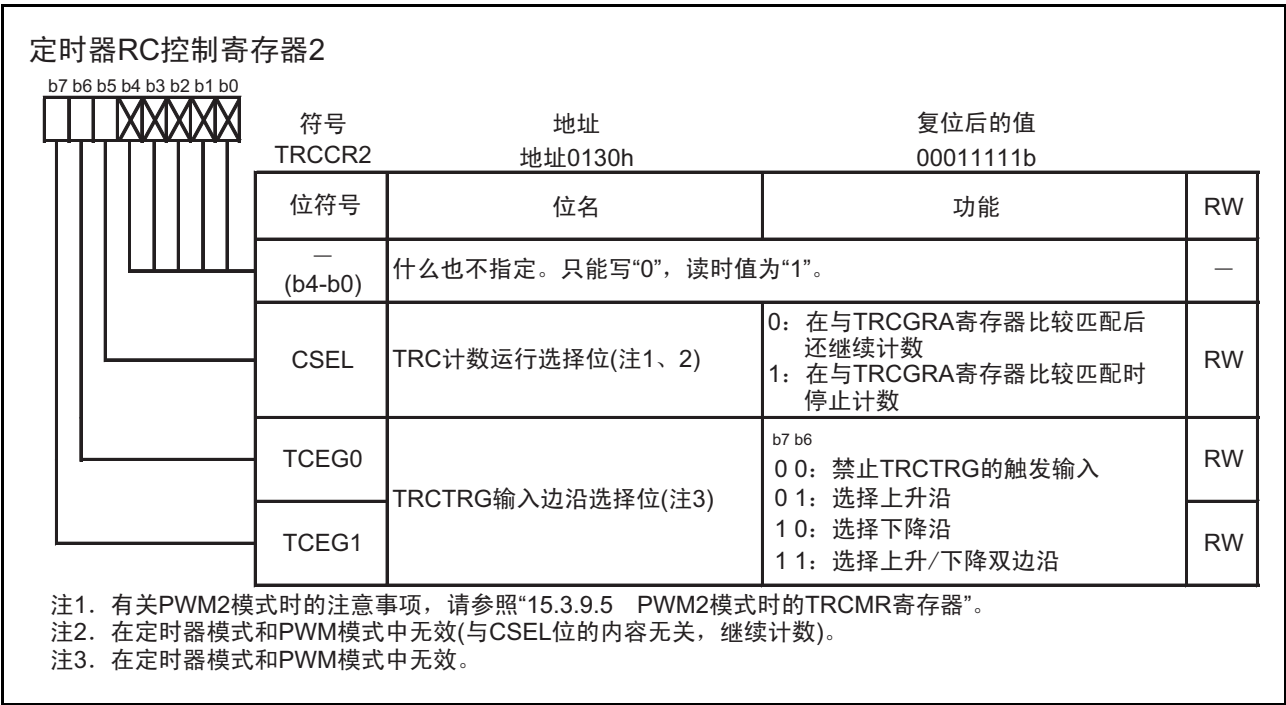
图 15.33 TRCCR2 寄存器
