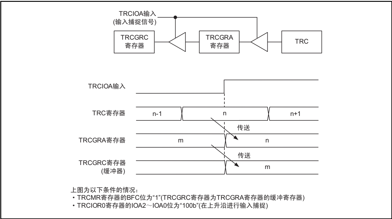
图 15.38 输入捕捉功能的缓冲器运行
