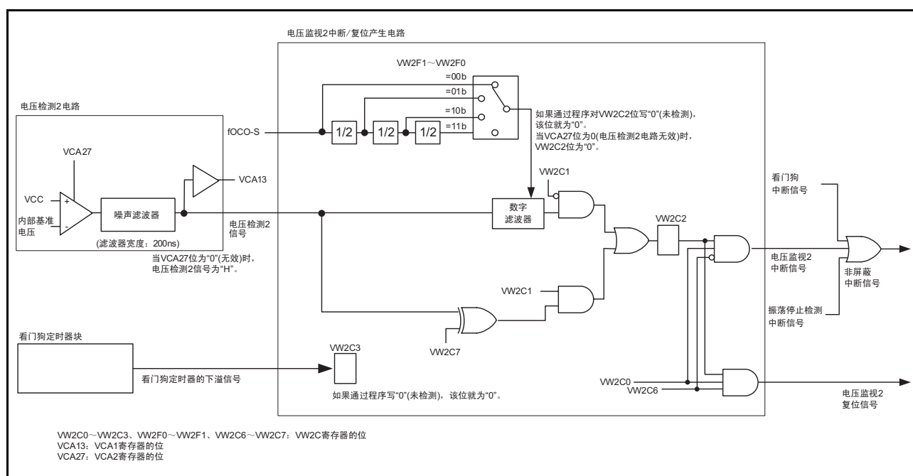
图 7.3 电压监视 2 中断 / 复位产生电路的框图
