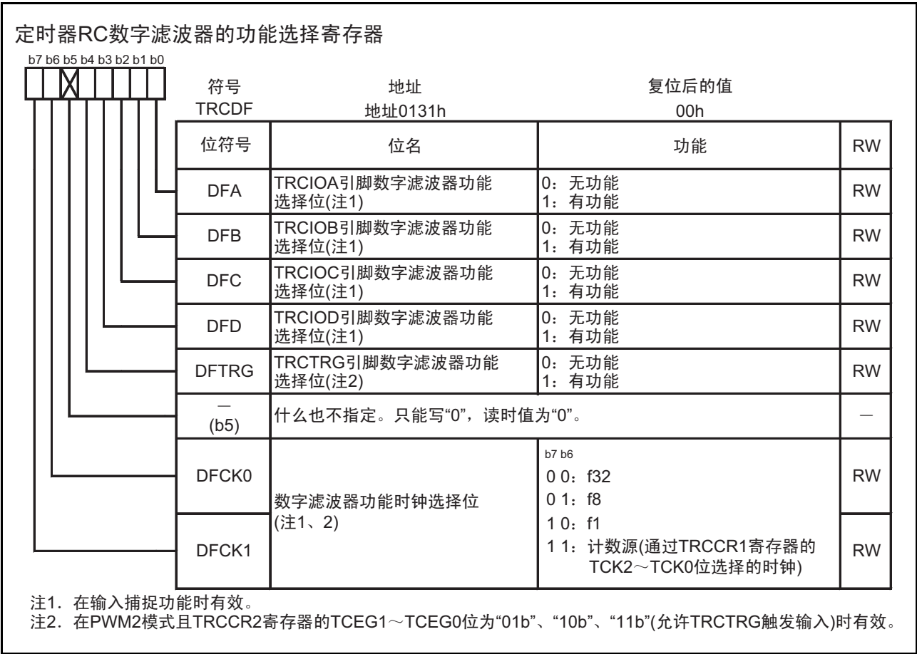
图 15.34 TRCDF 寄存器
