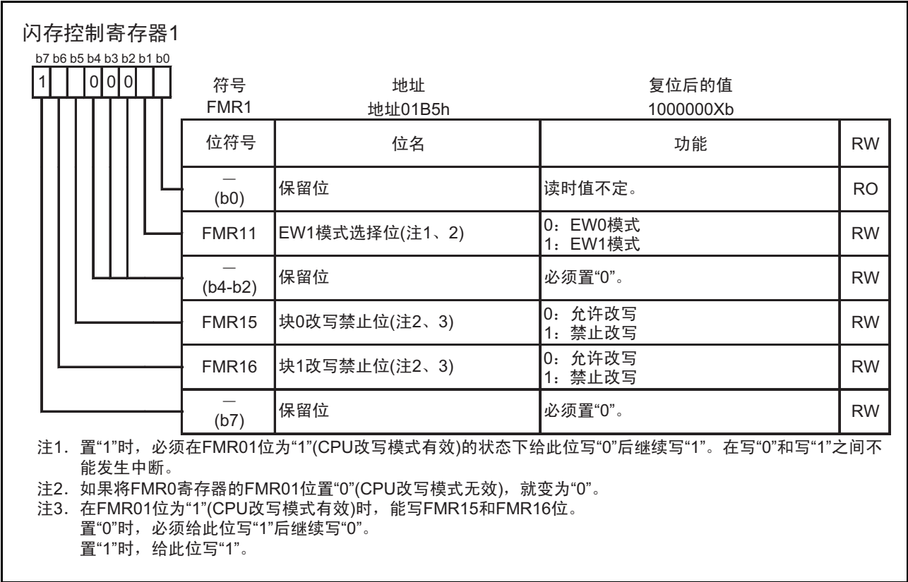
图 21.6 FMR1 寄存器
