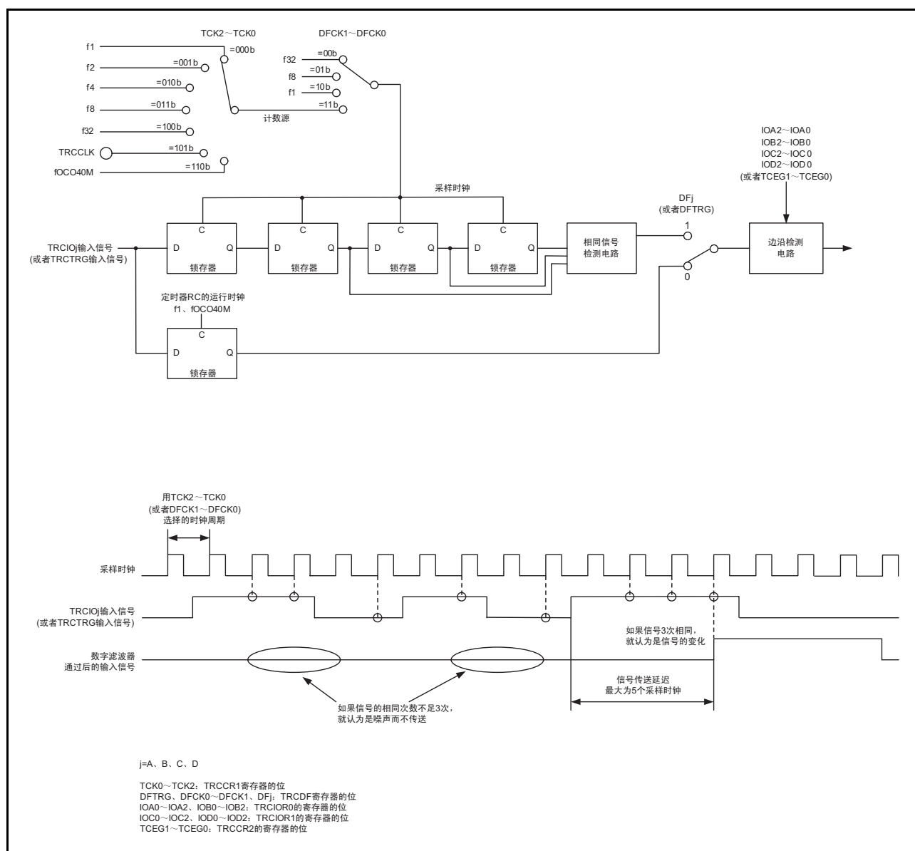
图 15.40 数字滤波器的框图
