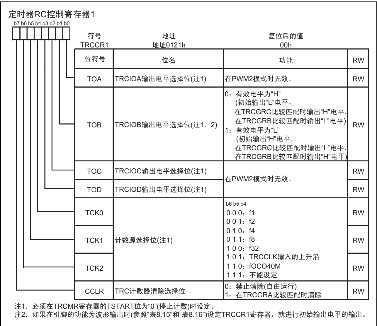
图 15.56 PWM2 模式时的 TRCCR1 寄存器
