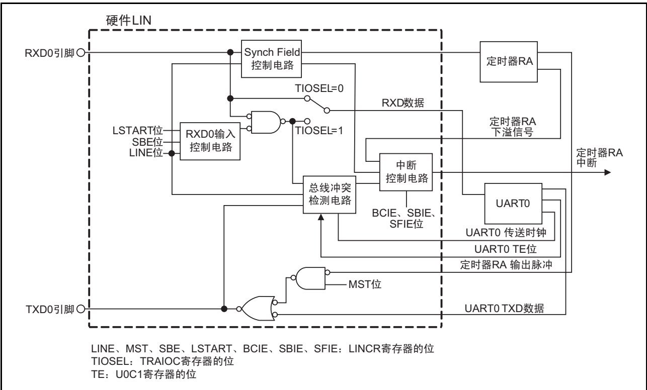
图 17.1 硬件 LIN 的框图
