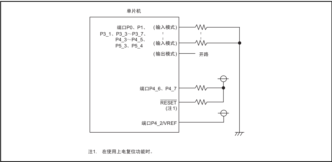
图 8.13 未使用引脚的处理例子
