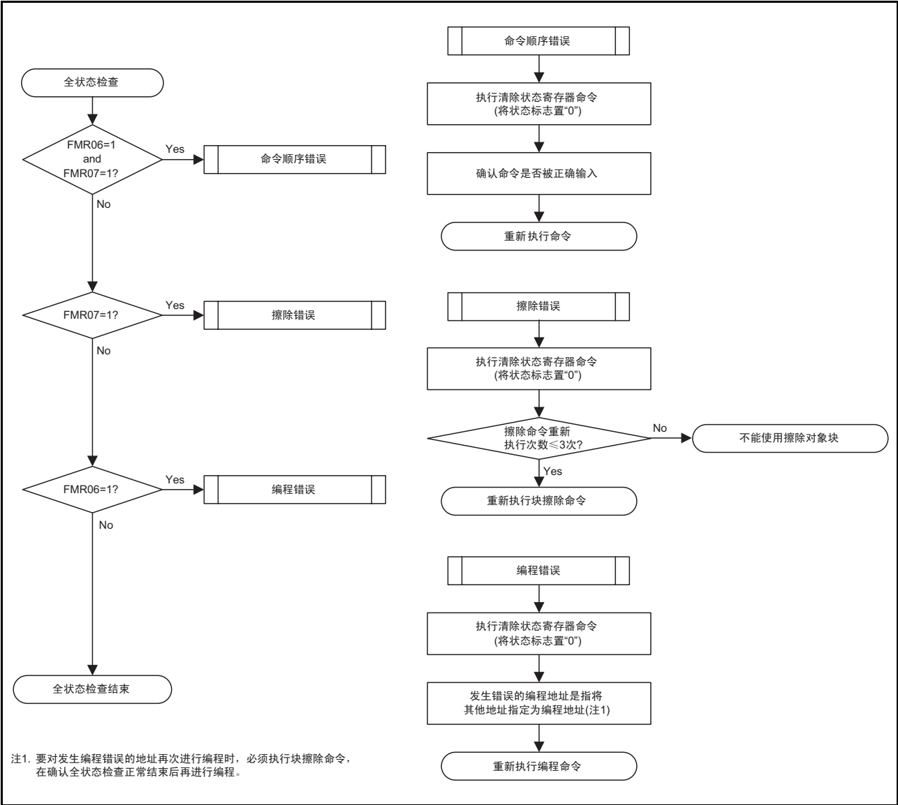
图 21.16 全状态检查流程图和发生各错误时的处理方法
