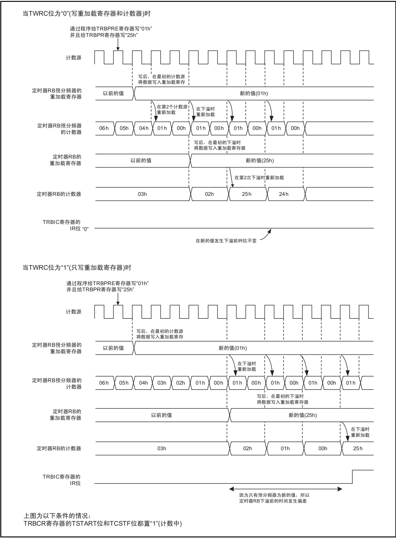
图 15.17 在定时器 RB 计数中改写计数值的运行例子
