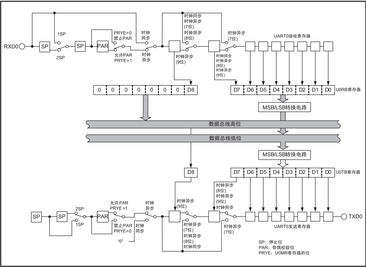
图 16.2 发送 / 接收部的框图
