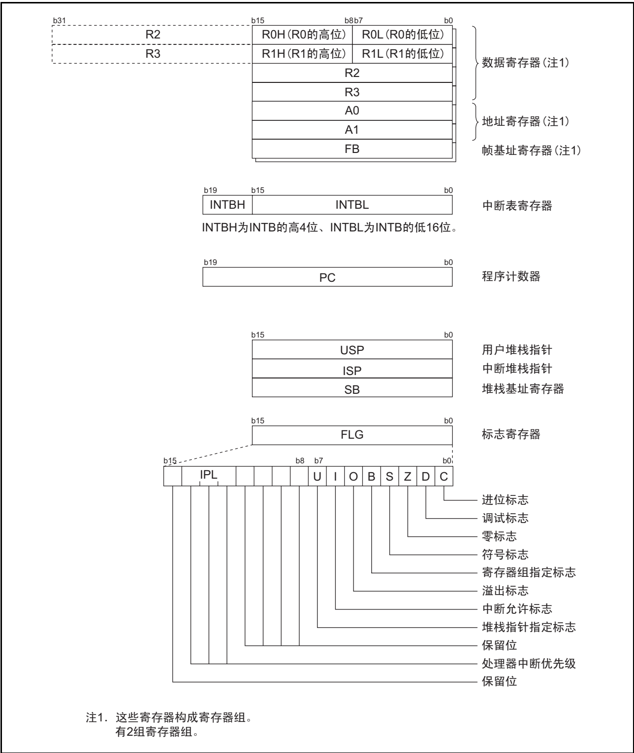
图 3.1 CPU 的寄存器
