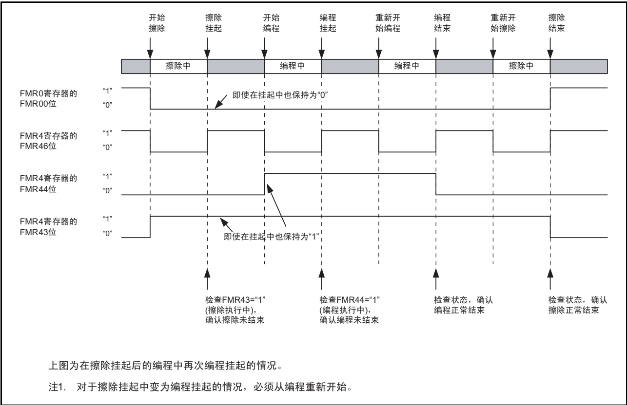
图 21.8 挂起运行的相关时序
