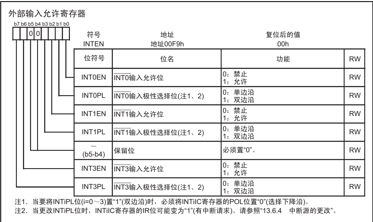
图 13.12 INTEN 寄存器
