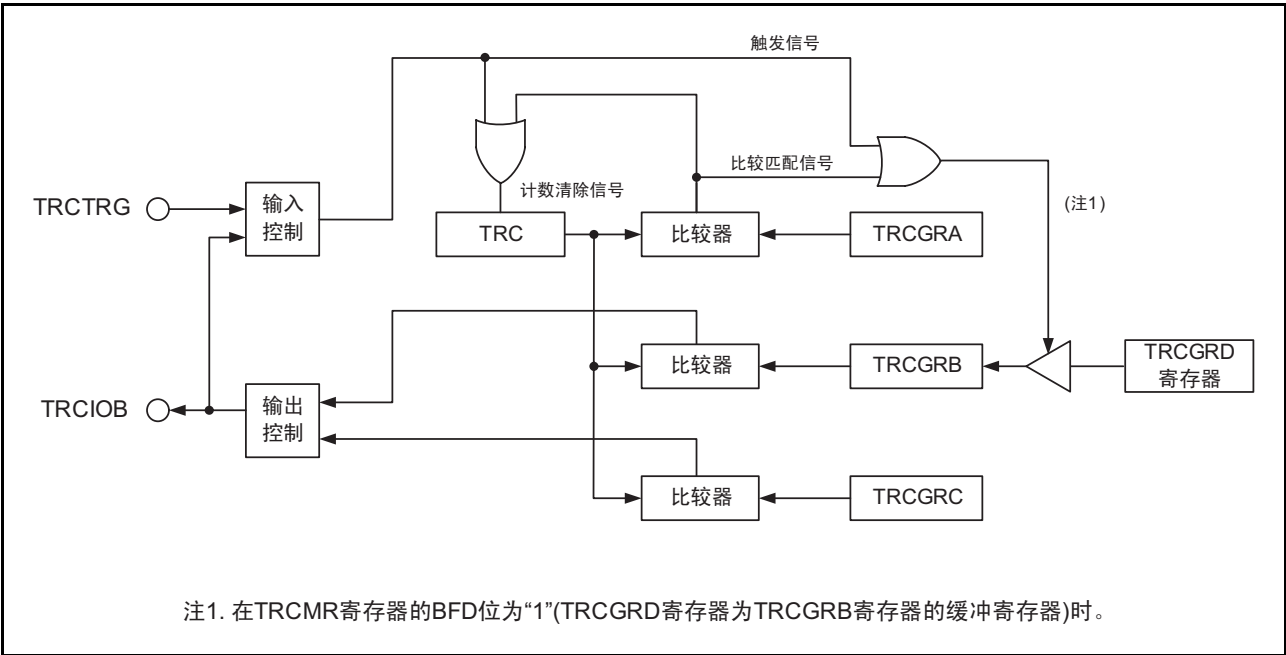
图 15.55 PWM2 模式的框图
