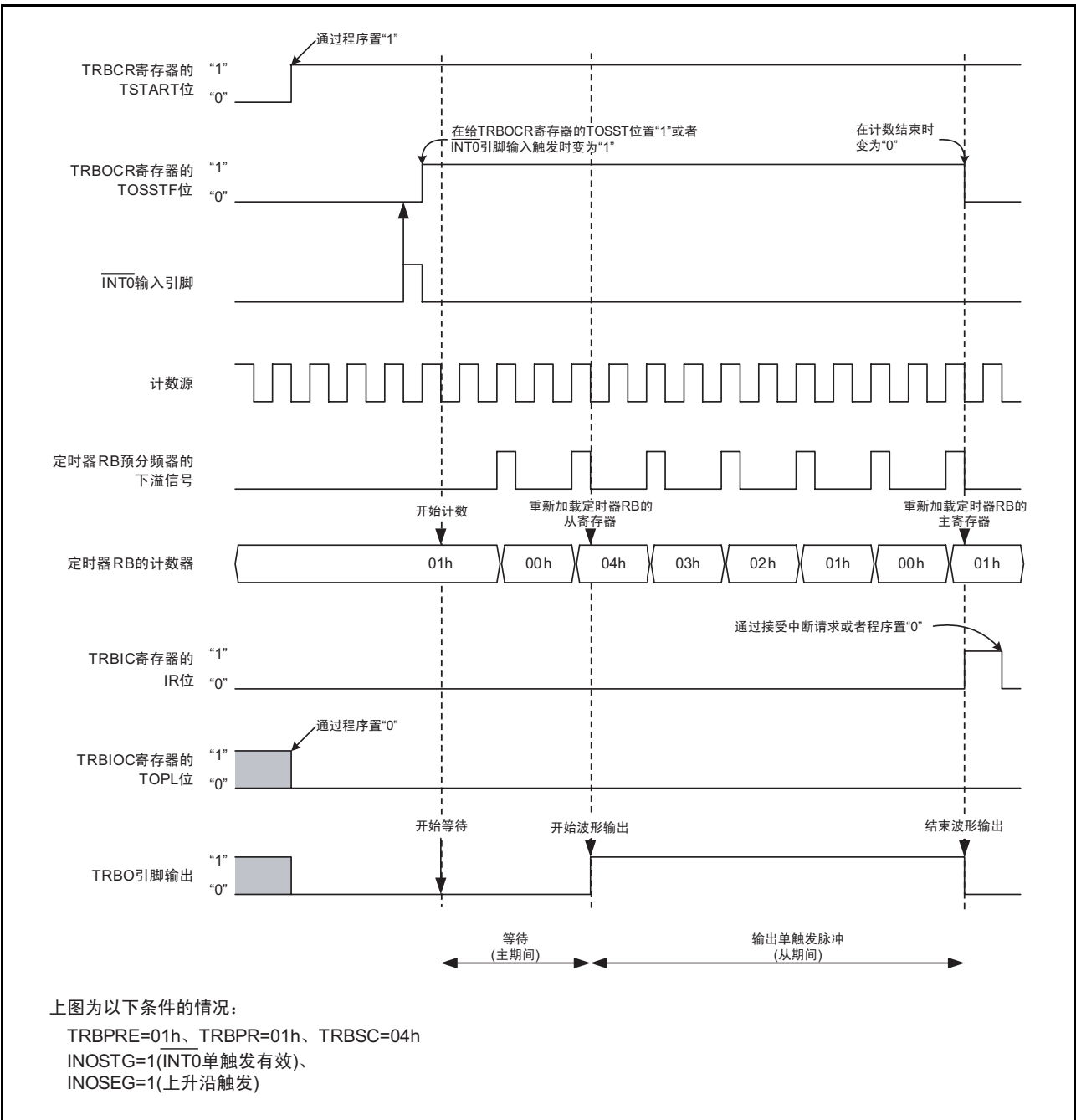
图 15.23 可编程等待单触发生模式时的运行例子
