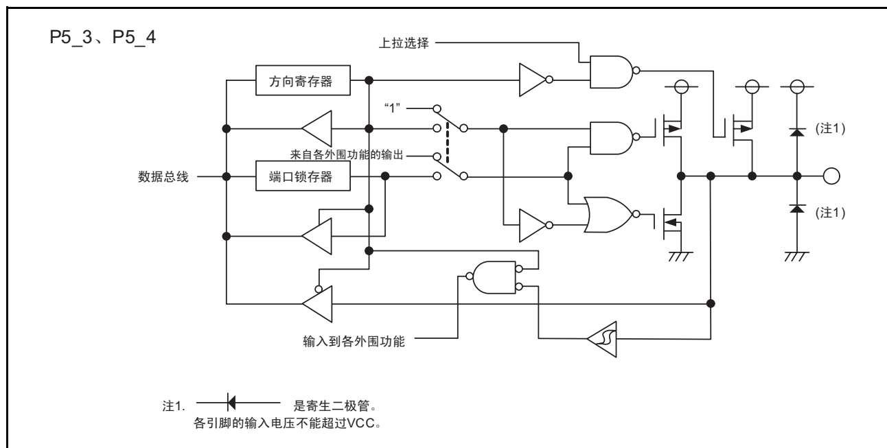
图 8.5 可编程输入 / 输出端口的结构 (5)
