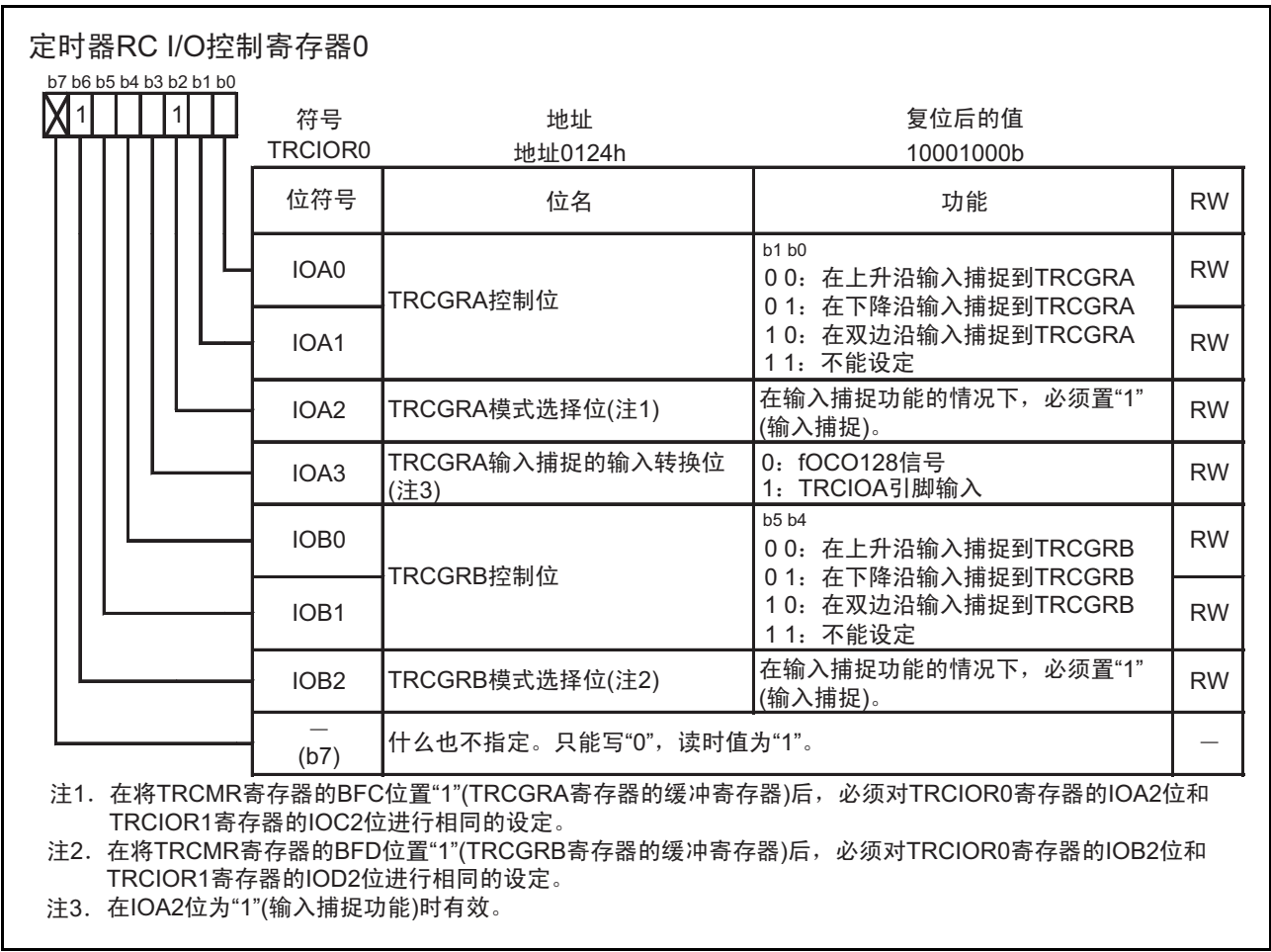
图 15.43 输入捕捉功能时的 TRCIOR0 寄存器
