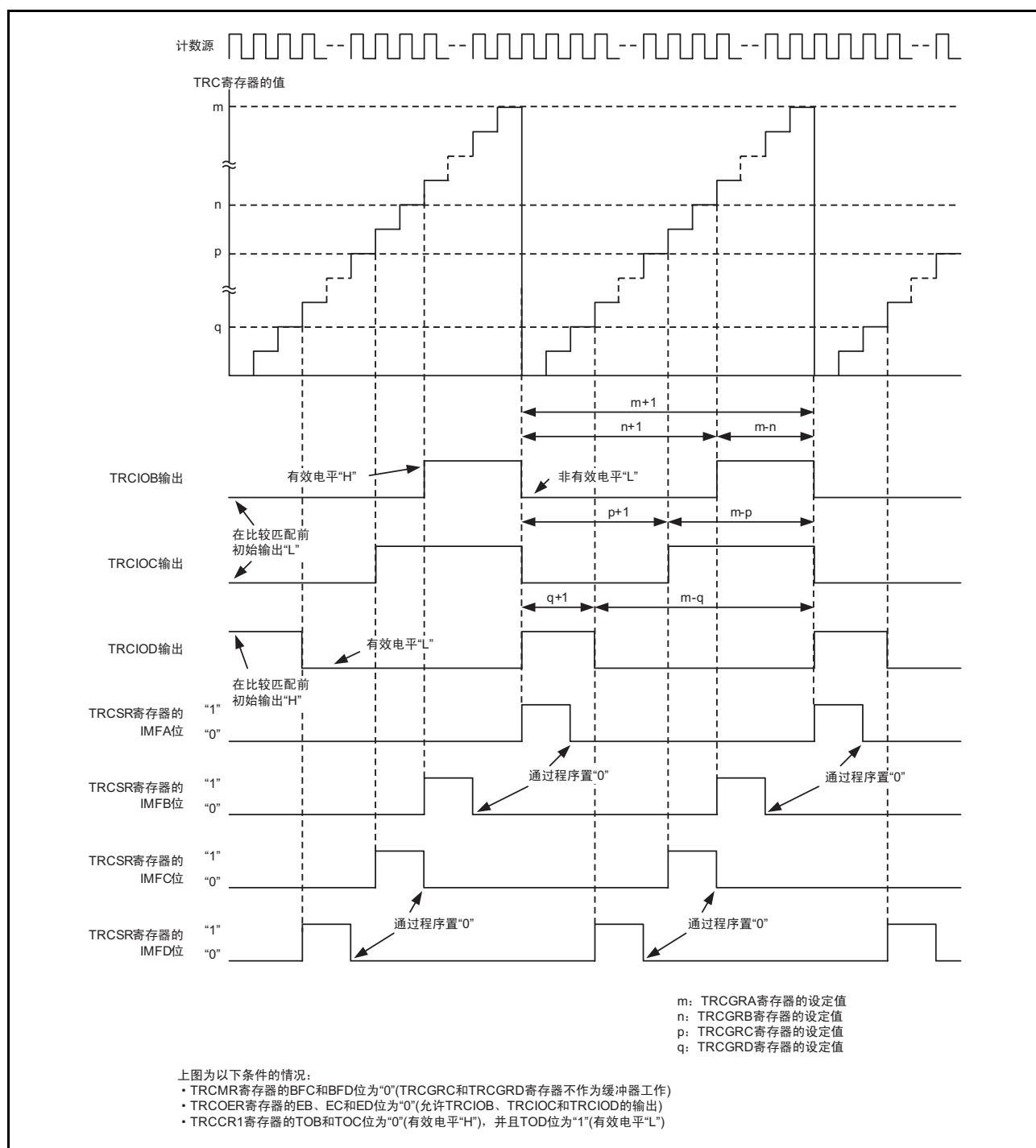
图 15.53 PWM 模式时的运行例子
