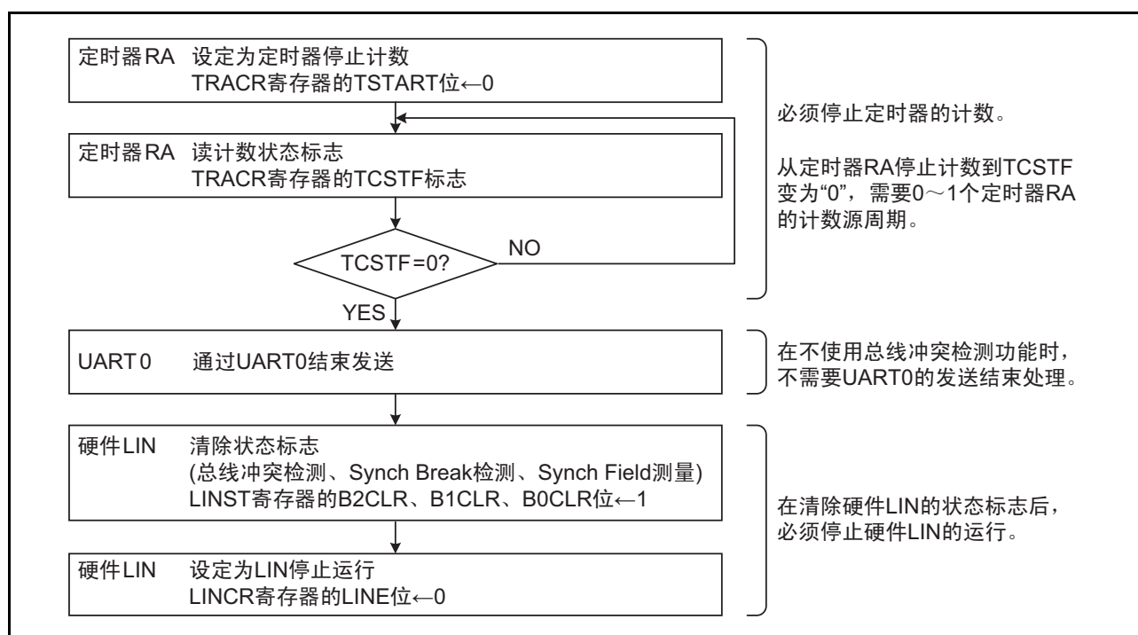
图 17.12 LIN 通信结束的流程图例子
