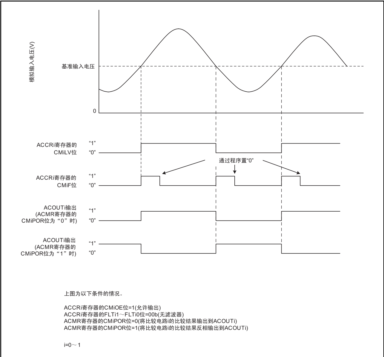
图 20.4 比较电路 i ( i=0 \sim 1 ) 的运行例子
