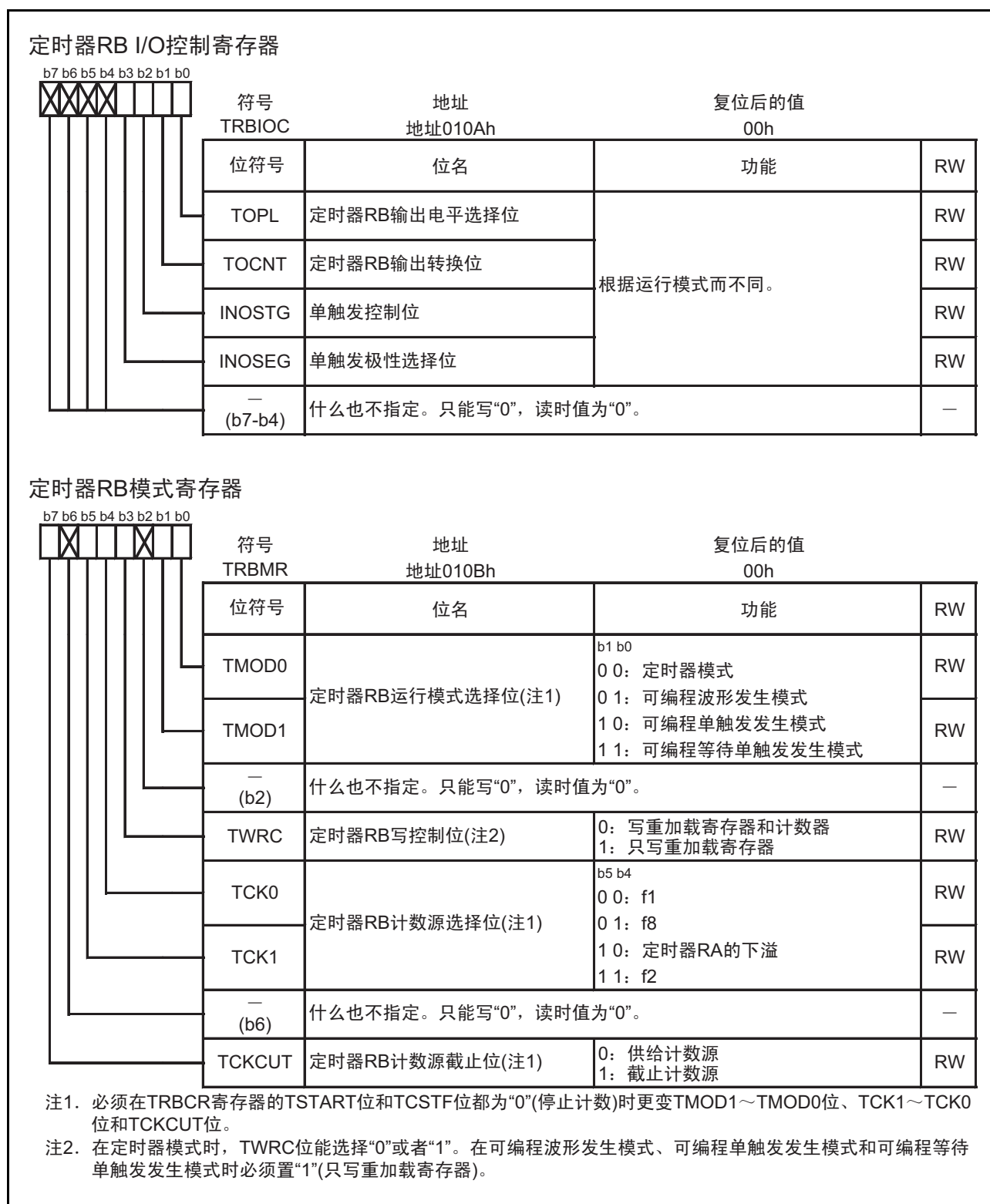
图 15.14 TRBIOC 和 TRBMR 寄存器
