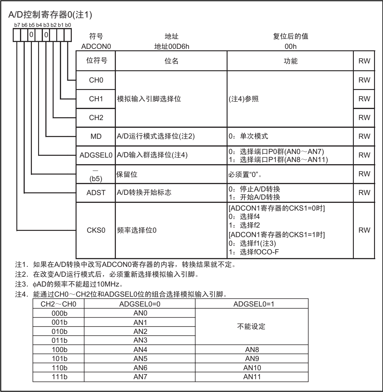
图 18.4 单次模式时的 ADCON0 寄存器
