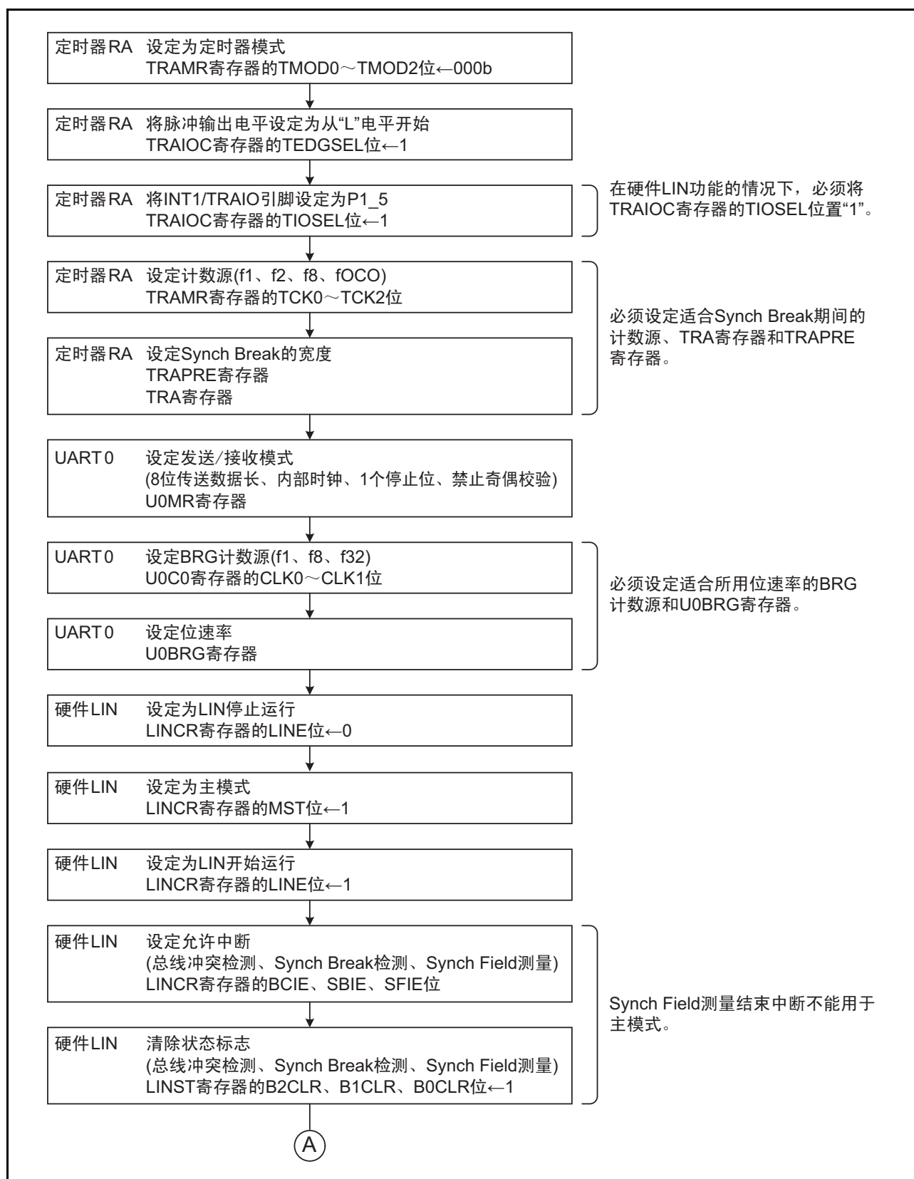
图 17.5 标题段的发送流程图例子 (1)
