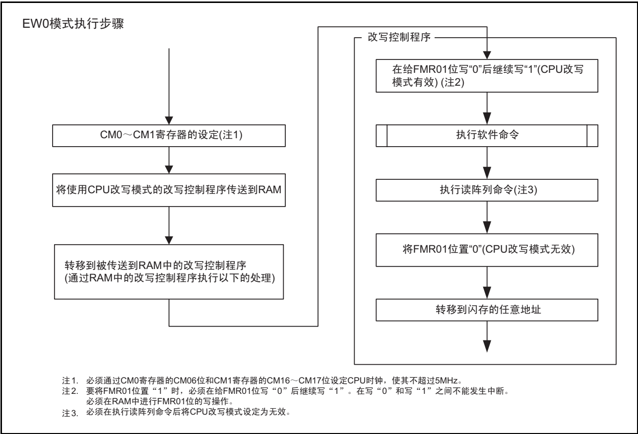
图 21.9 EW0 模式的设定和解除方法
