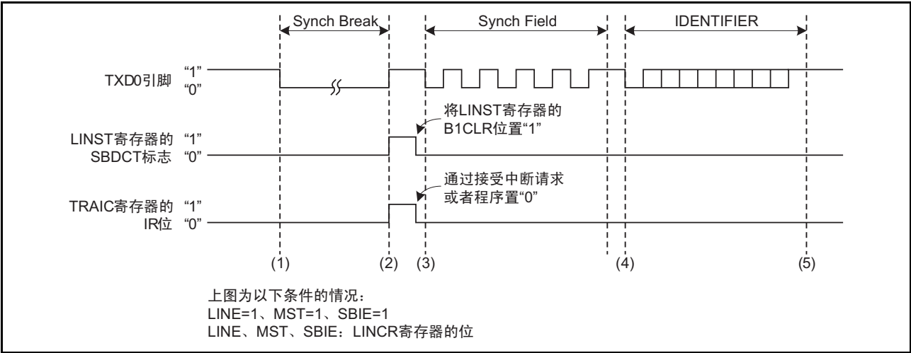
图 17.4 标题段的发送运行例子
