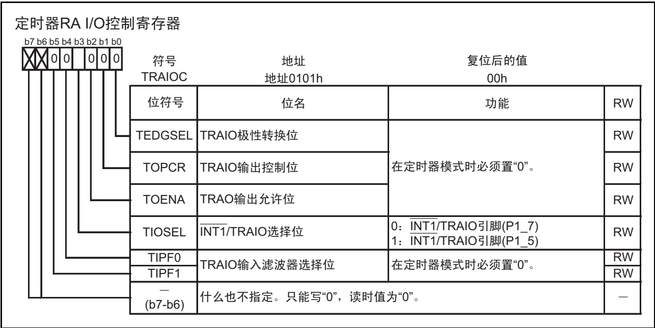
图 15.4 定时器模式时的 TRAIOC 寄存器
