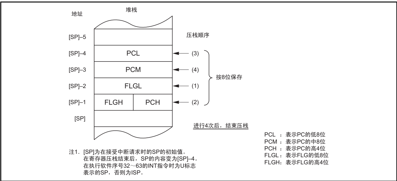
图 13.9 寄存器的压栈
