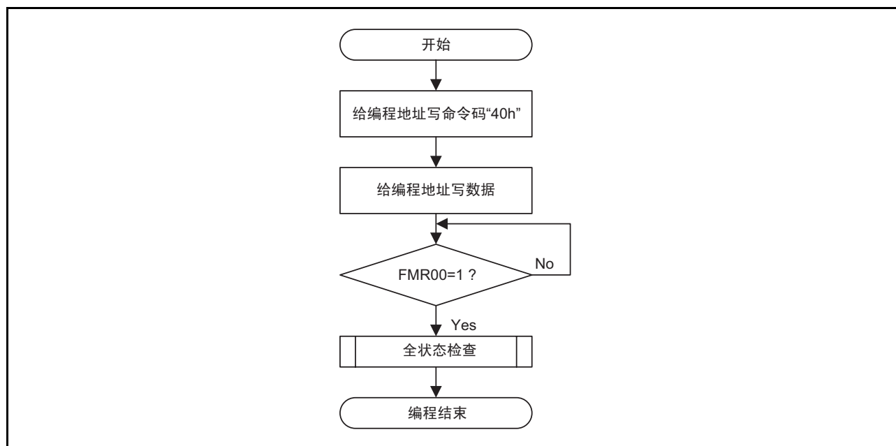
图 21.12 编程流程图（禁止挂起功能时）
