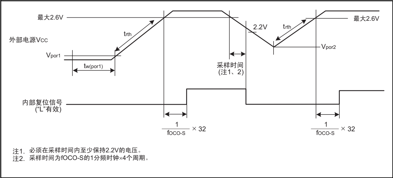
图 22.3 复位电路的电特性
