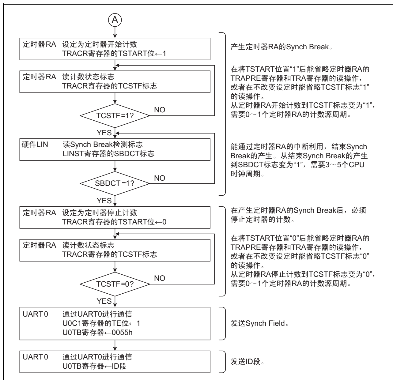
图 17.6 标题段的发送流程图例子 (2)
