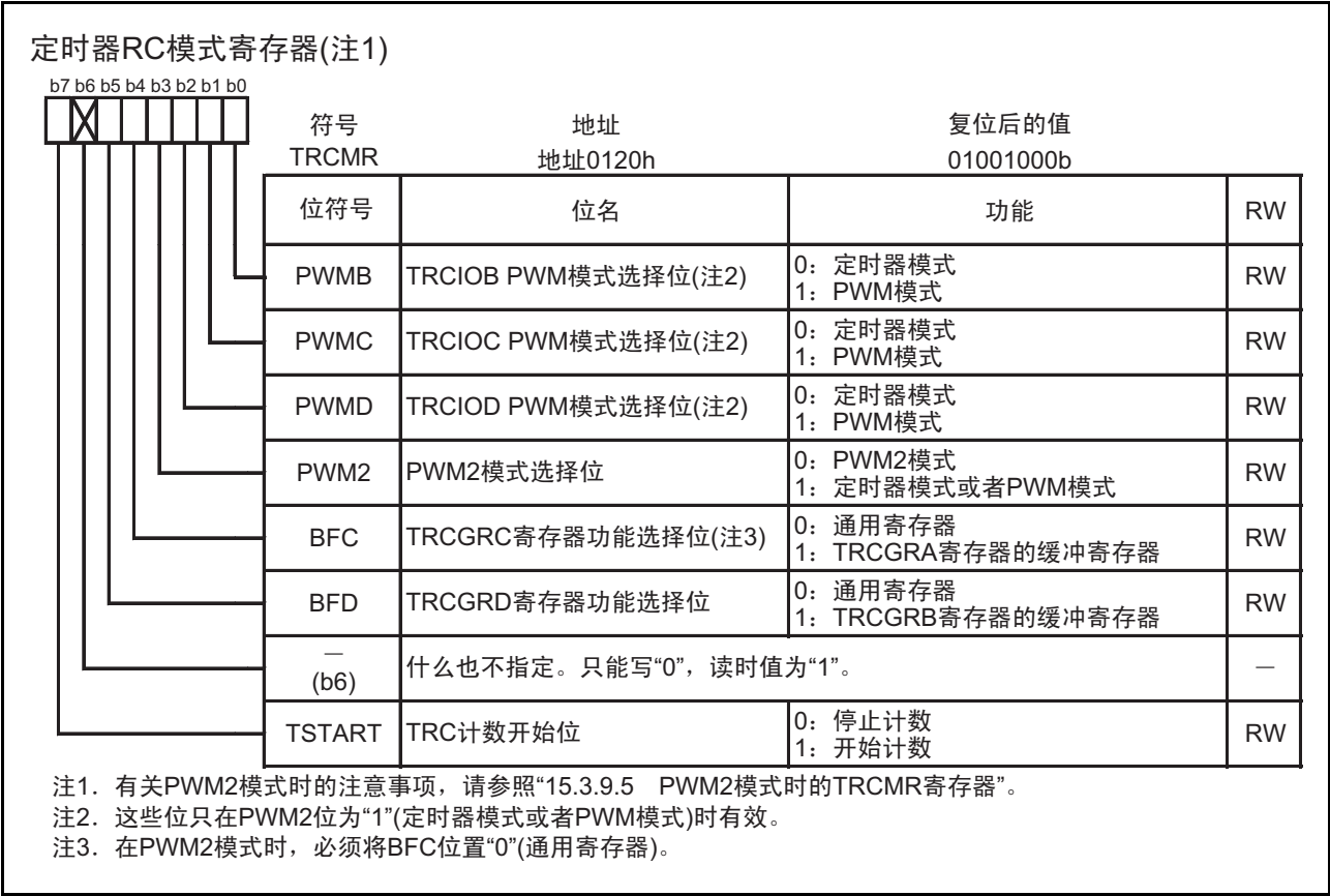
图 15.27 TRCMR 寄存器
