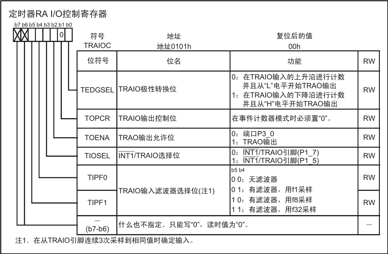
图 15.7 事件计数器模式时的 TRAIOC 寄存器
