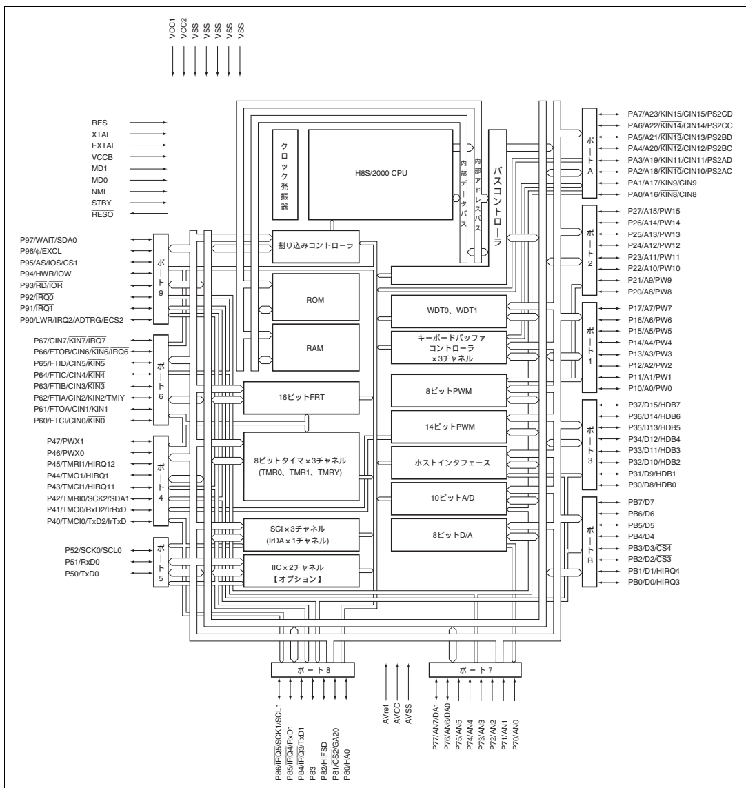
図 1.1 (b) H8S/2147N の内部ブロック図
