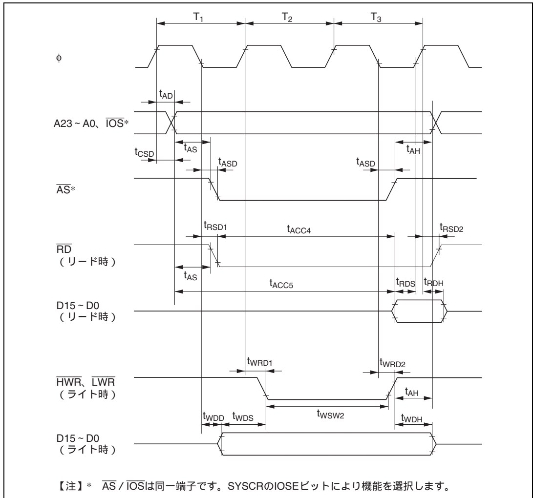
図 26.11 基本バスタイミング / 3 ステートアクセス
