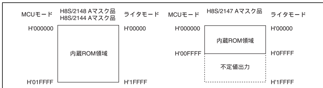
図 23.15 ライターモード時のメモリマップ
