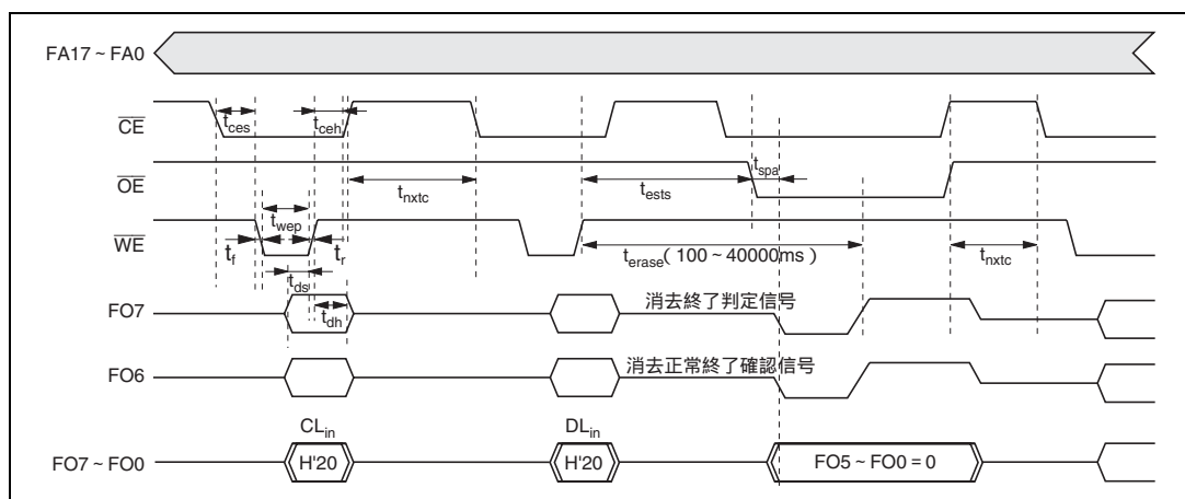
図 23.21 自動消去モードのタイミング波形
