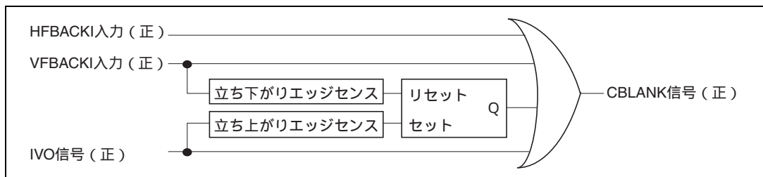
図 13.9 CBLANK 出力波形生成
