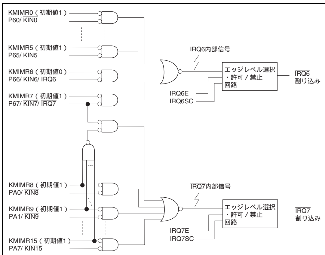
図 5.2 IRQ7、IRQ6 割り込みと KIN15~KIN0 割り込み、KMIMR、KMIMRA との関係
