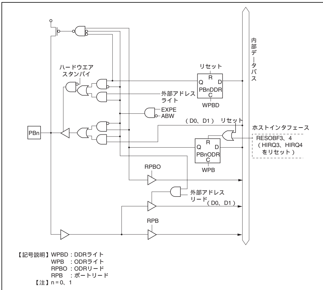
図 C.37 ポート B ブロック図 (PB0、PB1 端子)
