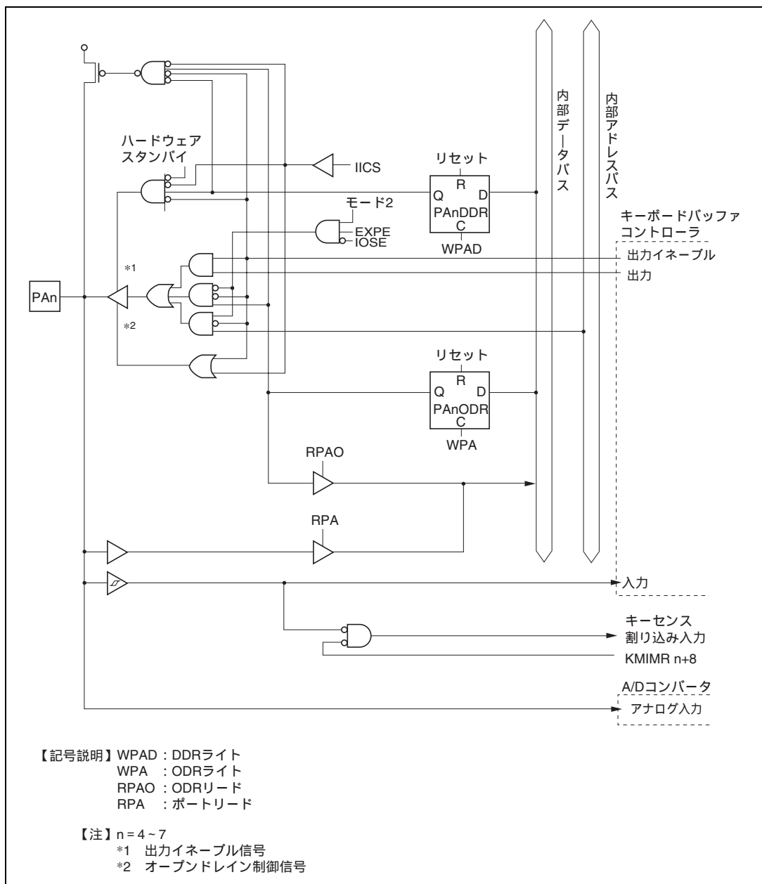
図 C.36 ポート A ブロック図 (PA4 ~ PA7 端子)
