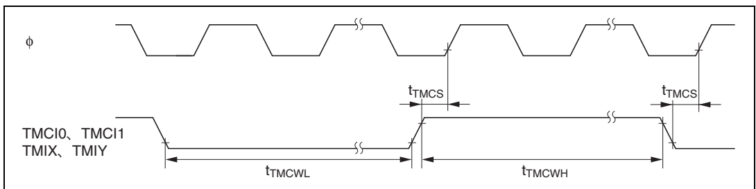
図 26.19 8 ビットタイマクロック入力タイミング
