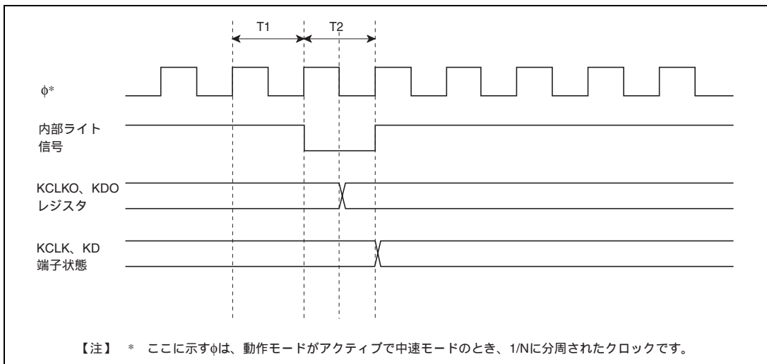
図 17.10 KCLKO、KDO のライトタイミング
