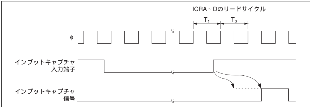
図 11.8 インプットキャプチャ信号タイミング
