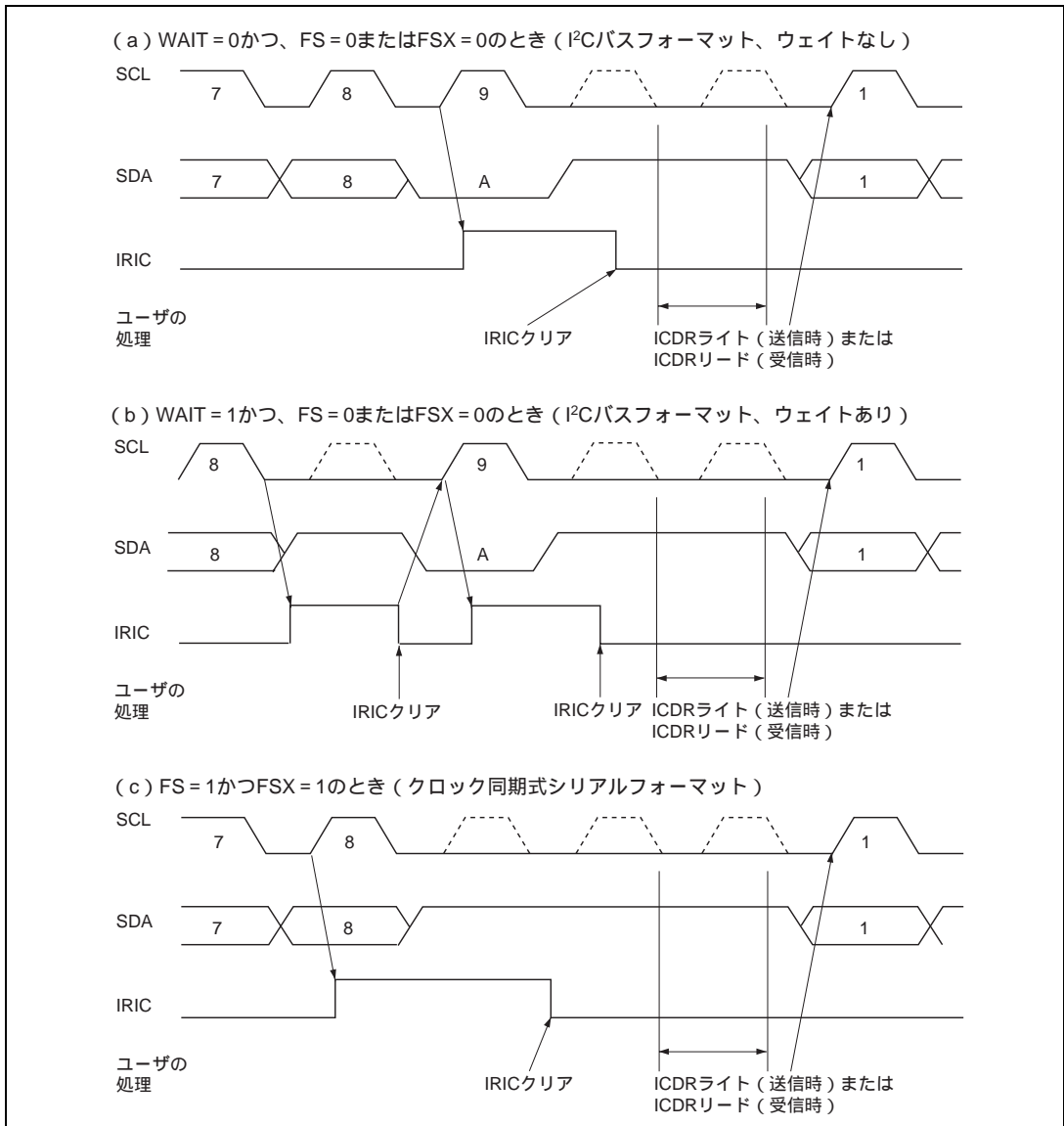
図 16.12 IRIC セットタイミングと SCL 制御
