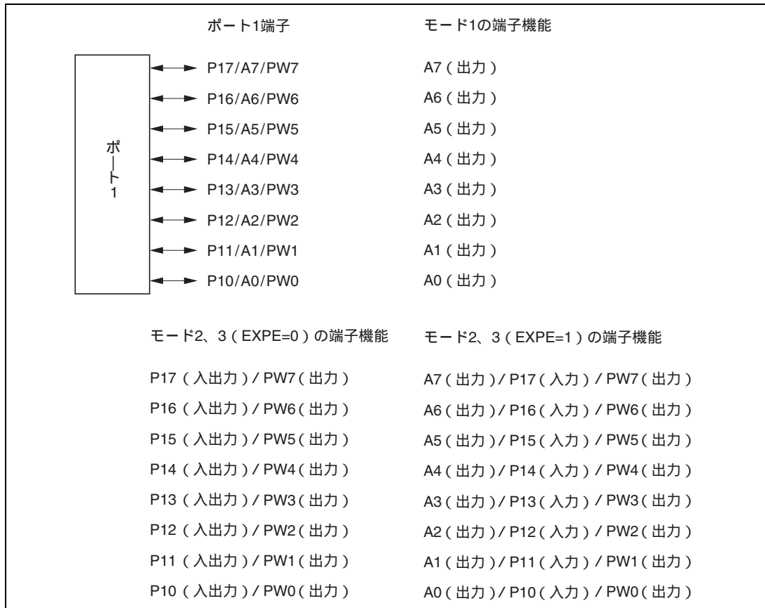
図 8.1 ポート 1 の端子機能
