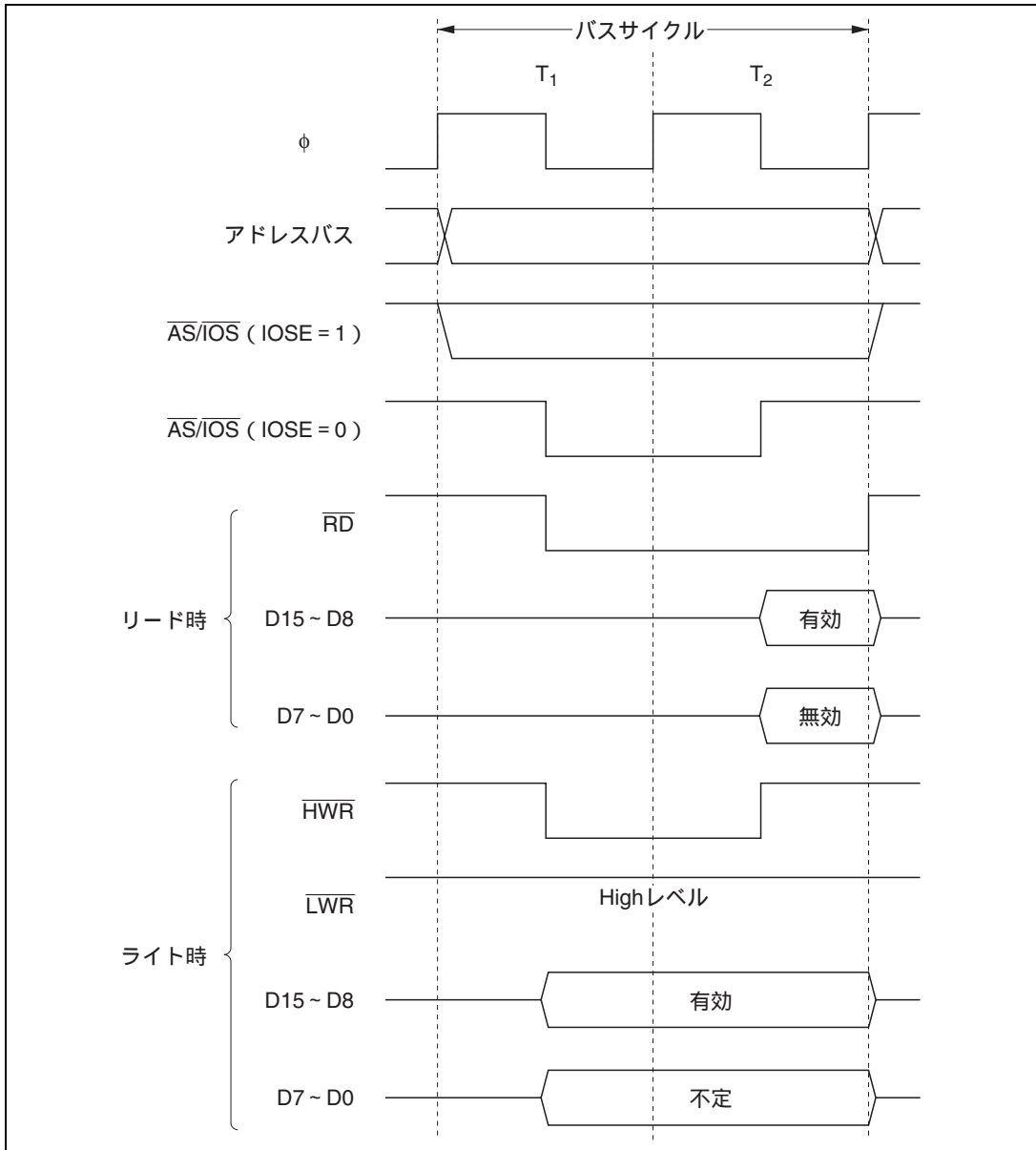
図 6.7 16ビット2ステートアクセス空間のバスタイミング(1) (偶数アドレスバイトアクセス)
