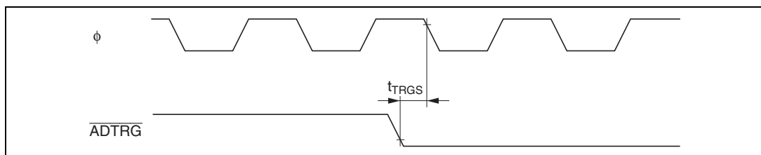
図 26.24 A/D 変換器外部トリガ入力タイミング
