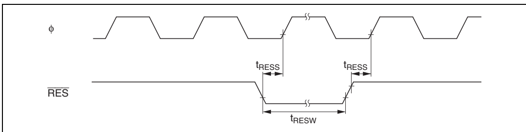
図 26.8 リセット入力タイミング
