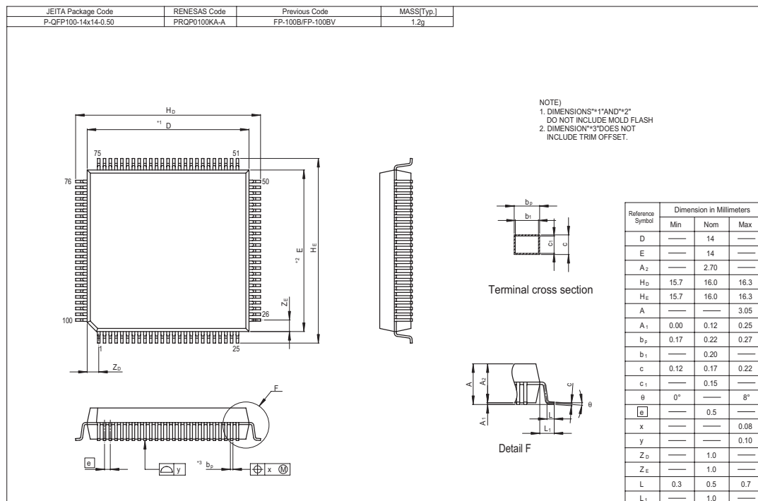
図 H.1 FP-100B の外形寸法図
