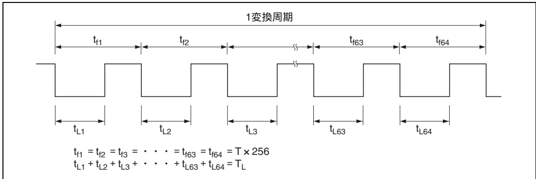
図 10.4 (2) 出力波形
