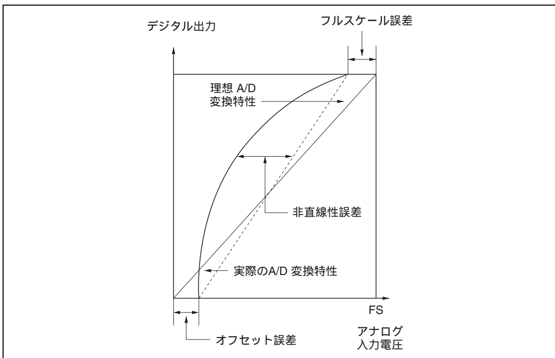
図 20.10 A/D 変換精度の定義 (2)
