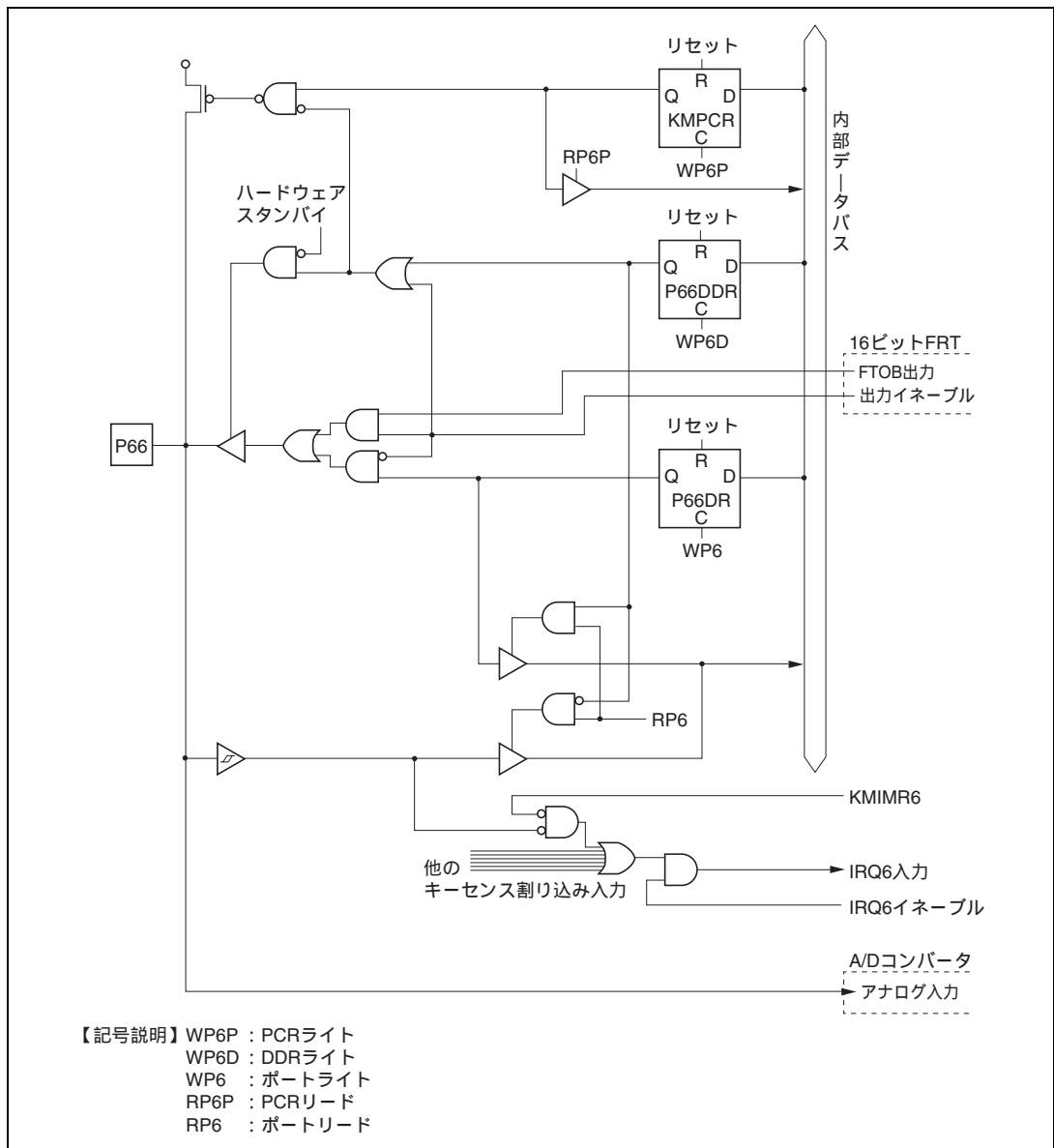
図 C.19 ポート 6 ブロック図 (P66 端子)
