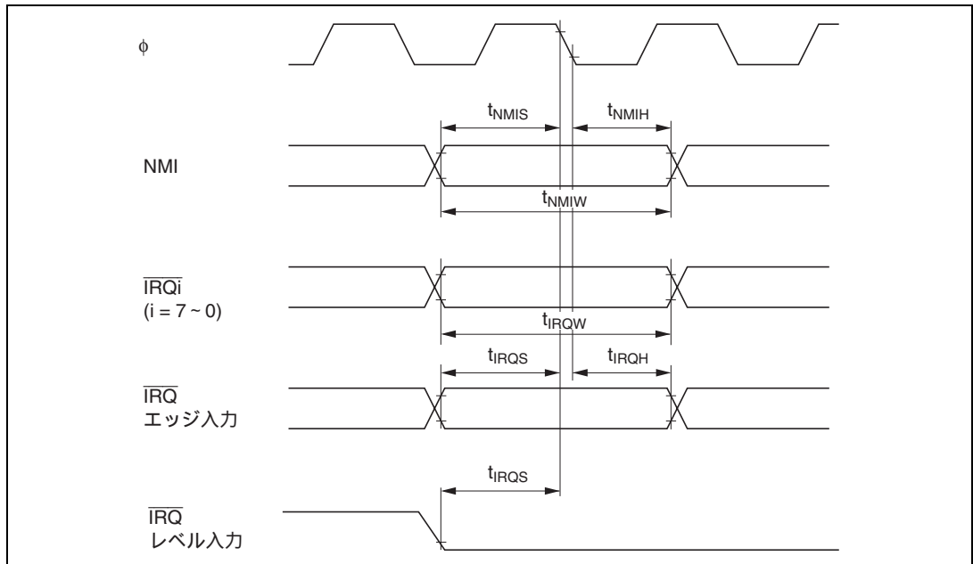
図 26.9 割り込み入力タイミング
