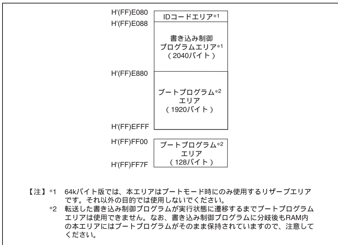
図 23.10 ブートモード時の RAM エリア
