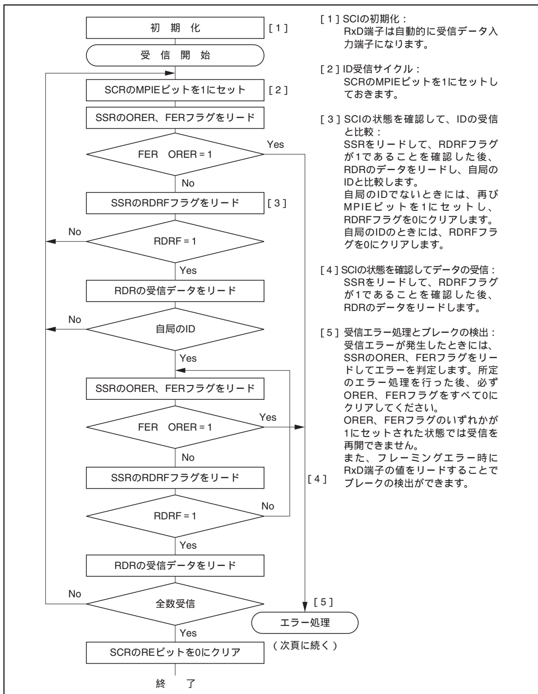
図 15.12 マルチプロセッサシリアル受信のフローチャートの例 (1)
