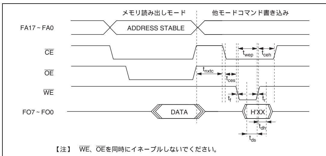
図 23.17 メモリ読み出しモードから他のモードへ遷移時のタイミング波形
