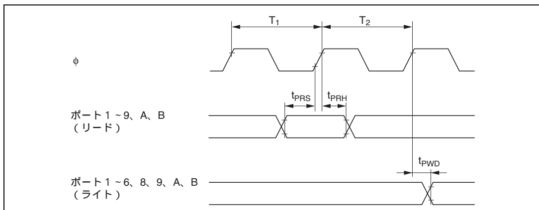
図 26.15 I/O ポート入出力タイミング
