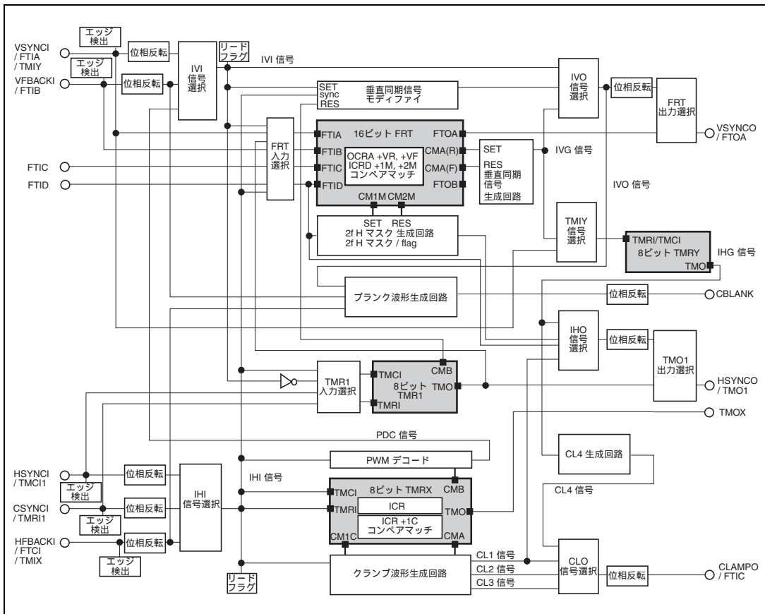
図 13.1 タイマコネクションのブロック図
