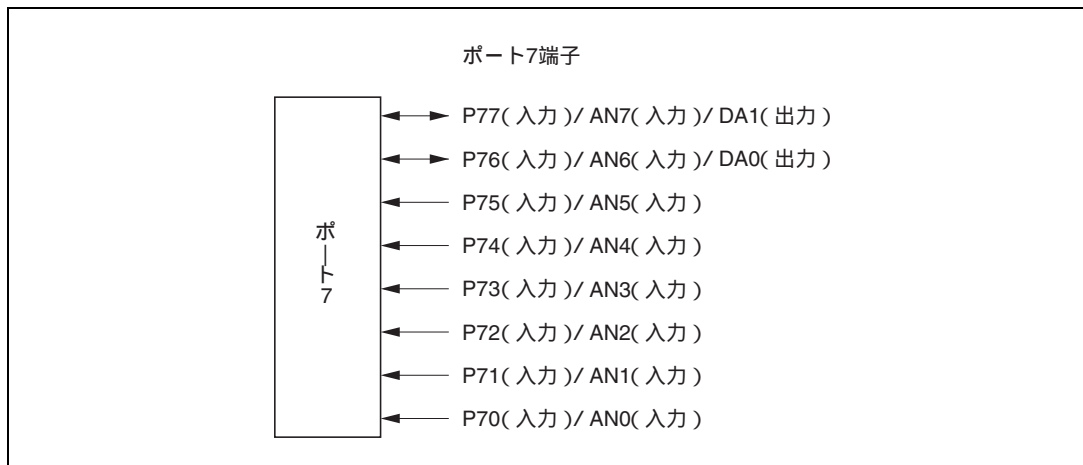
図 8.15 ポート 7 の端子機能
