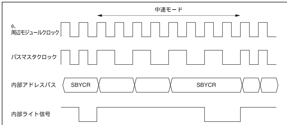
図 25.2 中速モードの遷移・解除タイミング
