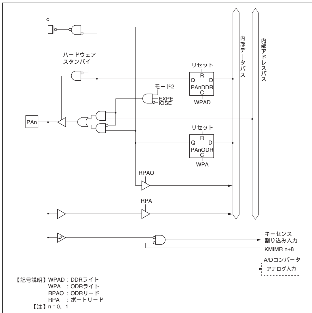
図 C.34 ポート A ブロック図 (PA0、PA1 端子)
