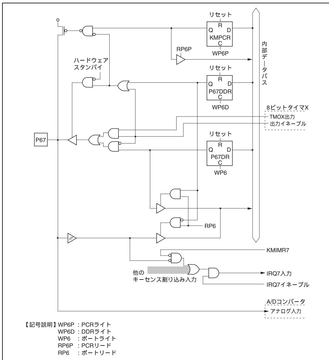
図 C.20 ポート 6 ブロック図 (P67 端子)
