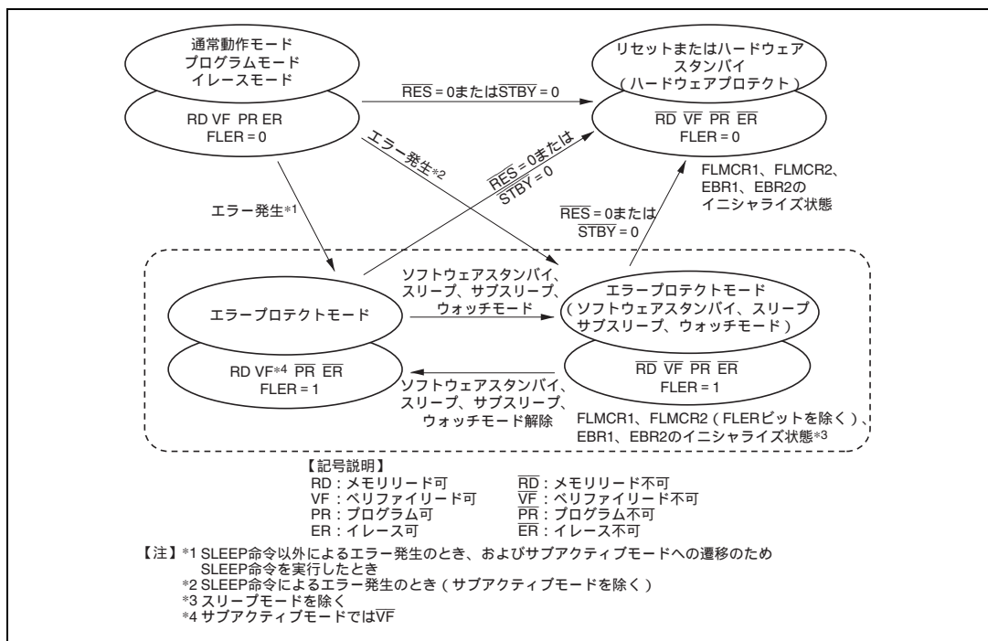
図 23.14 フラッシュメモリの状態遷移図
