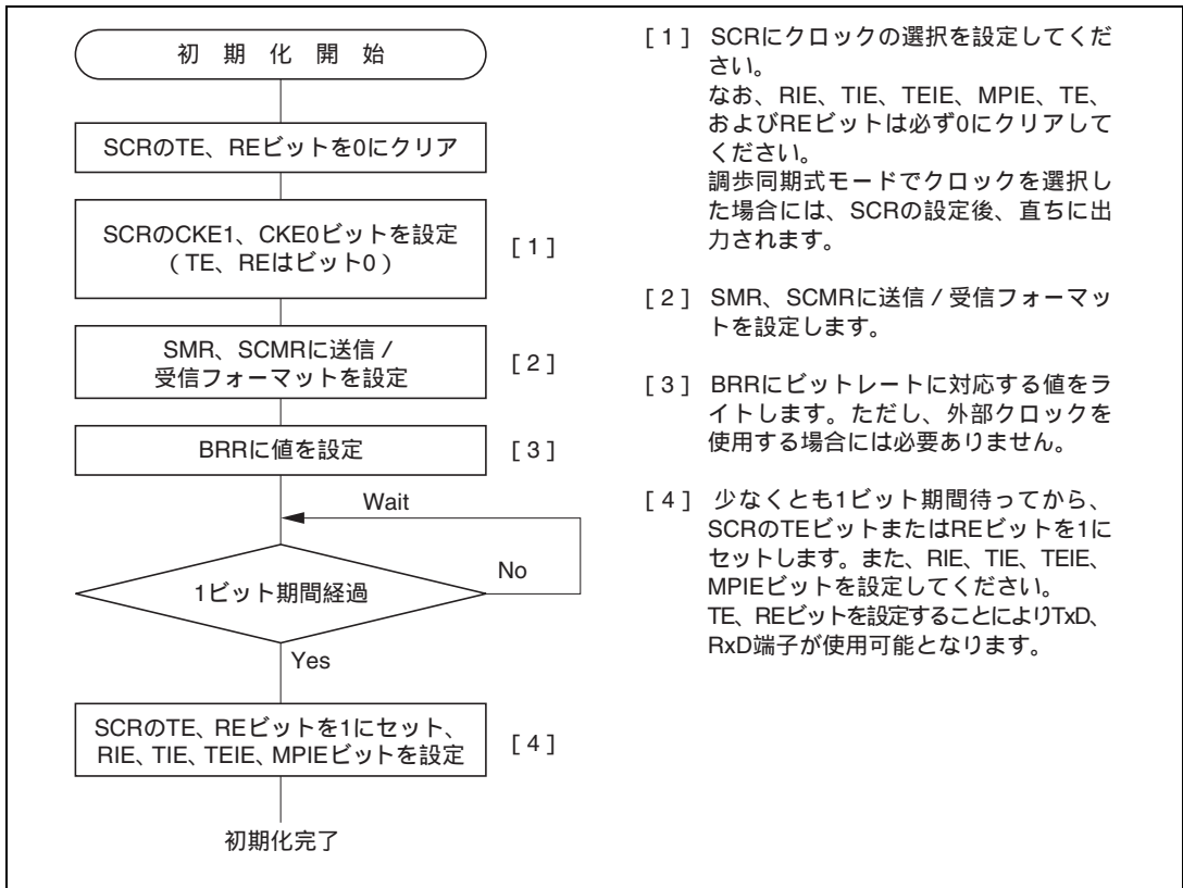
図 15.4 SCI の初期化フローチャートの例
