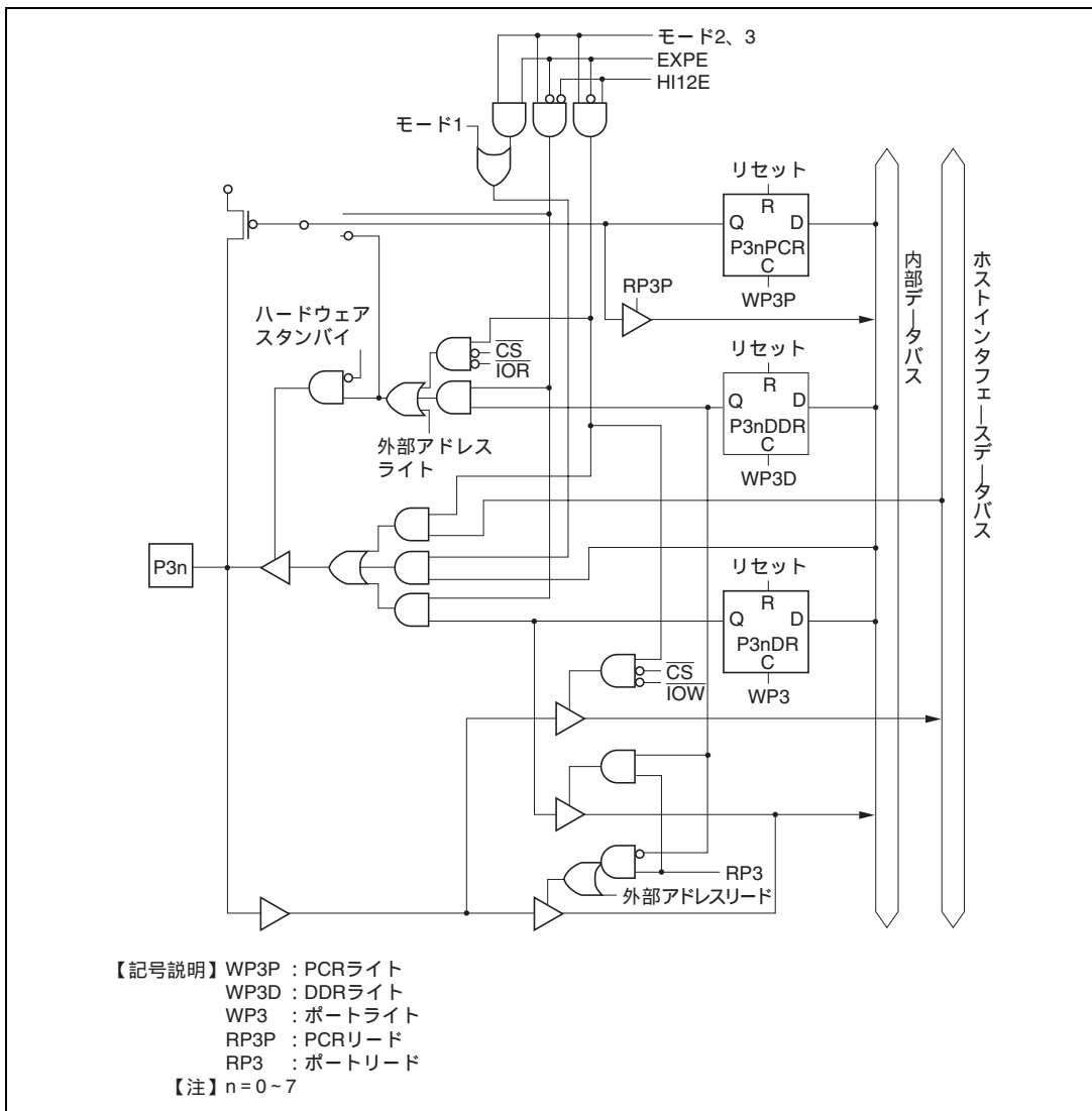
図 C.5 ポート 3 ブロック図
