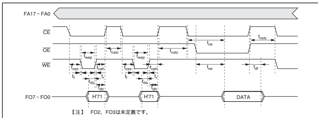
図 23.22 ステータス読み出しモードのタイミング波形
