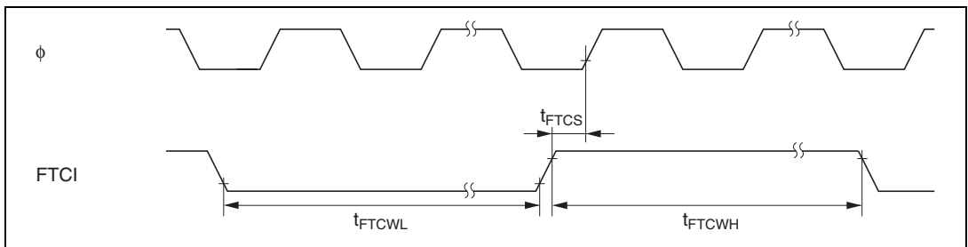
図 26.17 FRT クロック入力タイミング
