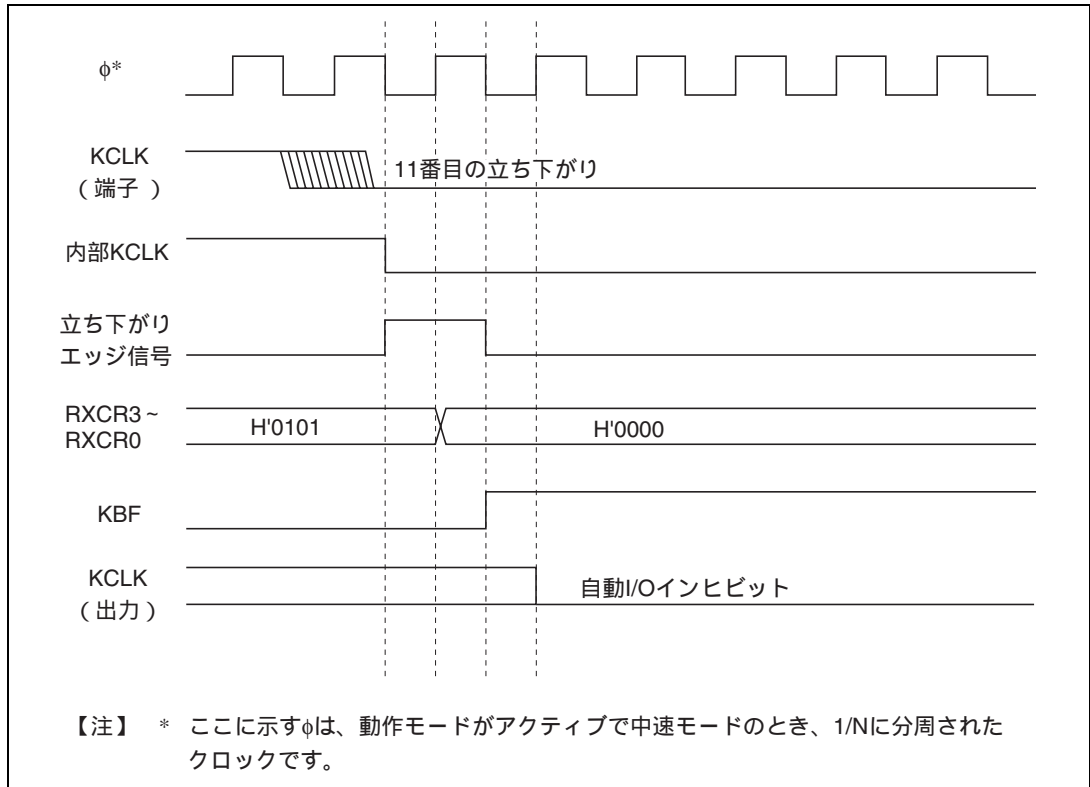
図 17.11 KBF セットと KCLK 自動 I/O インヒビット生成のタイミング
