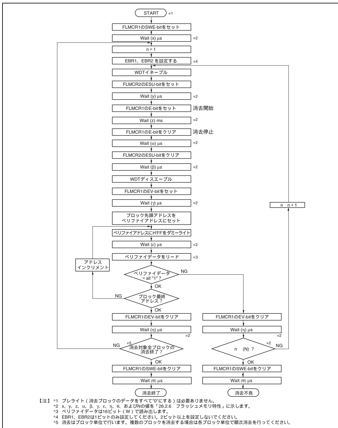
図 23.13 イレース/イレースペリファイフロー (単一ブロック消去)
