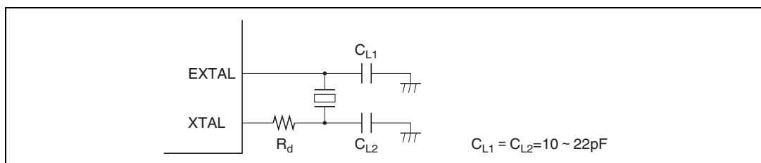
図 24.2 水晶発振子の接続例
