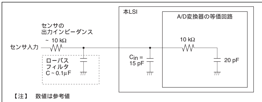
図 20.11 アナログ入力回路の例
