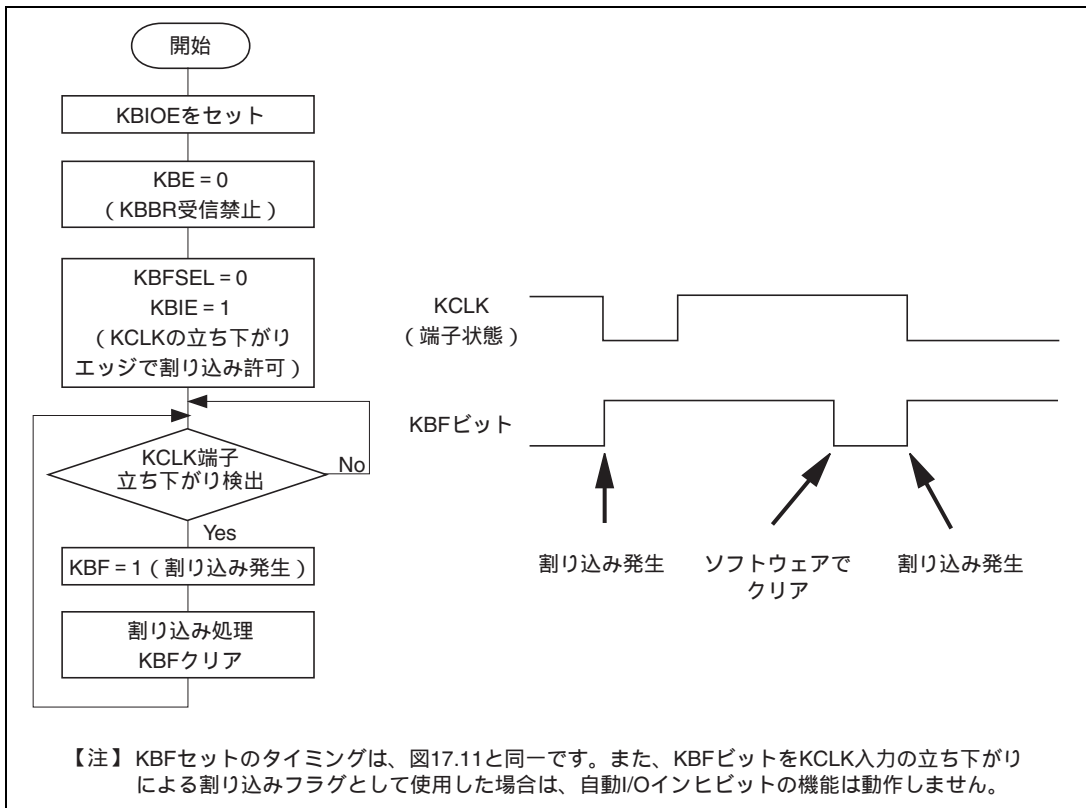
図 17.13 KCLK 入力の立ち下がりによる割り込み動作例
