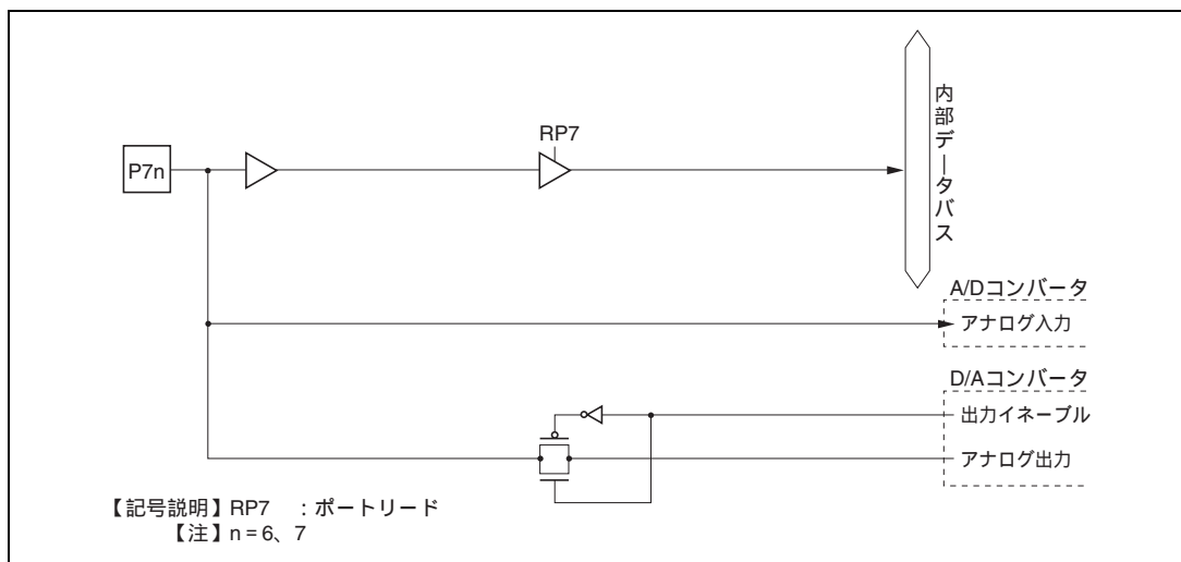
図 C.22 ポート7ブロック図 (P76、P77 端子)
