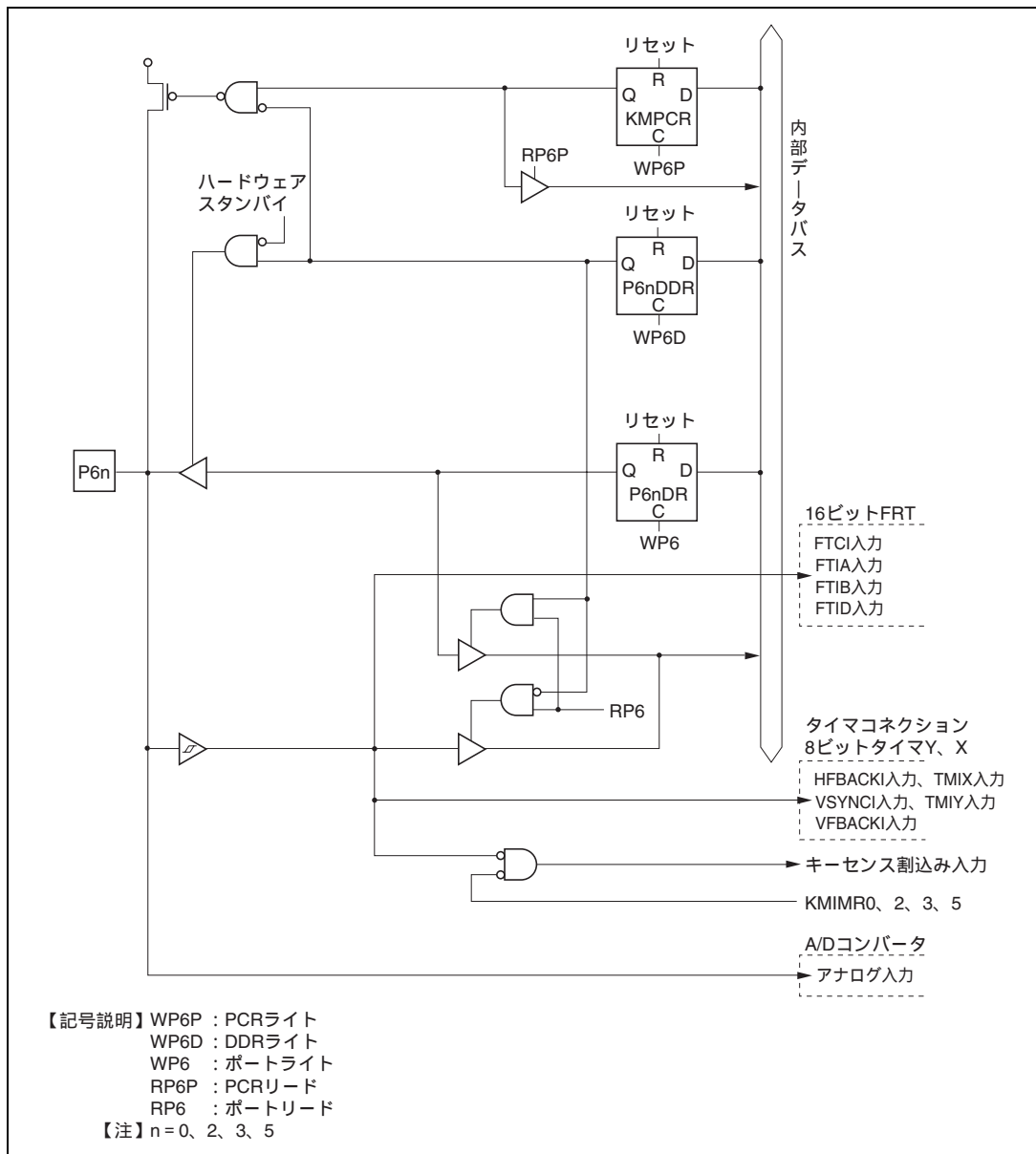
図 C.16 ポート 6 ブロック図 ( P60、P62、P63、P65 端子 )
