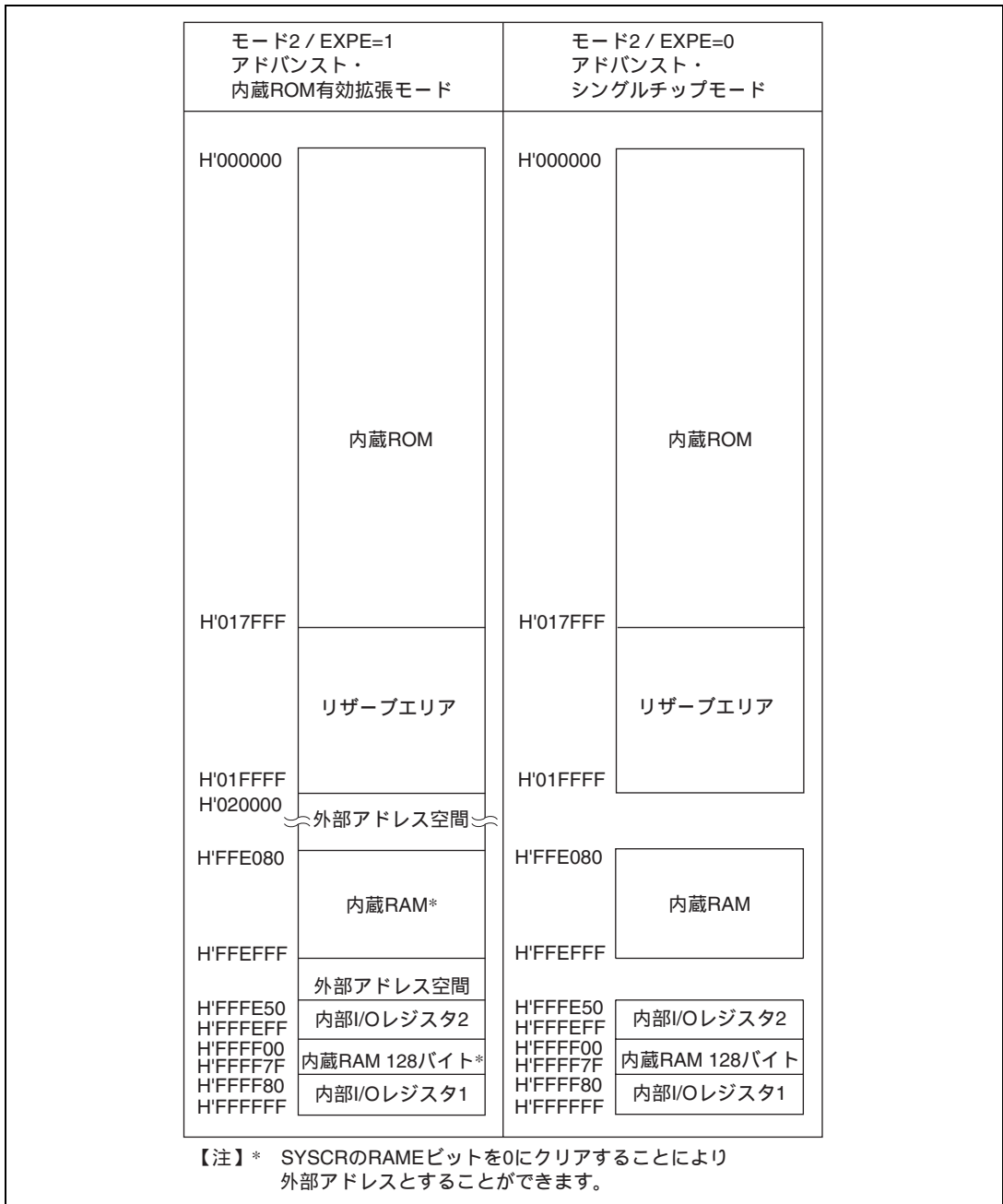
図 3.3 H8S/2143 の各動作モードのアドレスマップ (2)
