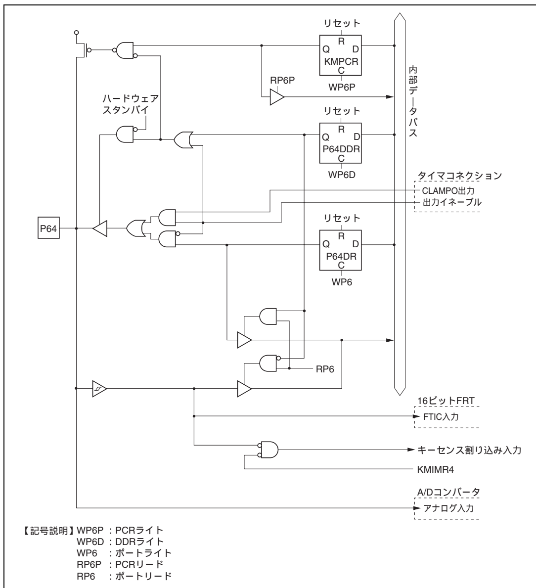
図 C.18 ポート 6 ブロック図 (P64 端子)
