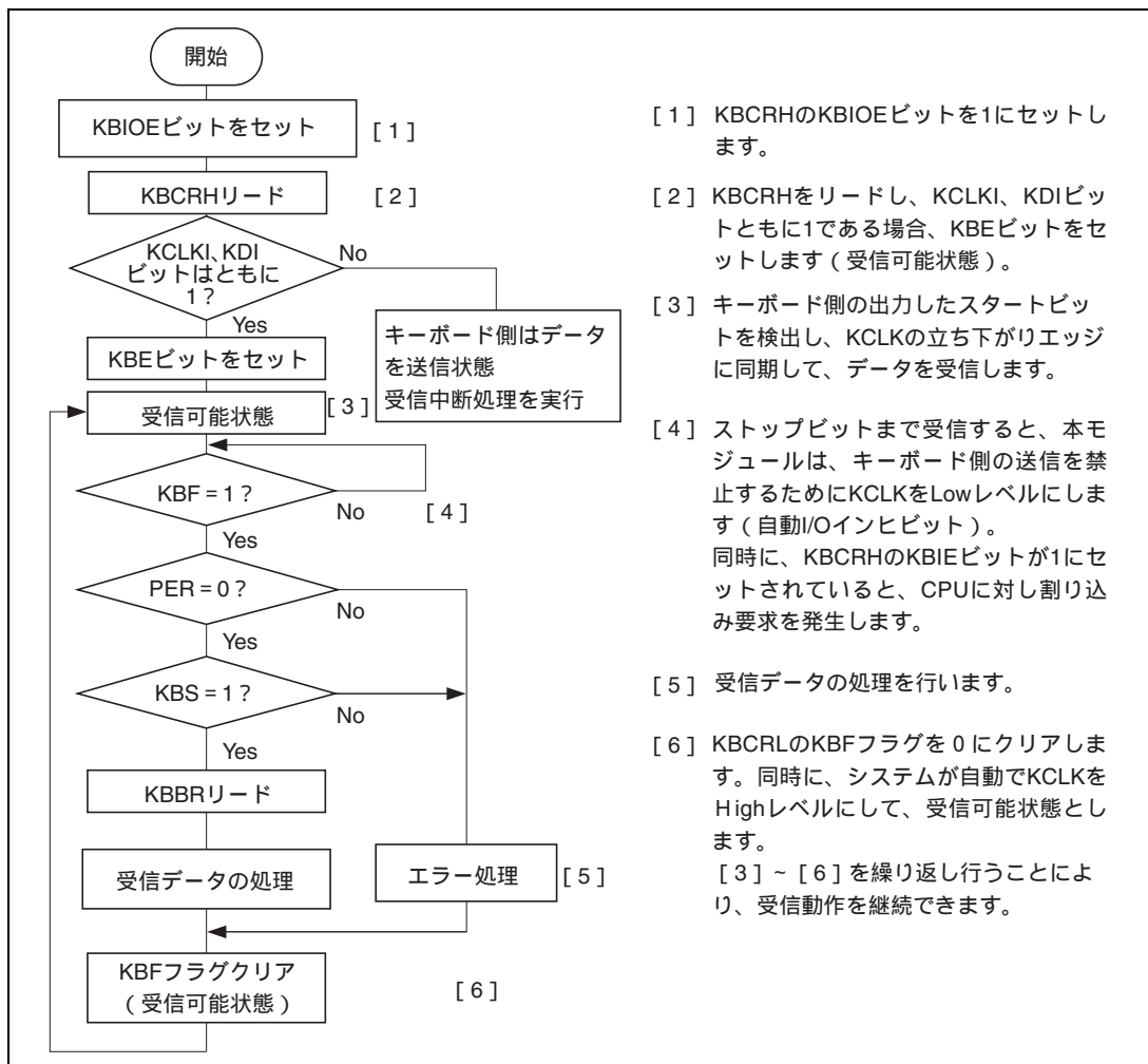
図 17.3 受信処理フローチャートの例
