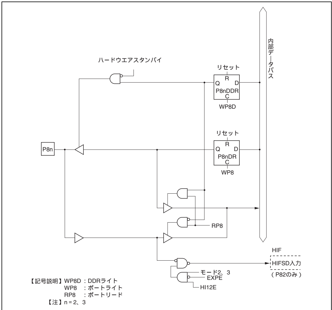
図 C.25 ポート 8 ブロック図 (P82、P83 端子)
