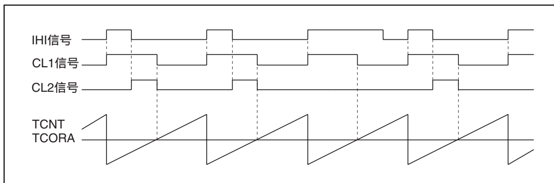
図 13.3 クランプ波形生成タイミングチャート (CL1 信号・CL2 信号)
