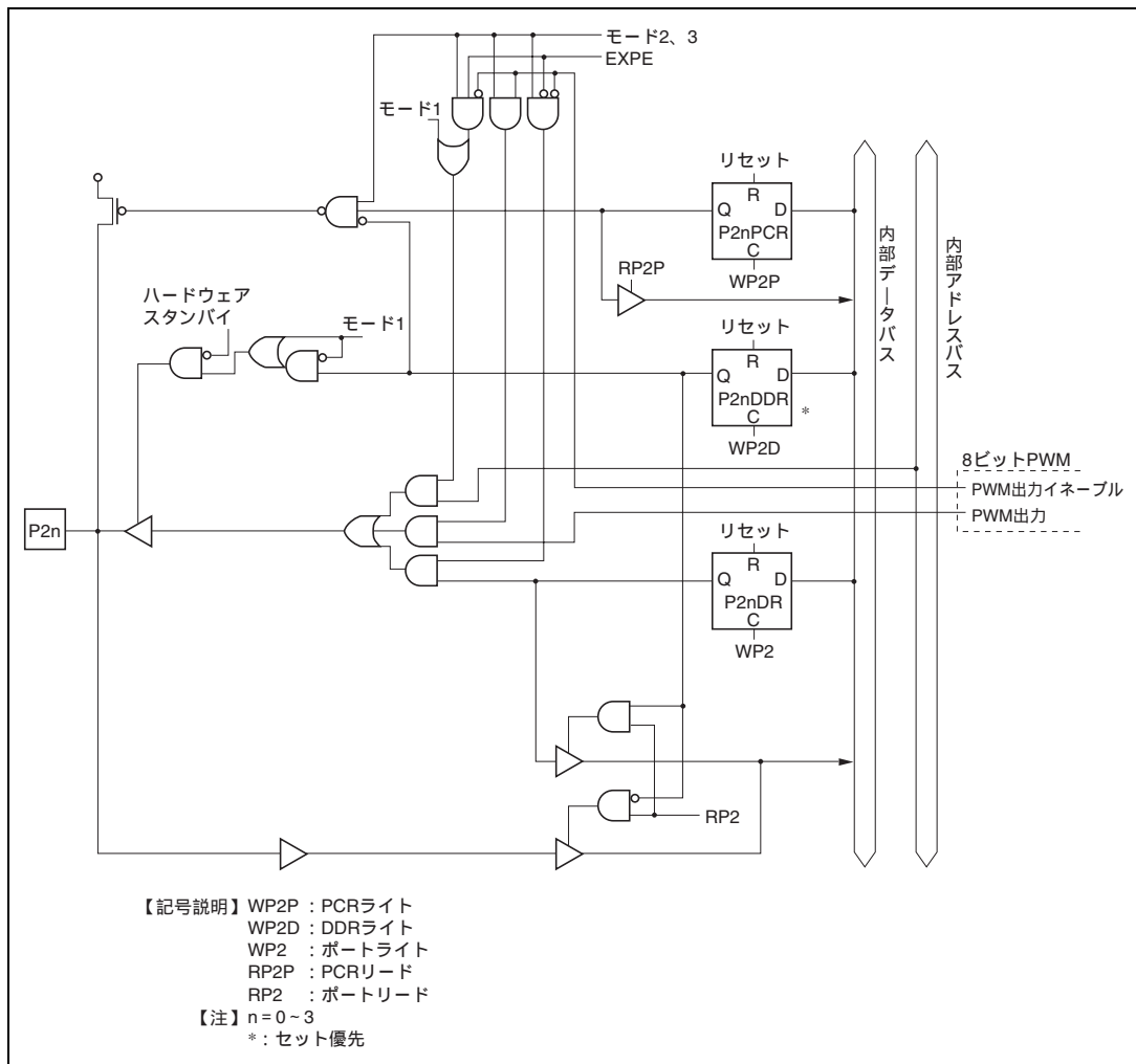
図 C.2 ポート 2 ブロック図 (P20 ~ P23 端子)
