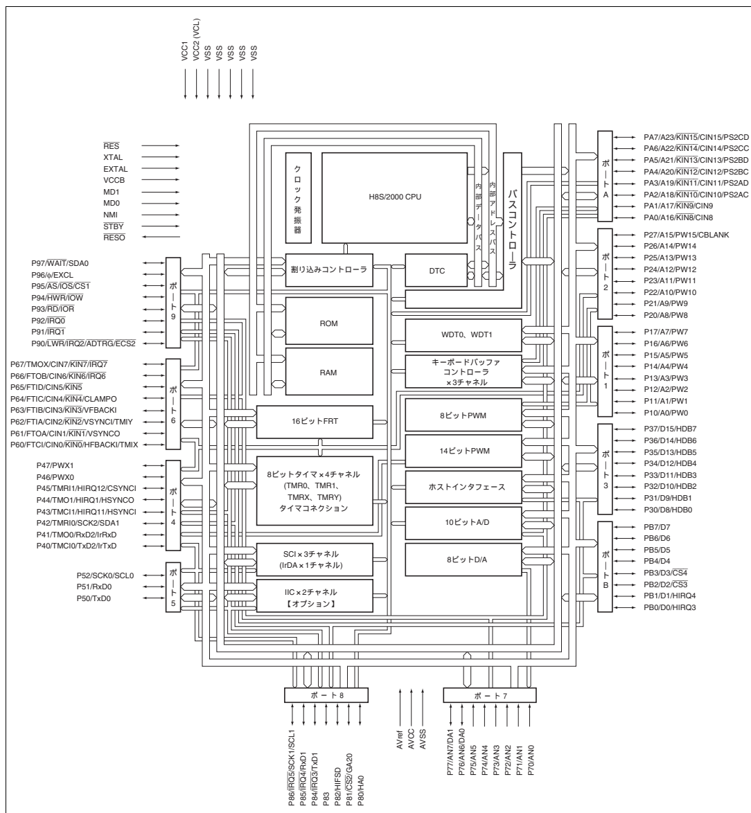
図 1.1 (a) H8S/2148 グループの内部ブロック図
