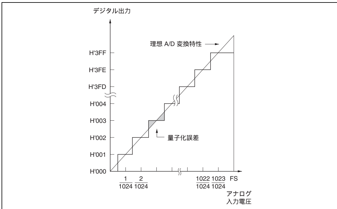
図 20.9 A/D 変換精度の定義 (1)
