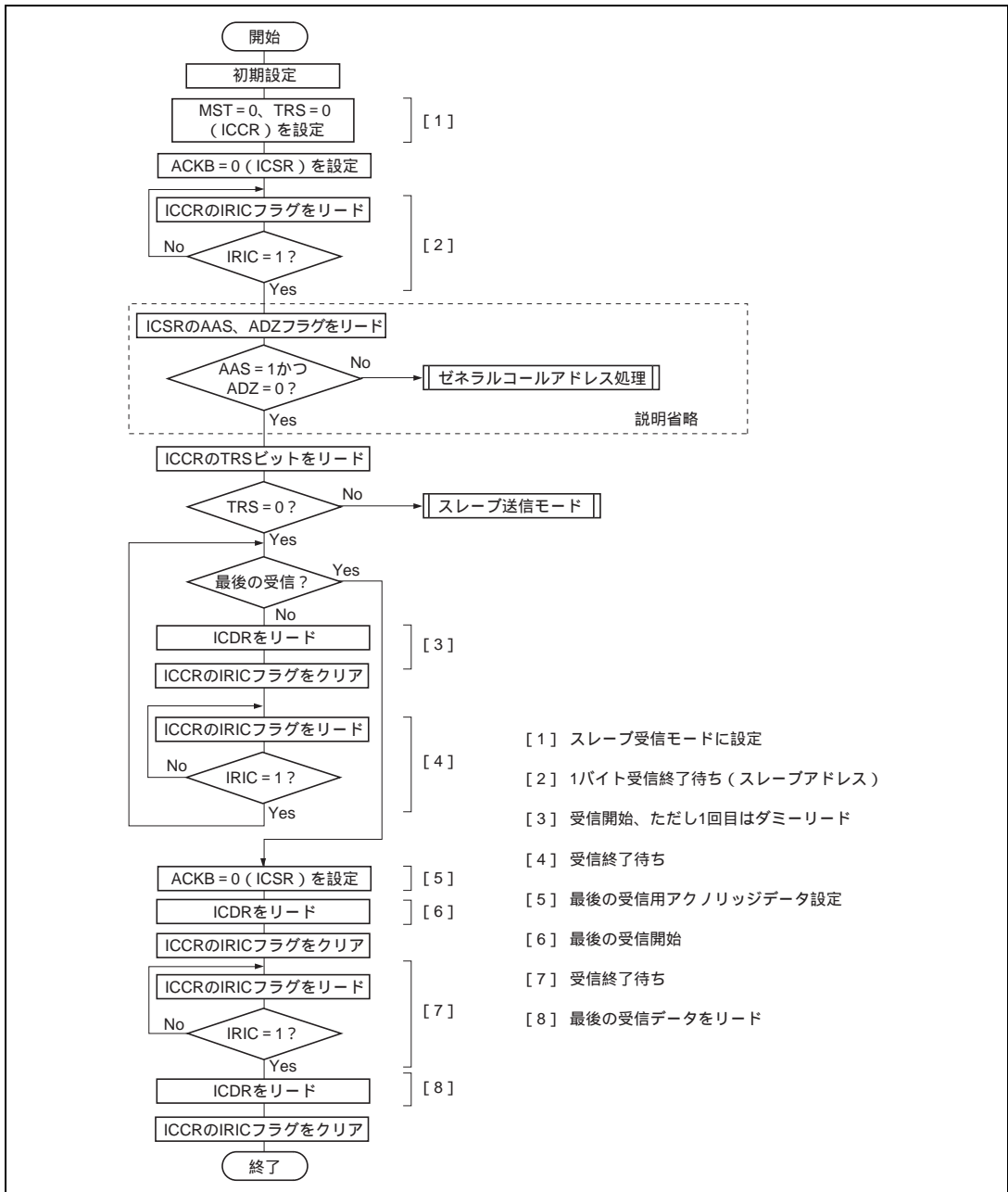
図 16.16 スレーブ受信モードフローチャート例
