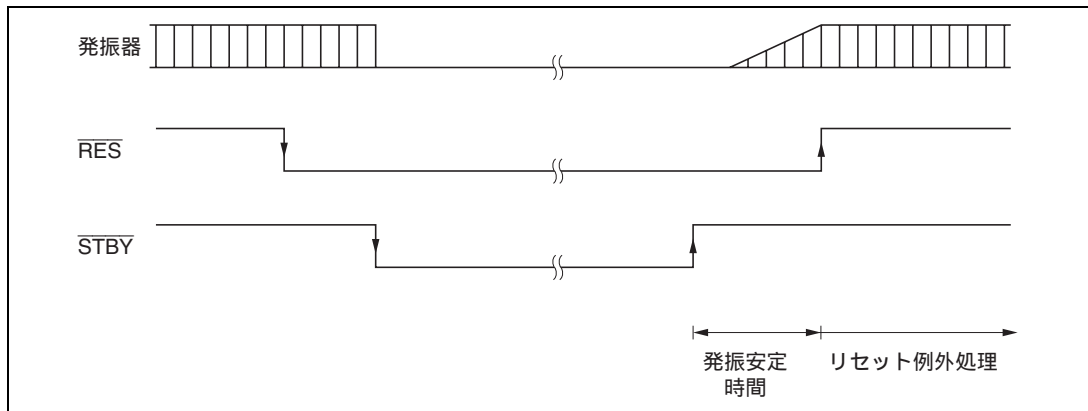
図 25.4 ハードウェアスタンバイモードのタイミング
