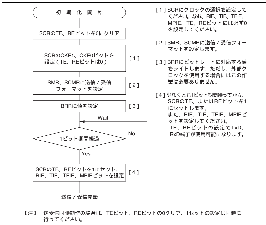
図 15.15 SCI の初期化フローチャートの例
