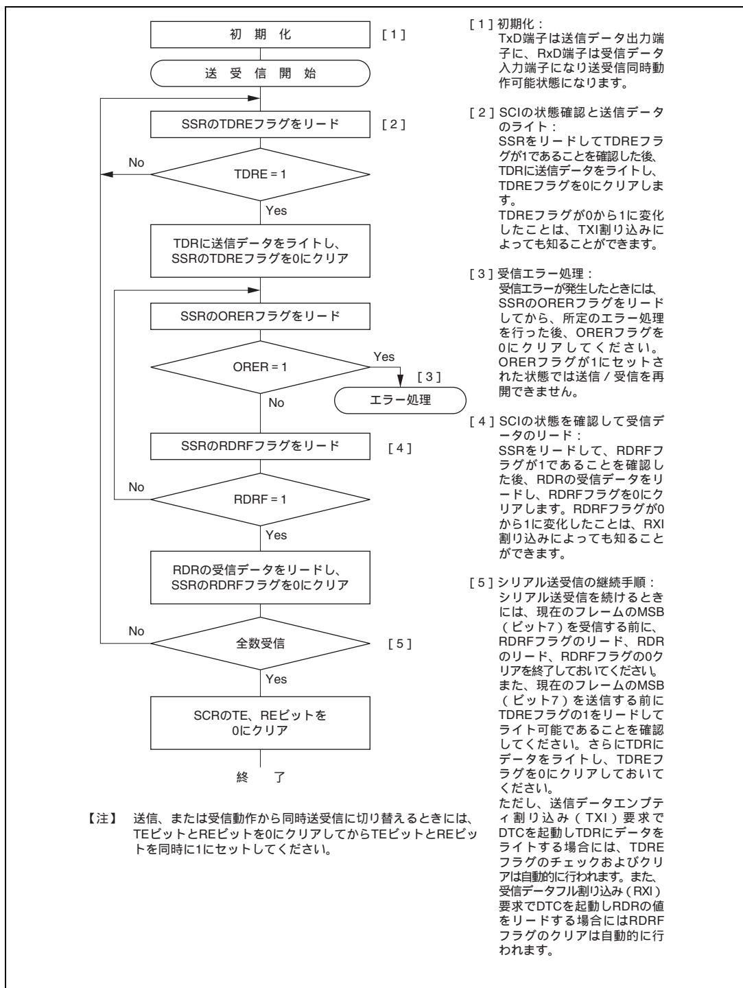
図 15.20 シリアル送受信同時動作のフローチャートの例
