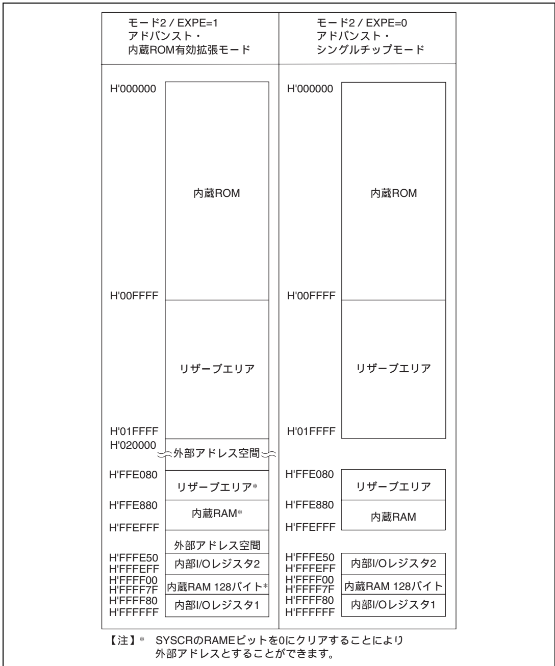
図 3.4 H8S/2147 (F-ZTAT A マスク品を除く)、H8S/2147N、H8S/2142 の各動作モードのアドレスマップ (2)
