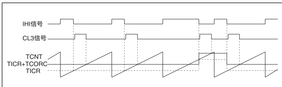
図 13.4 クランプ波形生成タイミングチャート (CL3 信号)
