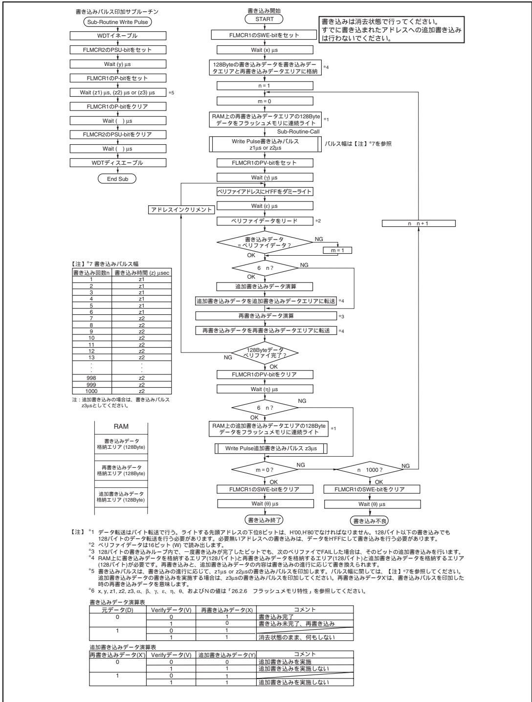
図 23.12 プログラム/プログラムベリファイフロー
