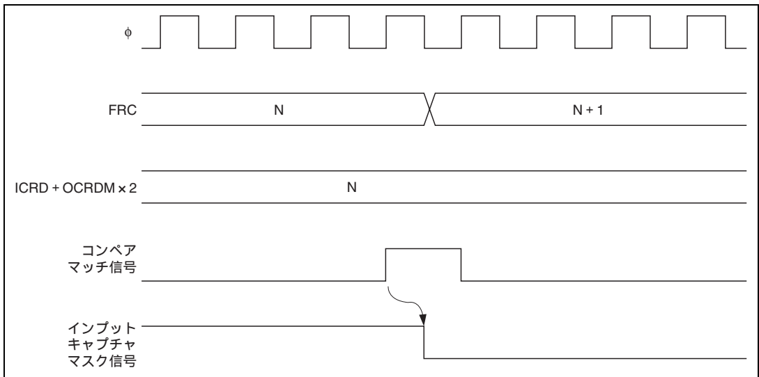
図 11.16 インพุットキャプチャマスク信号のクリアタイミング
