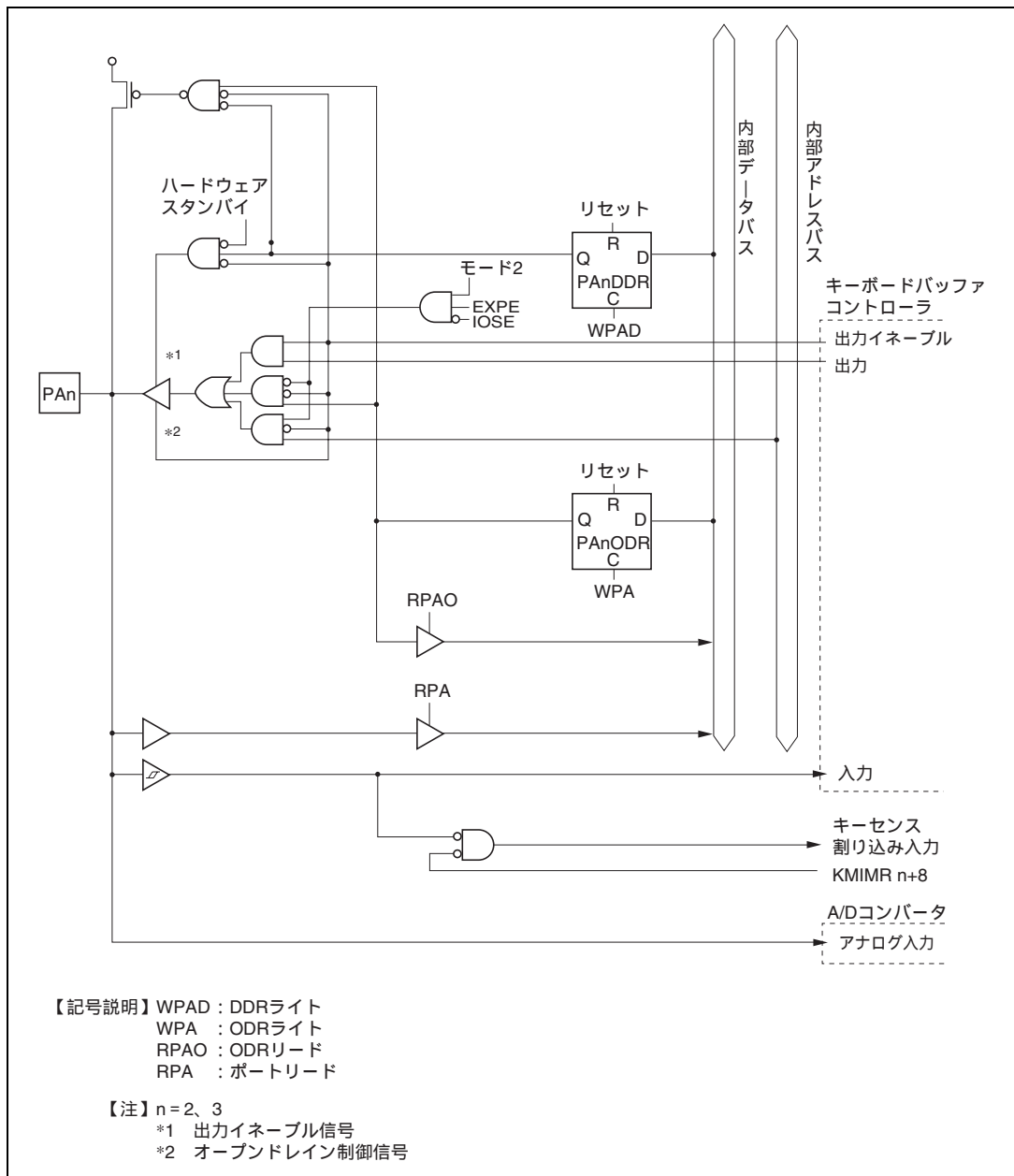
図 C.35 ポート A ブロック図 (PA2、PA3 端子)
