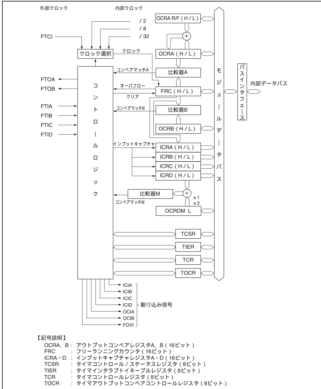
図 11.1 16ビットフリーランニングタイムのブロック図
