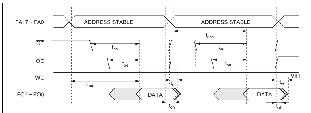
図 23.19 CE、OE クロック方式リード時のタイミング波形
