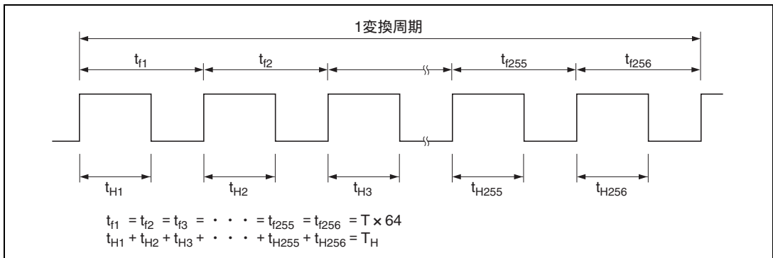
図 10.4 (3) 出力波形
