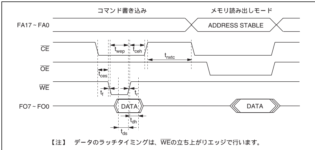
図 23.16 コマンド書き込み後メモリ読み出しタイミング波形
