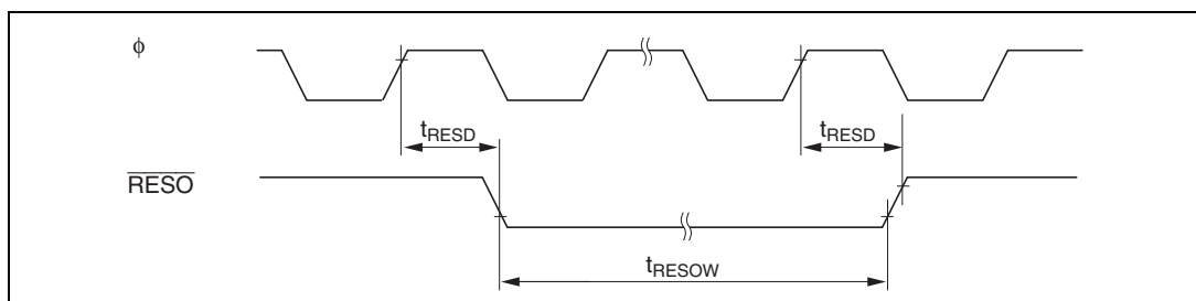
図 26.25 WDT 出力タイミング (RESO)
