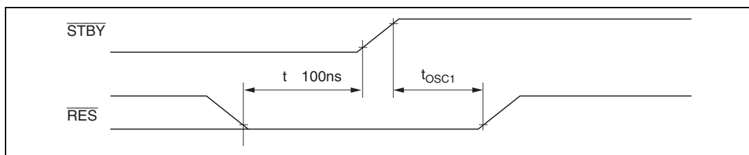
図 E.2 ハードウェアスタンバイモードからの復帰タイミング
