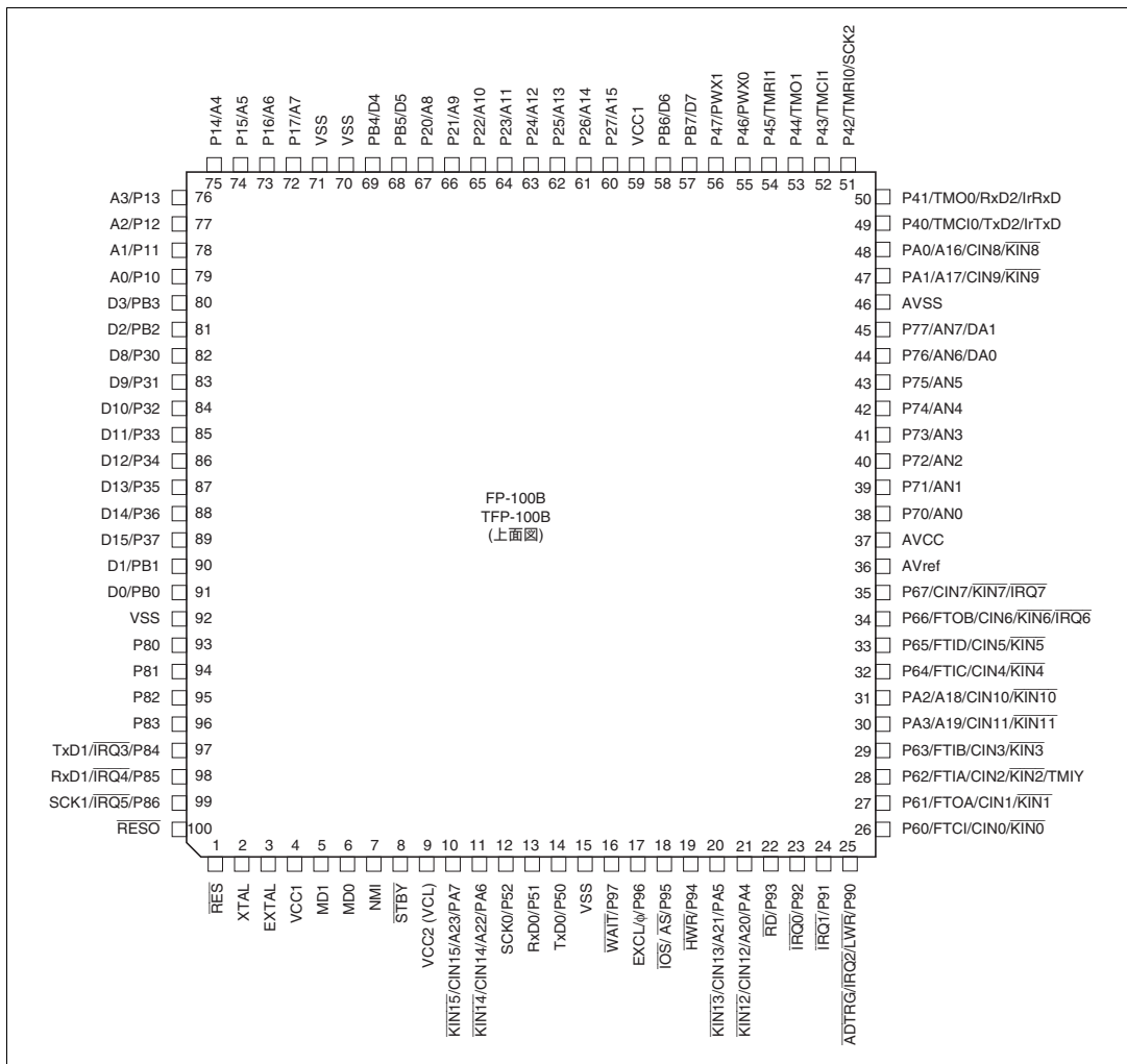
図 1.2 (c) H8S/2144 グループのピン配置図 (FP-100B、TFP-100B : 上面図)
