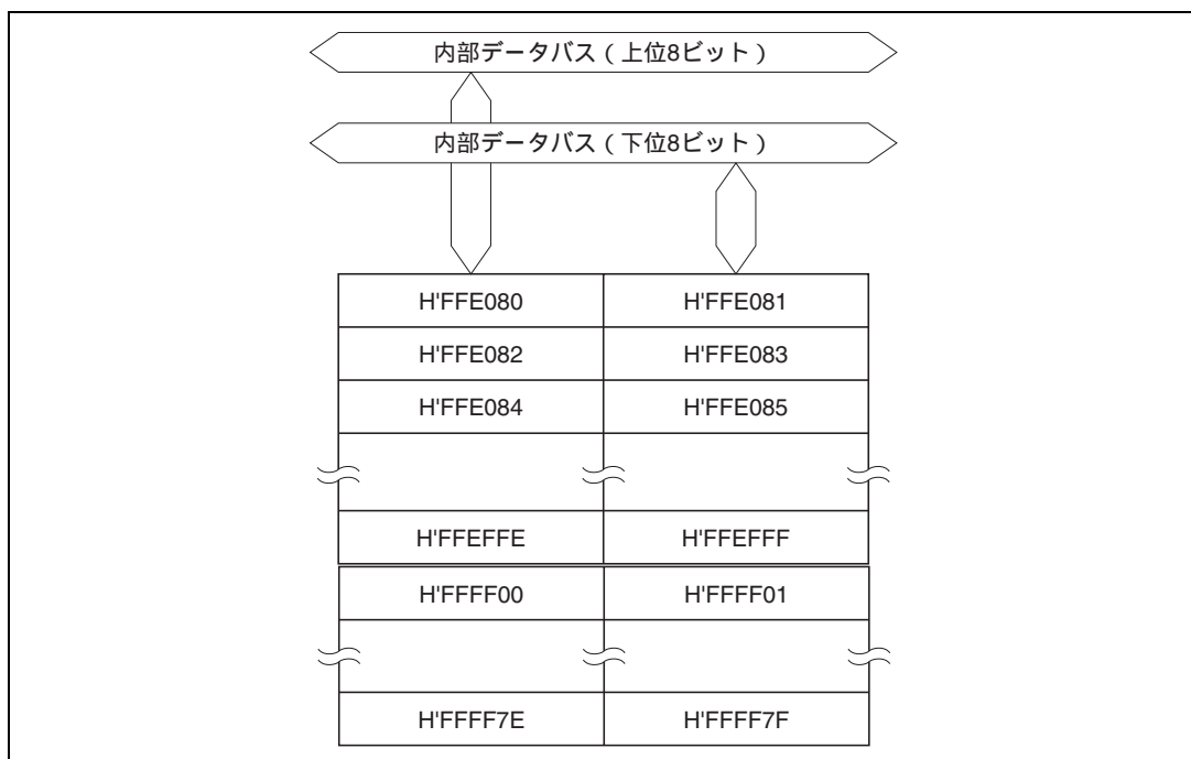
図 21.1 RAM のブロック図 (H8S/2148、H8S/2144、H8S/2143 の場合)
