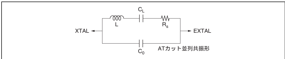
図 24.3 水晶発振子の等価回路
