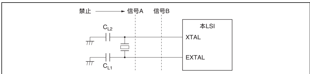
図 24.4 発振回路部のボード設計に関する注意事項
