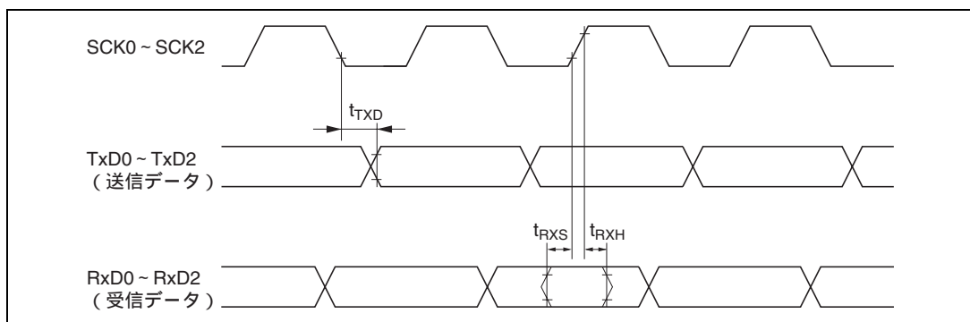
図 26.23 SCI 入出力タイミング/クロック同期式モード
