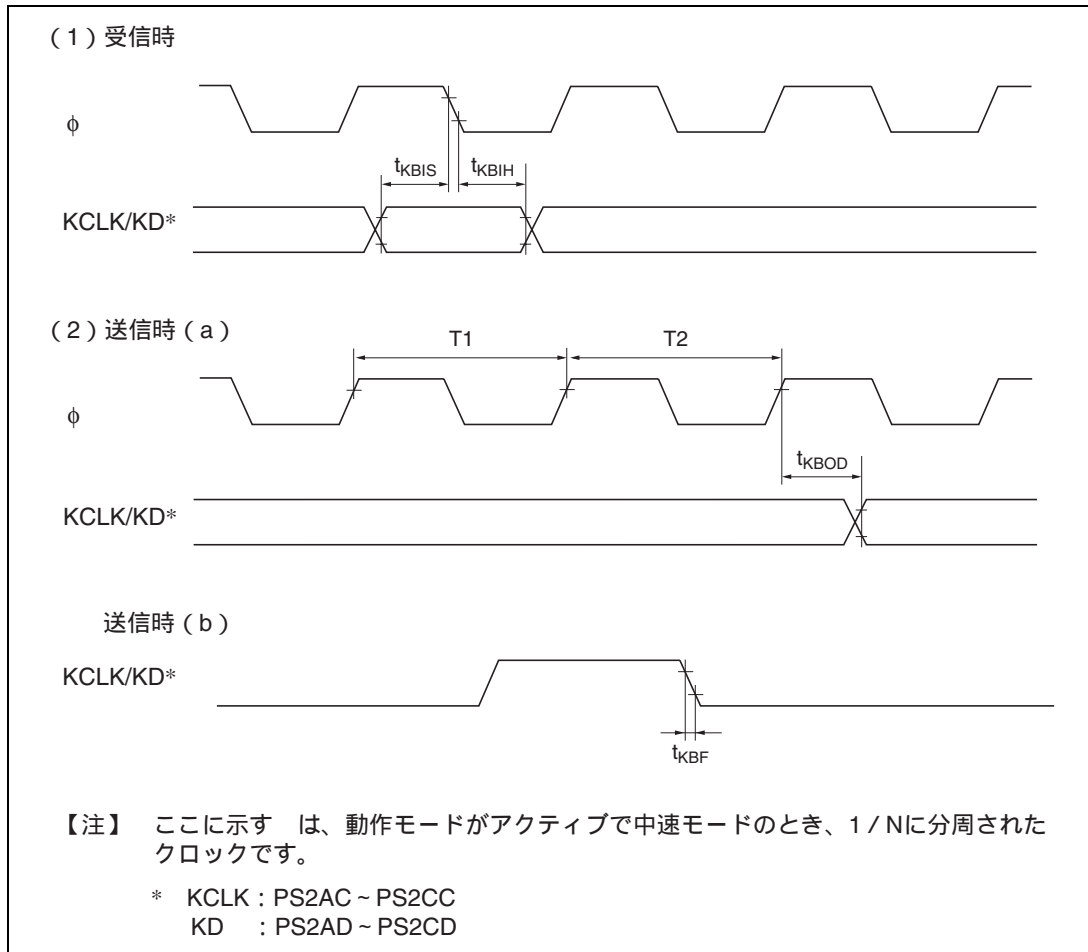
図 26.27 キーボードバッファコントローラタイミング
