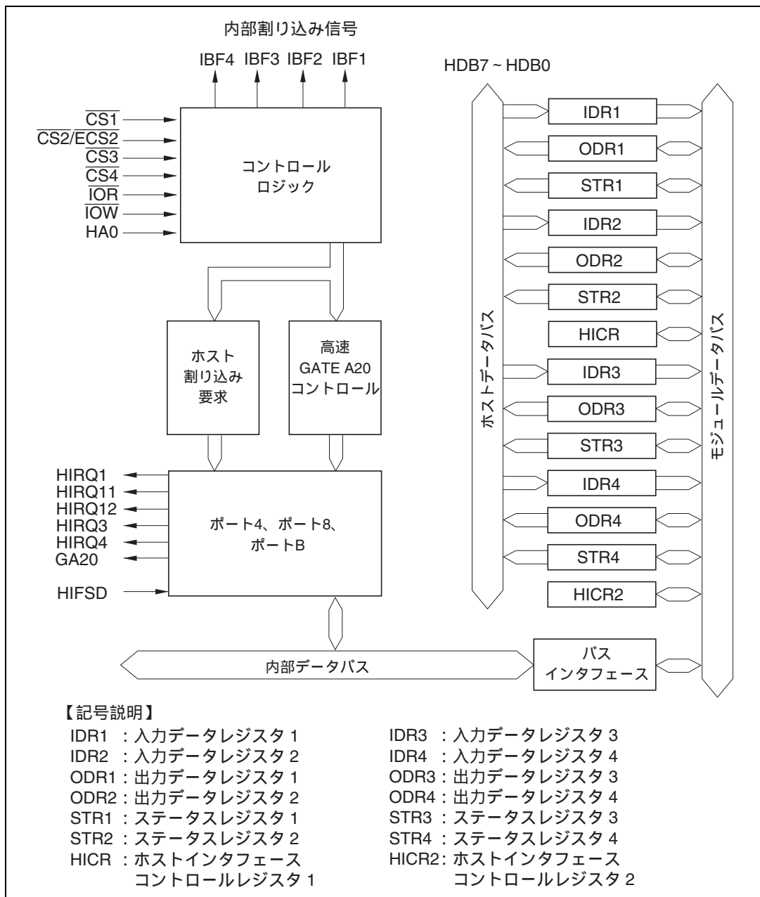
図 18.1 HIF のブロック図
