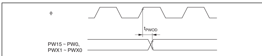
図 26.21 PWM、PWMX 出力タイミング
