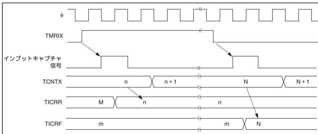
図 12.9 インプットキャプチャ動作タイミング
