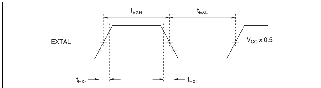
図 24.6 外部クロック入力タイミング
