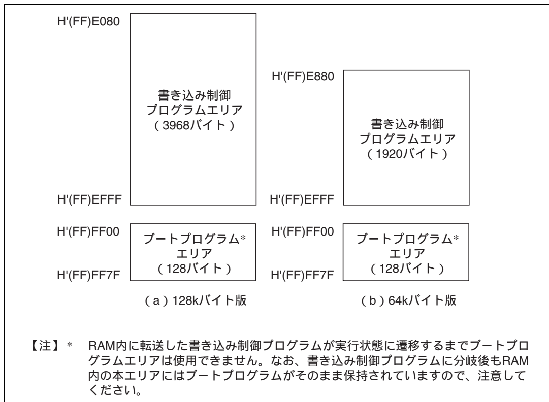
図 22.10 ブートモード時の RAM エリア
