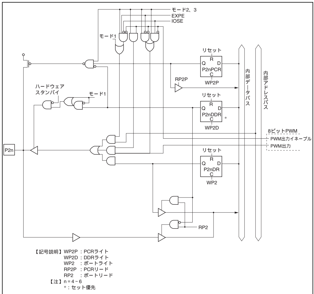
図 C.3 ポート 2 ブロック図 (P24~P26 端子)
