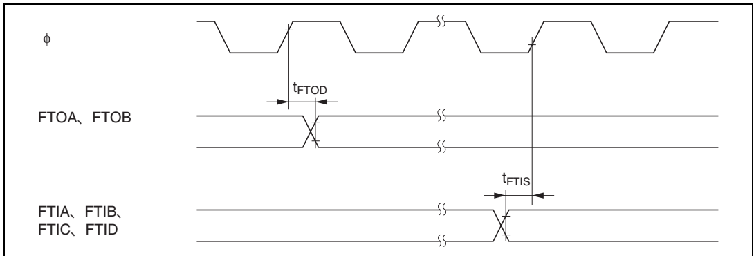
図 26.16 FRT 入出力タイミング
