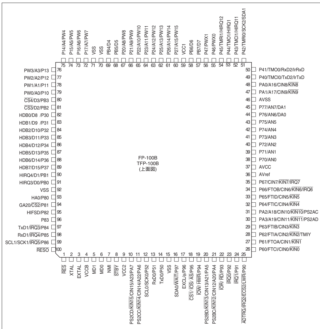
図 1.2 (b) H8S/2147N のピン配置図 (FP-100B、TFP-100B : 上面図)
