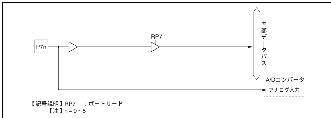
図 C.21 ポート7ブロック図 (P70~P75 端子)
