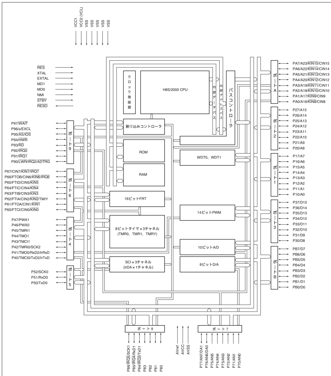
図 1.1 (c) H8S/2144 グループの内部ブロック図
