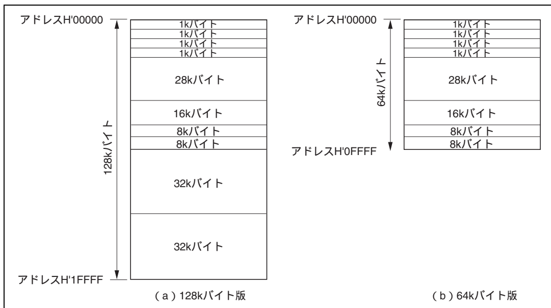
図 23.6 フラッシュメモリのブロック分割
