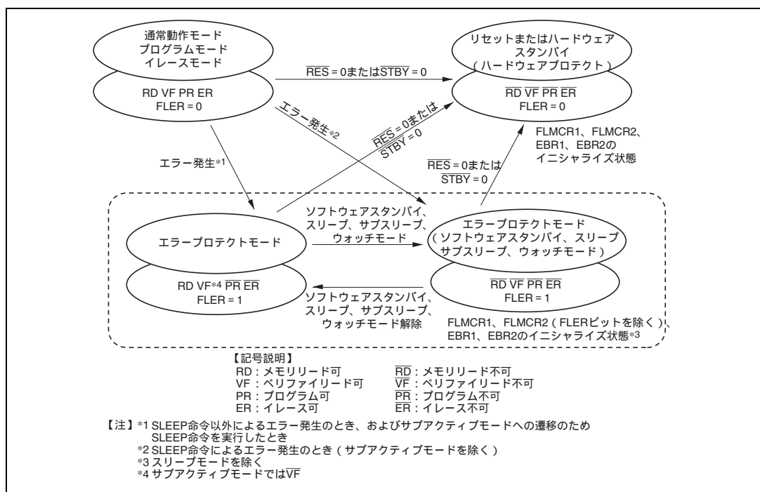
図 22.14 フラッシュメモリの状態遷移図
