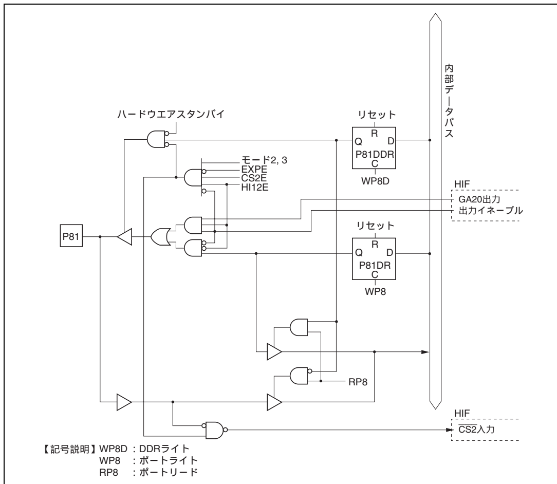
図 C.24 ポート 8 ブロック図 (P81 端子)
