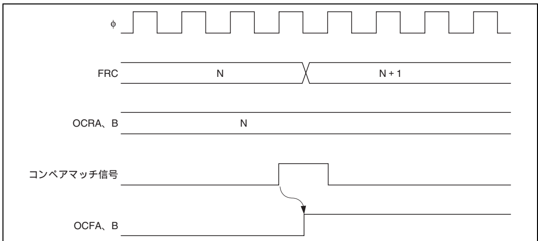
図 11.12 OCF セットタイミング
