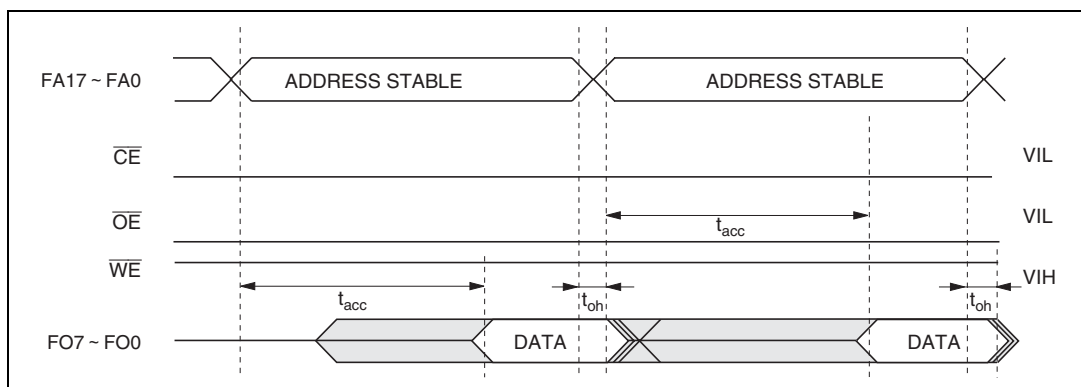
図 22.18 \overline{CE} 、 \overline{OE} イネーブル状態リード時のタイミング波形
