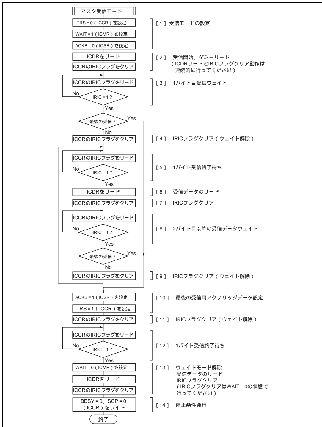
図 16.15 マスタ受信モードのフローチャート例
