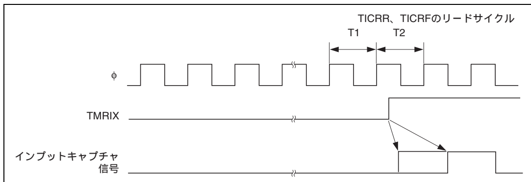
図 12.10 インプットキャプチャ信号タイミング (TICRR、TICRF のリード時に、インプットキャプチャ入力を入力した場合)
