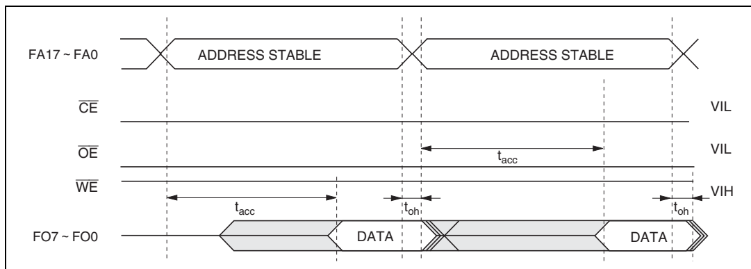
図 23.18 CE、OE イネーブル状態リード時のタイミング波形
