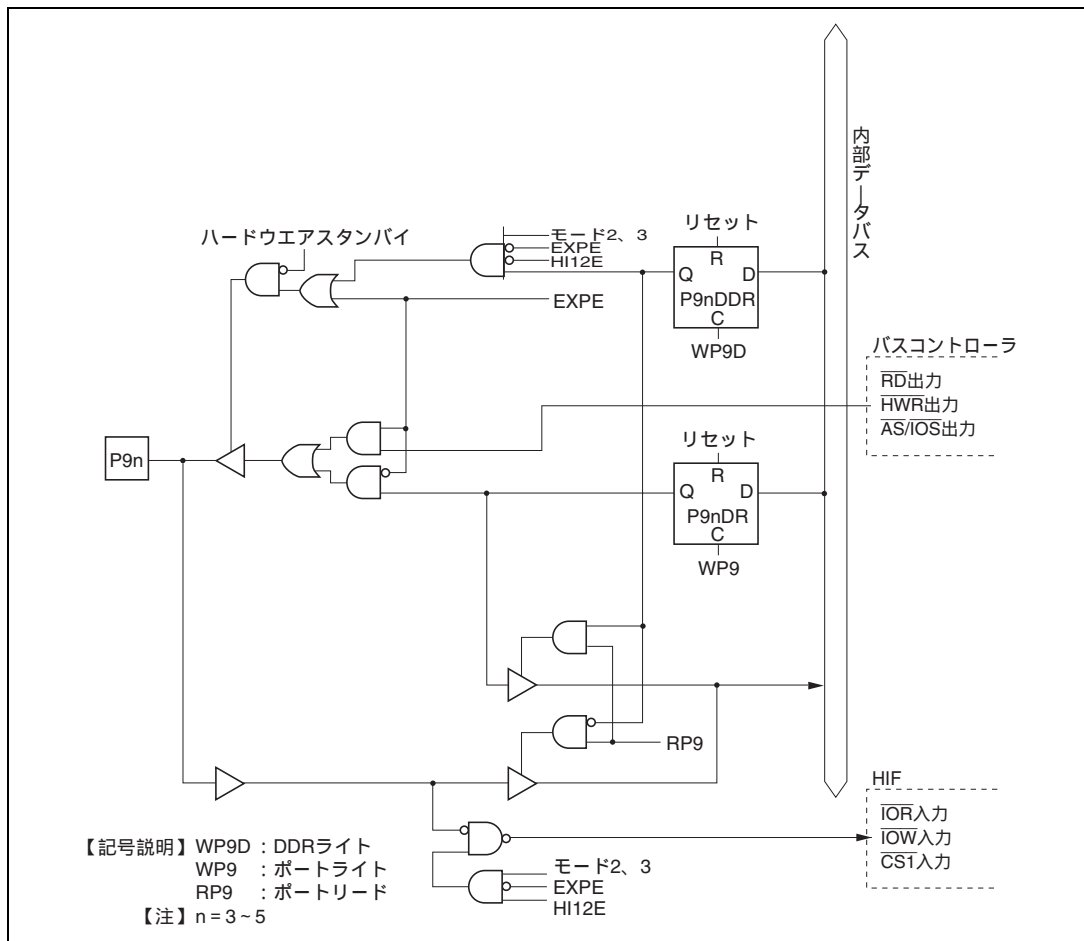
図 C.31 ポート 9 ブロック図 ( P93 ~ P95 端子 )
