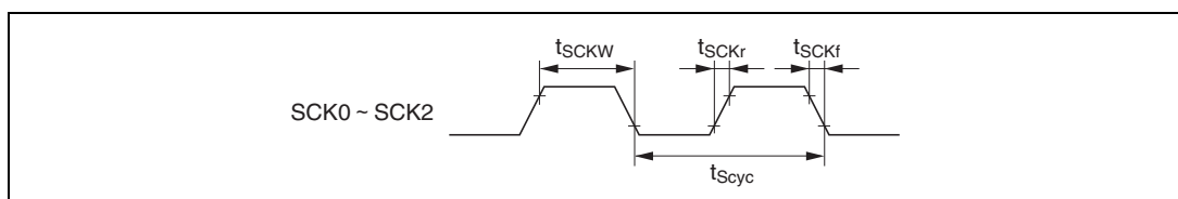
図 26.22 SCK クロック入力タイミング
