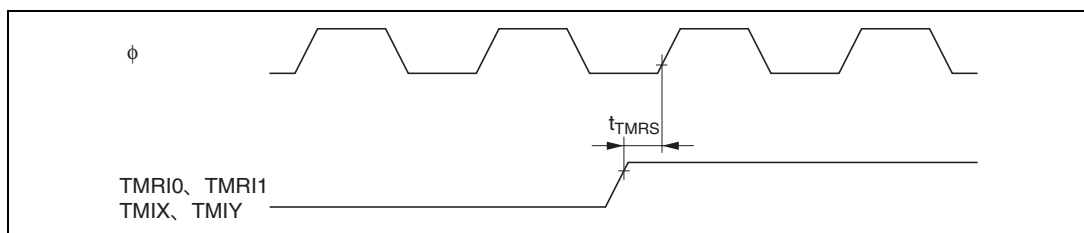
図 26.20 8ビットタイマリセット入力タイミング
