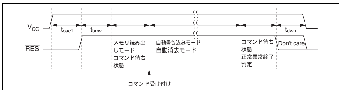
図 23.23 発振安定時間、ライタモードセットアップ、および電源立ち下げシーケンス
