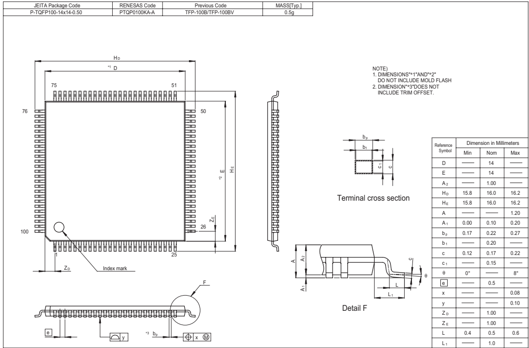
図 H.2 TFP-100B の外形寸法図
