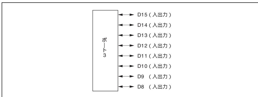
図 8.10 ポート 3 の端子機能 (モード 1~3 (EXPE=1))
