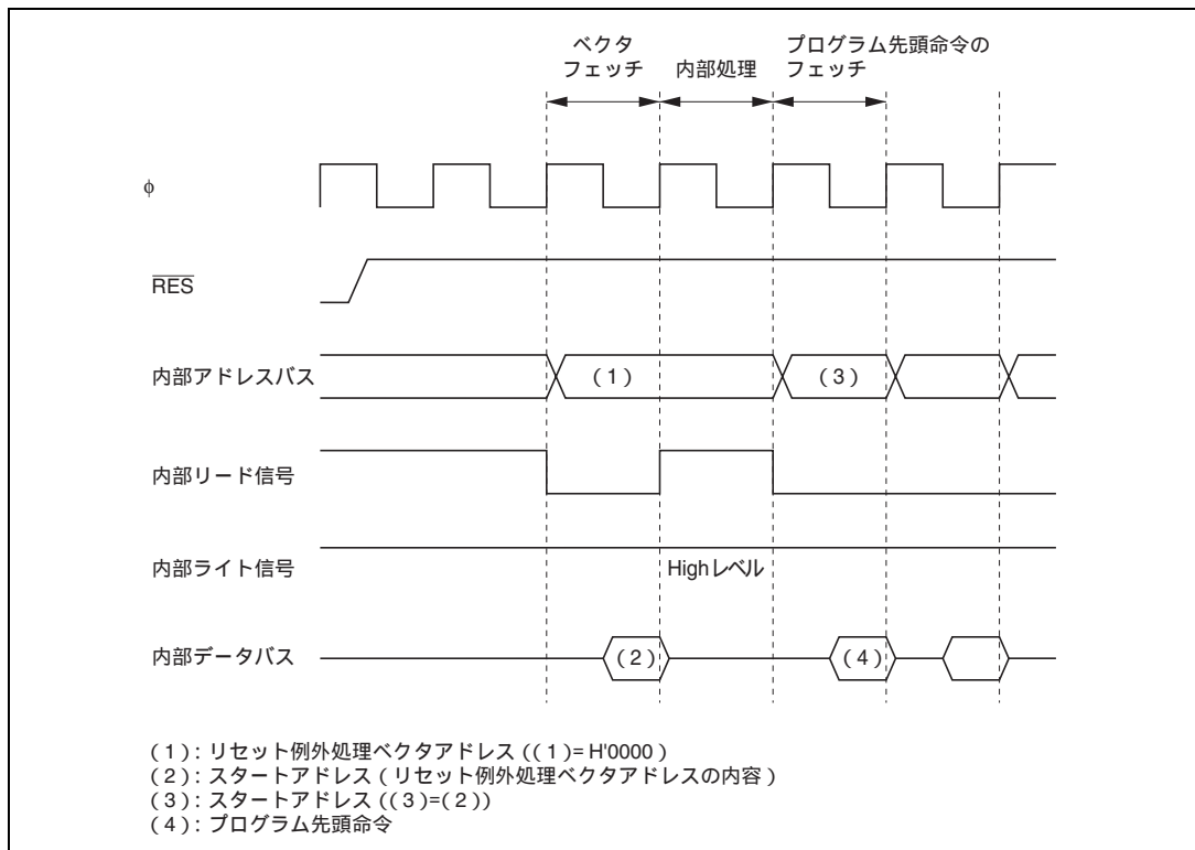
図 4.2 リセットシーケンス (モード 3)
