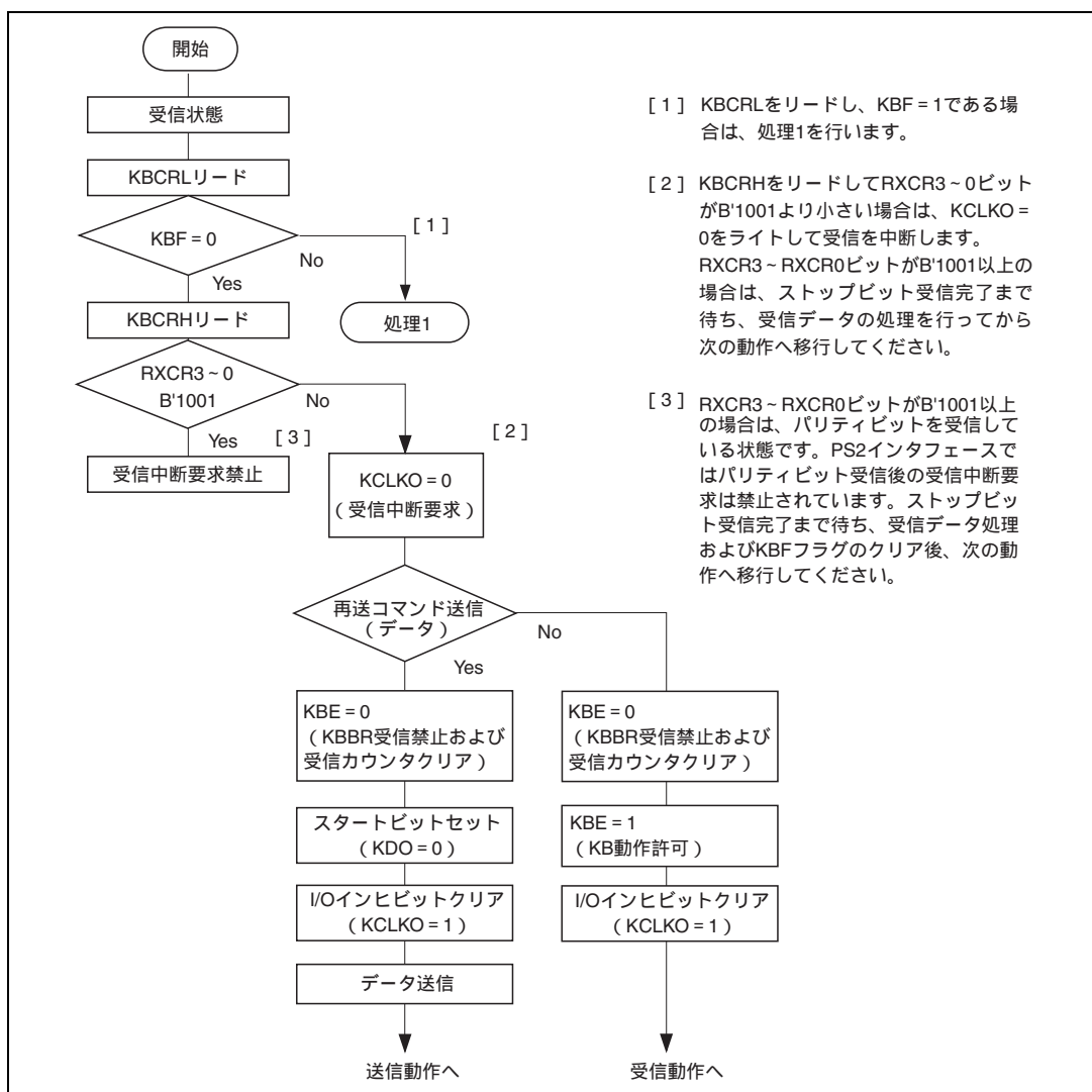
図 17.7 ( 1 ) 受信中断処理フローチャートの例
