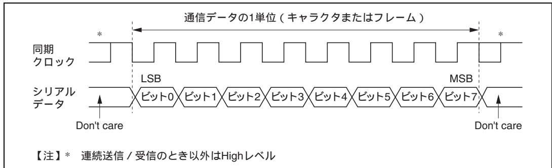
図 15.14 クロック同期式通信のデータフォーマット
