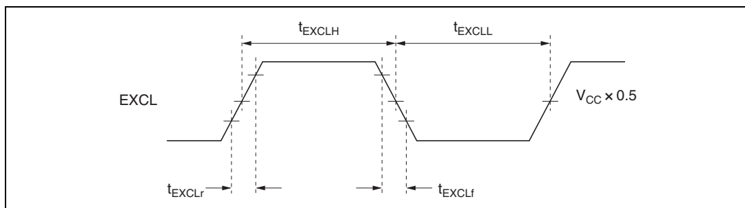
図 24.8 サブクロック入力タイミング
