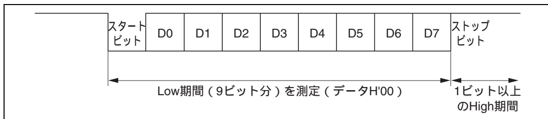
図 23.9 SCI ビットレート自動合わせ込み時の Rx/D1 入力信号
