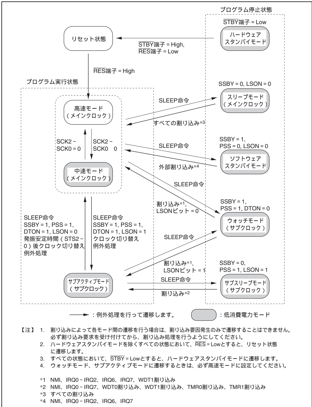
図 25.1 モード遷移図
