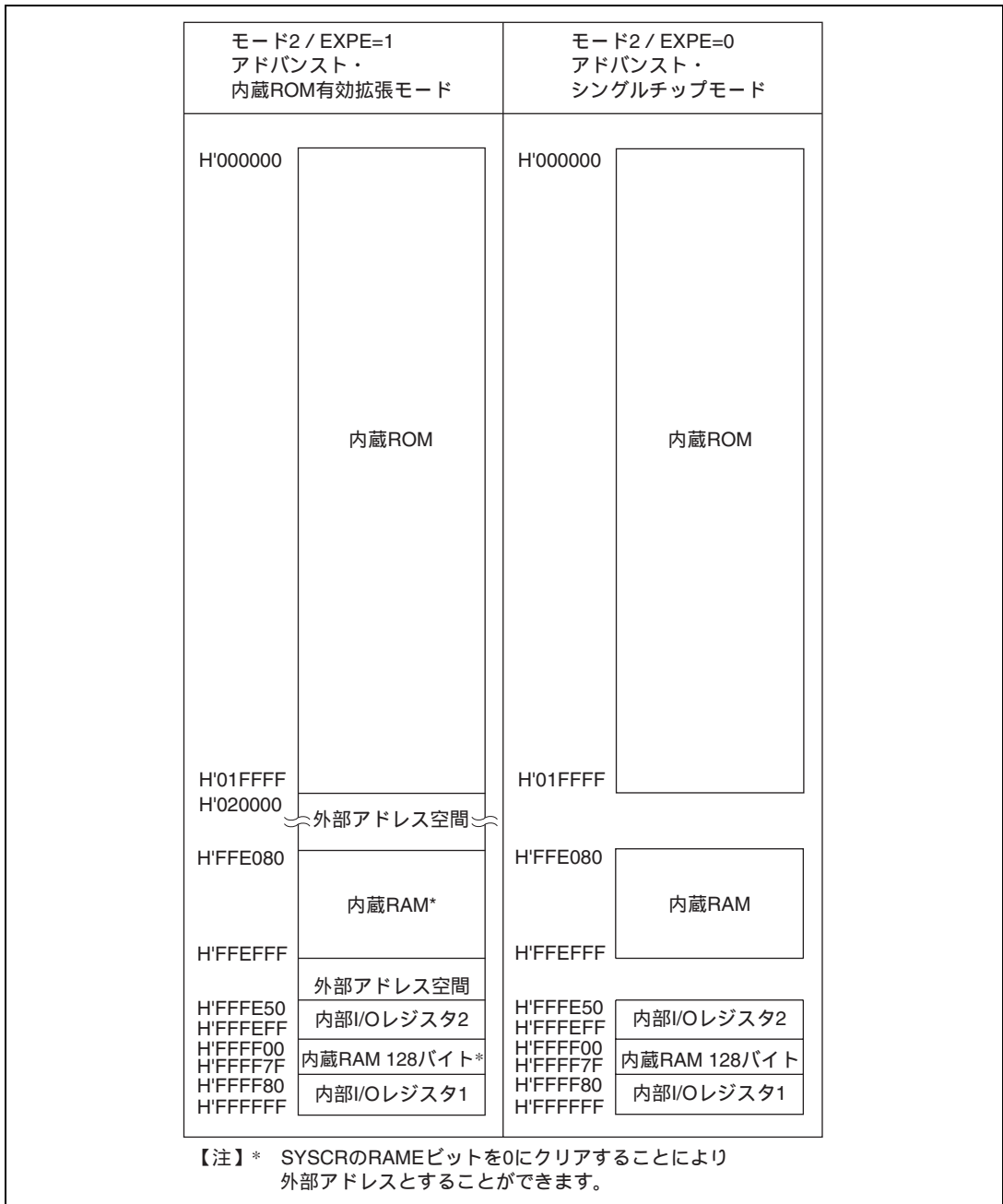
図 3.1 H8S/2148 (F-ZTAT A マスク品を除く)、H8S/2144 の各動作モードのアドレスマップ (2)
