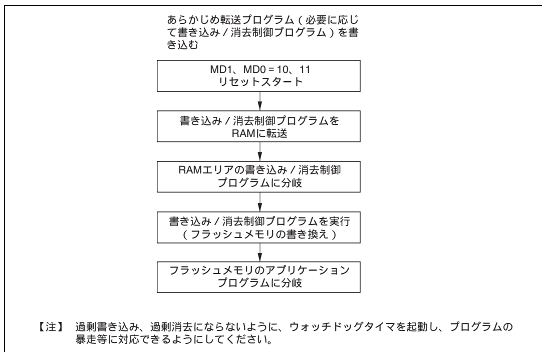
図 23.11 ユーザプログラムモードの実行手順例
