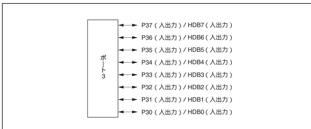
図 8.11 ポート 3 の端子機能 (モード 2、3 (EXPE=0))
