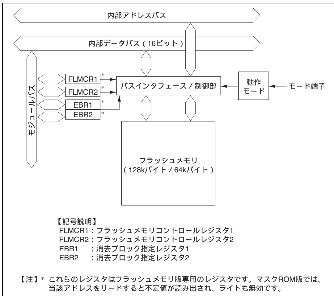
図 22.2 フラッシュメモリのブロック図
