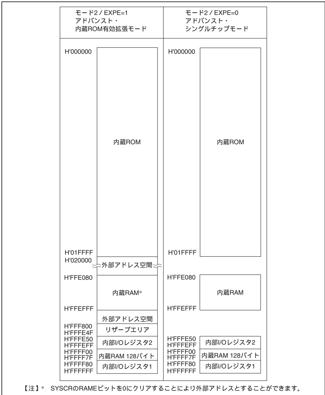
図 3.2 H8S/2148 F-ZTAT A マスク品の各動作モードのアドレスマップ (2)
