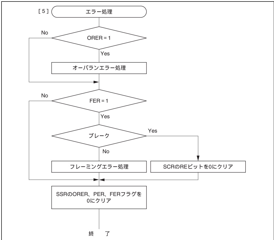
図 15.12 マルチプロセッサシリアル受信のフローチャートの例 (2)
