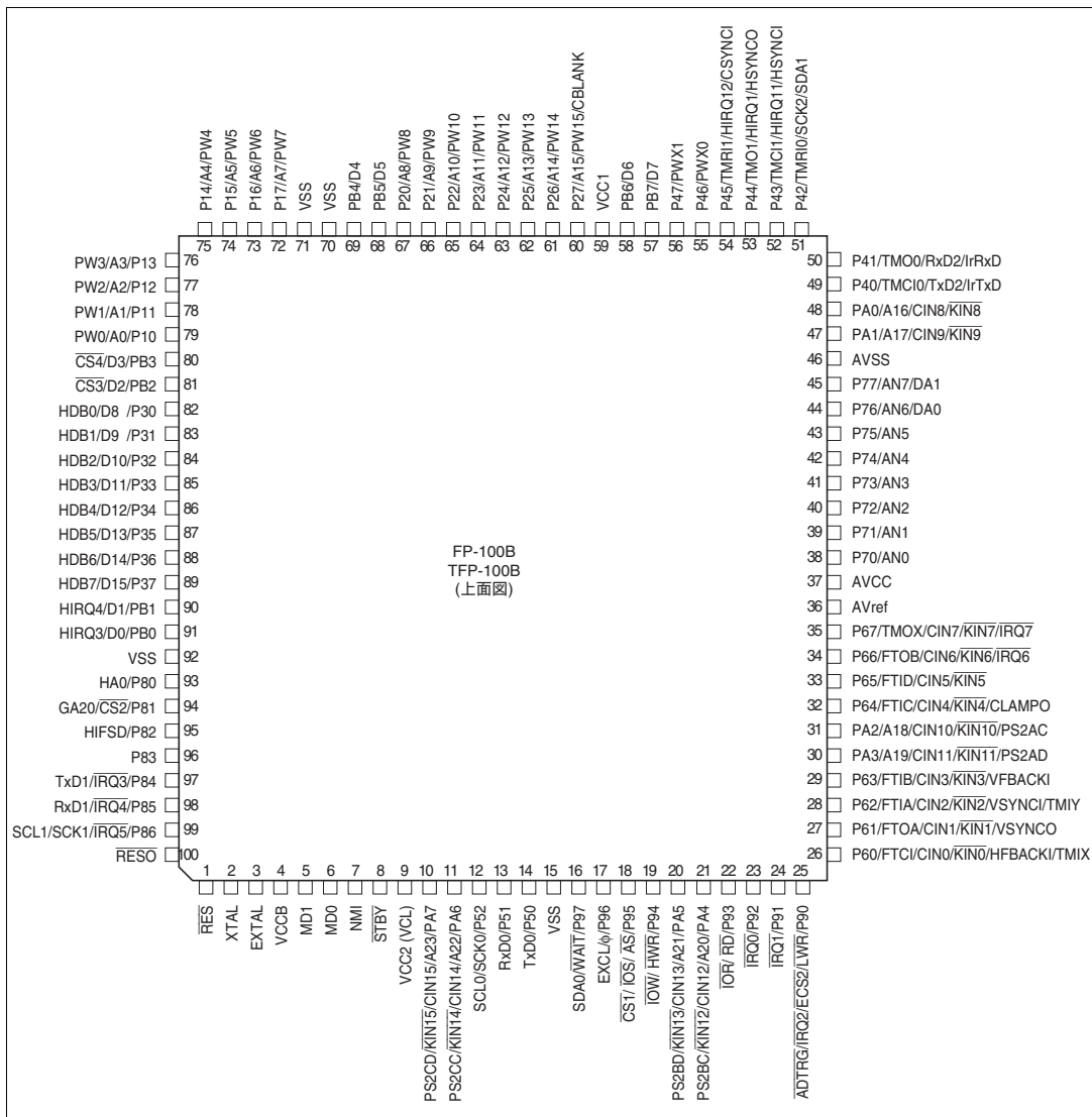
図 1.2 (a) H8S/2148 グループのピン配置図 (FP-100B、TFP-100B : 上面図)
