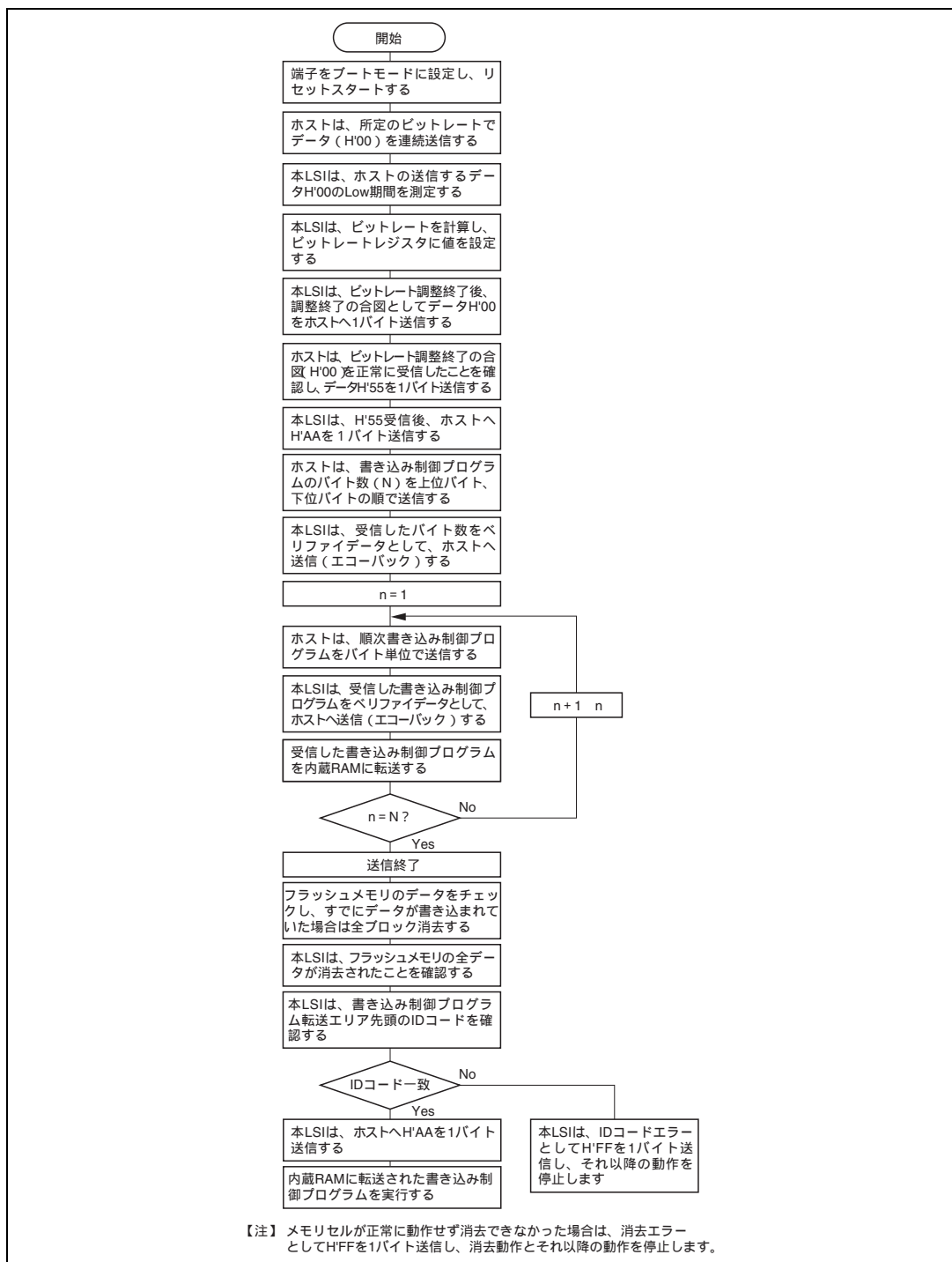
図 23.8 ブートモード実行手順
