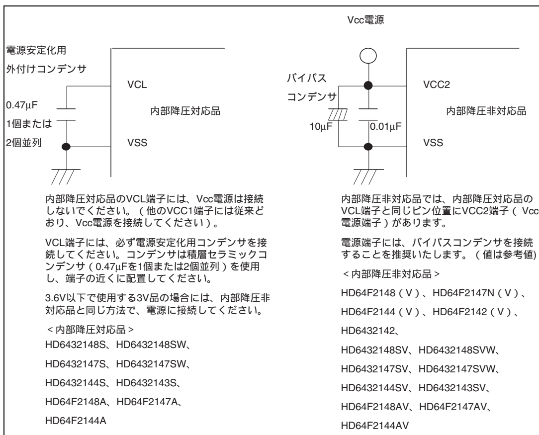
図 26.3 内部降圧対応マスクROM品のVCLコンデンサ接続方法と内部降圧非対応品との違い
