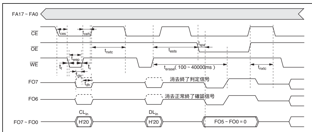
図 22.21 自動消去モードのタイミング波形
