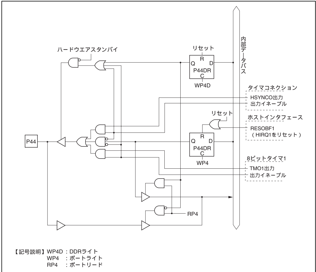
図 C.10 ポート 4 ブロック図 (P44 端子)
