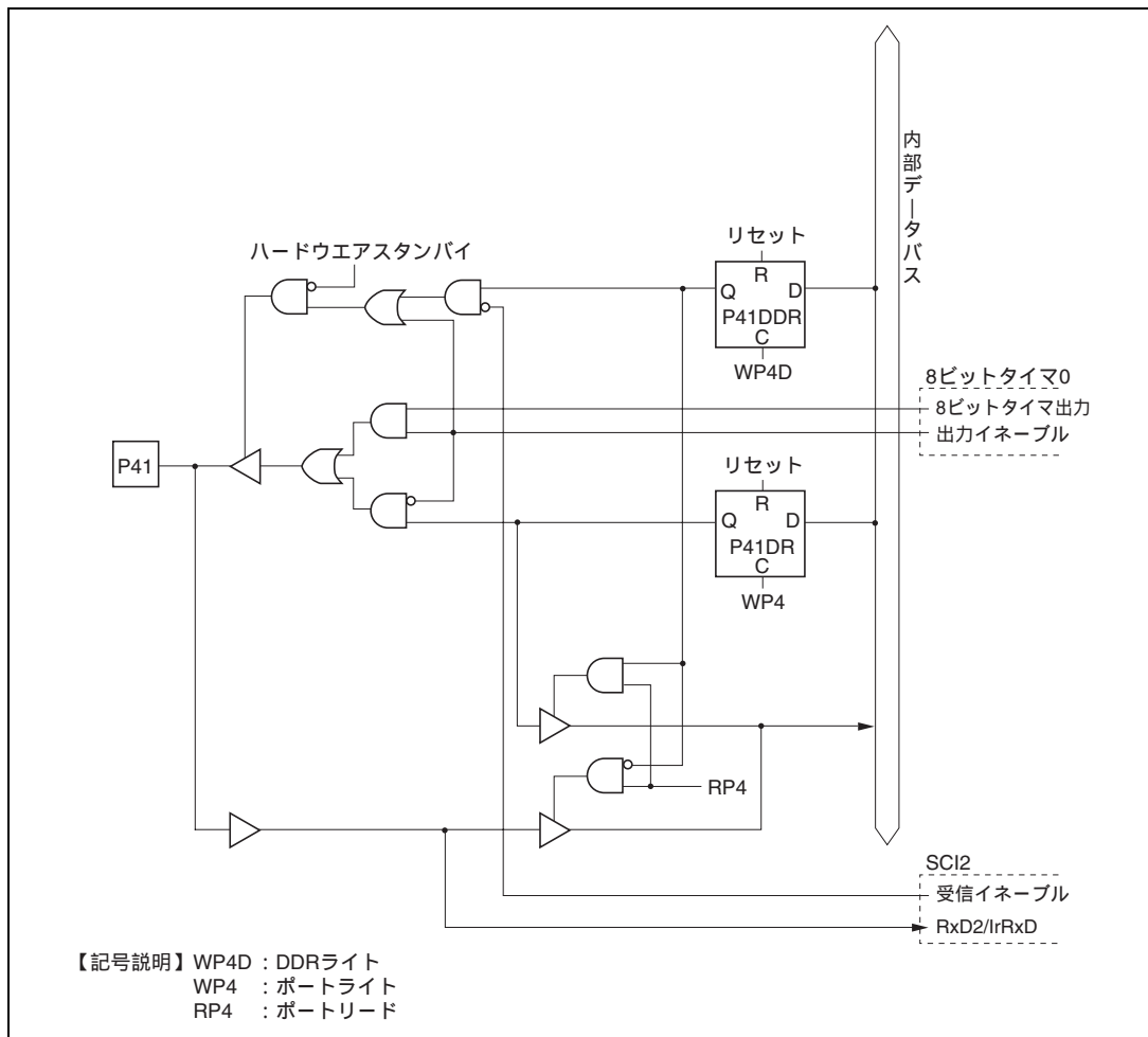
図 C.7 ポート 4 ブロック図 ( P41 端子 )
