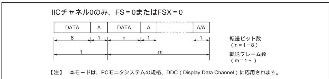
図 16.4 フォーマットレス
