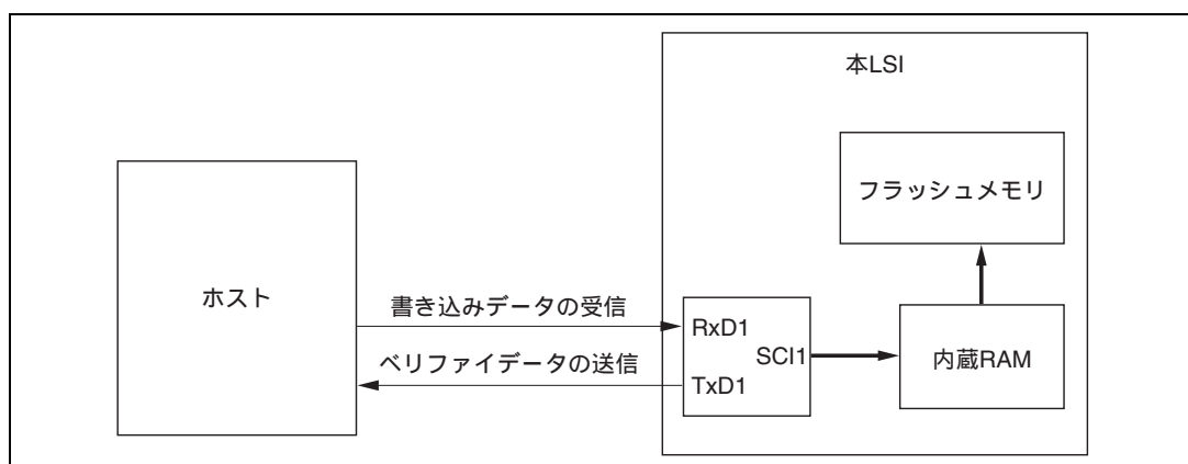
図 22.7 ブートモード時のシステム構成図
