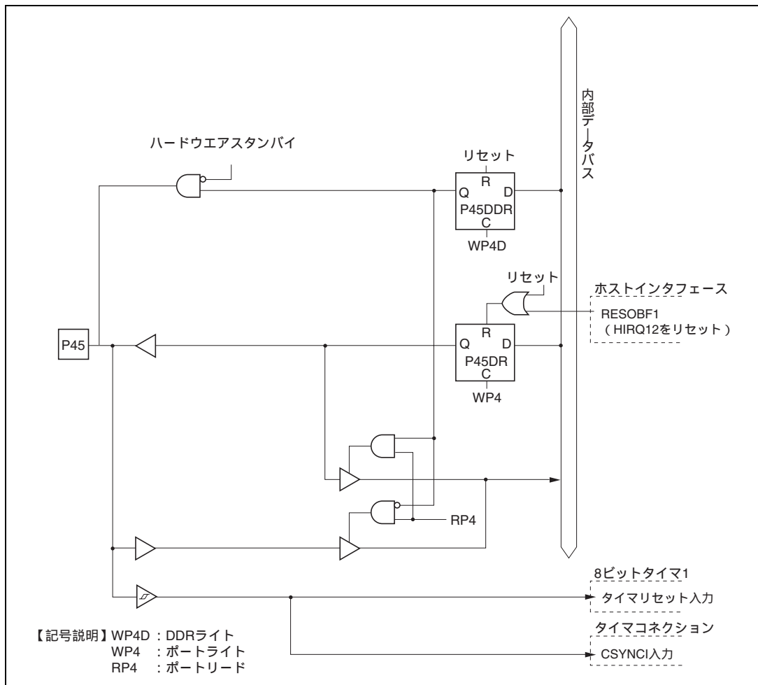
図 C.11 ポート 4 ブロック図 (P45 端子)
