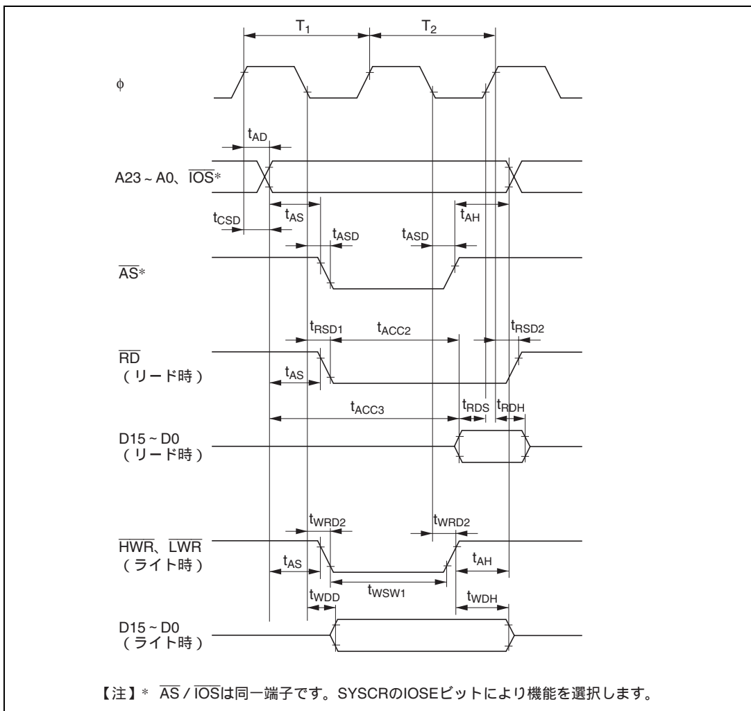
図 26.10 基本バスタイミング / 2 ステートアクセス
