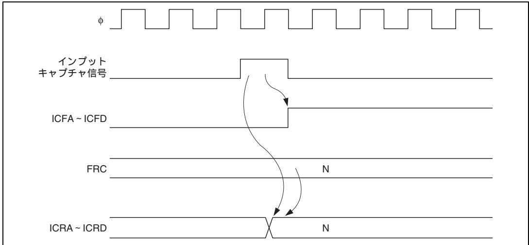
図 11.11 ICFA~D のセットタイミング
