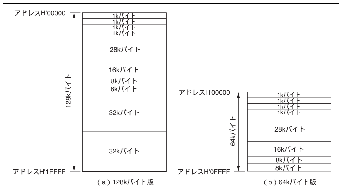
図 22.6 フラッシュメモリのブロック分割
