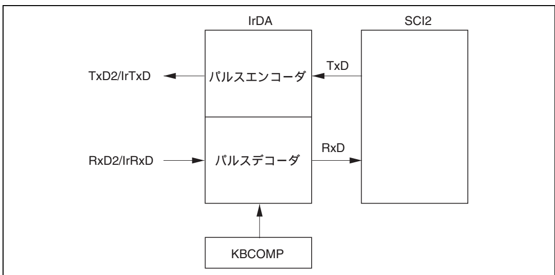
図 15.21 IrDA ブロック図
