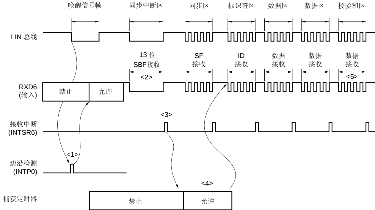
图 11-2. LIN 接收操作
