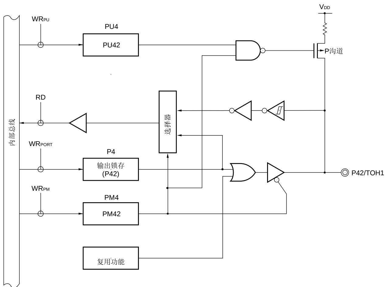
图 4-10 P42 的框图
