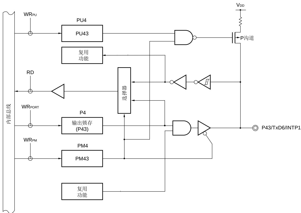
图 4-11 P43 的框图
