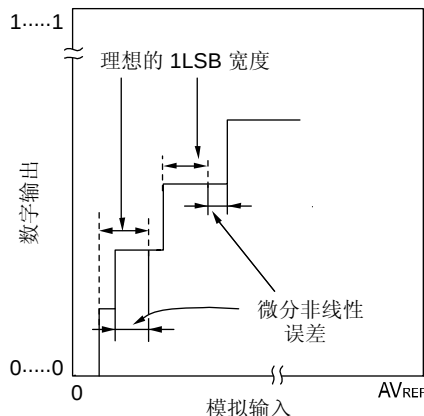
图 10-18. 微分线性误差
