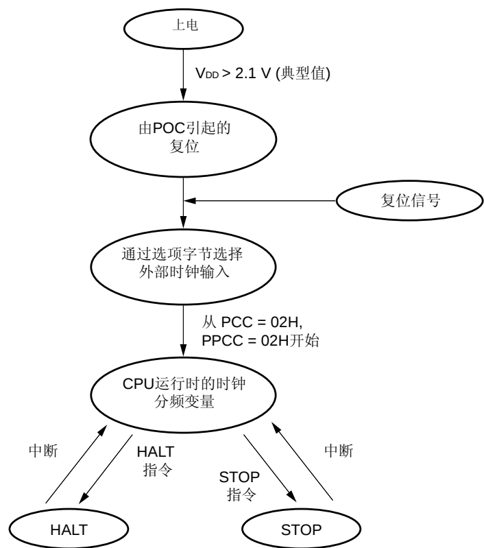
图 5-13 默认由外部时钟输入启动时的状态转换框图
