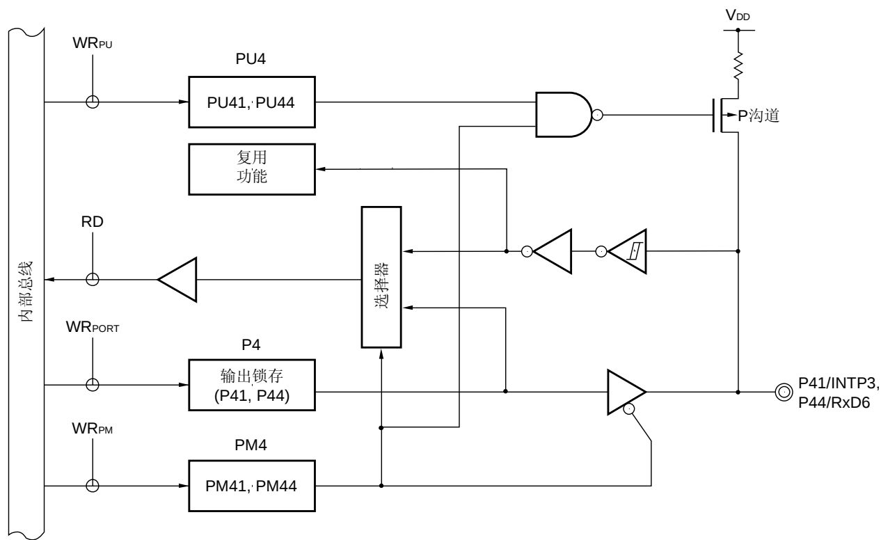
图 4-9 P41 和 P44 的框图
