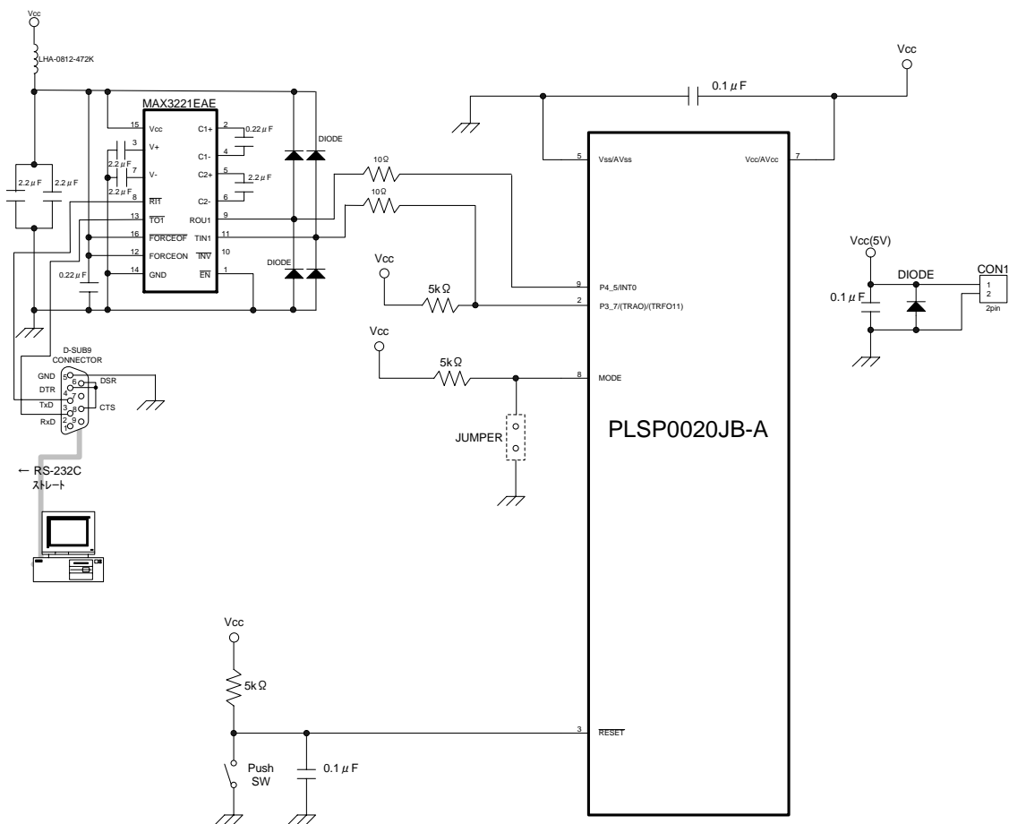
図 2 RS-232C ケーブルを使用した回路例(R8C/2H,2J グループ)
