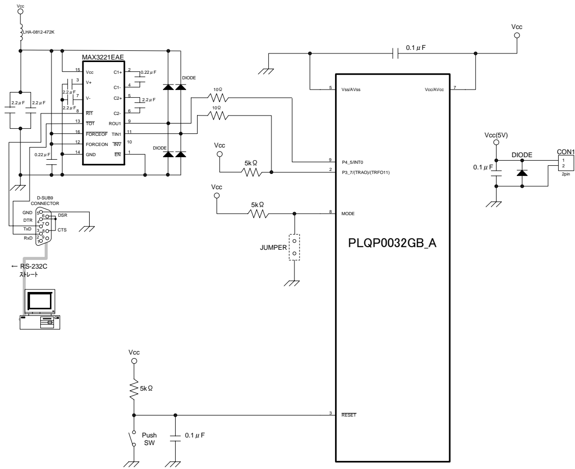
図 3 RS-232C ケーブルを使用した回路例(R8C/2G グループ)
