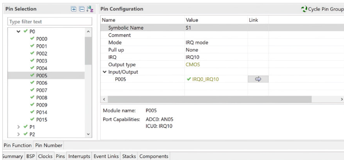
図9-6: ポートP005 はIRQ10 として適切に設定されているはずですが。
