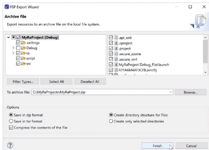
図5-6: e 2 studioのFSP エクスポートウィザード
