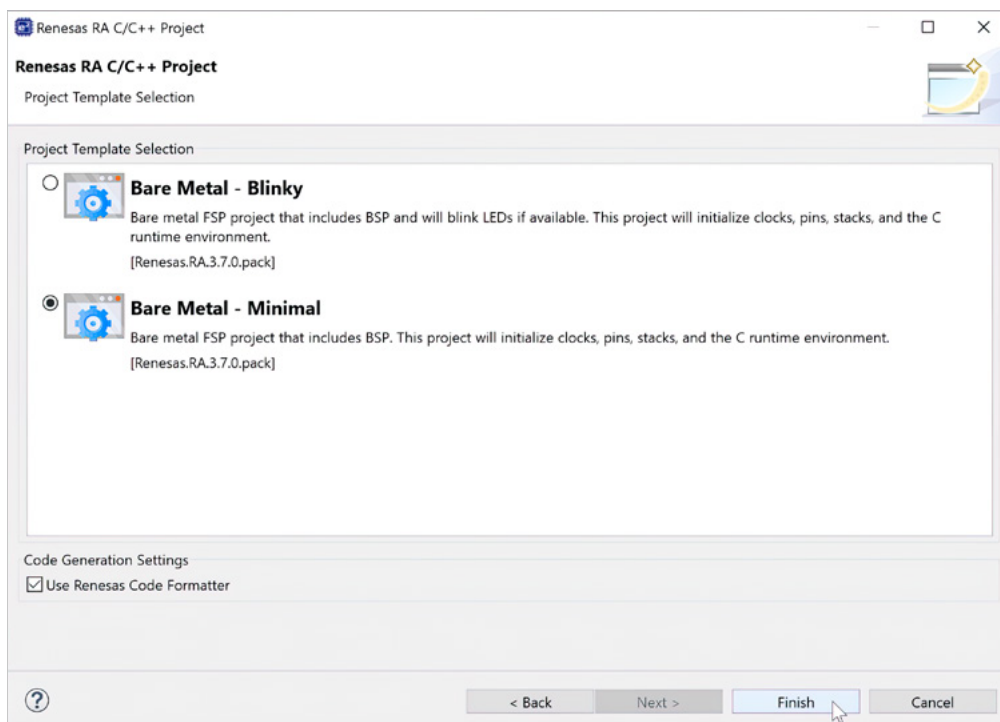
図8-7: 「Project Template Selection」は、プロジェクトの最初のコンテンツで使用可能なテンプレートが表示されます。
