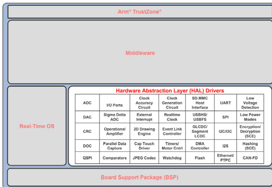
図2-3: HAL レイヤは、オンチップペリフェラルのドライバを提供します
