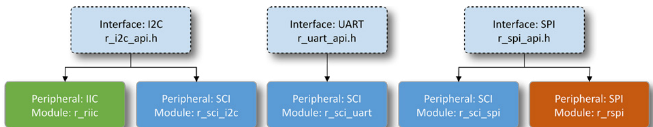
図3-4: RA ファミリのマイクロコントローラでは、一部のペリフェラルはインタフェースとインスタンスの間で1対1のマッピングを持ち、その他のペリフェラルは1対1のマッピングを持ちます
