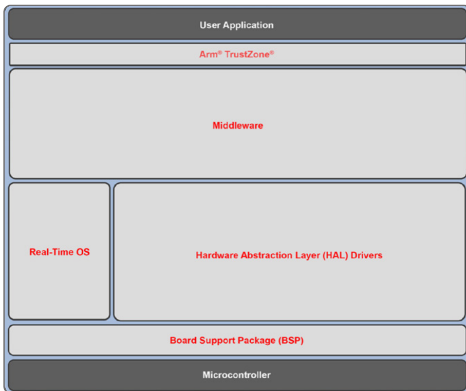
図3-1: フレキシブルソフトウェアパッケージのさまざまなレイヤ
