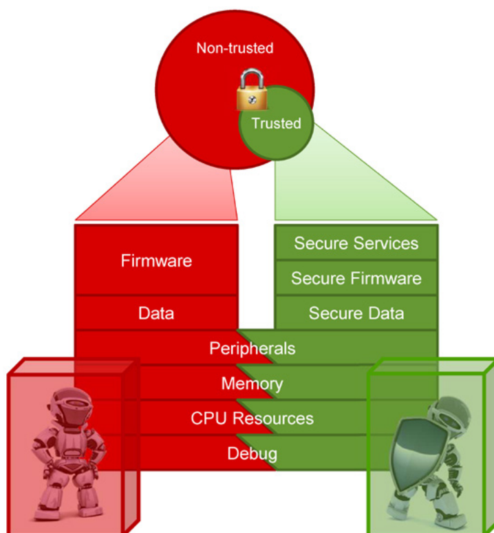
図11-1: TrustZone®を使用すると、マイクロコントローラのリソースを非セキュア領域とセキュア領域に分割できます。
