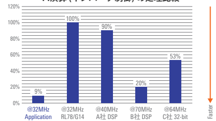
PI演算 (インバータ制御) の処理比較
