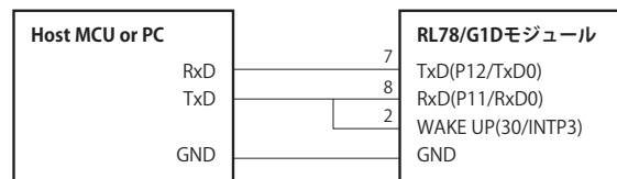
Host MCU との接続はUART 2線分岐接続方式
