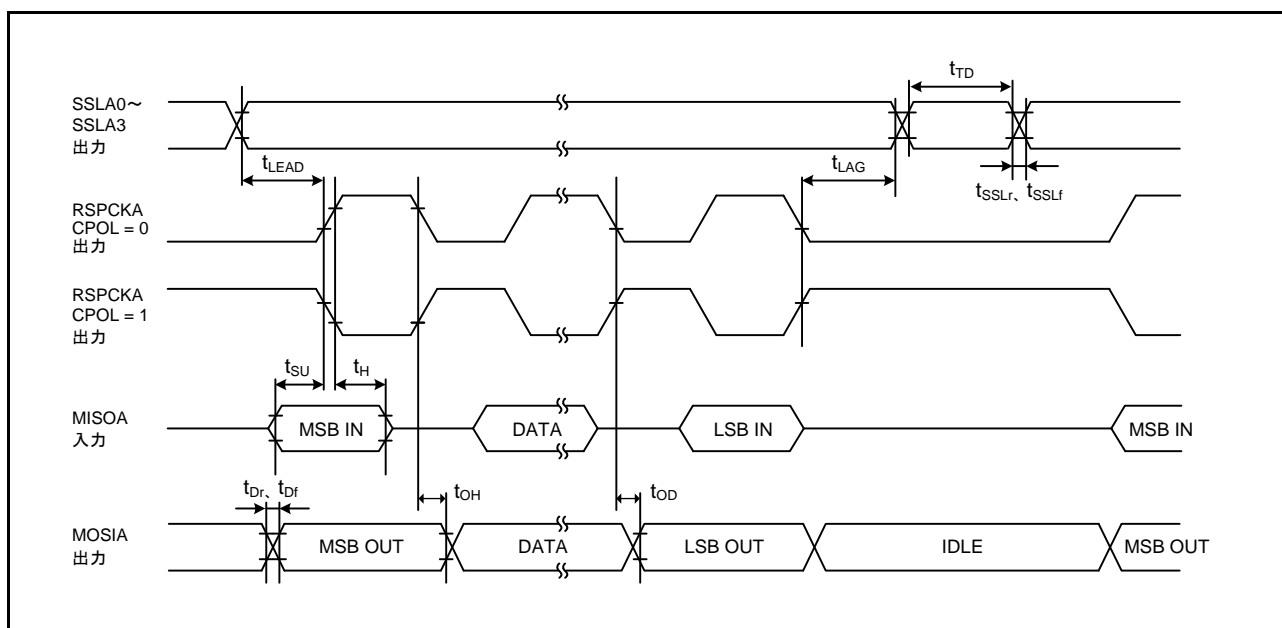
図 2.69 RSPCK タイミング (マスタ、CPHA = 0) (ビットレート : PCLKA を 2 分周以外に設定)
