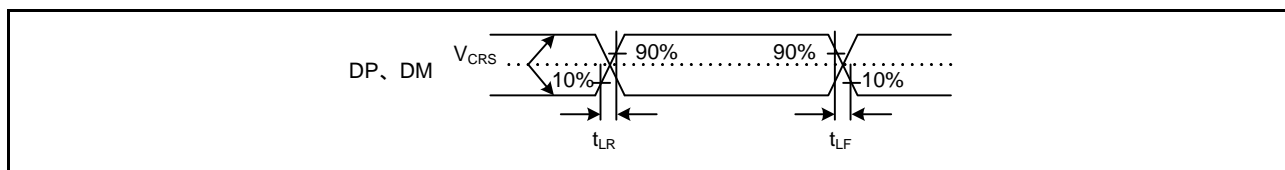
図 2.89 DP、DM 出カタイミング (ロースピード時)
