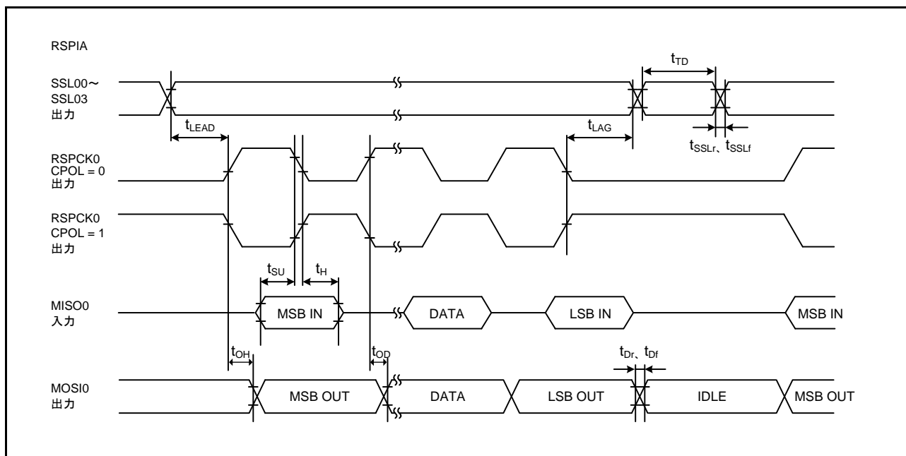
図 2.77 RSPIA タイミング ( マスタ、Motorola SPI、CPHA = 1)
