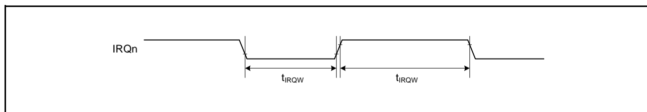
図 2.16 IRQ 割り込み入力タイミング
