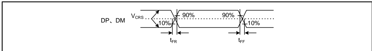
図 2.91 DP、DM 出カタイミング (フルスピード時)
