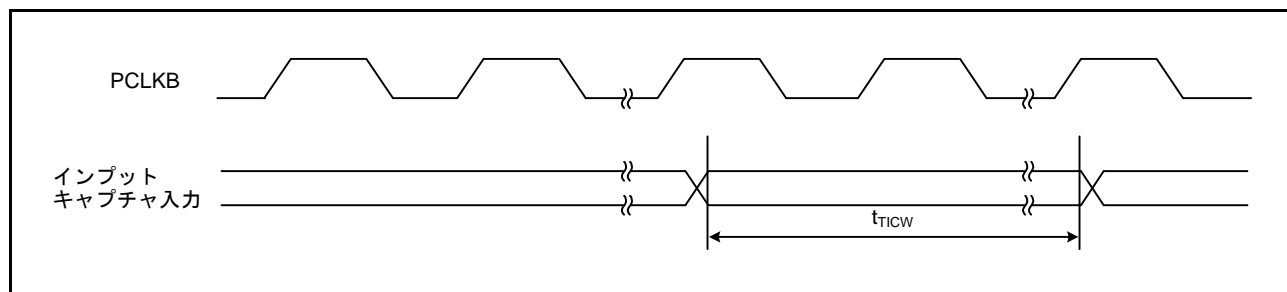
図 2.35 TPU インプットキャプチャ入力タイミング
