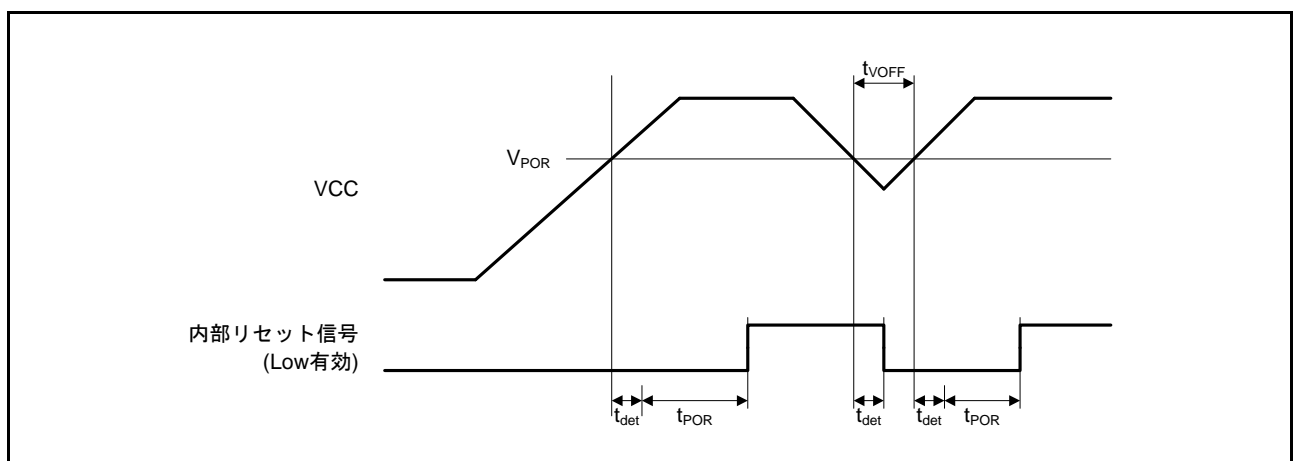
図 2.93 パワーオンリセットタイミング
