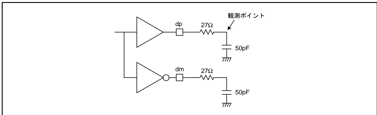
図 2.92 測定回路 (フルスピード時)
