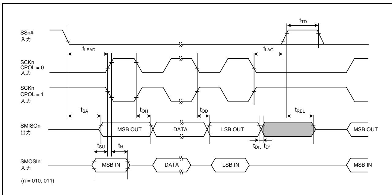
図 2.61 簡易 SPI タイミング (スレーブ、CPHA = 0)
