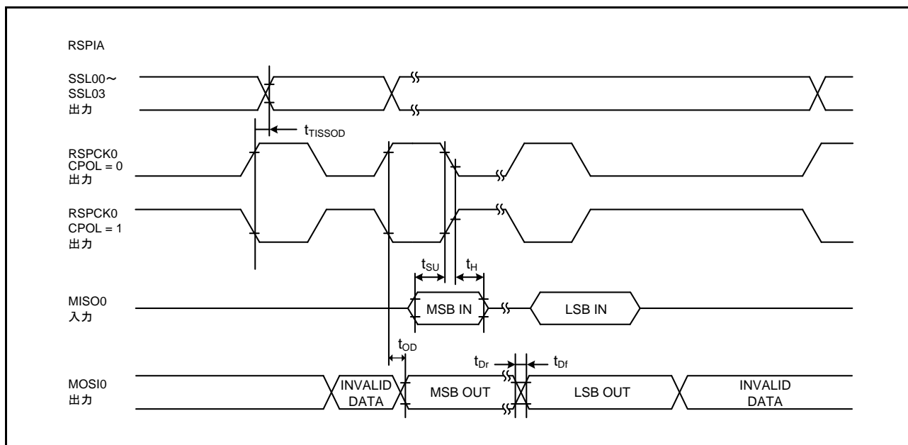
図 2.78 RSPIA タイミング ( マスタ、TI SSP)
