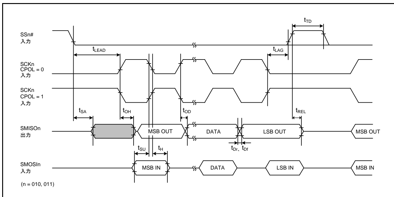
図 2.62 簡易 SPI タイミング (スレーブ、CPHA = 1)
