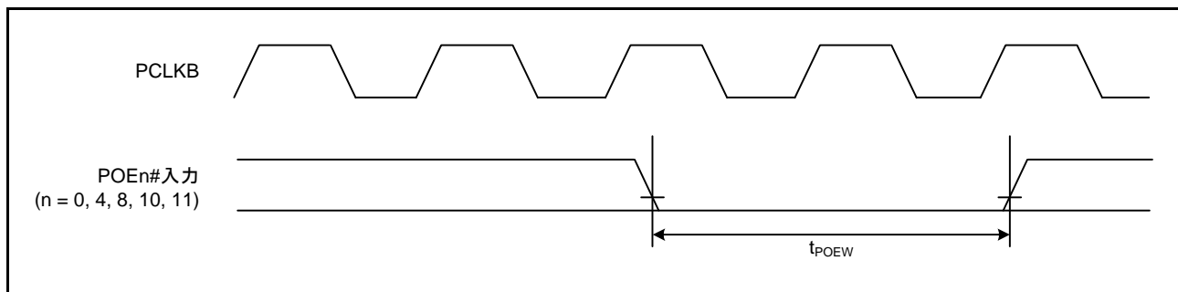
図 2.41 POE# 端子入力タイミング
