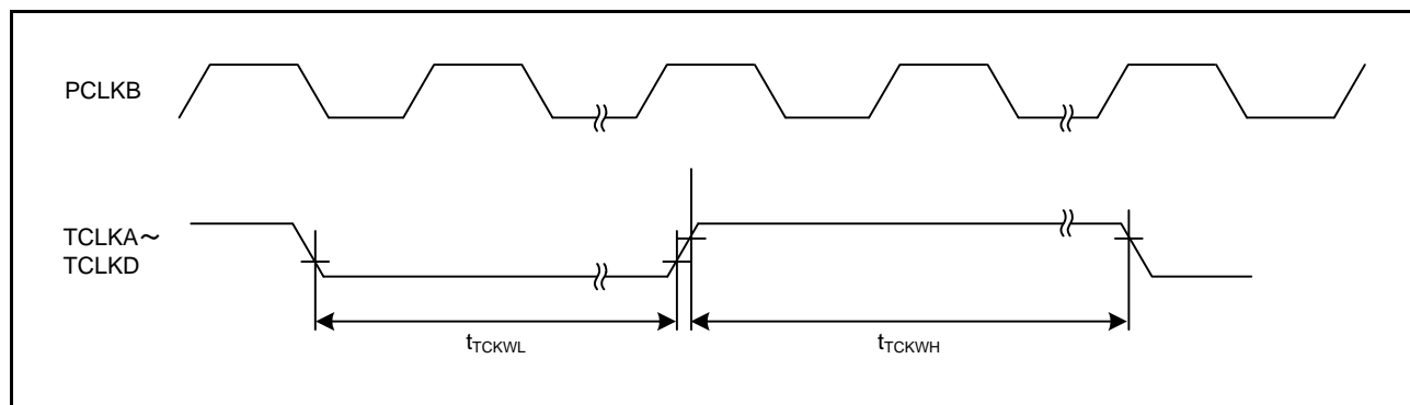
図 2.36 TPU クロック入力タイミング
