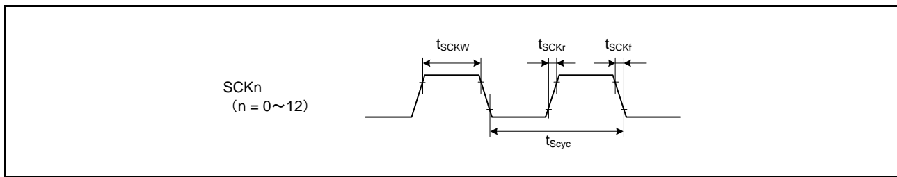
図 2.47 SCK クロック入力タイミング
