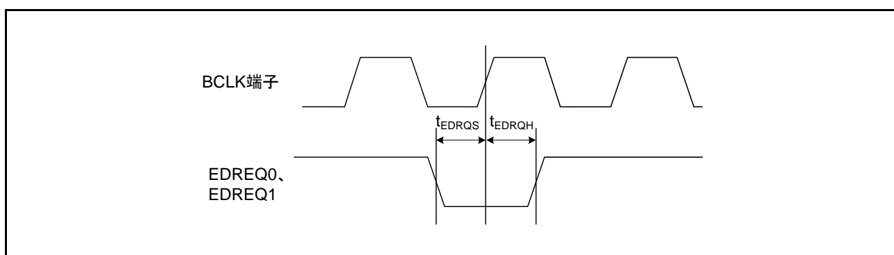
図 2.31 EDREQ0, EDREQ1 入カタイミング
