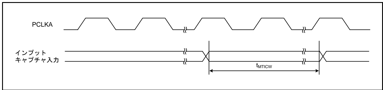
図 2.39 MTU 入力キャプチャ入力タイミング
