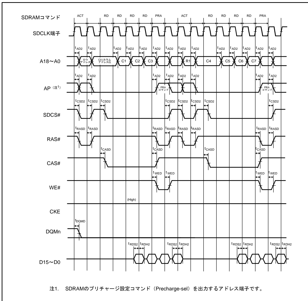
図 2.28 SDRAM 空間複数リード行またぎバスタイミング
