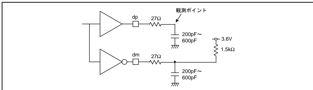
図 2.90 測定回路 (ロースピード時)
