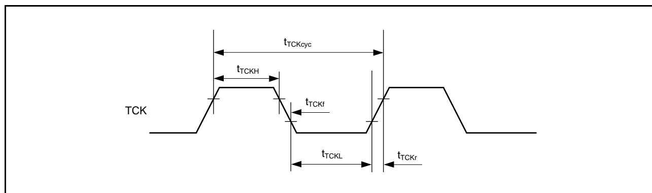
図 2.102 バウンダリスキャン TCK タイミング
