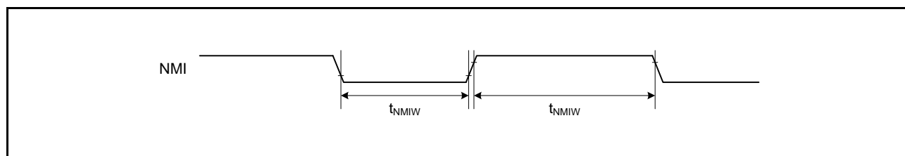
図 2.15 NMI 割り込み入力タイミング
