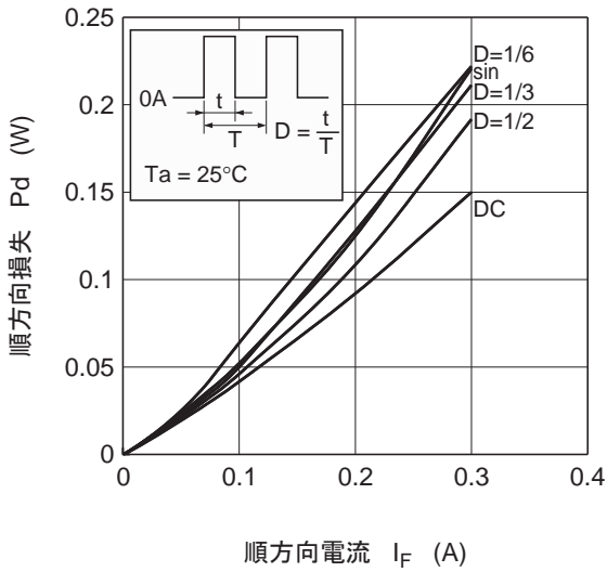
図4. 順方向損失 対 順電流特性 ( T_a = 25^\circ\text{C} )
