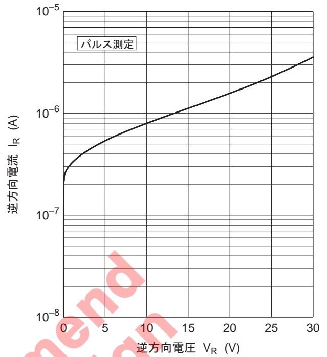
図2. 逆方向特性
