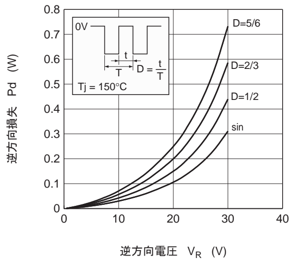
図5. 逆方向損失 対 逆電圧特性 ( T_j = 150^\circ\text{C} )
