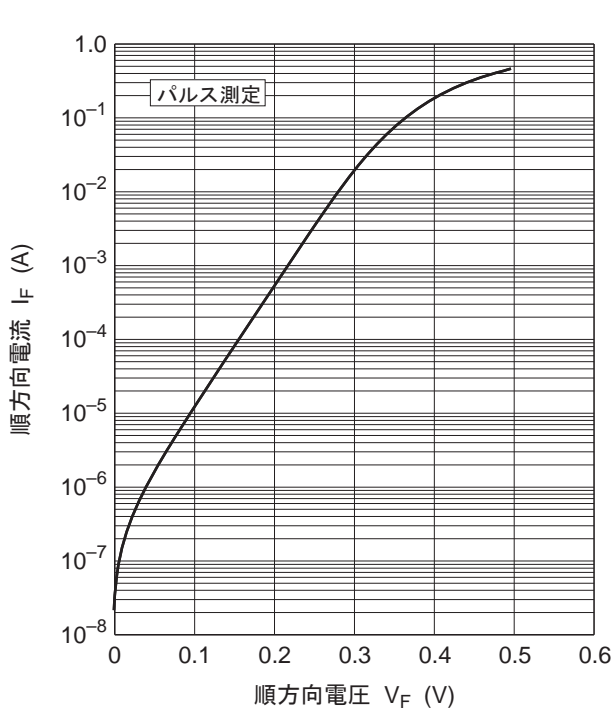
図1. 順方向特性
