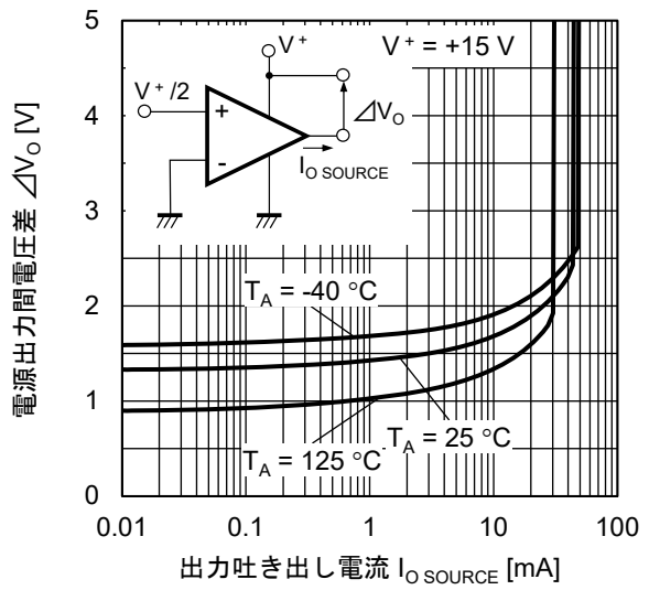
\Delta V_O - I_{O\text{ SOURCE}} 特性
