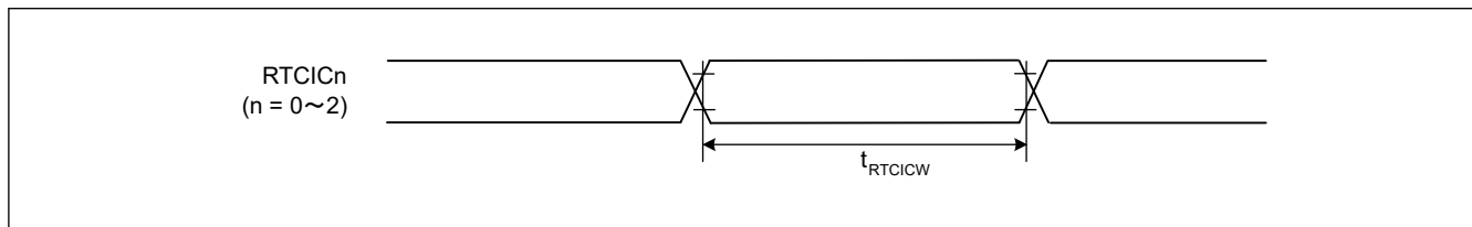
図 2.43 RTCICn 入カタイミング
