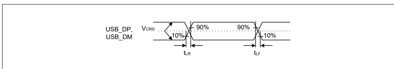
図 2.108 Low-speed モードにおける USB_DP、USB_DM の出力タイミング
