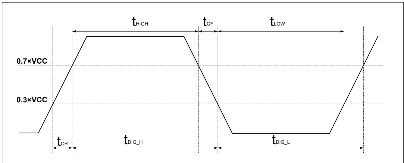
図 2.74 t_{DIG\_H} 、 t_{DIG\_L}
