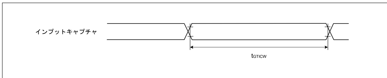
図 2.45 GPT インพุットキャプチャタイミング
