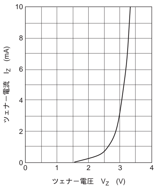
図1. ツェナー特性
