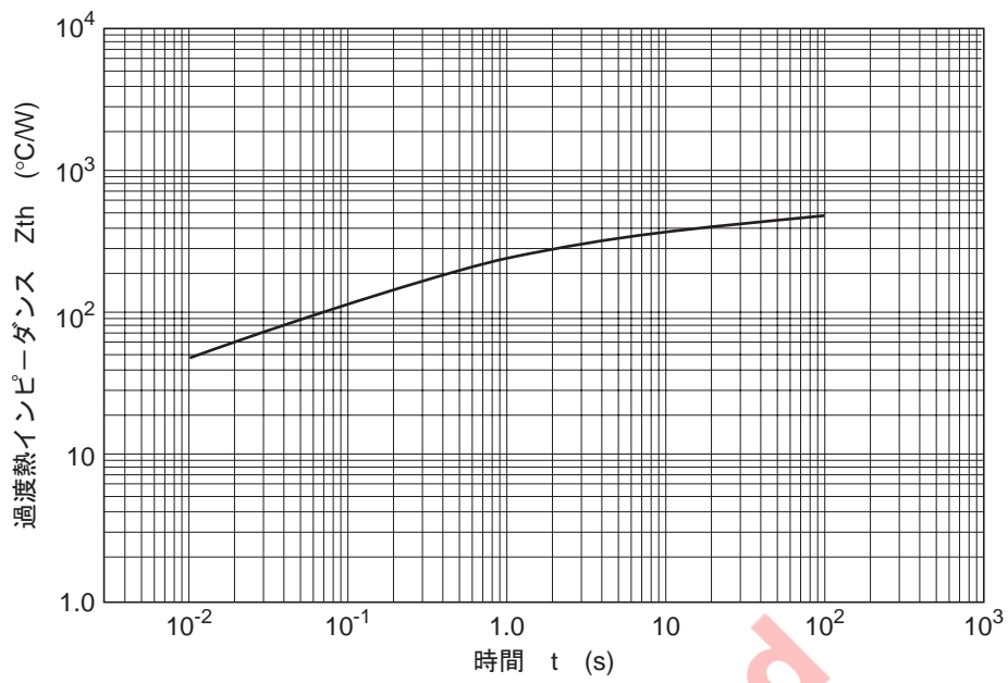
図4. 過渡熱インピーダンス特性
