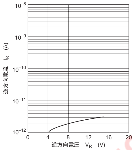
图1. 逆方向特性
