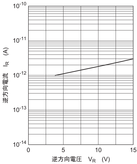
图1. 逆方向特性
