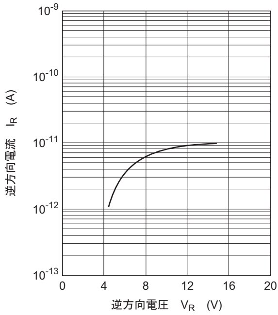
图1. 逆方向特性
