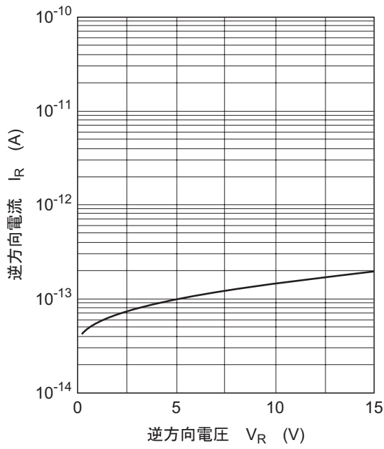
図1. 逆方向特性
