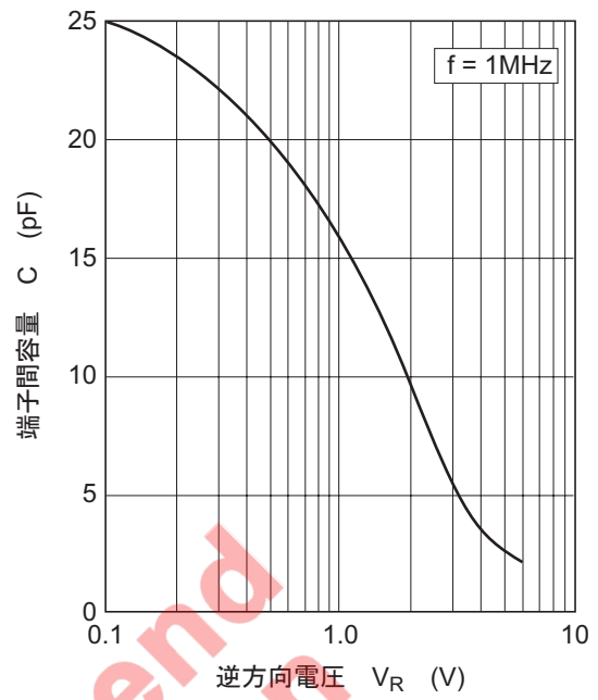
図2. 端子間容量 对 逆電圧特性
