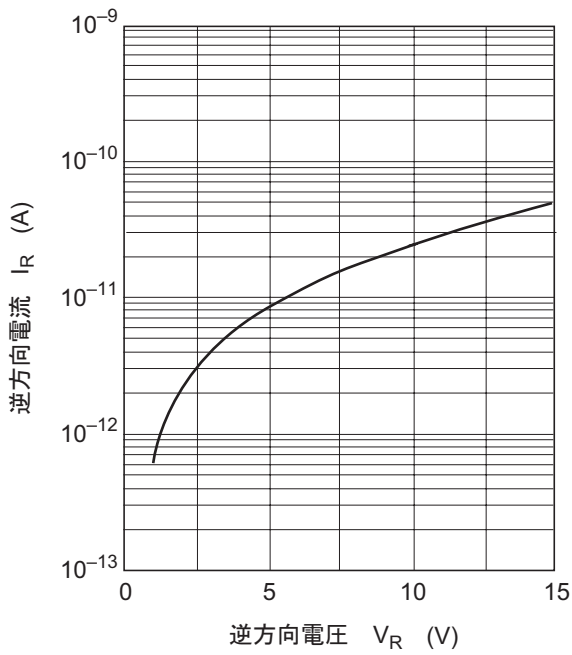
图1. 逆方向特性
