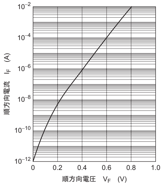
图1. 顺方向特性
