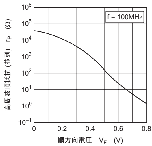
图5 高周波順抵抗 (並列) 对 順方向電圧
