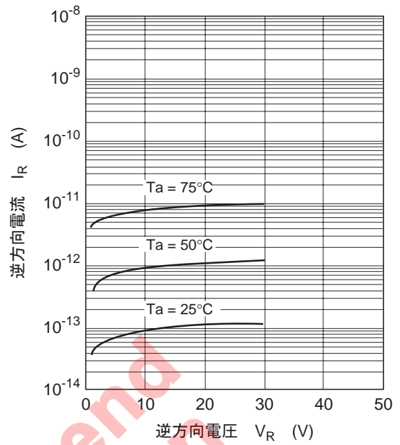
图2. 逆方向特性
