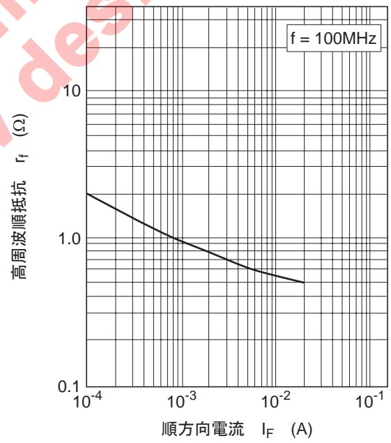
图4. 高周波順抵抗 对 順電流特性
