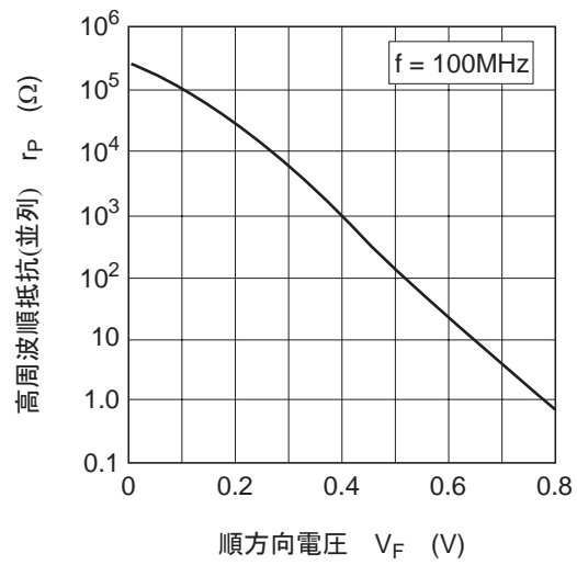
図5. 高周波順抵抗(並列) 对 順電圧特性
