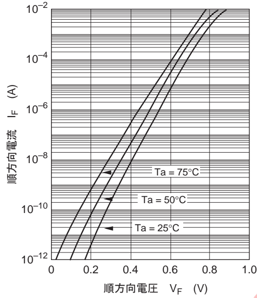
图1. 顺方向特性
