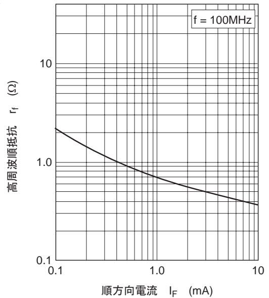
图4. 高周波顺抵抗 对 顺电流特性
