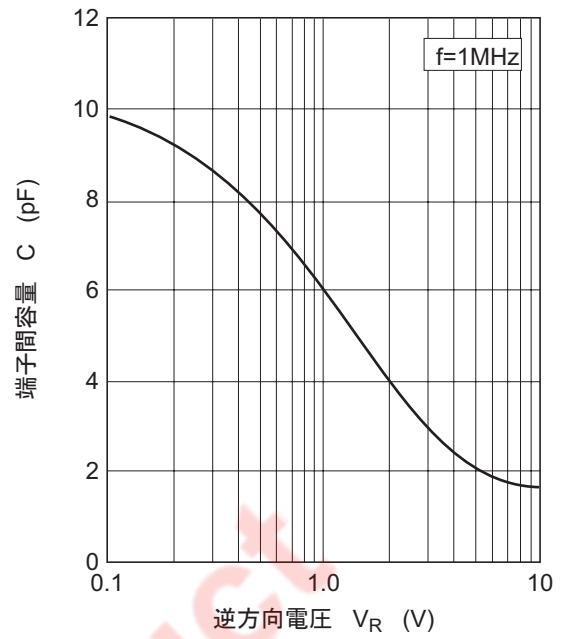
図2. 端子間容量 对 逆電圧特性
