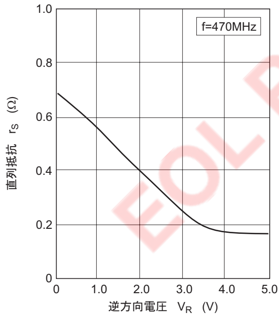
図3. 直列抵抗 对 逆電圧特性
