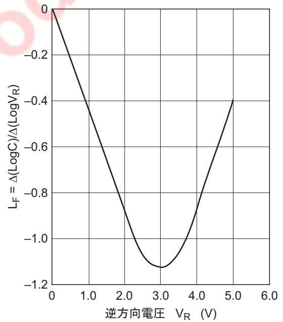
図4. L_F 对 逆電圧特性
