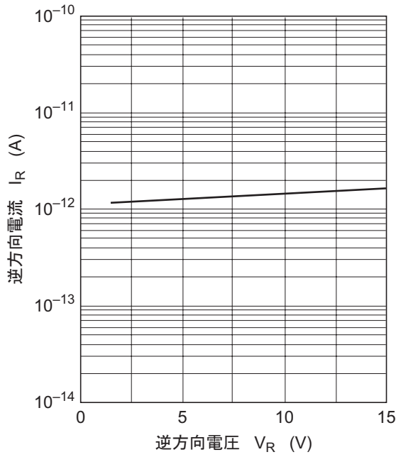
図1. 逆方向特性
