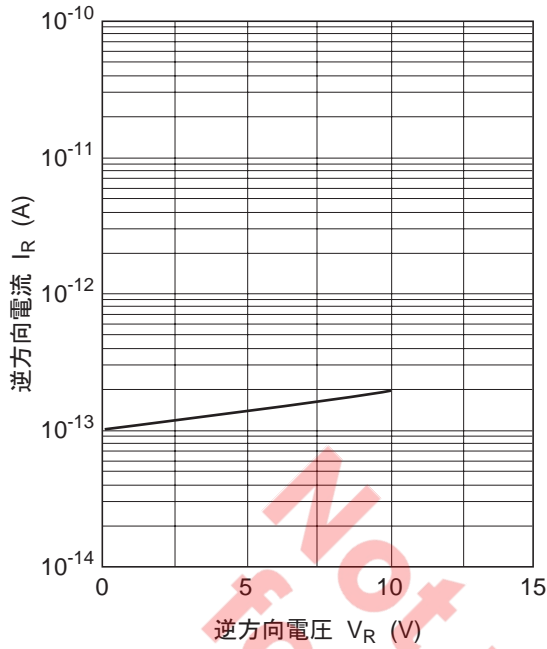
图1. 逆方向特性
