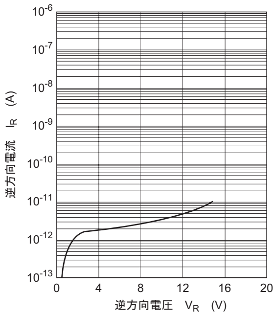
图1. 逆方向特性
