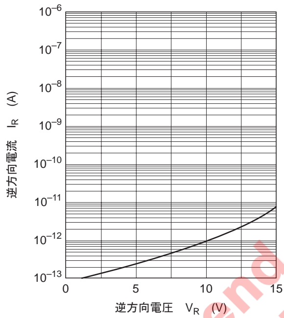
图2. 逆方向特性
