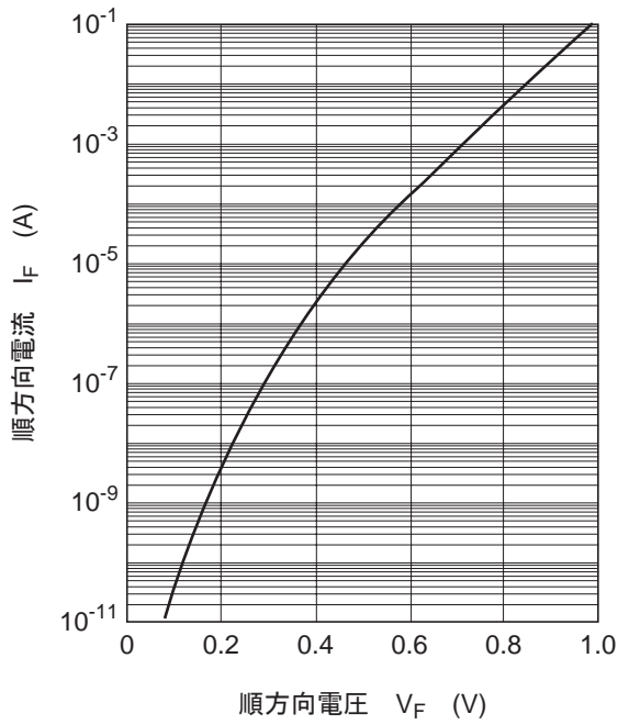
图1. 順方向特性
