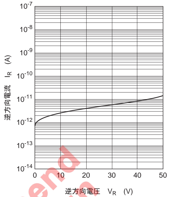
图2. 逆方向特性
