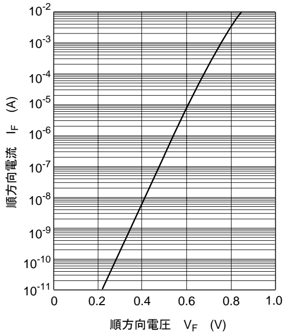
图1. 顺方向特性
