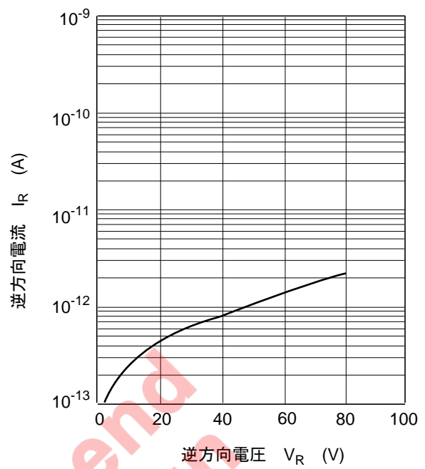
图2. 逆方向特性
