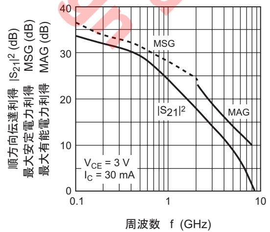
最大有能電力利得, 最大安定電力利得 対周波数特性
