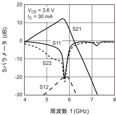
Sパラメータ 対 周波数特性
