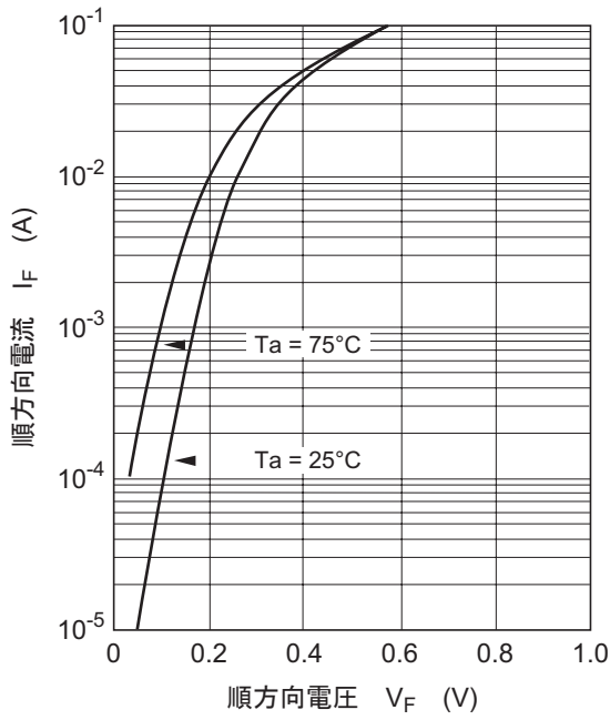
图1. 順方向特性
