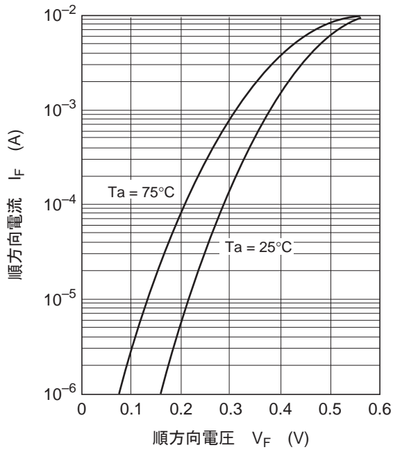
图1. 顺方向特性
