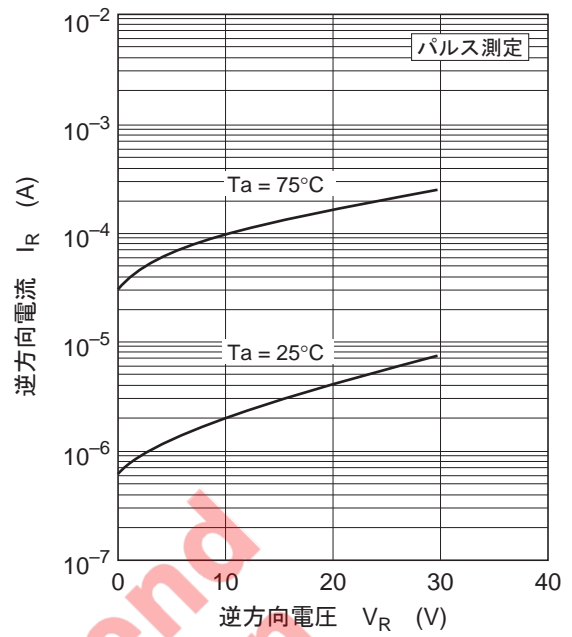
図2. 逆方向特性
