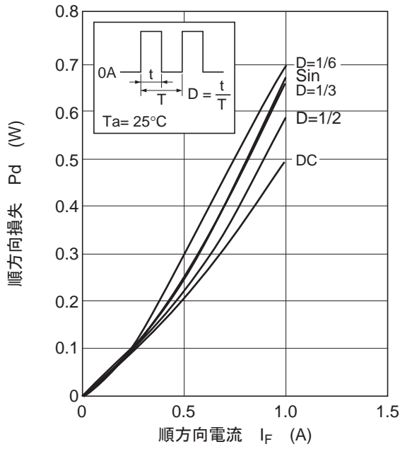
图4. 順方向損失 对 順電流特性
