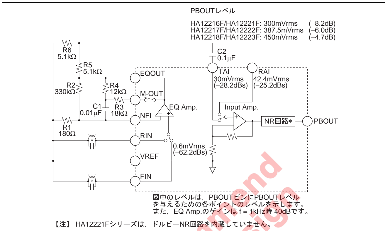
図3 入力部のブロック図
