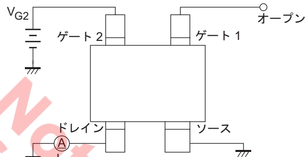
動作項目のDCバイアス回路 ( I_{D(op)} , |y_{fs}| , C_{iss} , C_{oss} , C_{rss} , NF, PG)
