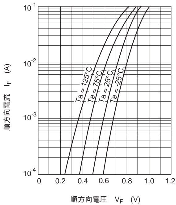
图1. 顺方向特性
