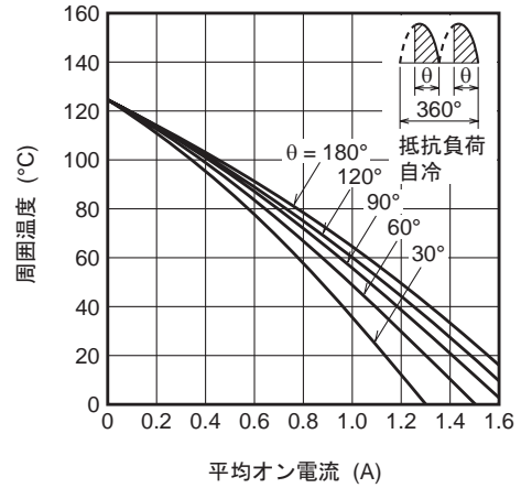
平均オン電流の限界値 (単相両波)
