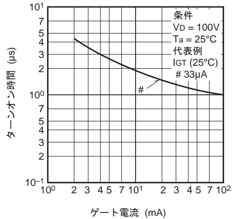
ターンオン時間-ゲート電流
