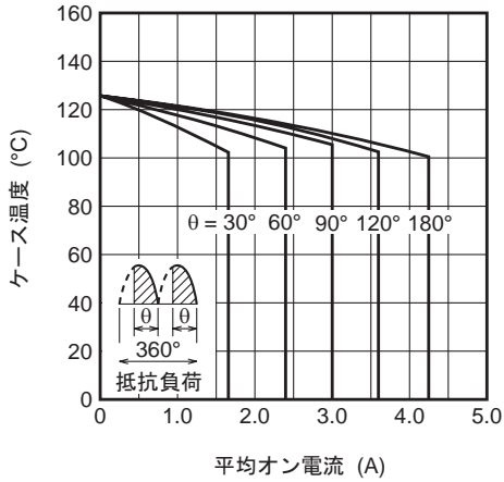
平均オン電流の限界値 (単相両波)
