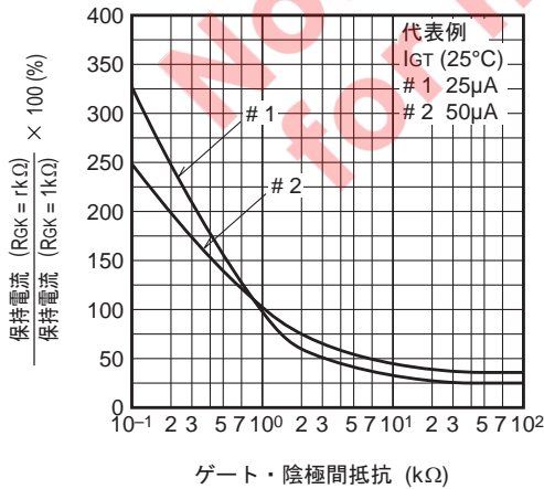
保持電流-ゲート・陰極間抵抗
