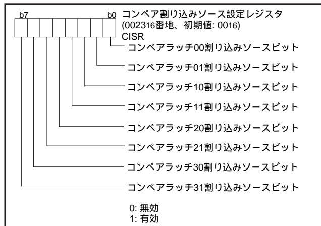
図 38 . コンペア割り込みソース設定レジスタの構成
