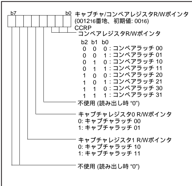
図 32 . キャプチャ/コンペアレジスタ R/W ポインタの構成
