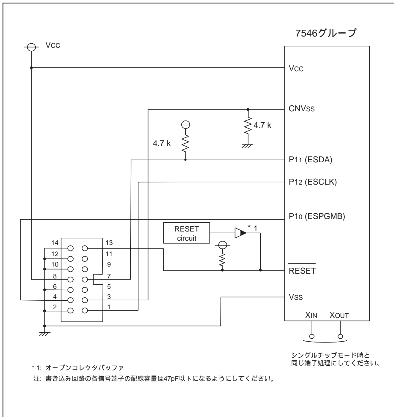
図 92 . E8 プログラム使用時の基板上の端子処理例
