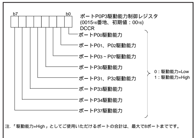
図 14 . ポート P0P3 駆動能力制御レジスタの構成
