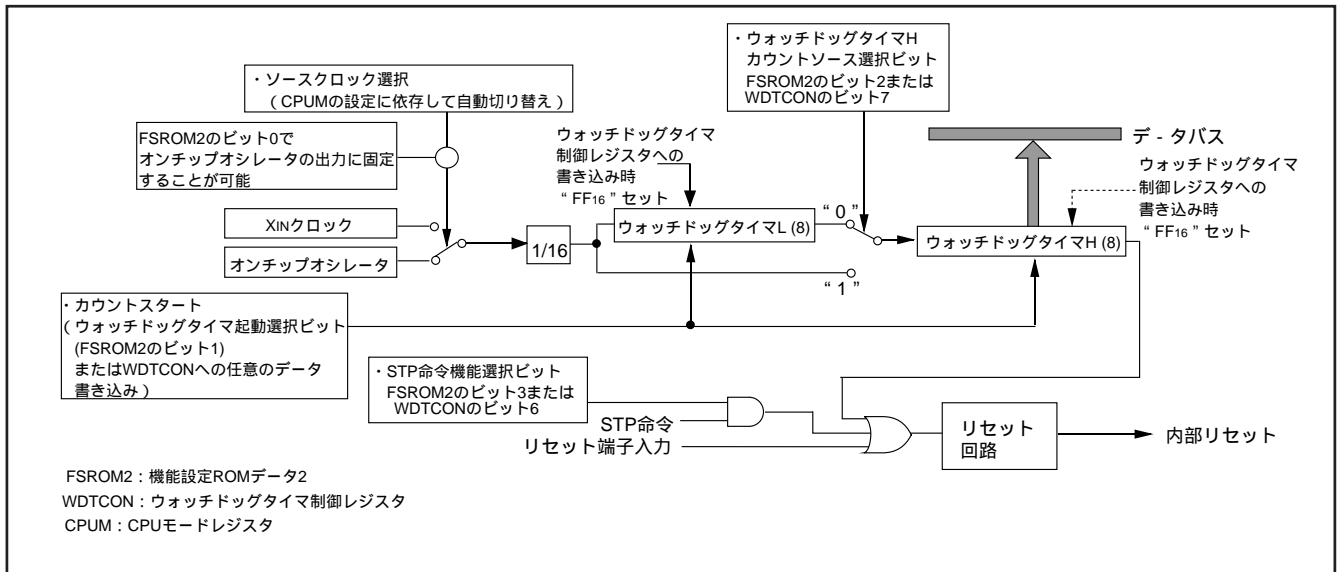
図 68 . ウォッチドッグタイマのブロック図
