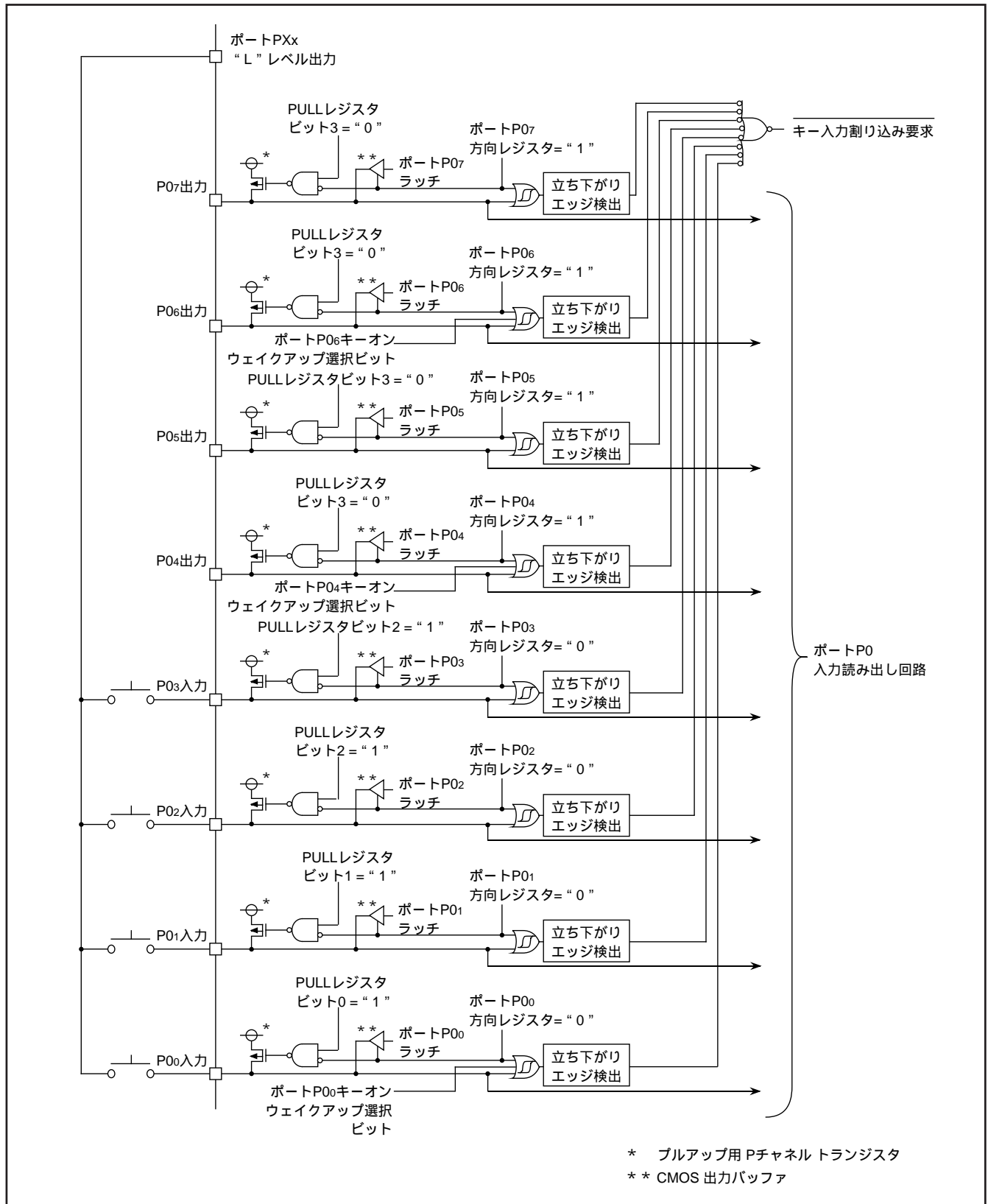
図 25 . キー入力割り込み使用時の結線例とポート P0 のブロック図
