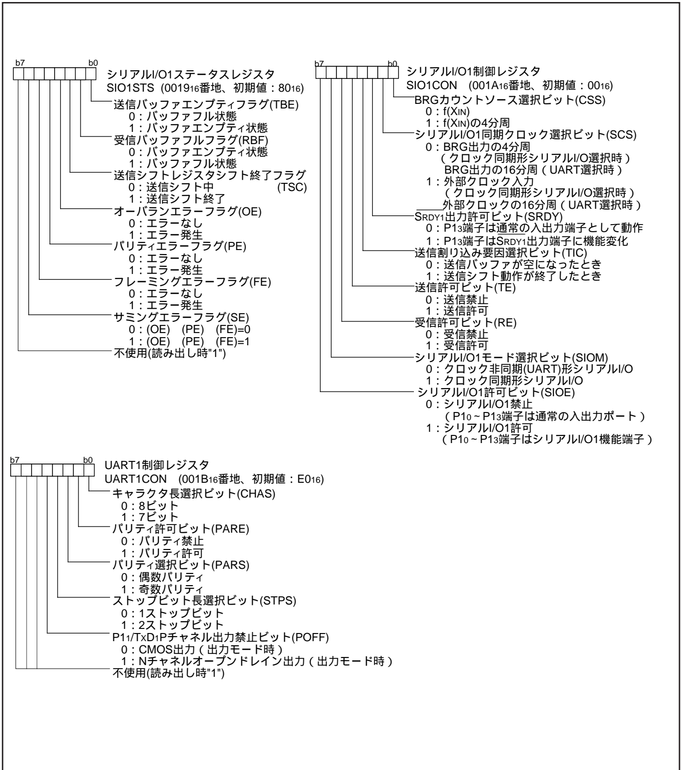
図 56 . シリアルI/O1 関係レジスタの構成
