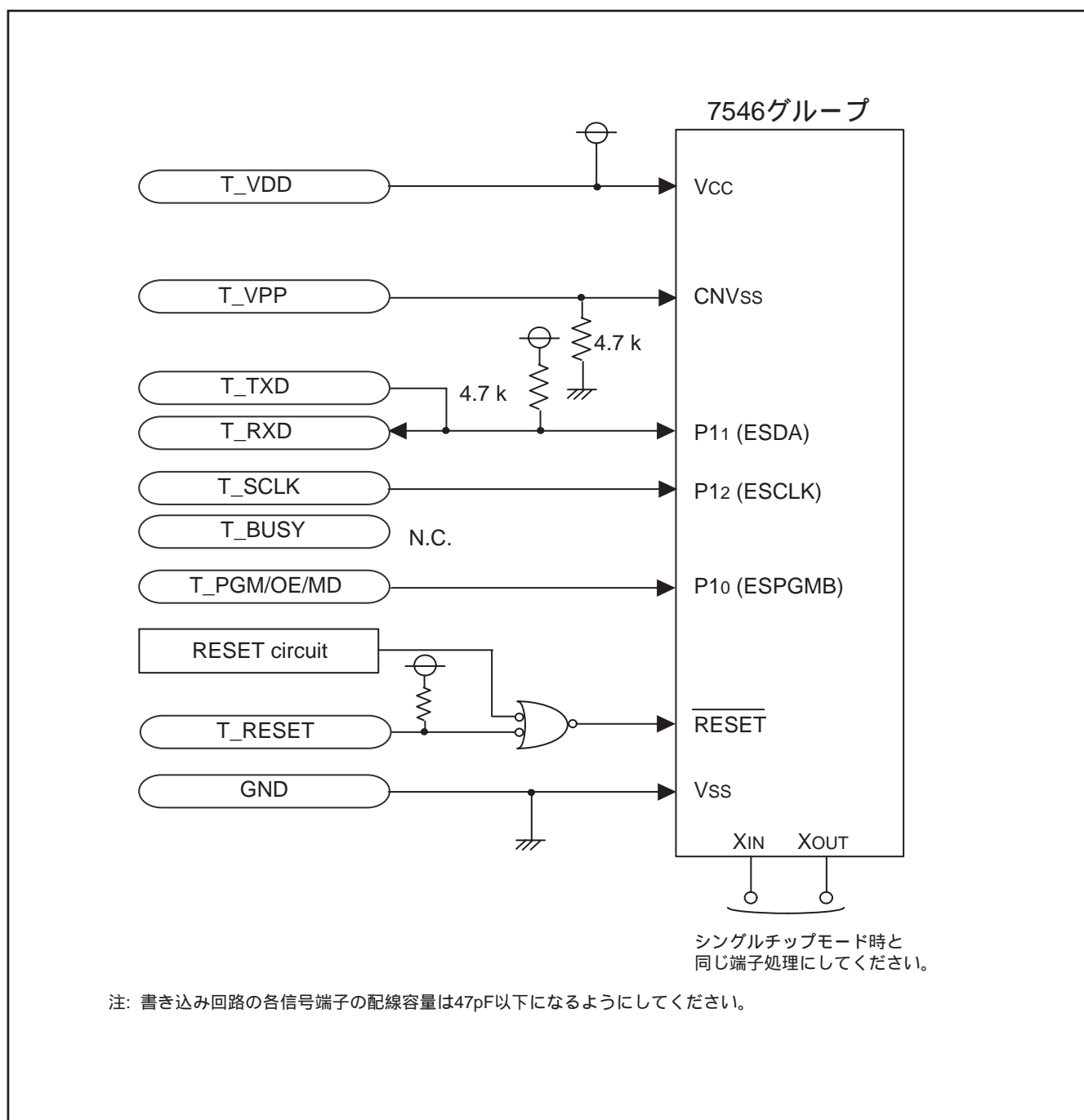
図 93 . 彗星電子システム製プログラマ使用時の基板上的端子処理例
