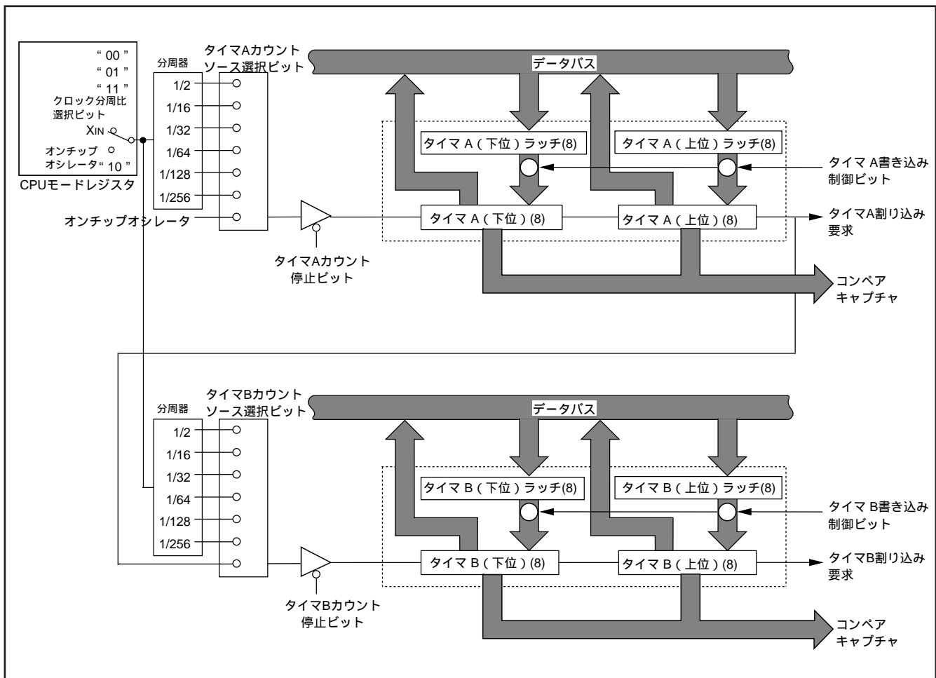
図 31 . タイマ A 及びタイマ B のブロック図
