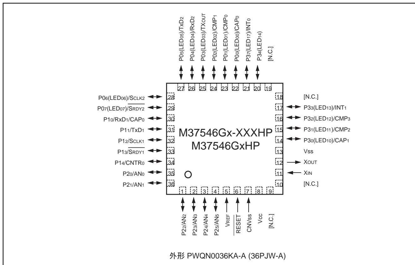
図 3 . ピン接続図 ( PWQN0036KA-A パッケージ )
