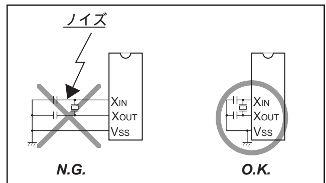
図 96 . クロック入出力端子の配線
