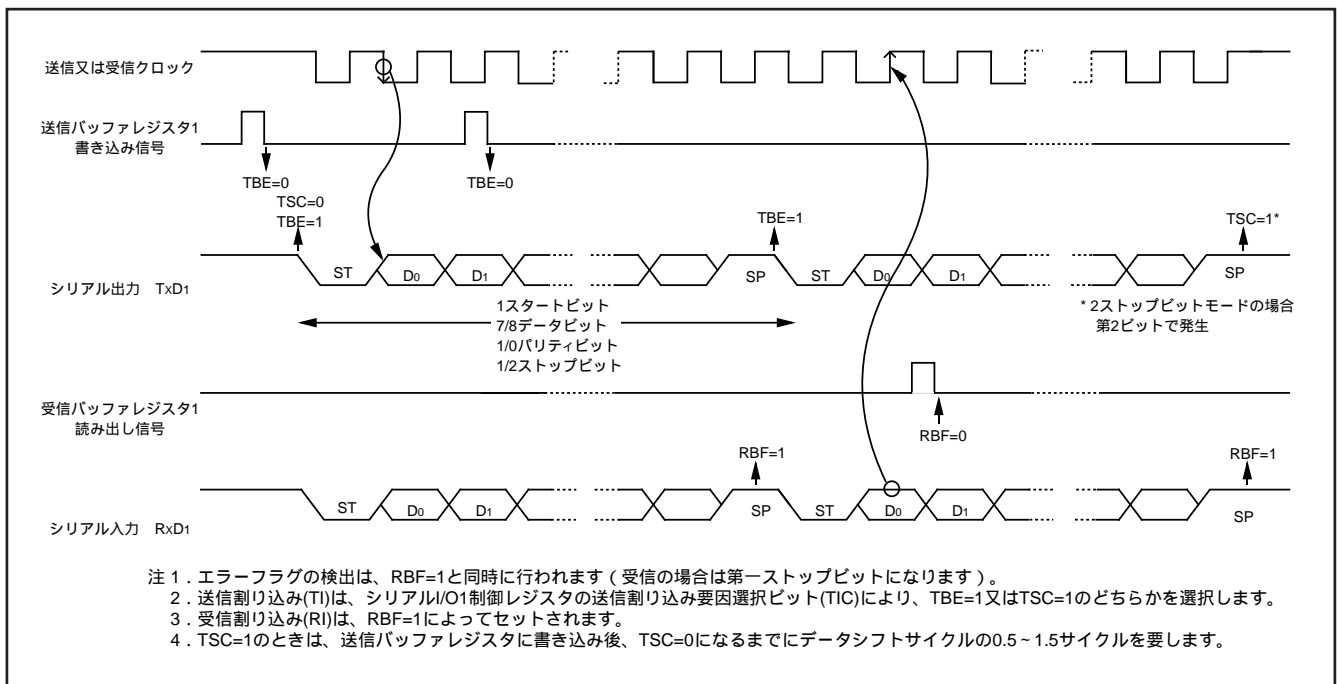
図 55 . UART 形シリアル I/O1 動作図
