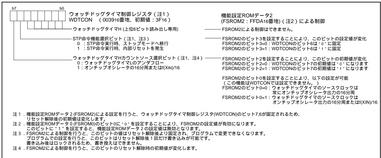
図 69 . ウォッチドッグタイマ制御レジスタの構成
