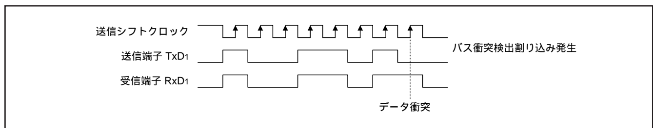
図 59 . バス衝突検出割り込みのタイミング図
