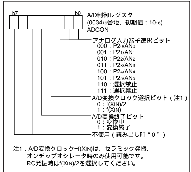
図 65 . A/D 制御レジスタの構成
