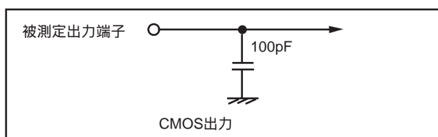
図 106 . スイッチング特性測定回路図
