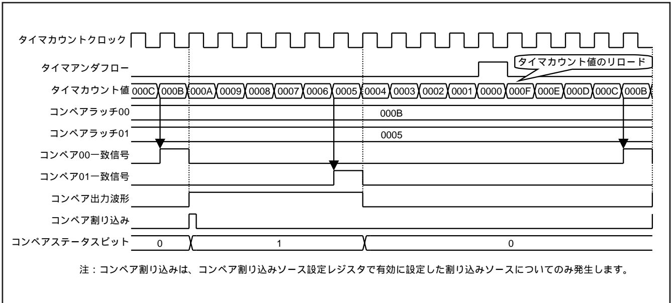
図 42 . コンペア出力波形図 (基本波形)
