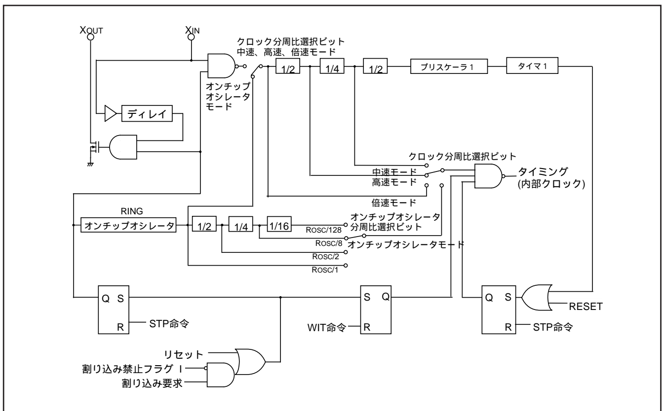
図 81 . システムクロック発生回路ブロック図 (RC 発振時)
