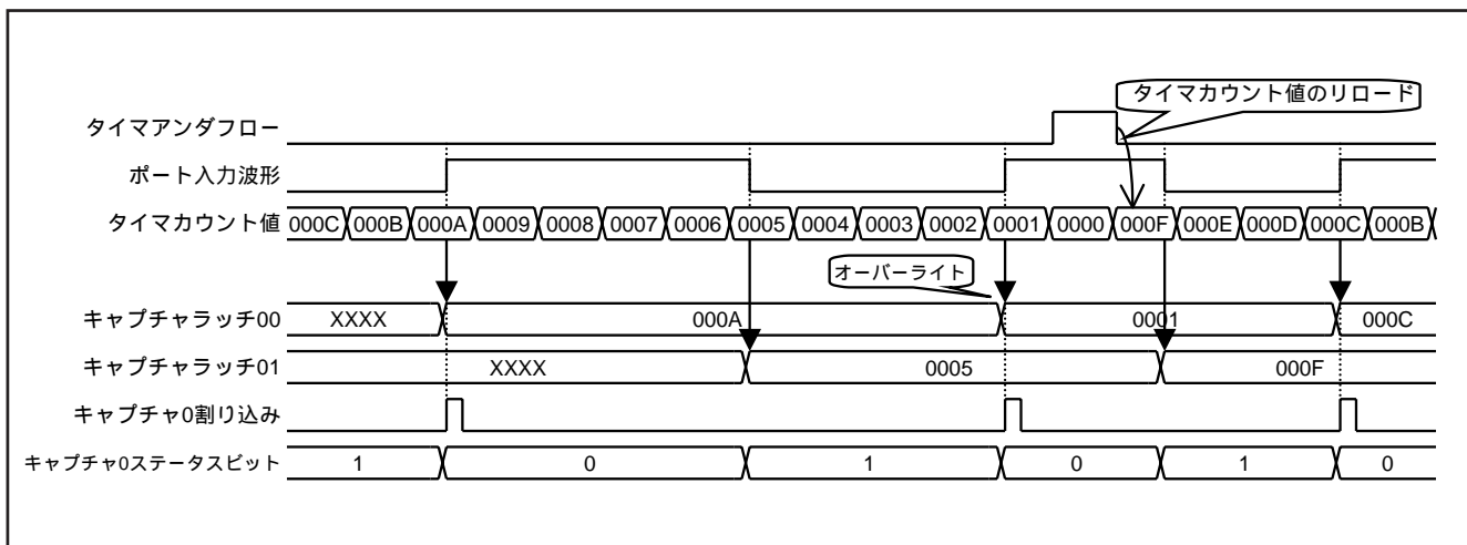
図 50 . キャプチャ入力波形図 (キャプチャ0 割り込みエッジ選択ビット : 立ち上がり選択時)
