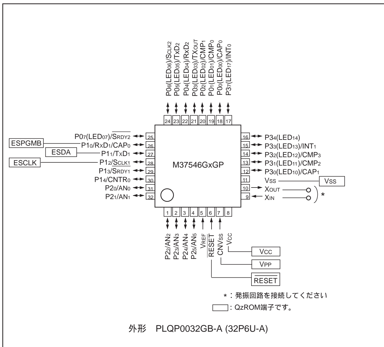
図 89 . 端子結線図(M37546GxGP)
