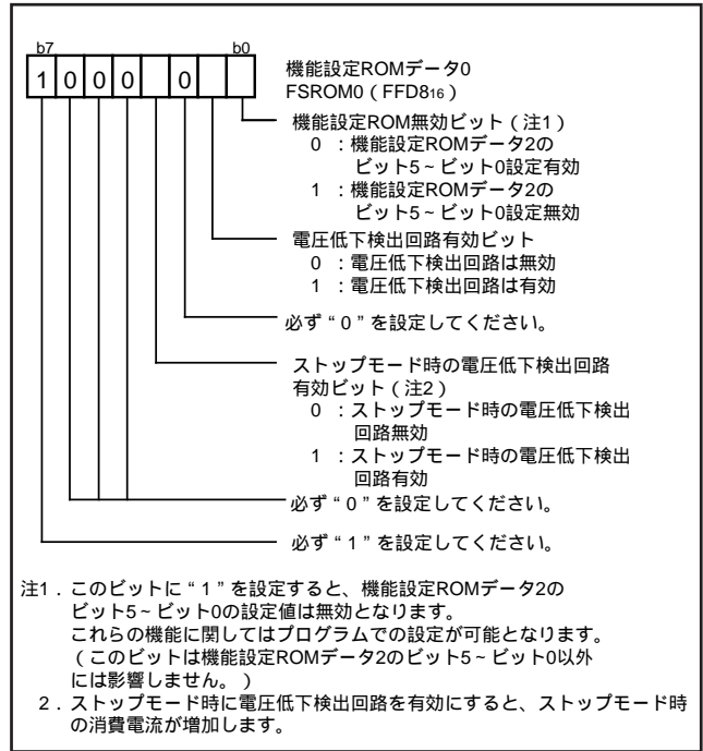
図 86 . 機能設定 ROM データ 0 の構成
