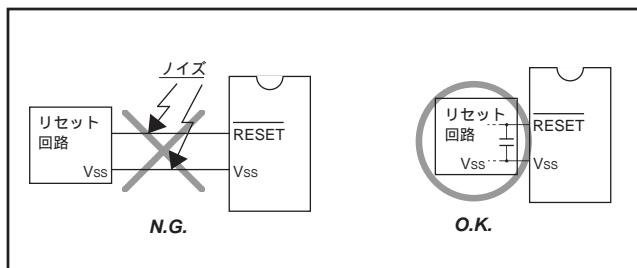
図 95 . リセット入力端子の配線
