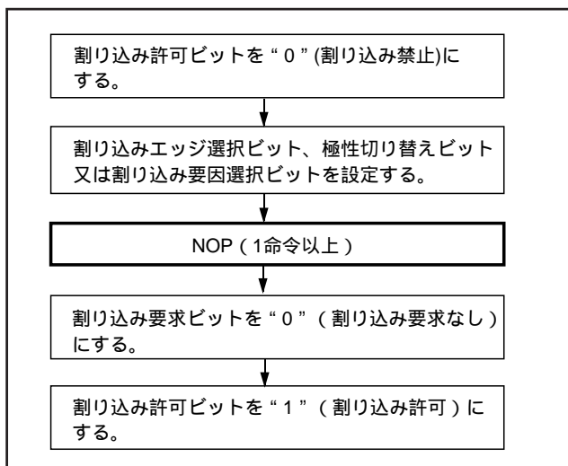
図4. 関連レジスタの設定手順
