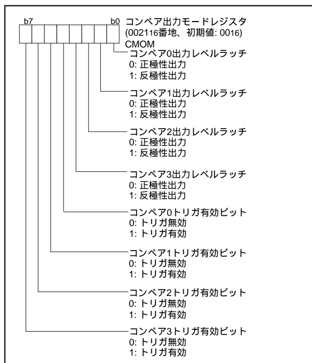
図 36 . コンペア出力モードレジスタの構成
