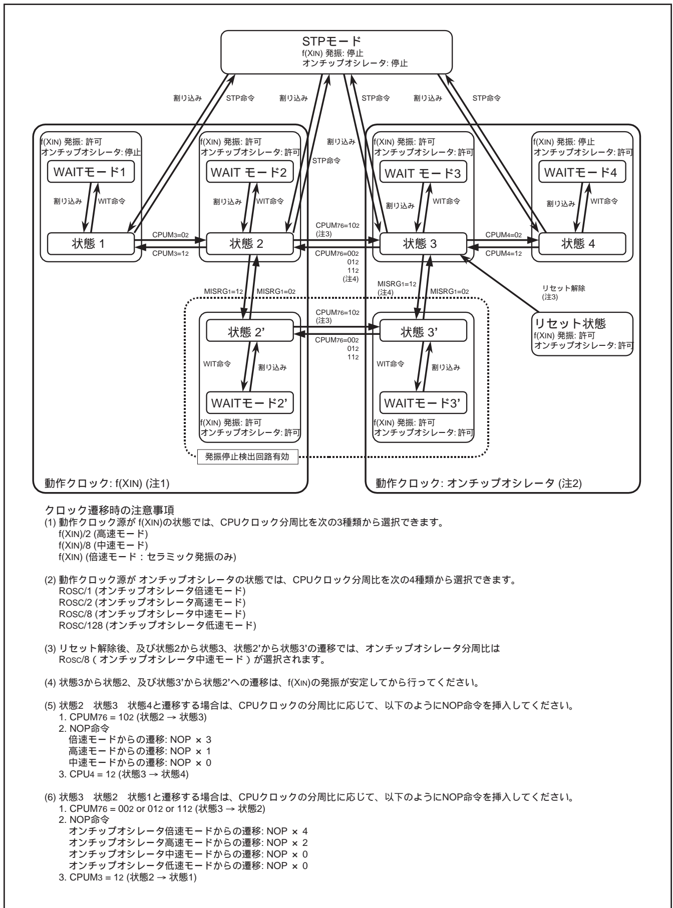
図 82 . クロック発生回路状態遷移図
