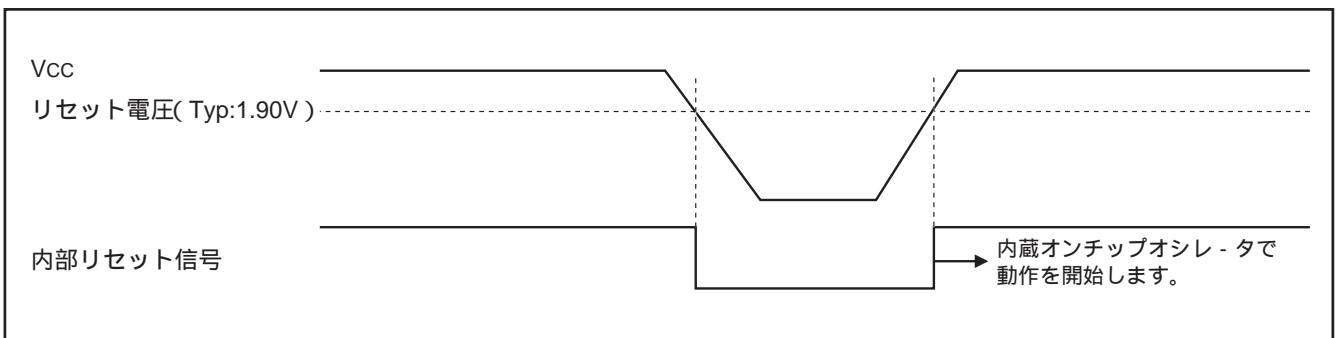
図71. 電圧低下検出回路の動作波形図
