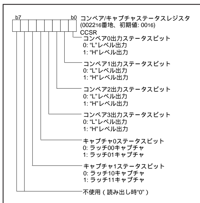
図 37 . キャプチャ/コンペアステータスレジスタの構成
