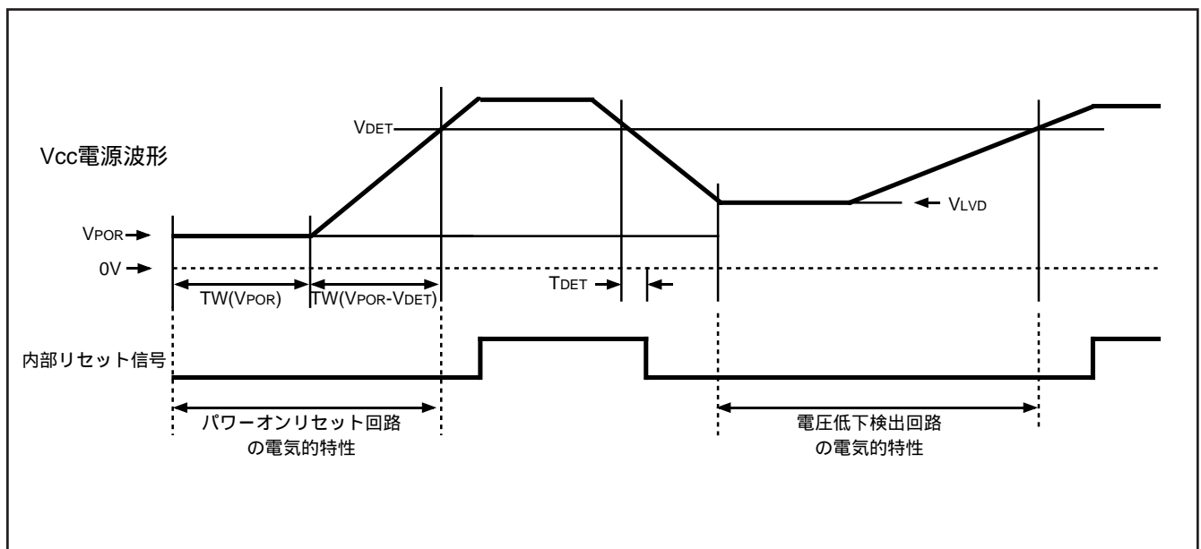
図 105 . パワーオンリセット回路、電圧低下検出回路の電気的特性
