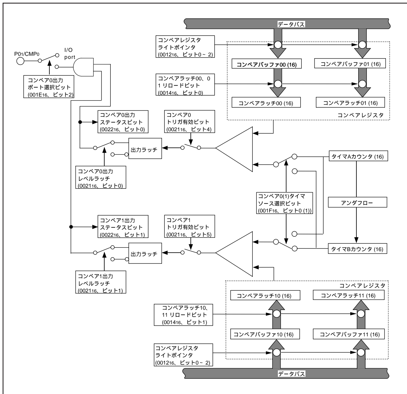
図 41 . 変調出力モード時のブロック図
