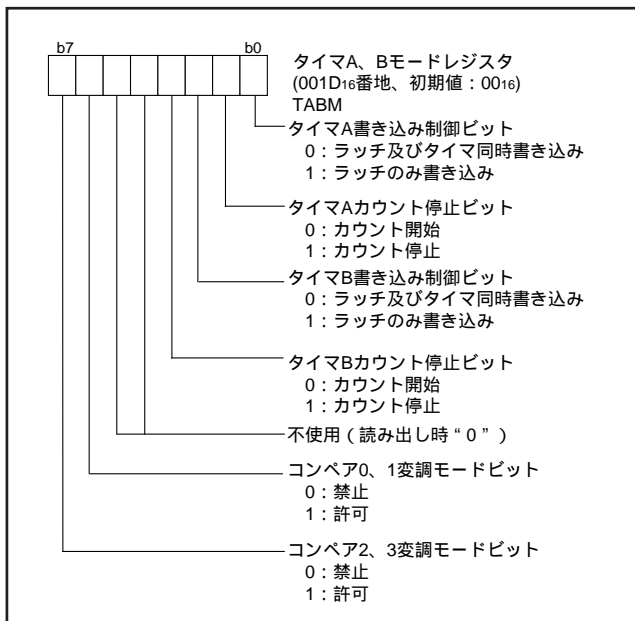
図 29 . タイマ A、B モードレジスタの構成
