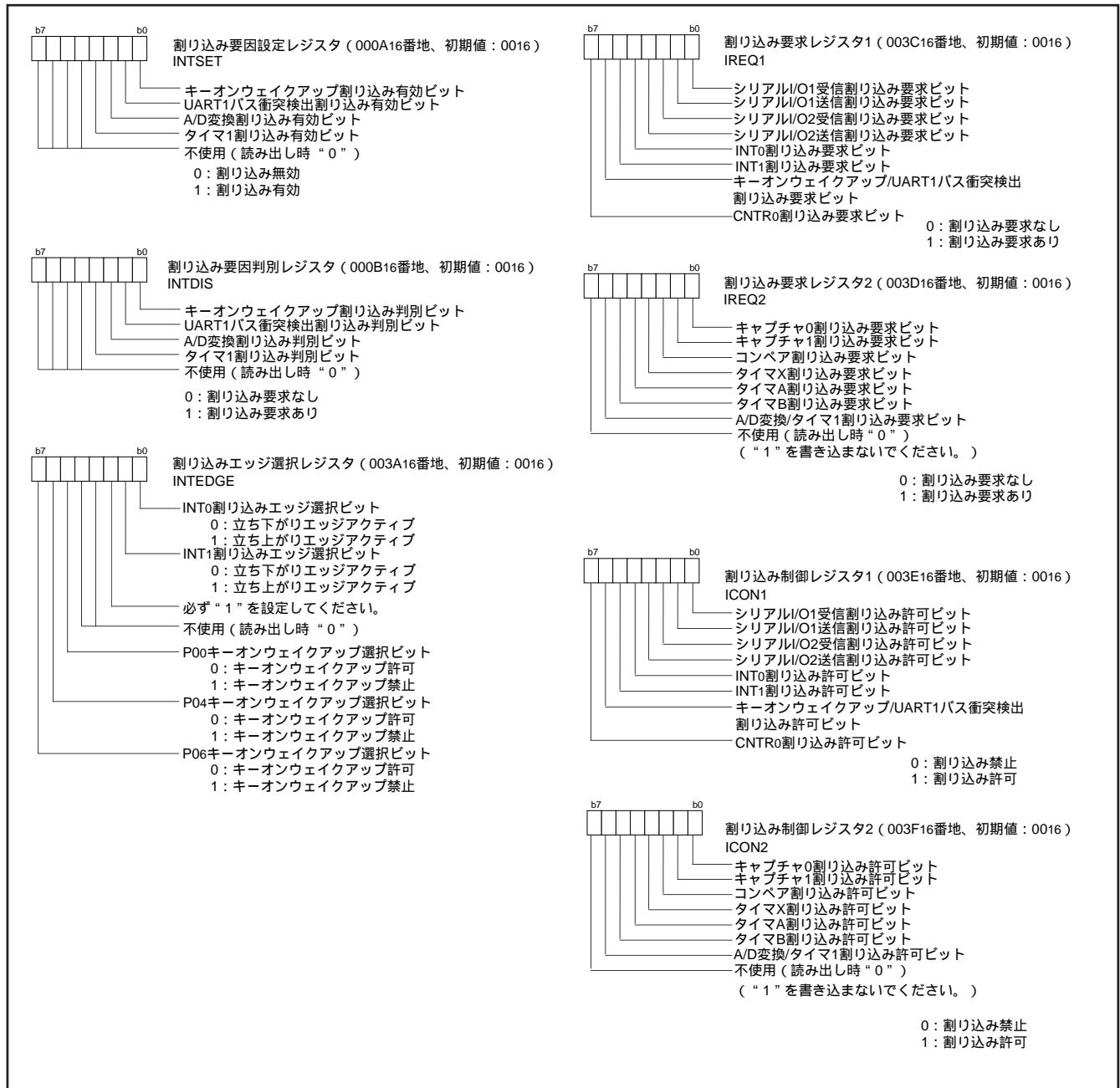
図 21 . 割り込み関係レジスタの構成
