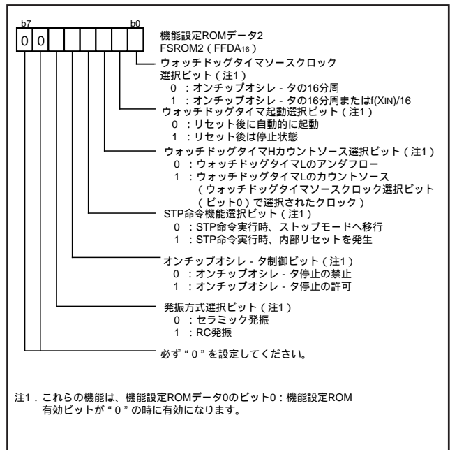
図 88 . 機能設定 ROM データ 2 の構成
