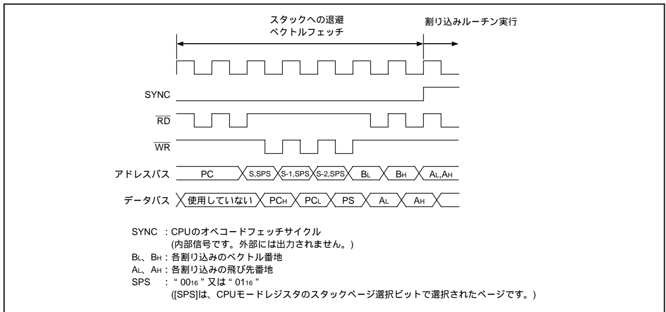
図23. 割り込みシーケンス
