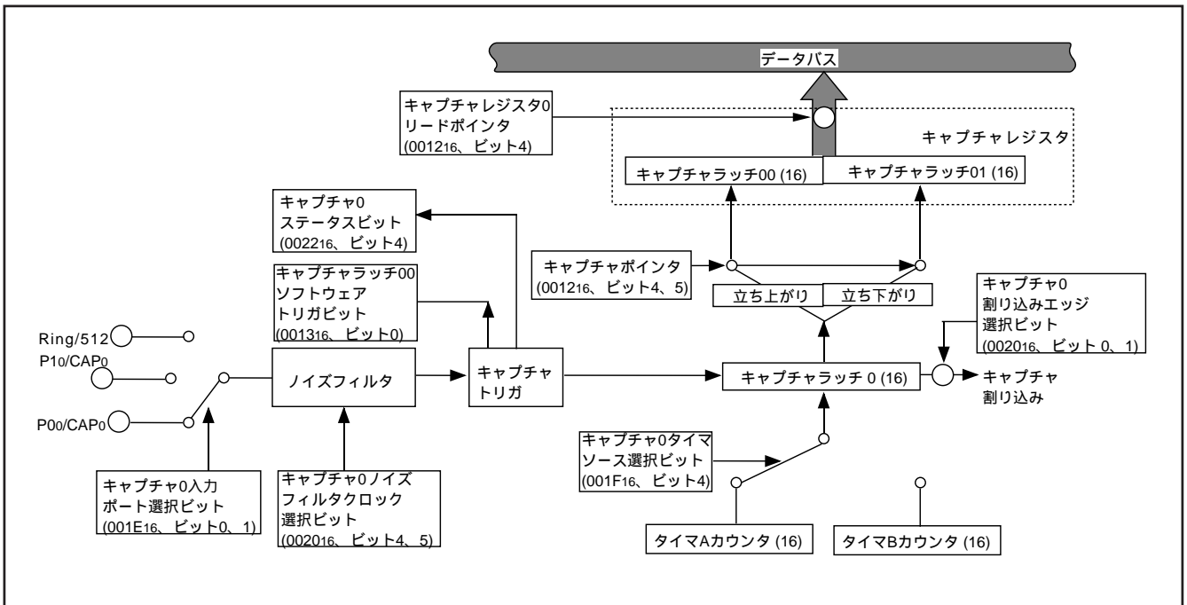
図 49 . キャプチャチャンネル0のブロック図
