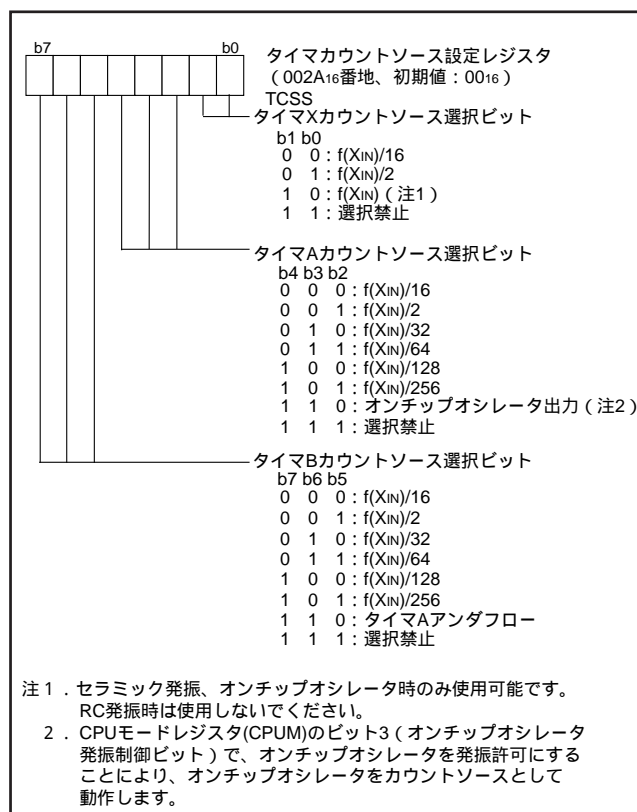
図 27. タイマカウントソース設定レジスタの構成
