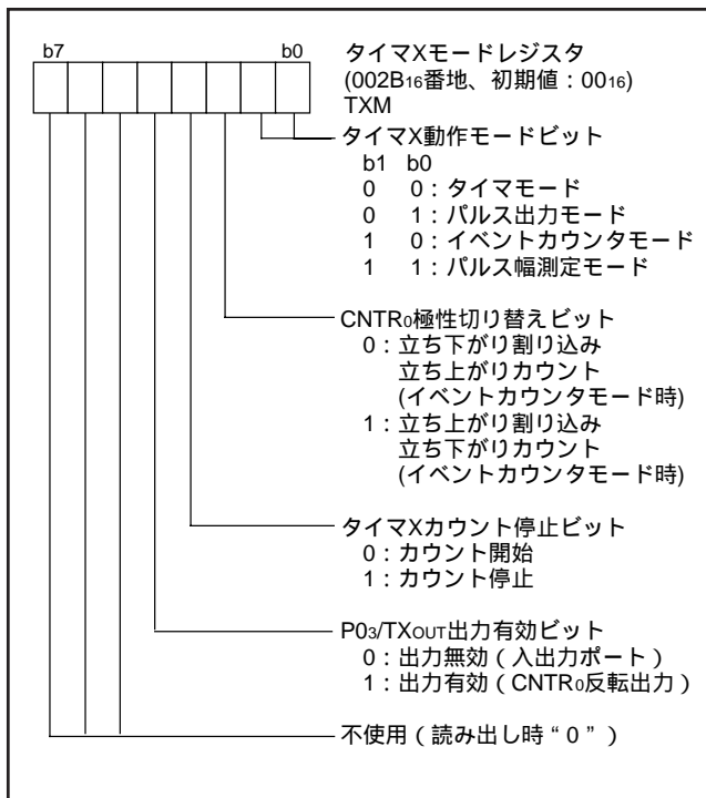
図 26. タイマXモードレジスタの構成
