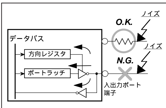
図102. 入出力ポート処理
