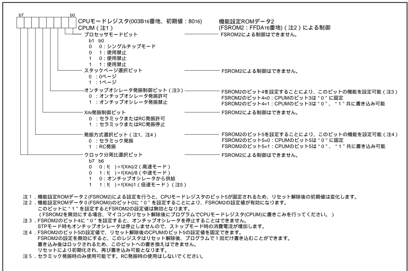
図 11 . CPUモードレジスタの構成
