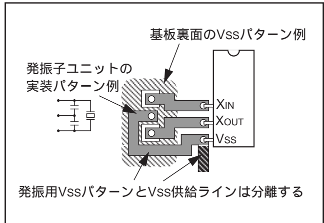
図101．発振子の裏面のVssパターン
