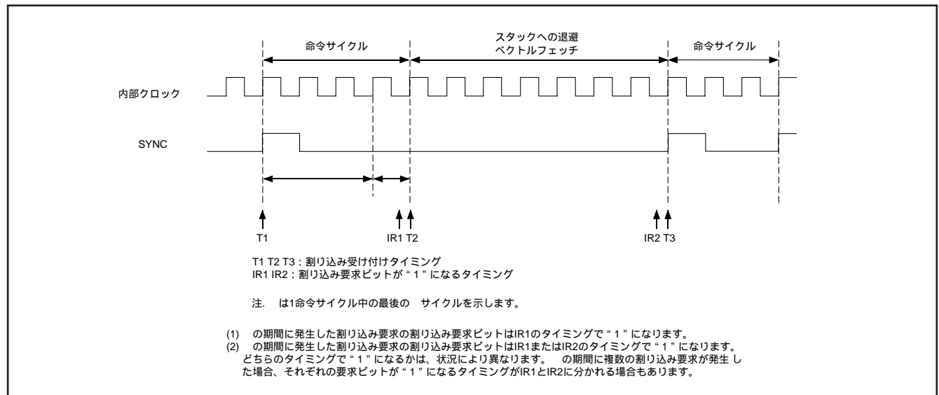
図24. 割り込み要求発生と割り込み要求ビット、割り込み要求受け付けのタイミング
