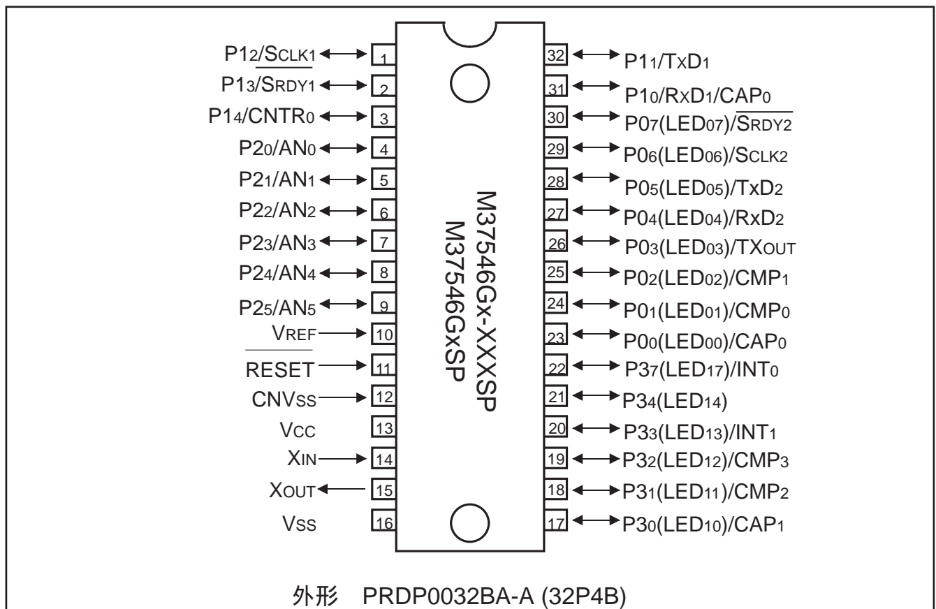
図 2. ピン接続図 (PRDP0032BA-A パッケージ)
