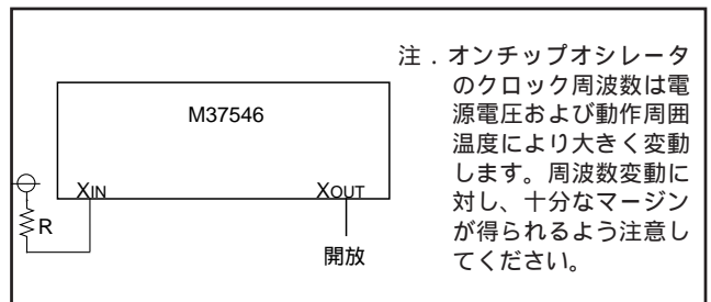
図74．オンチップオシレータ動作時のXIN、XOUT端子の処理
