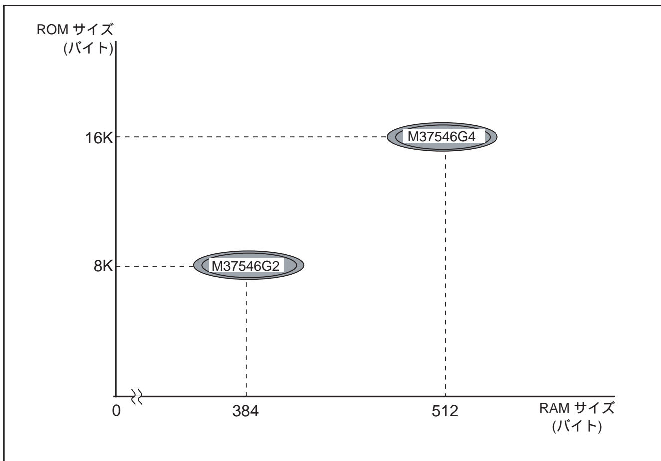
図7. ROM及びRAM展開計画
