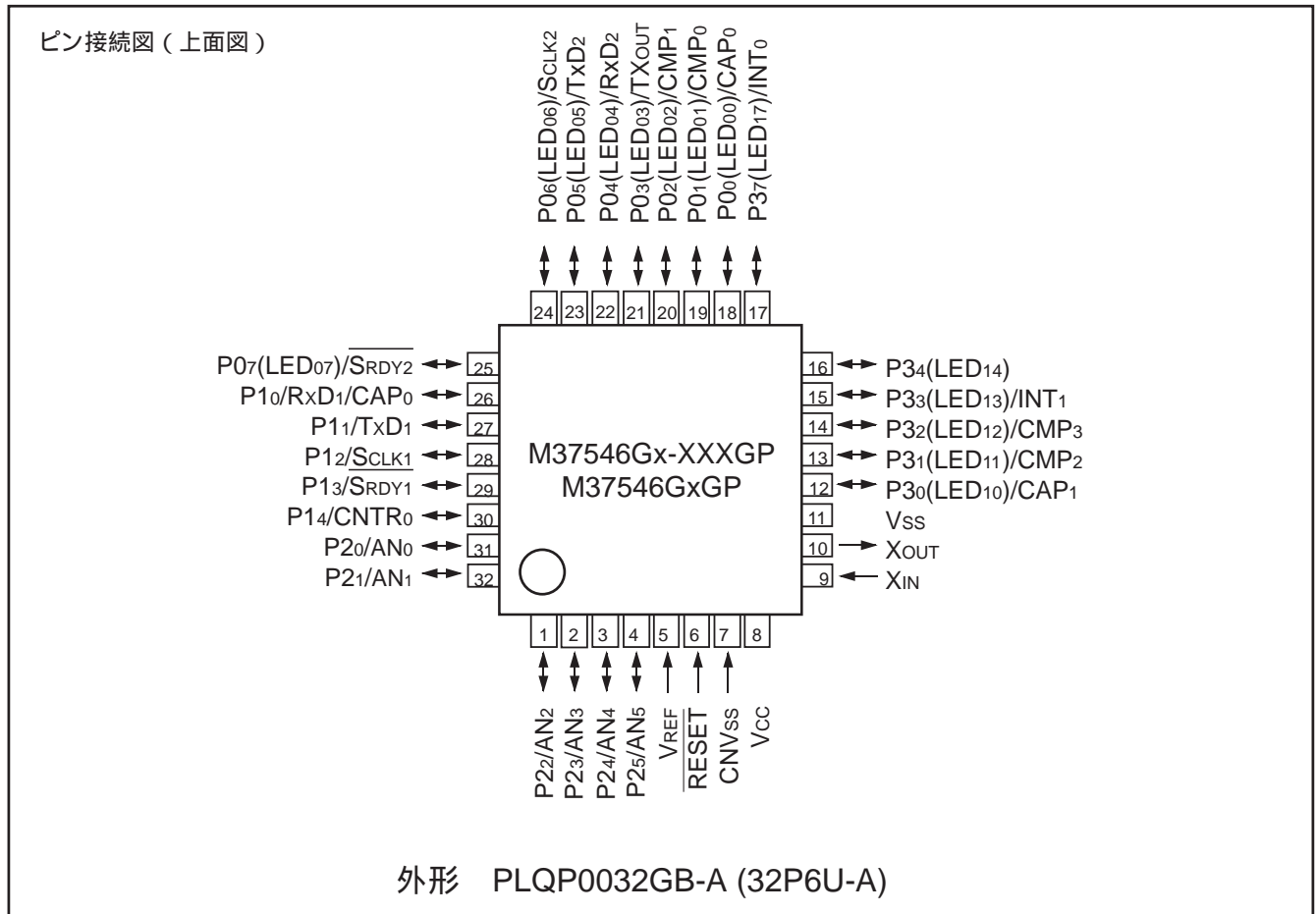
図 1. ピン接続図 (PLQP0032GB-A パッケージ)
