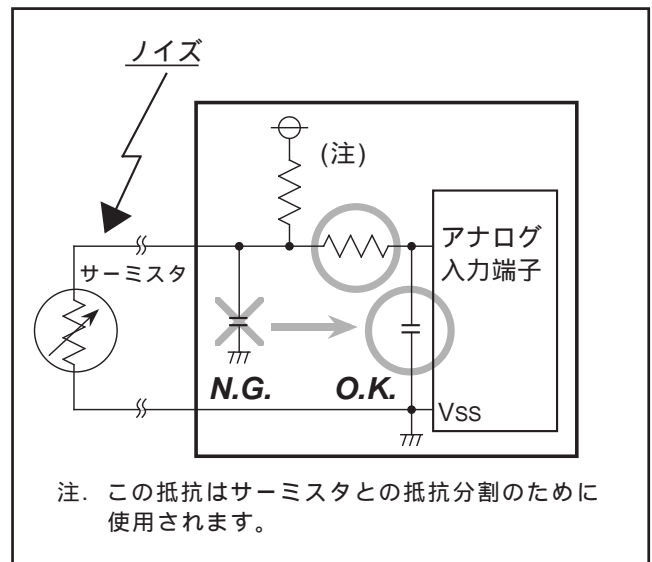
図99 . アナログ信号線と抵抗及びコンデンサ
