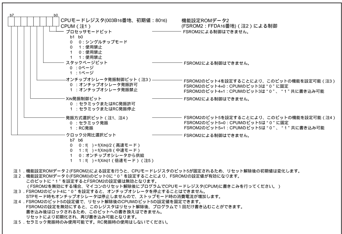
図 78 . CPU モードレジスタの構成
