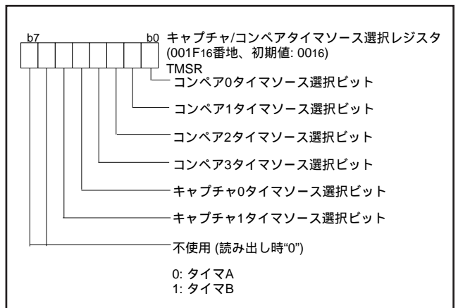
図 35 . キャプチャ/コンペアタイマソース選択レジスタの構成
