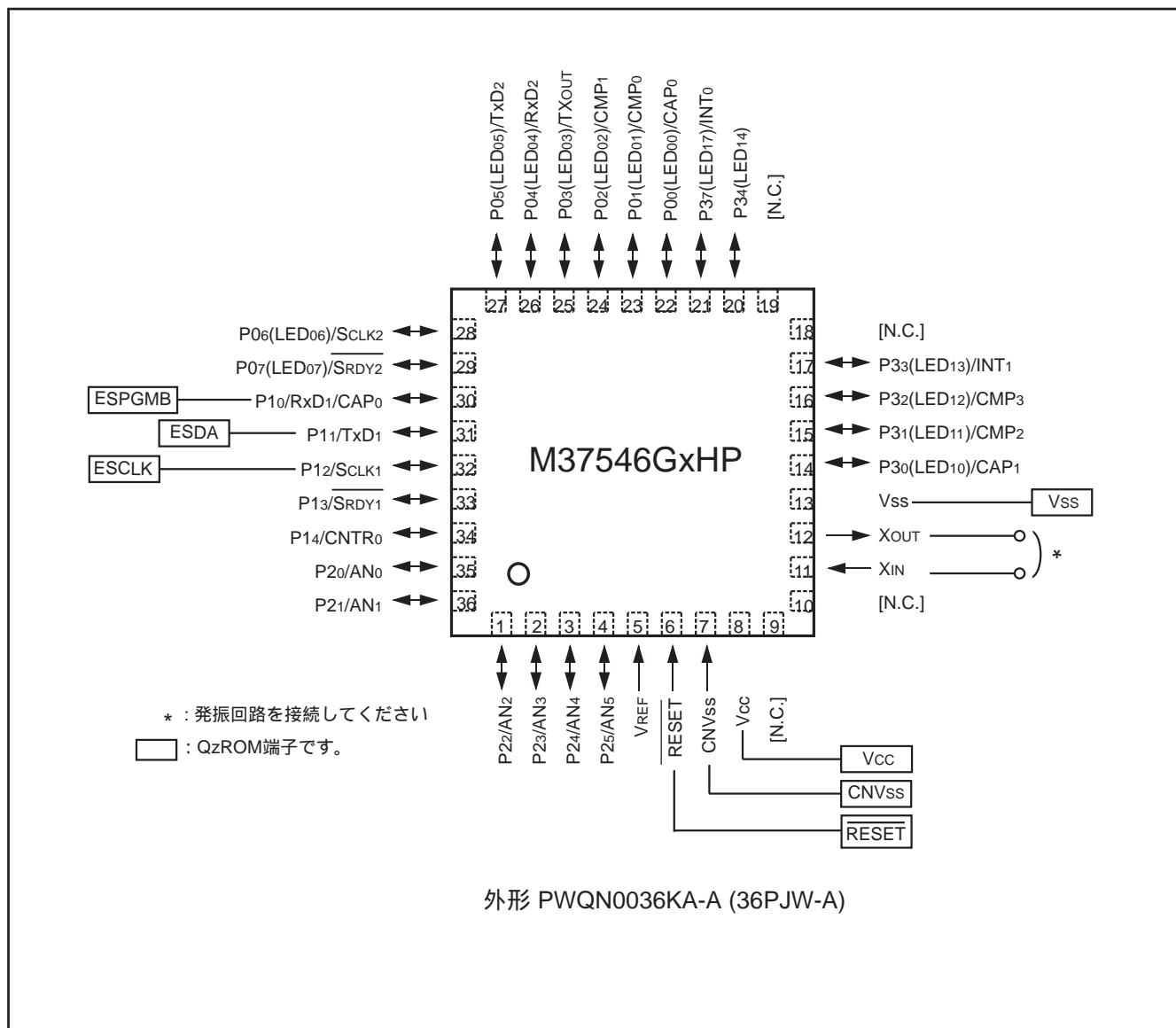
図 91 . 端子結線図(M37546GxHP)
