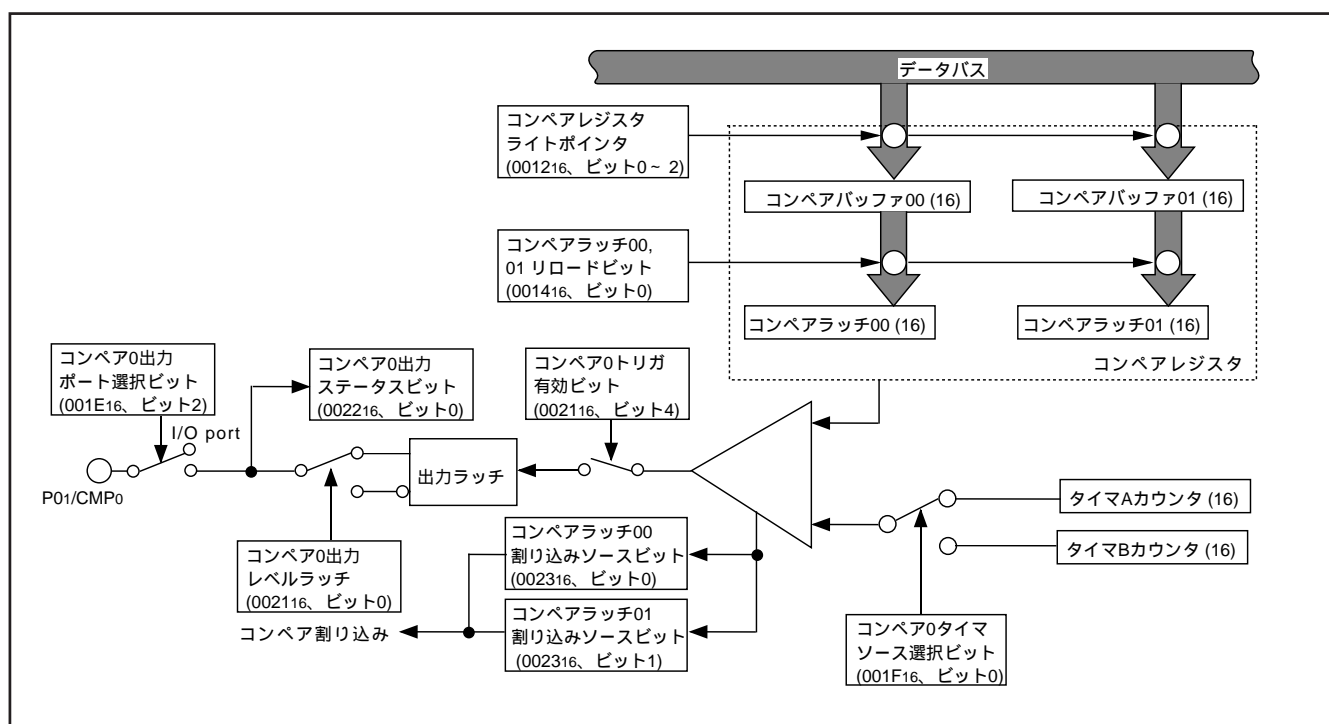
図 40 . コンペアチャンネル0のブロック図
