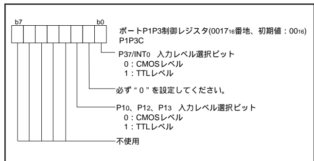
図 16 . ポート P1P3 制御レジスタの構成
