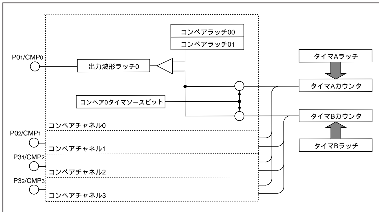
図 39 . コンペア出力回路のブロック図
