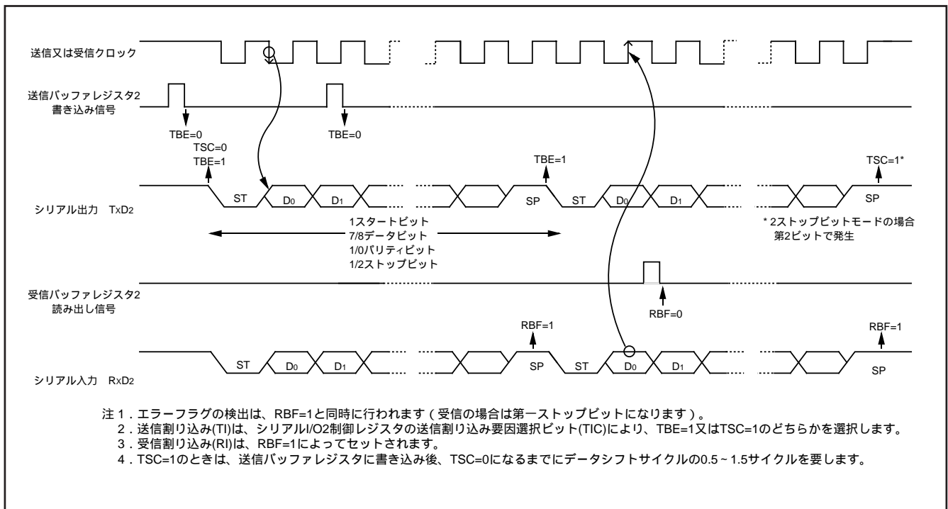
図 63 . UART 形シリアル I/O2 動作図
