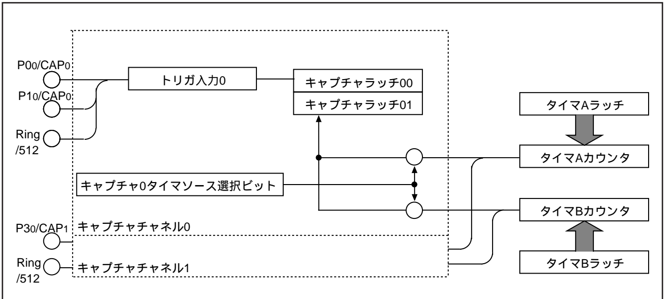
図 48 . キャプチャ入力回路のブロック図
