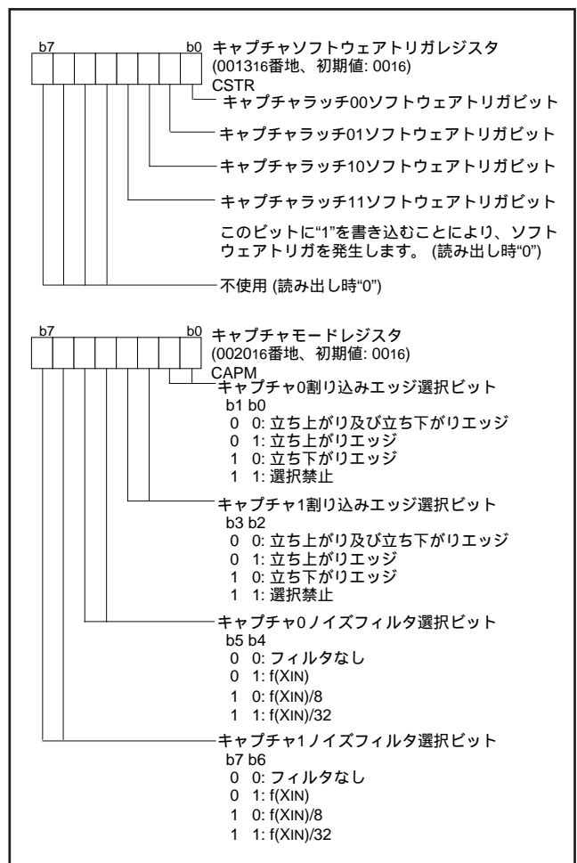
図47. キャプチャソフトウェアトリガレジスタ/キャプチャモードレジスタの構成
