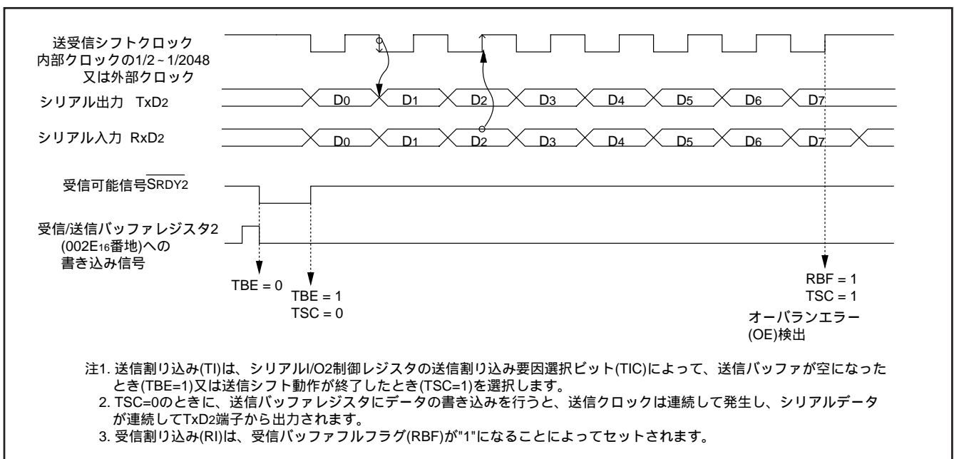
図 61 . クロック同期形シリアルI/O2 動作図
