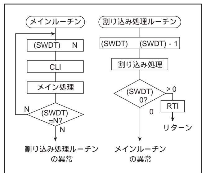
図103. ソフトウェアによるウォッチドッグタイマ
