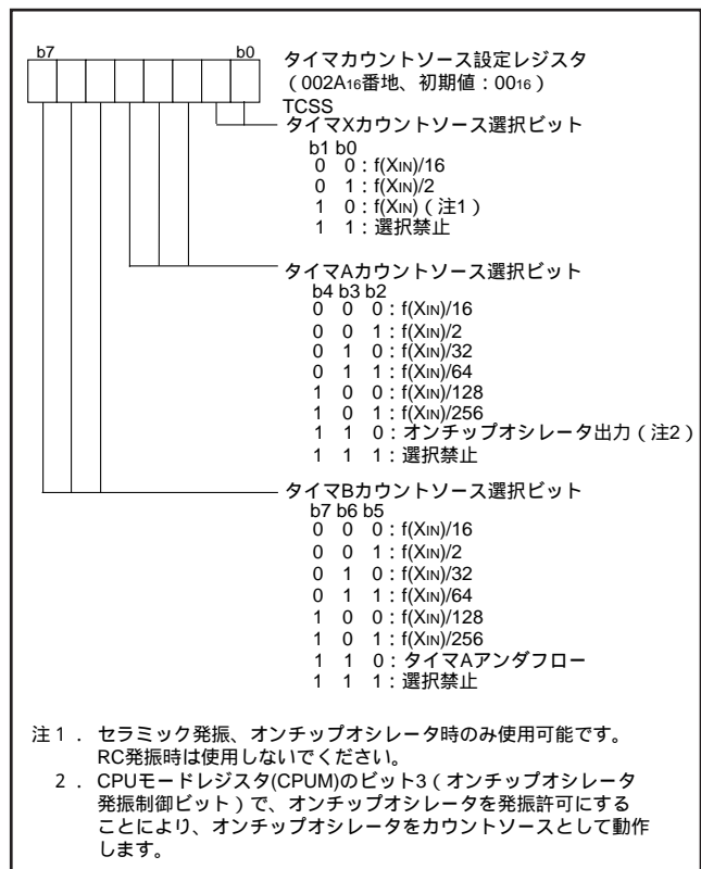
図 30 . タイマカウントソース設定レジスタの構成
