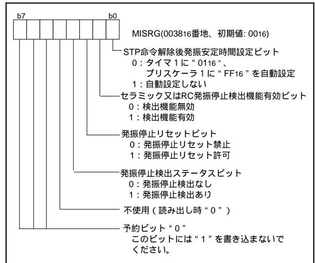
図83 . MISRG の構成
