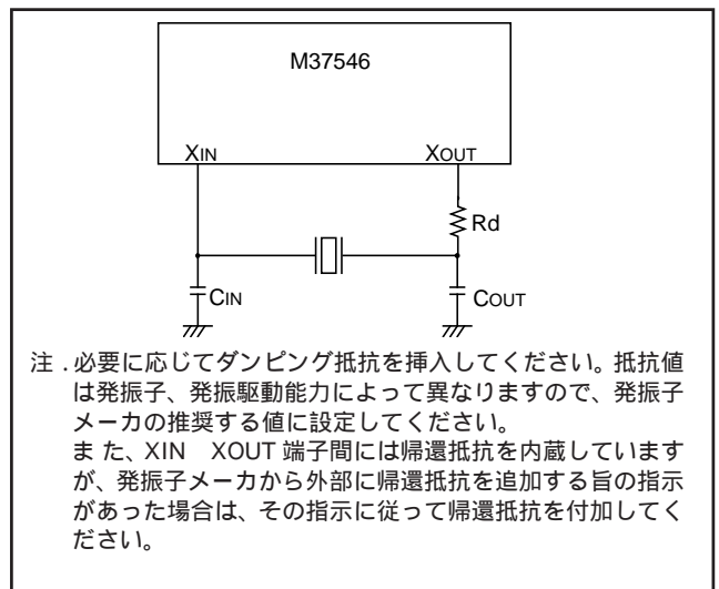
図75．セラミック共振子外付け回路
