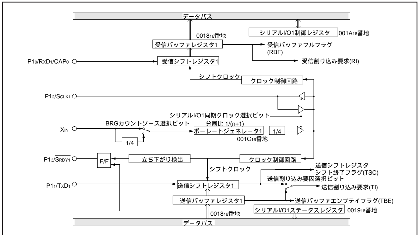
図 52 . クロック同期形シリアルI/O1 ブロック図
