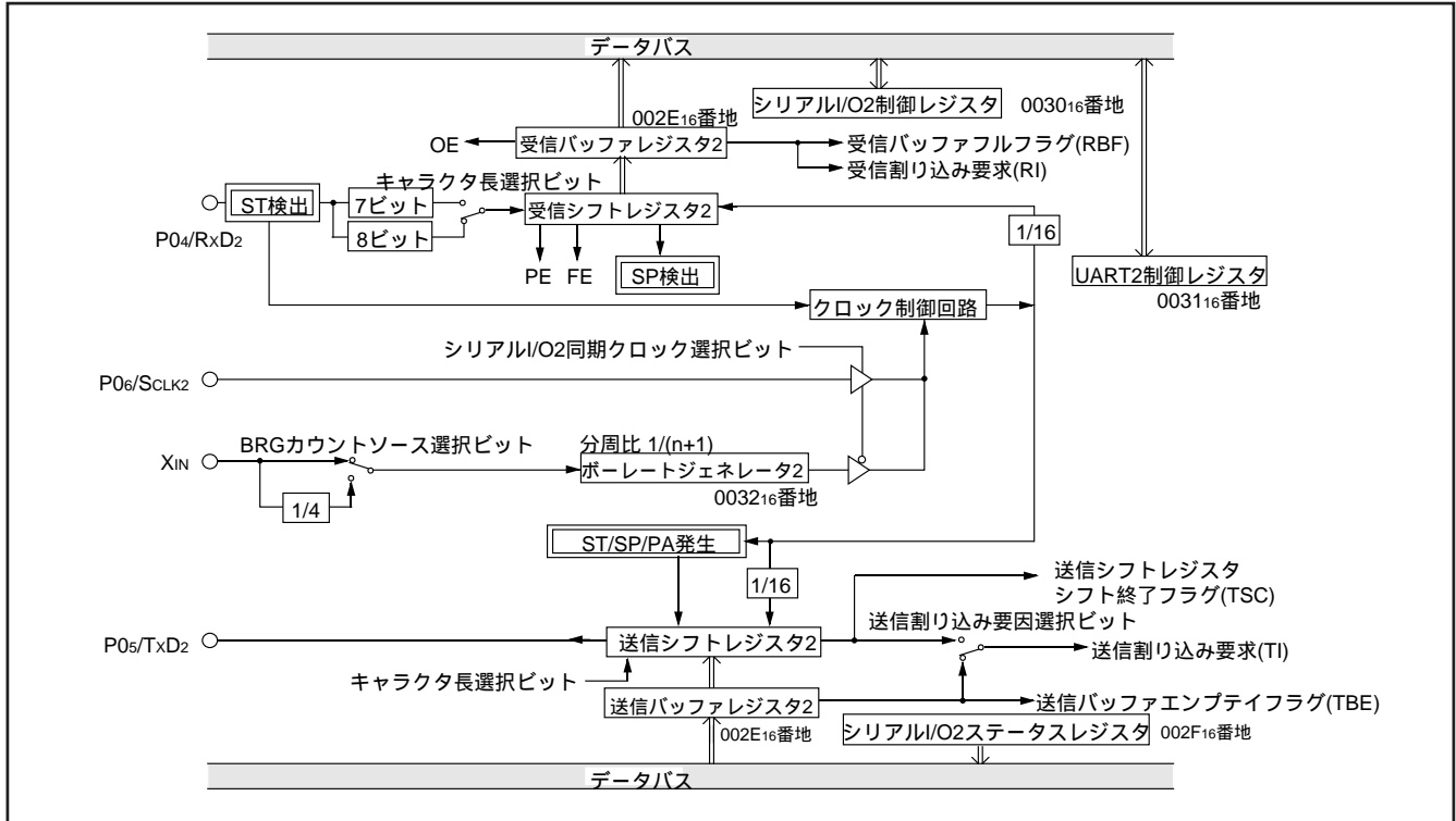
図 62 . UART 形シリアル I/O2 ブロック図
