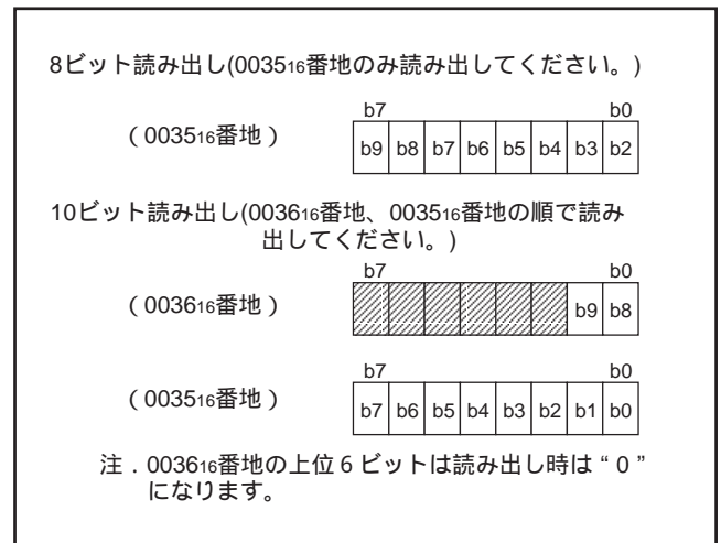
図 66 . A/D 変換レジスタの構成
