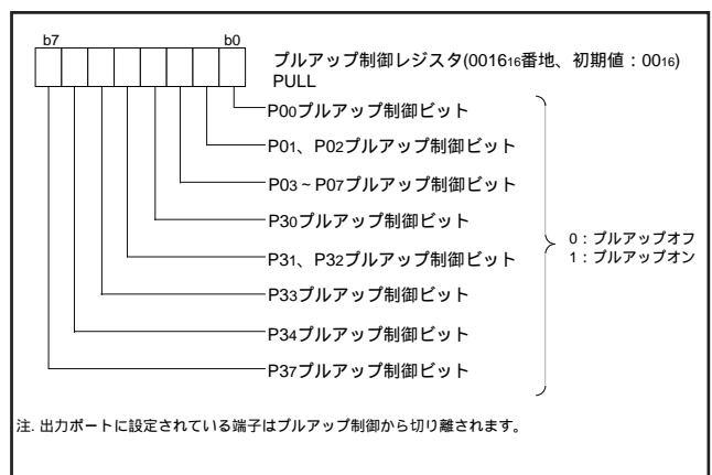
図 15 . プルアップ制御レジスタの構成
