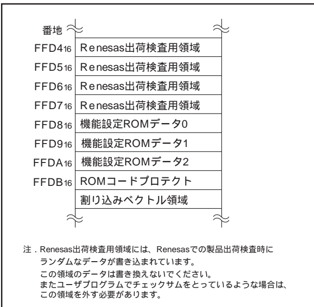
図 85 . 機能設定 ROM 領域の配置
