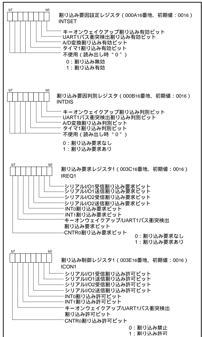
図 57 . バス衝突検出関連レジスタ
