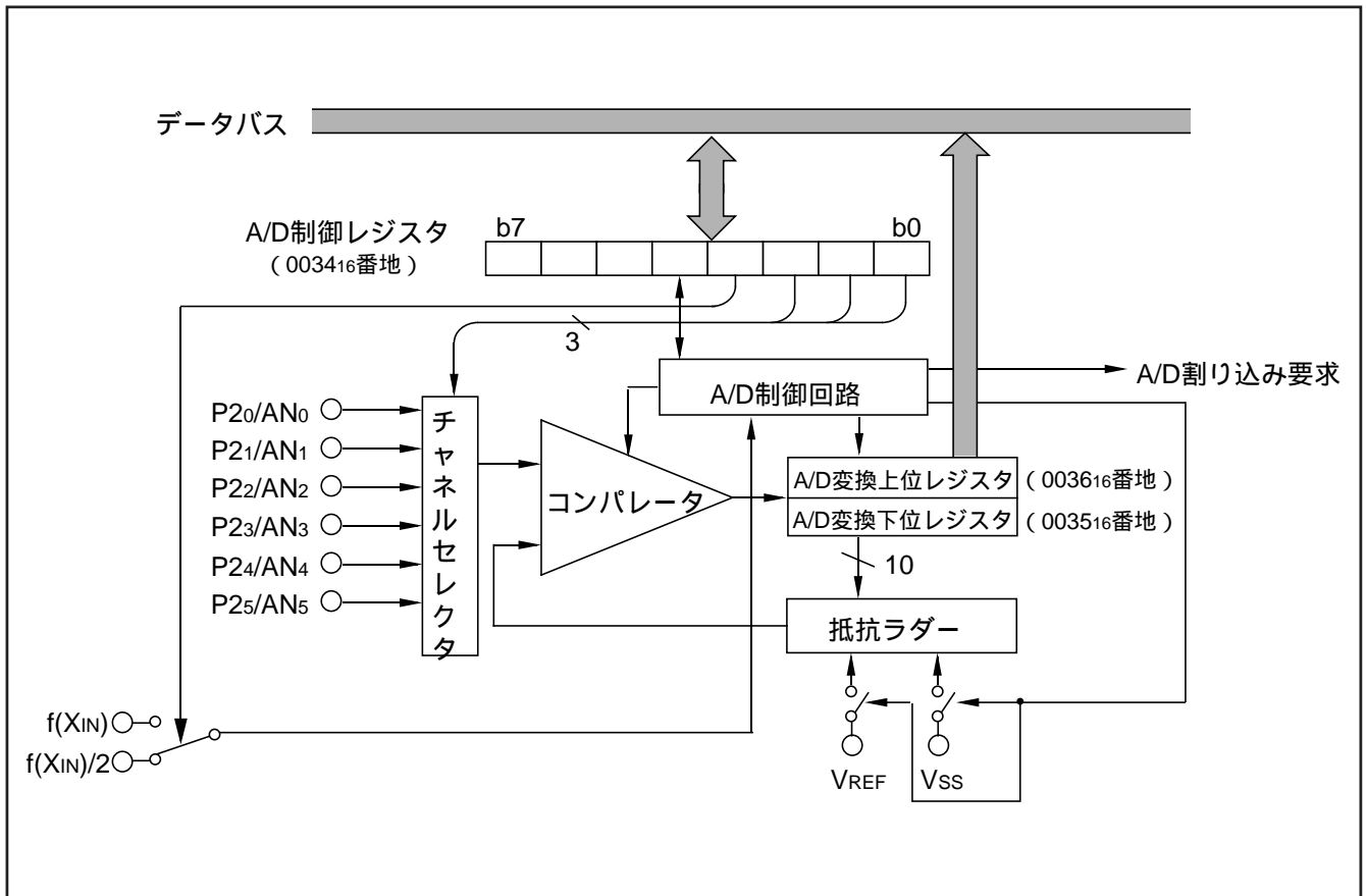
図 67 . A/D コンバータブロック図
