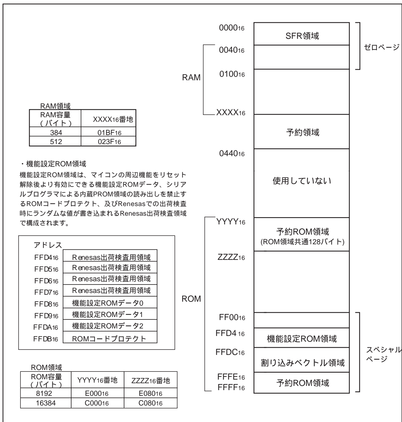
図 10 . メモリ配置図
