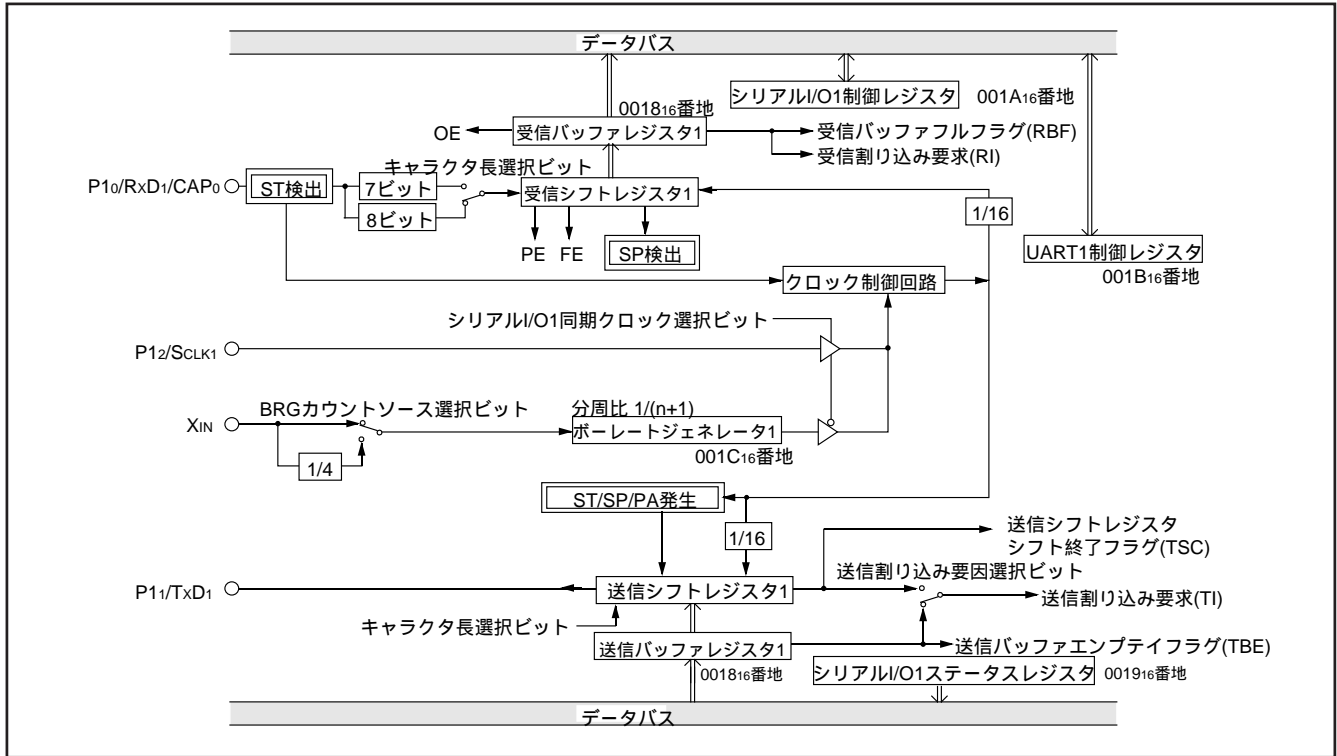
図 54 . UART 形シリアル I/O1 ブロック図
