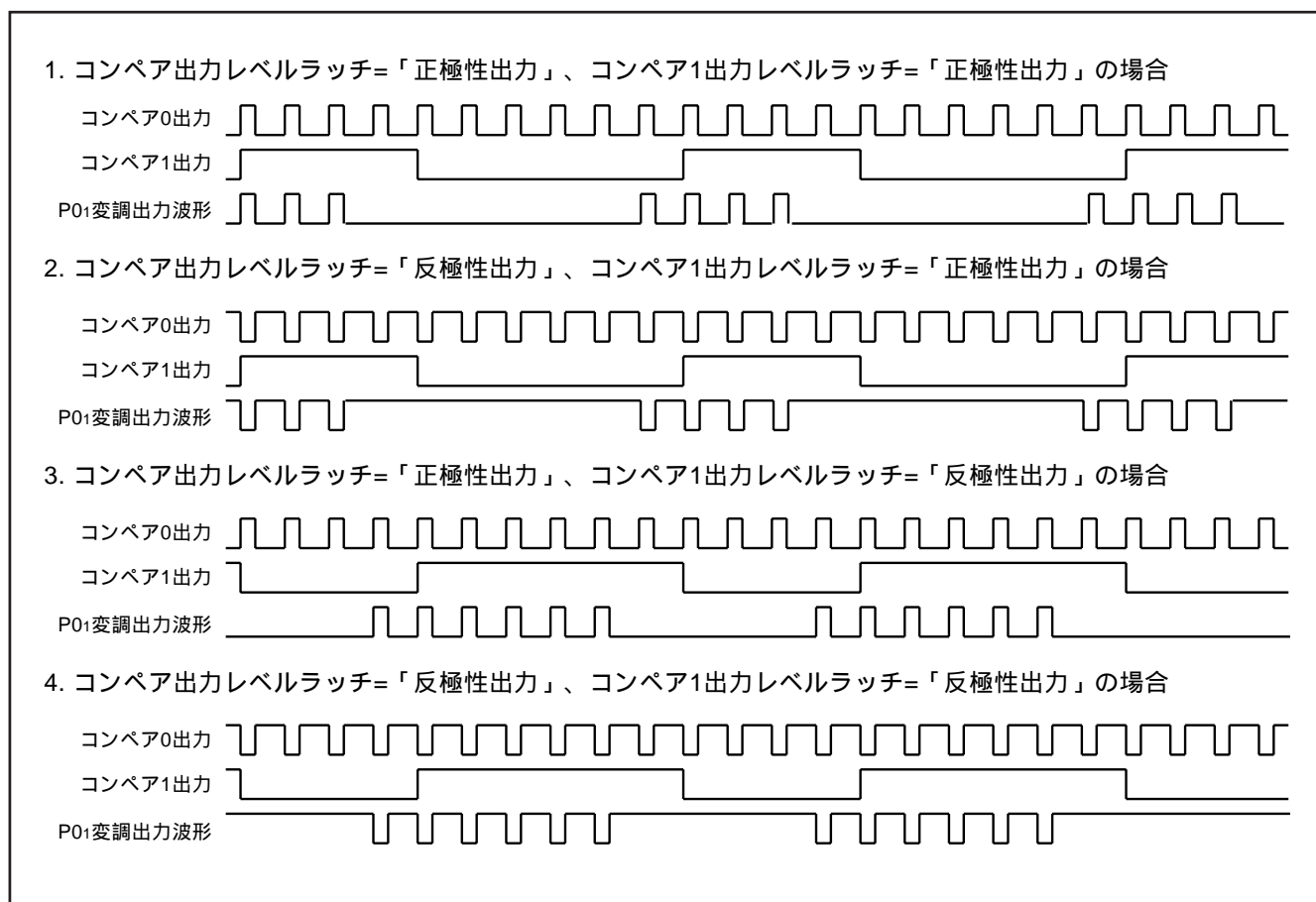
図 45 . コンペア出力波形図 (コンペア 0、1 変調出力モード : 出力レベルラッチの設定による出力波形の変化)
