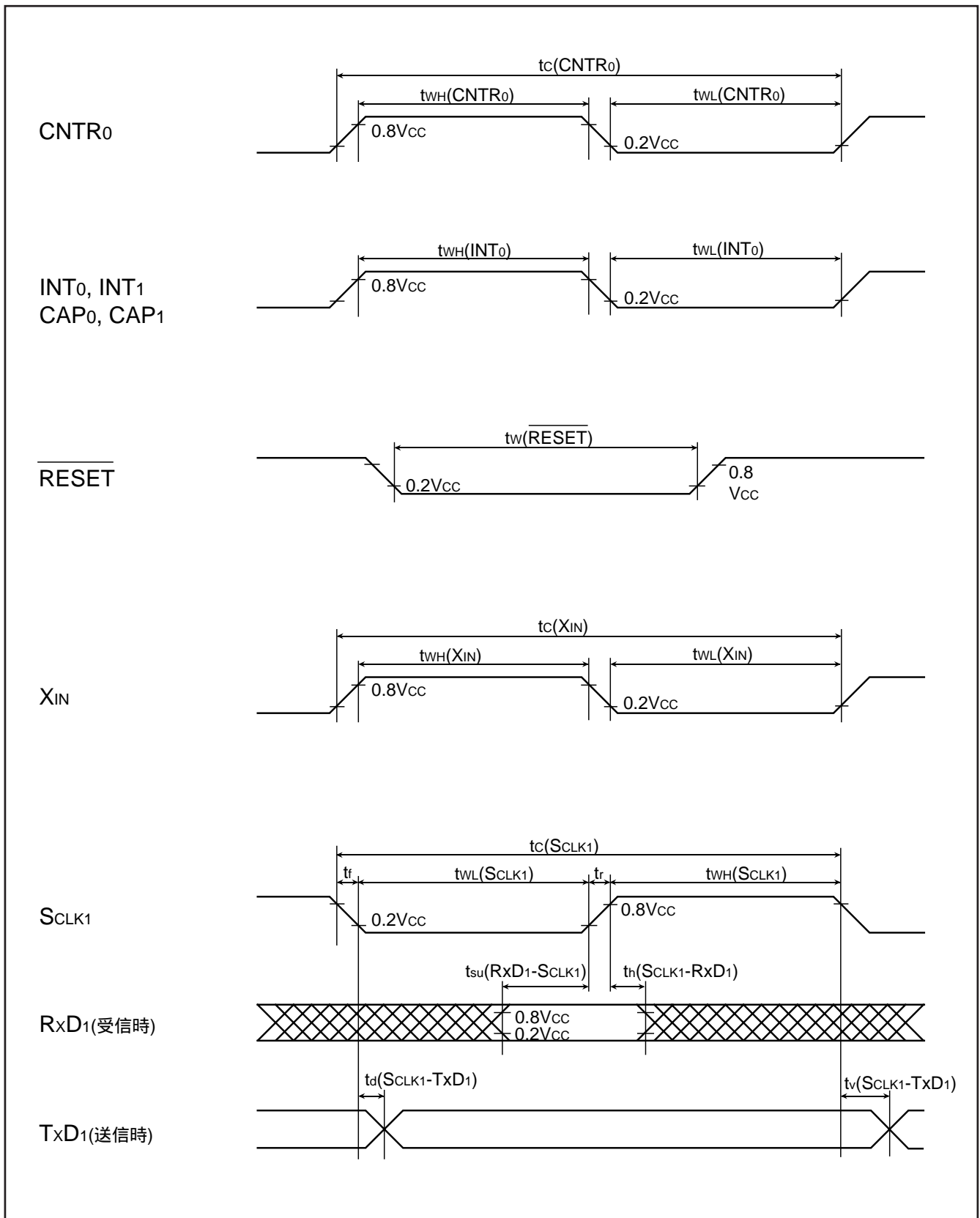
図 107 . タイミング図
