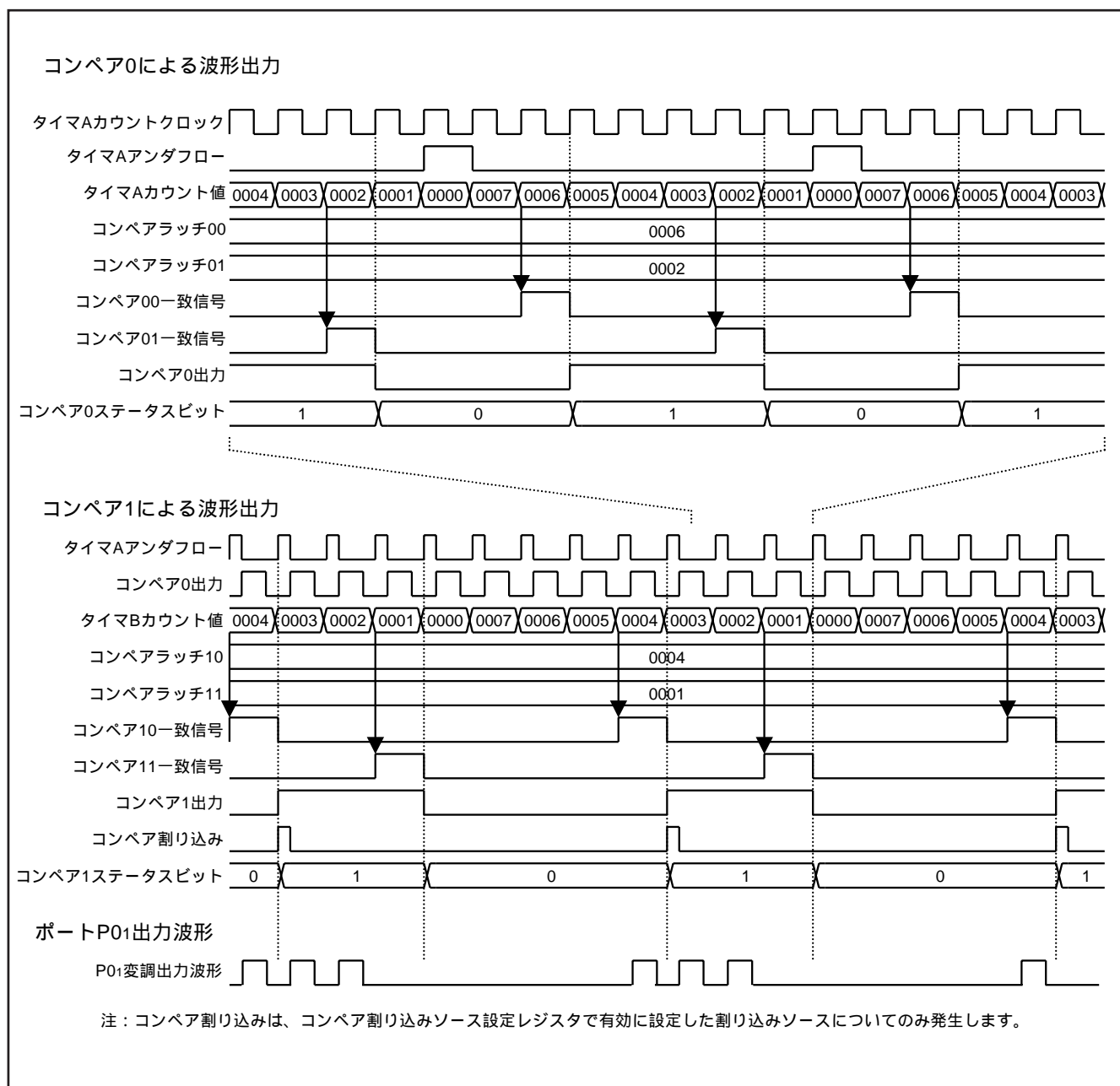
図44 . コンペア出力波形図(コンペア0、1変調出力モード)
