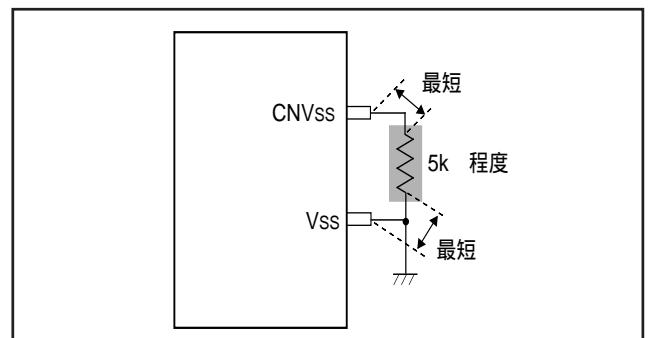
図 97 . QzROM 版の CNVss 端子の配線
