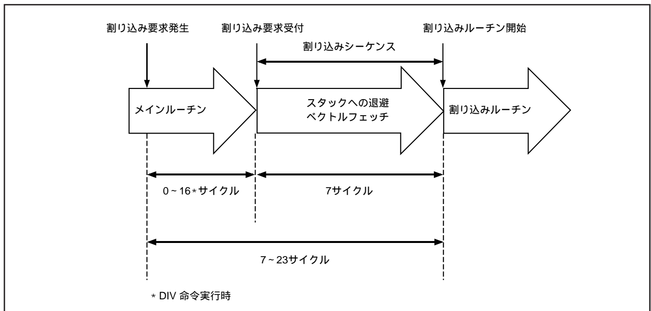
図22．割り込み処理ルーチンを実行するまでの時間
