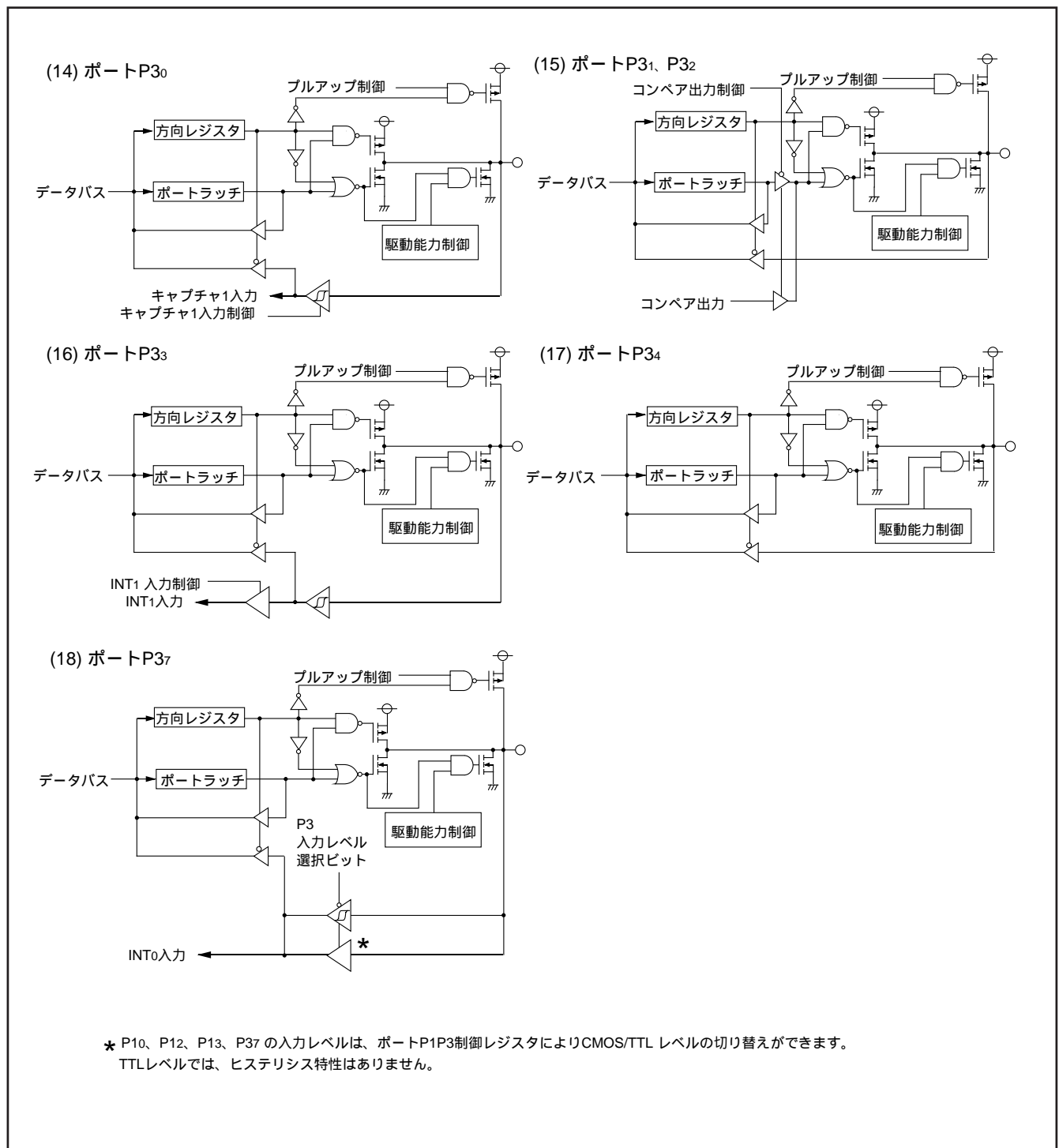
図 19 . ポートのブロック図 ( 3 )
