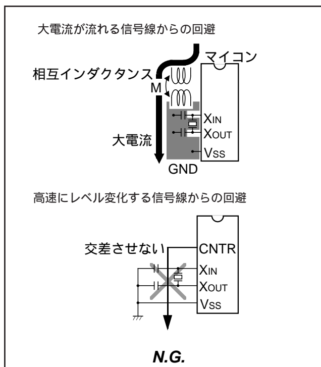
図100．大電流が流れる信号線の配線/高速にレベル変化する信号線の配線
