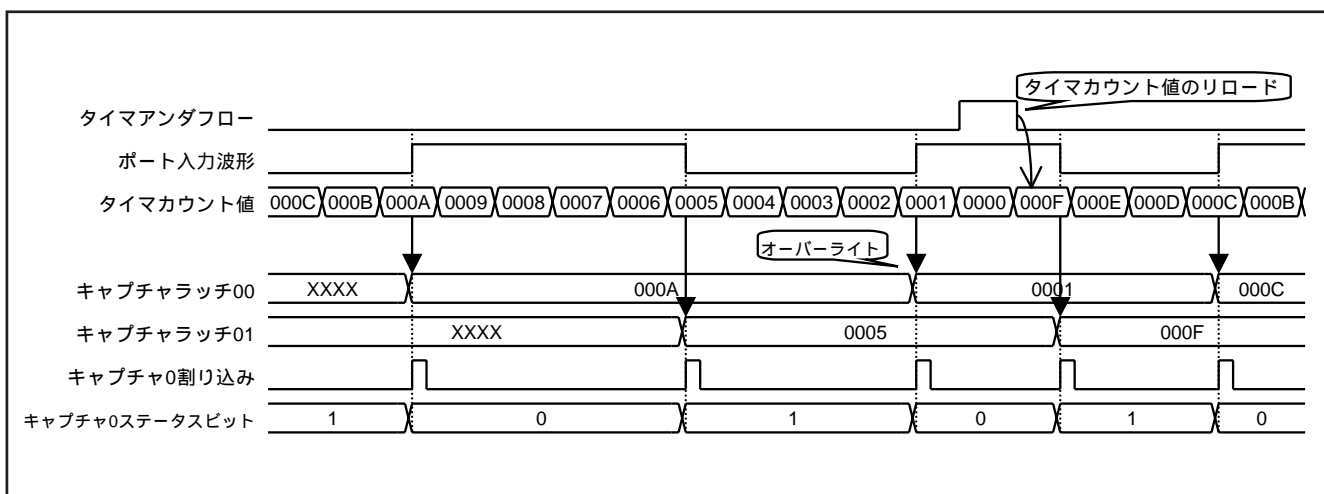
図 51 . キャプチャ入力波形図 (キャプチャ0 割り込みエッジ選択ビット : 立ち上がり及び立ち下がり選択時)
