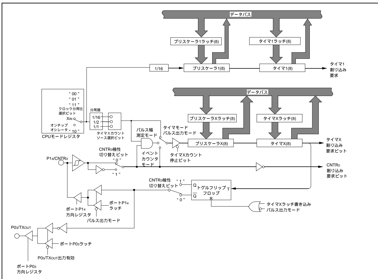
図 28. タイマ1及び、タイマXのブロック図
