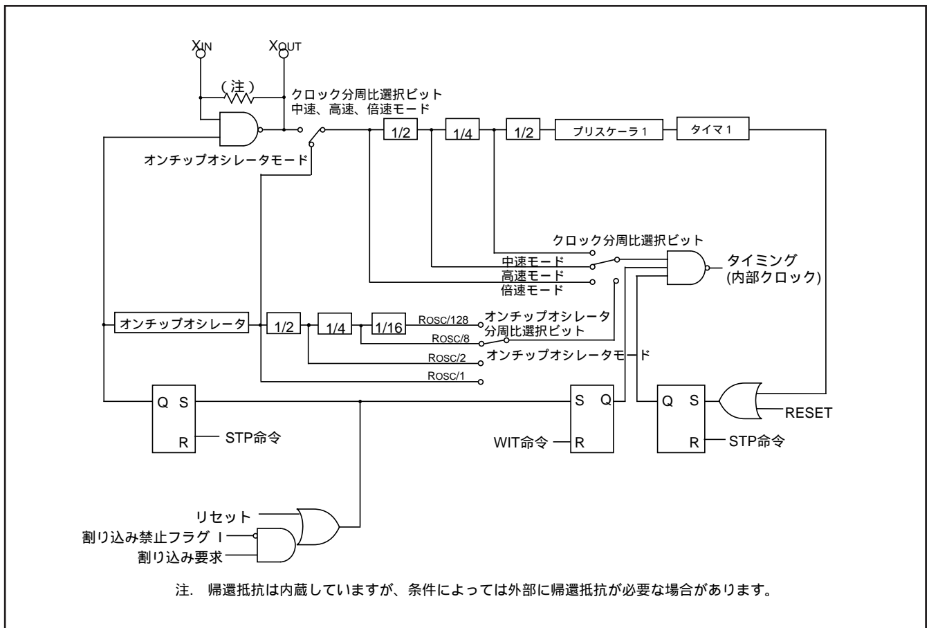
図 80 . システムクロック発生回路ブロック図 (セラミック発振時)
