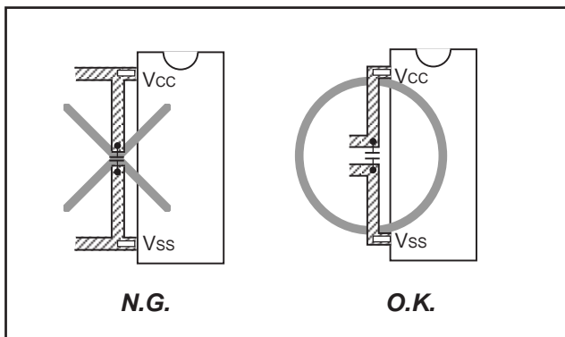
図98 . VSS - VCCライン間のバイパスコンデンサ
