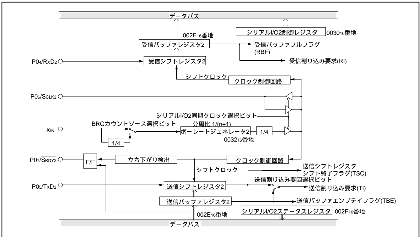
図 60 . クロック同期形シリアルI/O2 ブロック図
