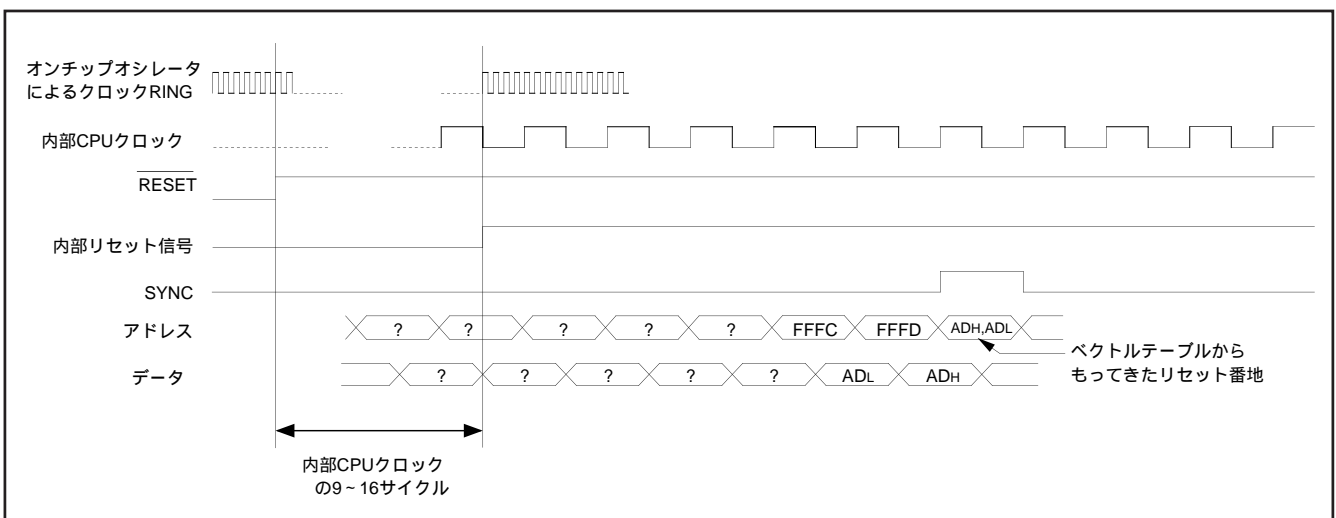
図72. リセット時のタイミング図
