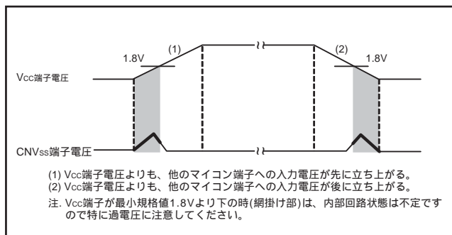
図 104. タイミング図 (太線の区間が該当)
