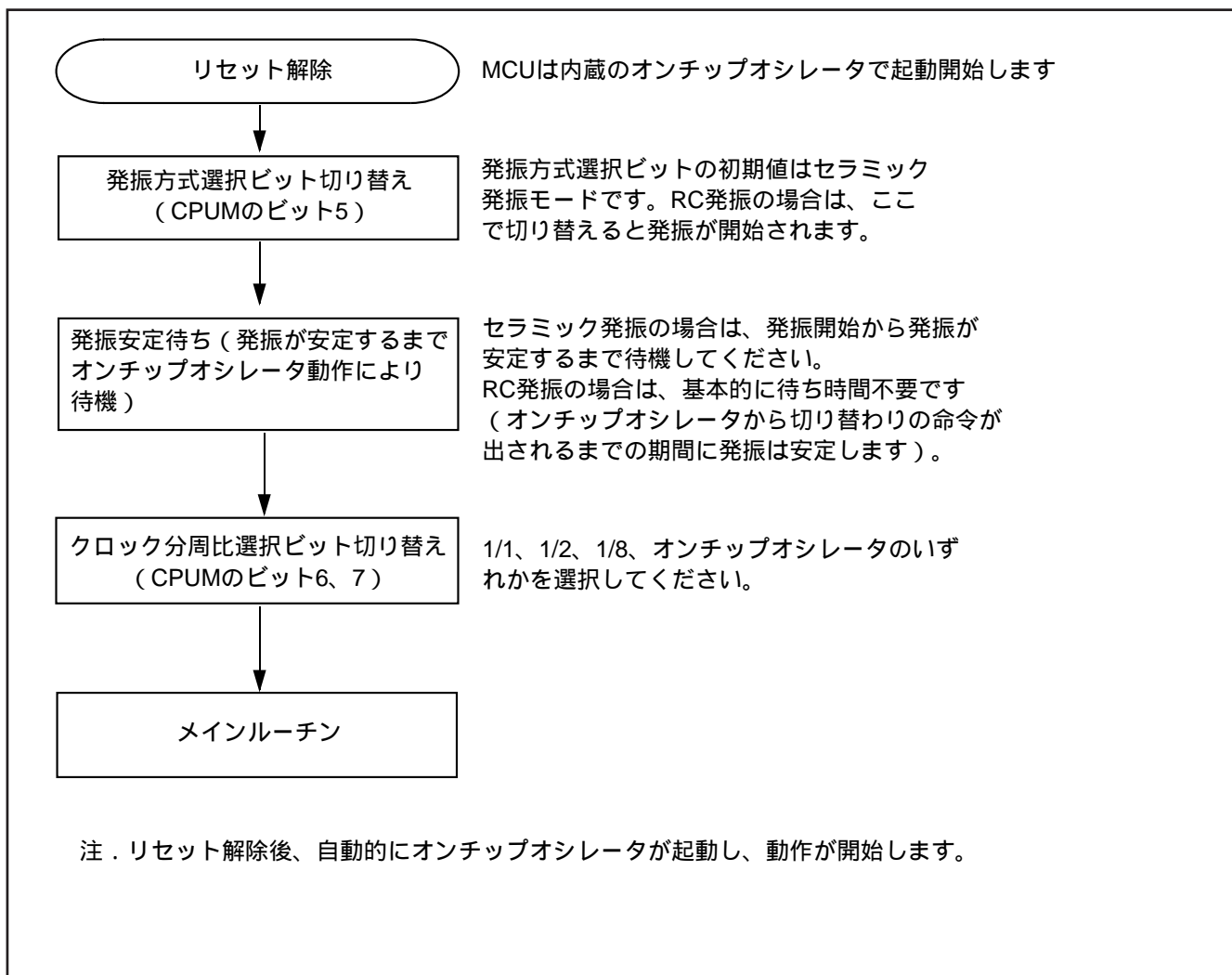
図 12 . CPU モードレジスタの切り替え手順
