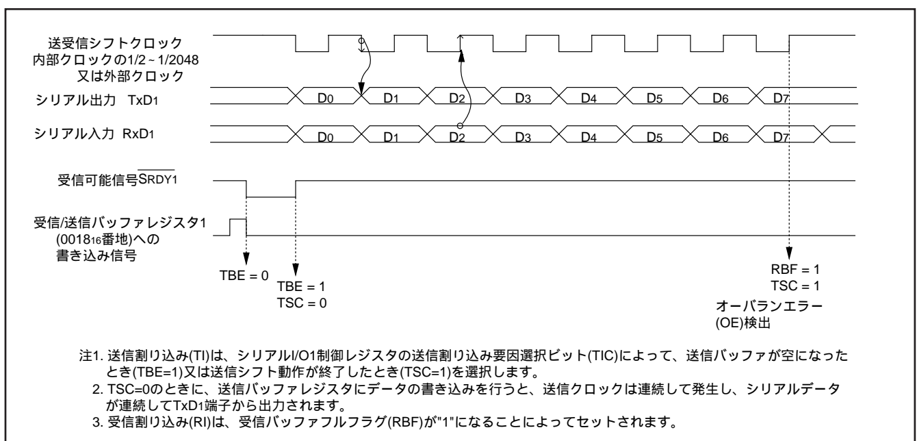
図 53 . クロック同期形シリアルI/O1 動作図
