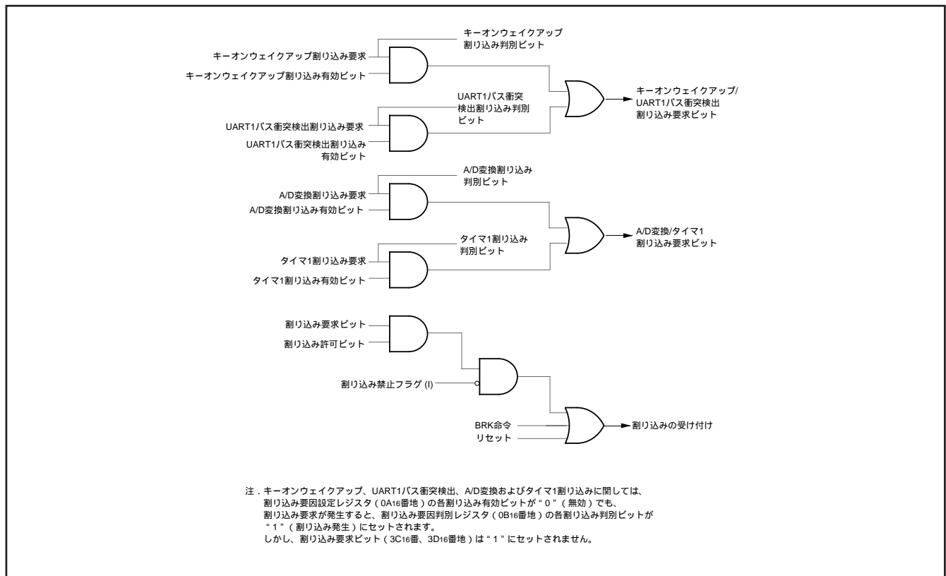
図20. 割り込み制御図
