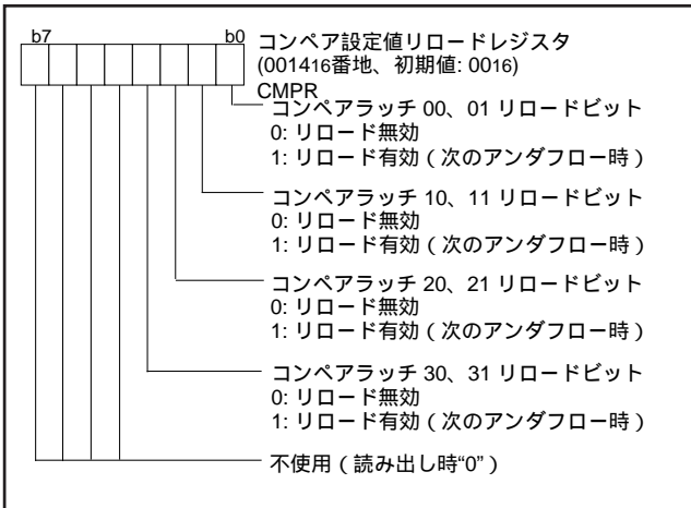
図 33 . コンペア設定値リロードレジスタの構成
