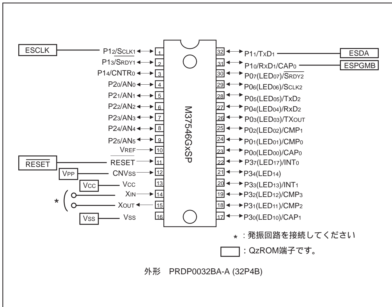
図 90 . 端子結線図(M37546GxSP)
