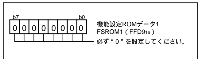
図 87 . 機能設定 ROM データ 1 の構成
