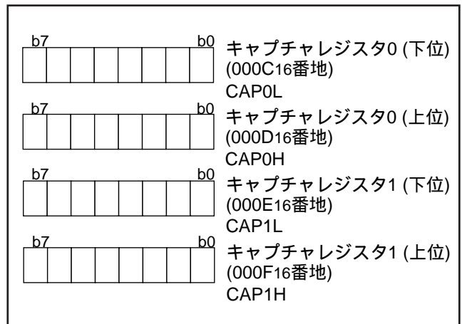
図46. キャプチャレジスタの構成
