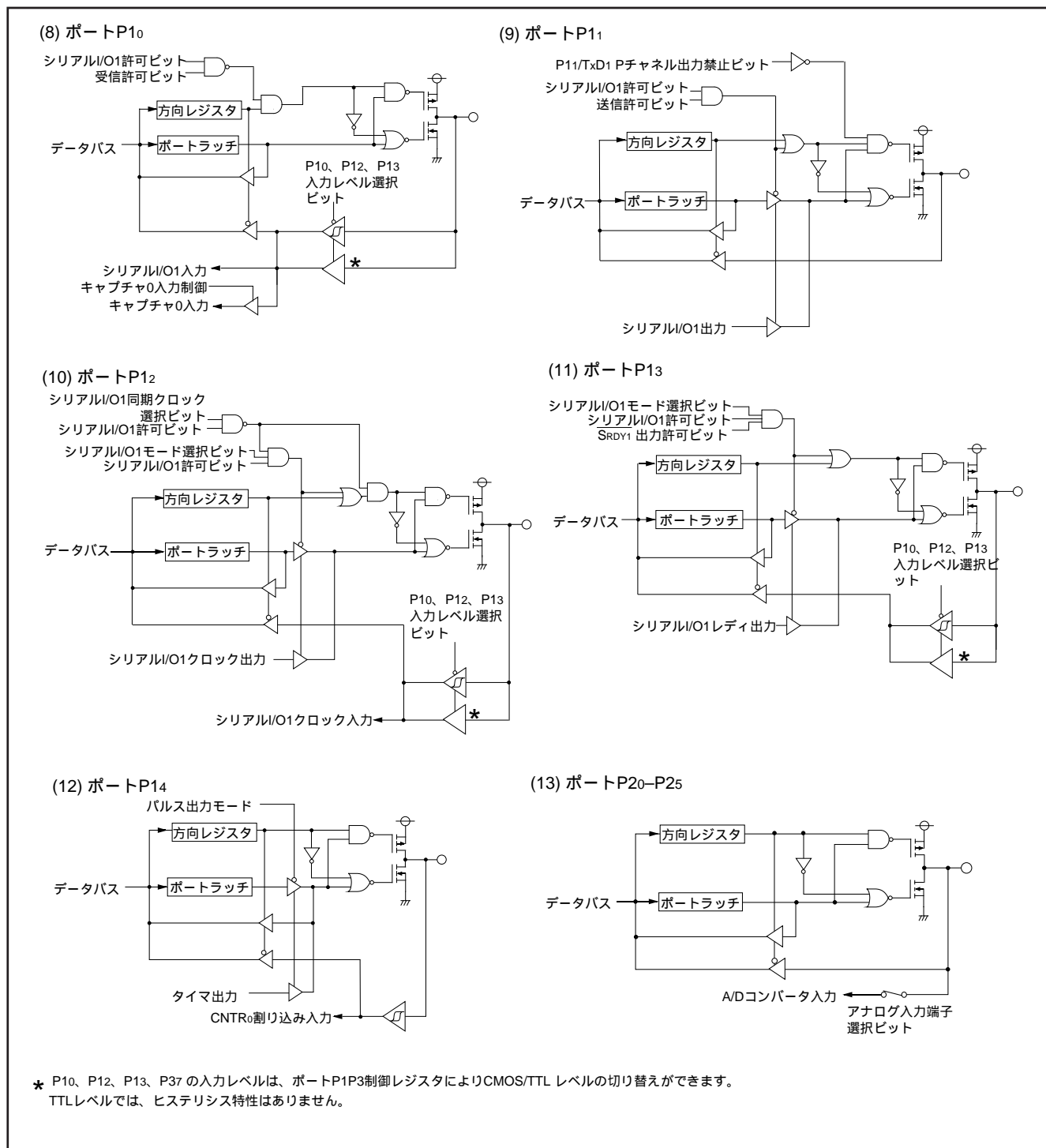
図 18 . ポートのブロック図 ( 2 )
