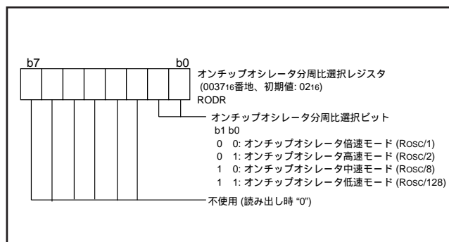
図 79 . オンチップオシレータ分周比選択レジスタの構成
