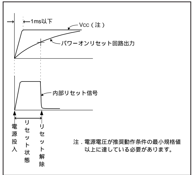
図70. パワーオンリセット回路動作波形図
