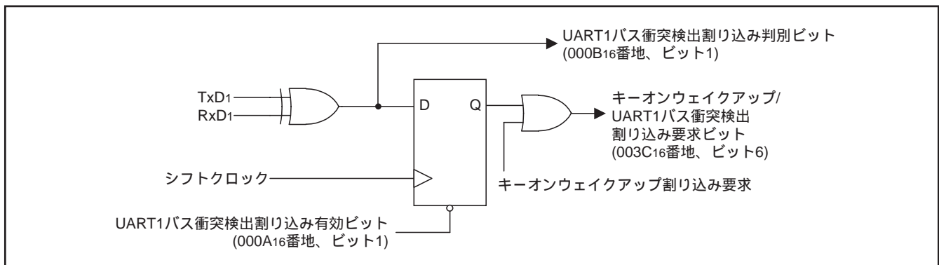
図 58 . バス衝突検出割り込み回路のブロック図
