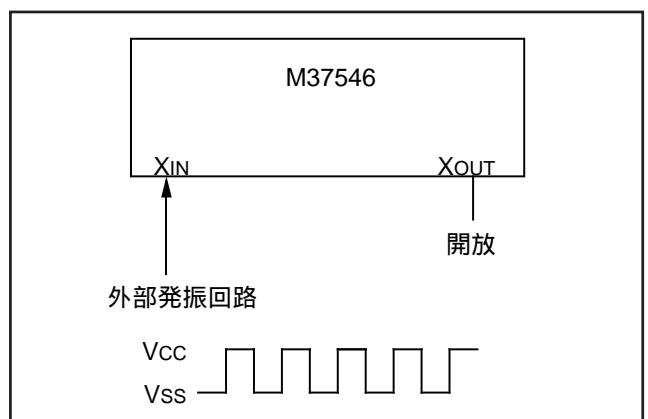
図77．外部クロック入力回路
