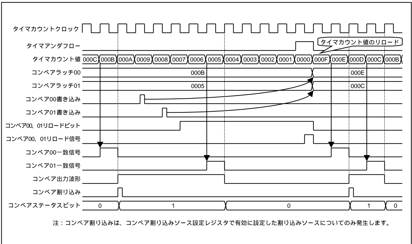
図 43 . コンペア出力波形図 (コンペアレジスタの書き込み時)
