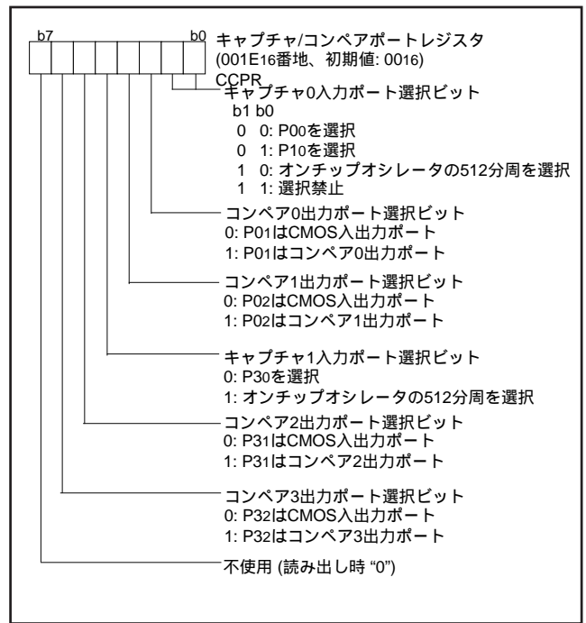
図 34 . キャプチャ/コンペアポートレジスタの構成
