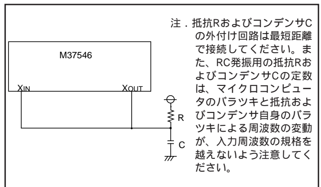
図76．RC外付け発振回路
