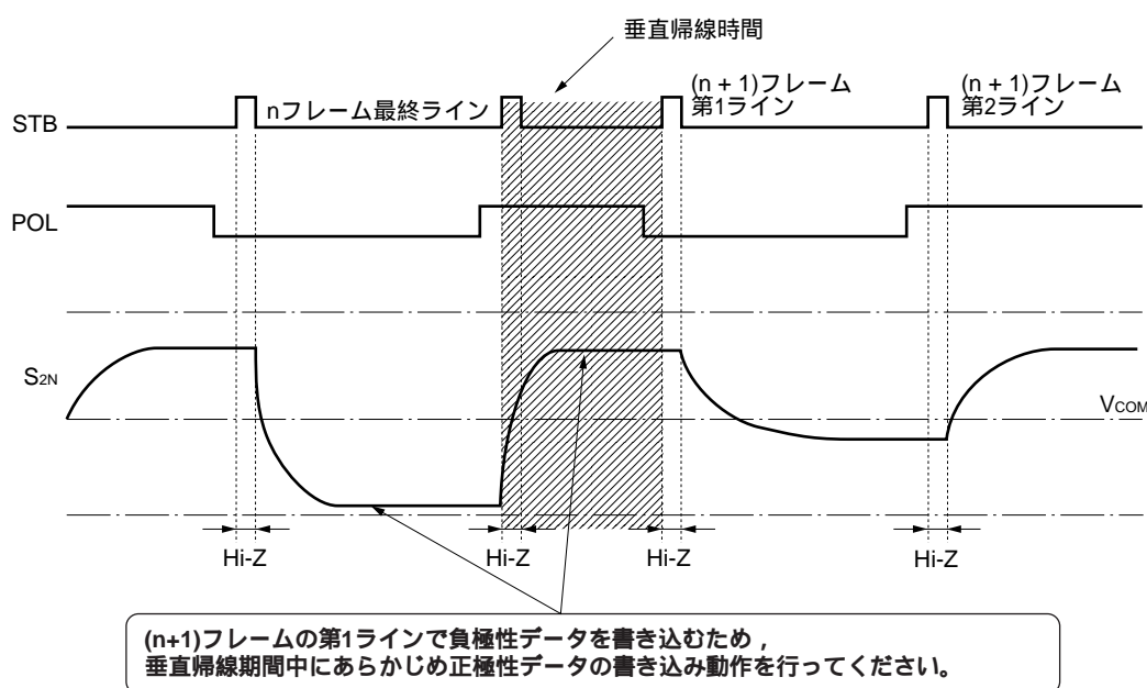
図8-2 極性反転と書き込み動作
