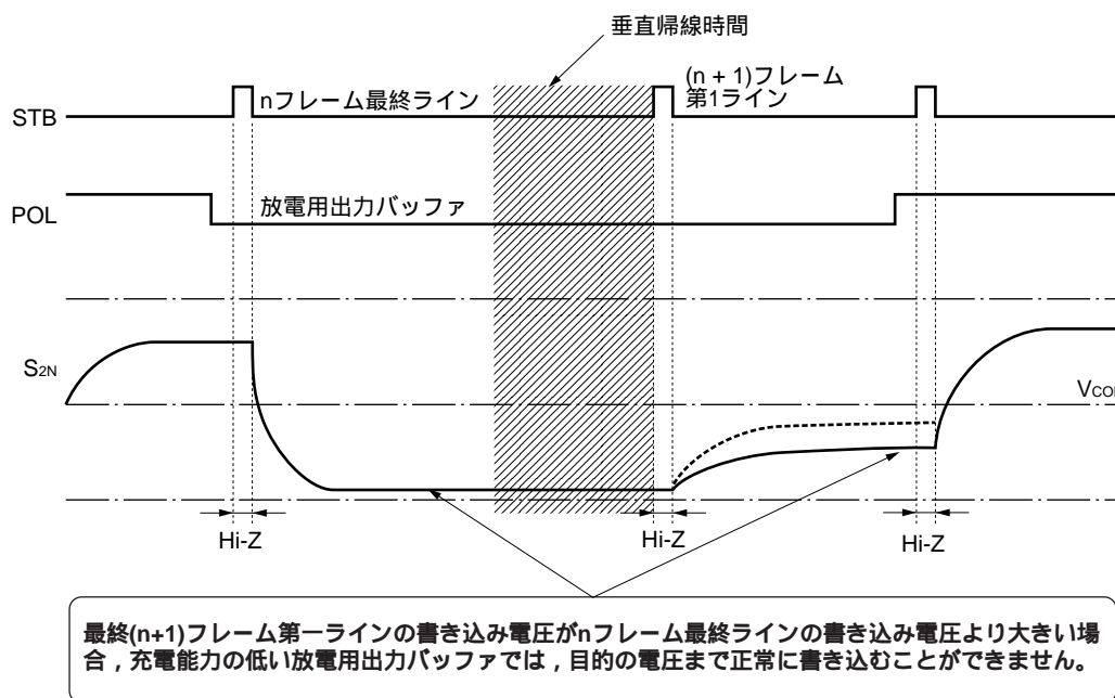
図8-1 出力電圧が正常に書き込めない場合
