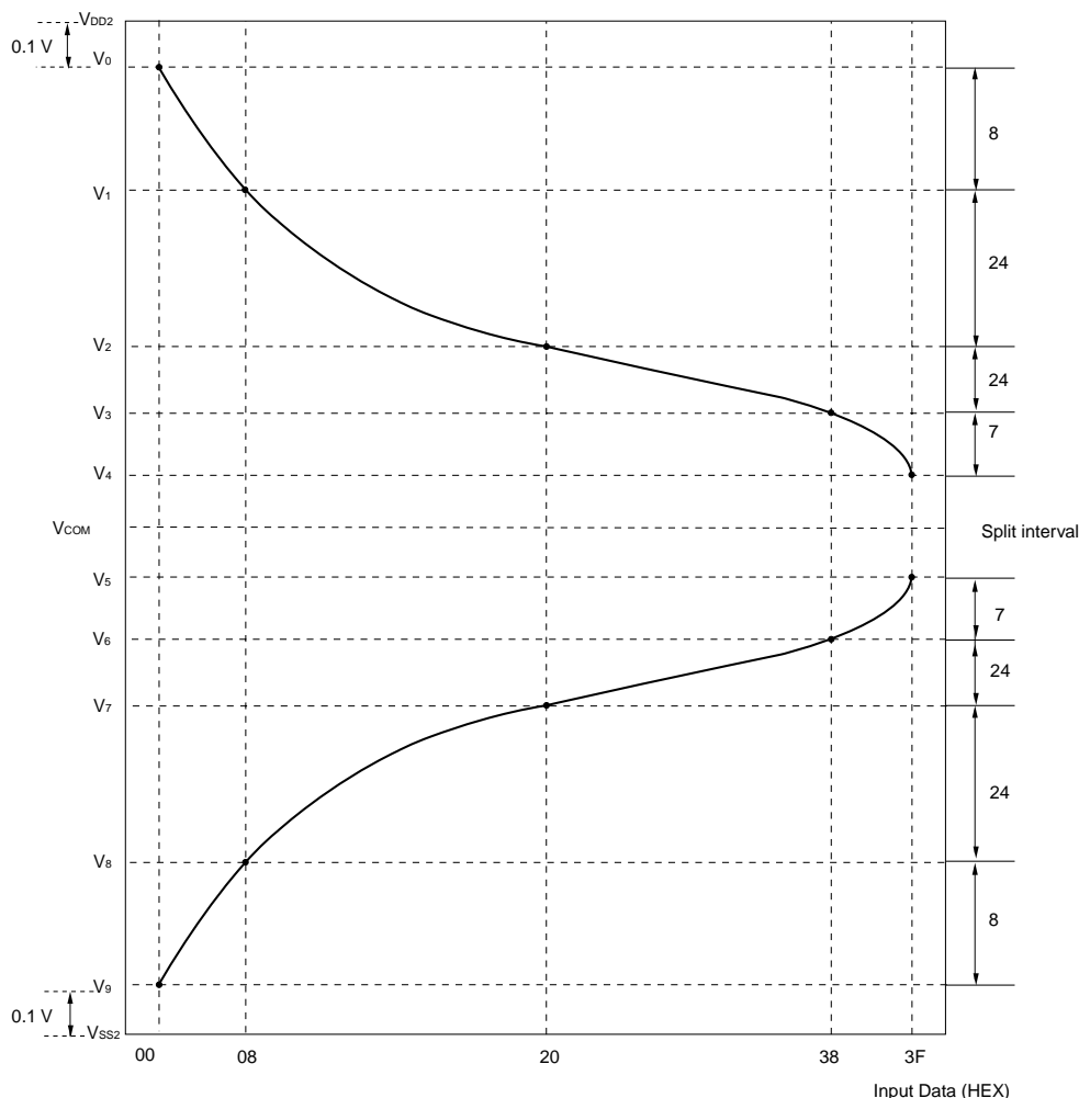
図5 - 1 入力データとγ補正電源の関係
