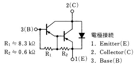
等価回路
