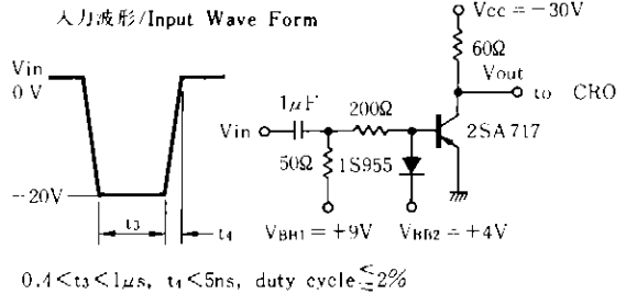
t_{sig, toff} 測定回路 / t_{sig, toff} Test Circuit
