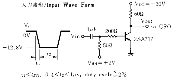
t_{on} 測定回路 / t_{on} Test Circuit
