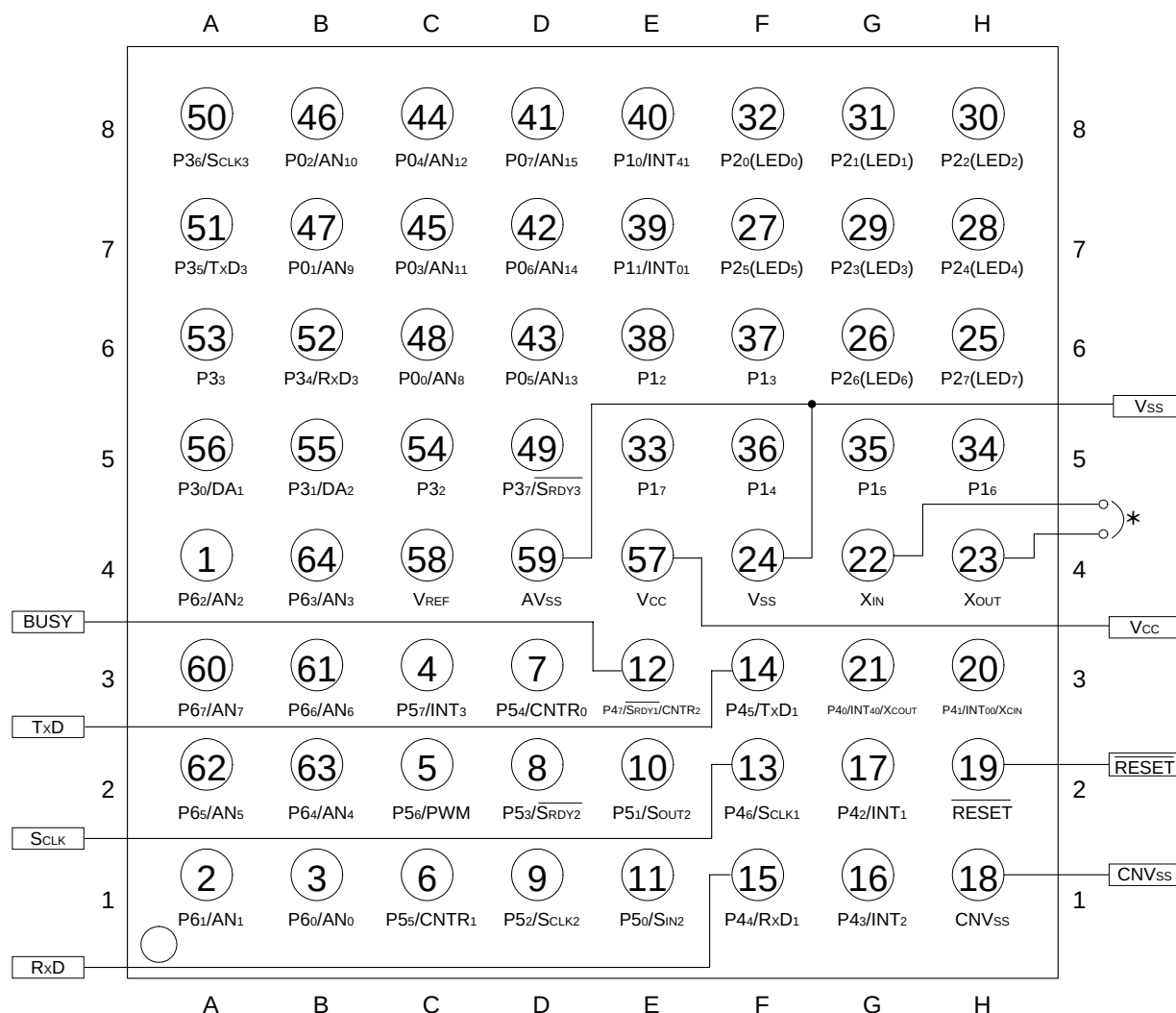
ピン接続図 (上面図)
