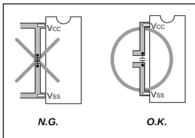
図92. Vss－Vccライン間のバイパスコンデンサ
