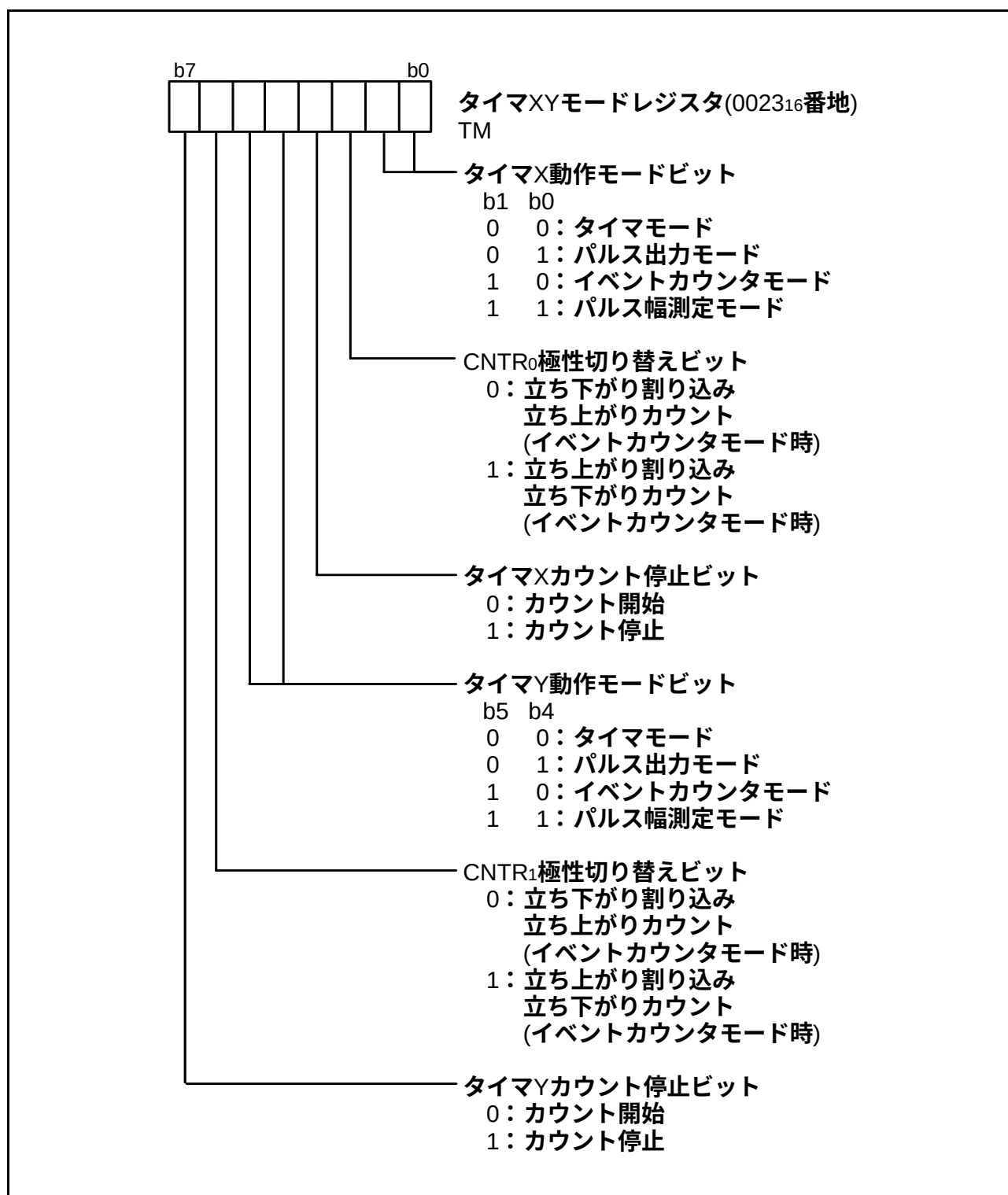
図26. タイマXYモードレジスタの構成
