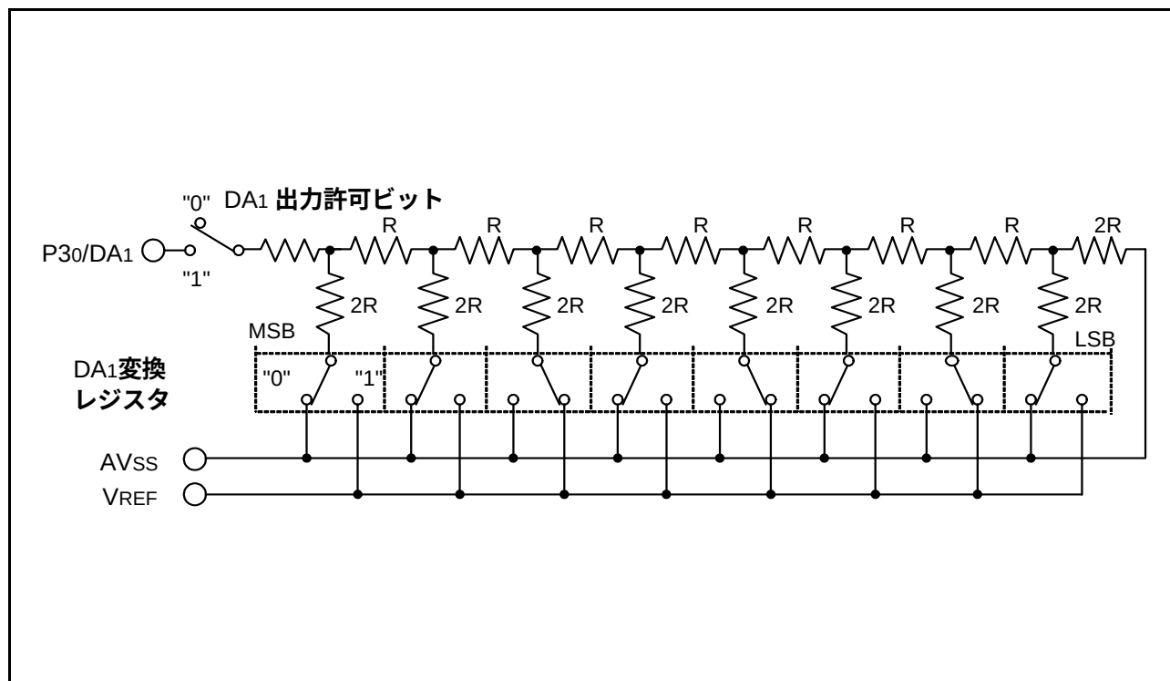
図57. D/Aコンバータ等価回路図(D/A1)
