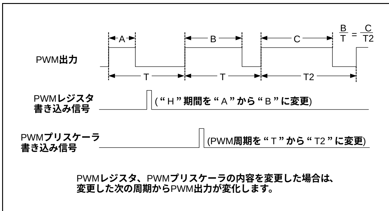
図52. PWMレジスタおよびPWMプリスケアラ変更時のPWM出力タイミング図
