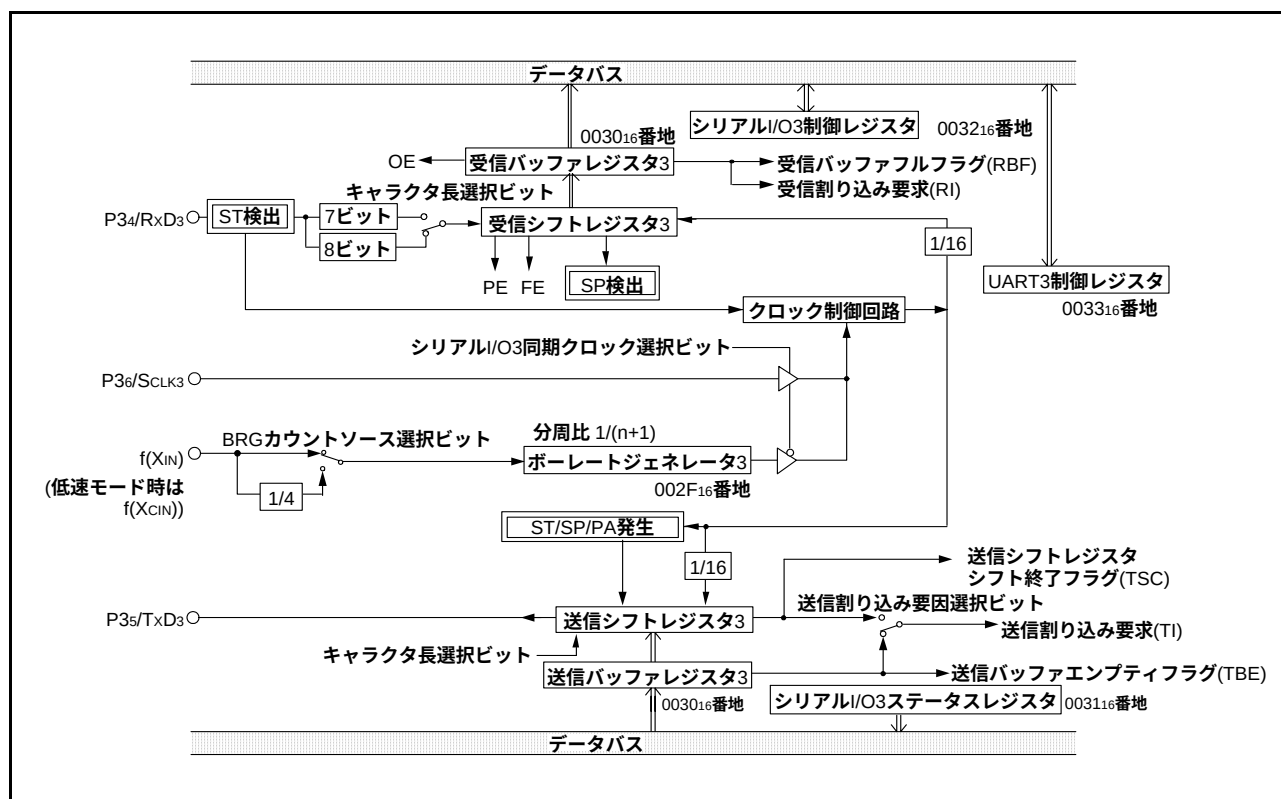
図46. UART形シリアルI/O3ブロック図
