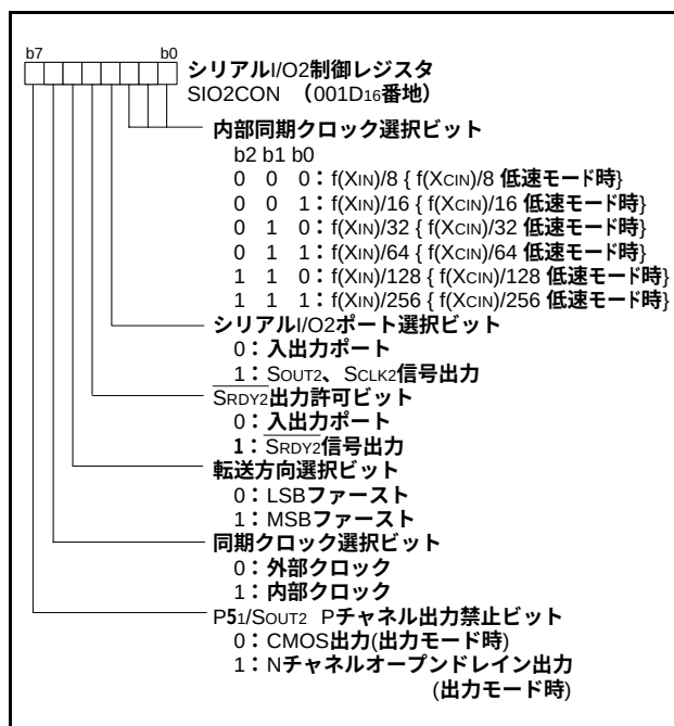
図41. シリアルI/O2制御レジスタの構成
