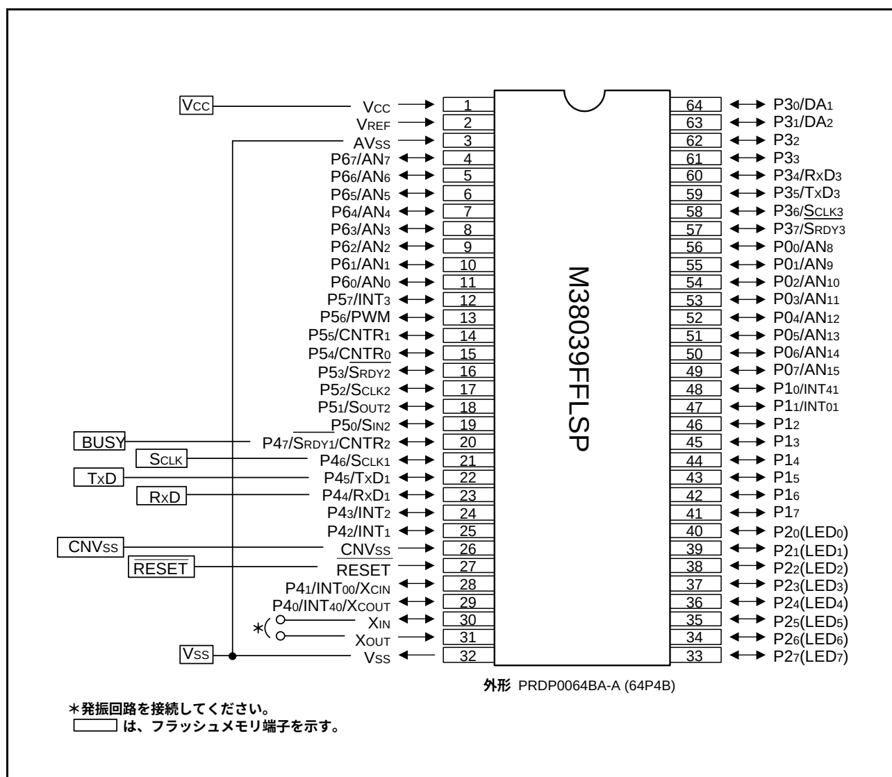
図 79. 標準シリアル入出力モード 1 時の端子結線図 (M38039FFLSP)
