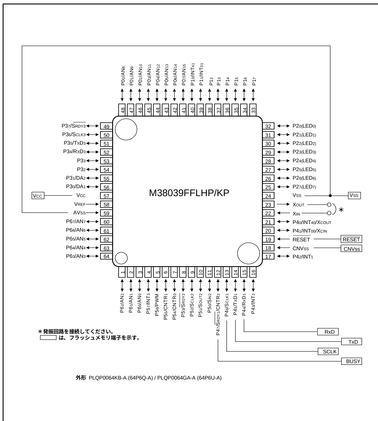
図 77. 標準シリアル入出力モード 1 時の端子結線図 (M38039FFLHP/KP)
