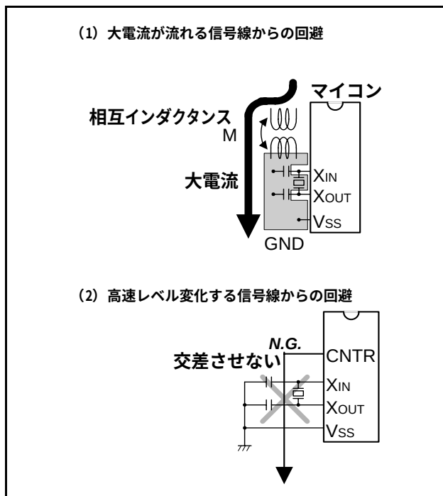
図93. 大電流が流れる信号線の配線/高速にレベル変化する信号線の配線
