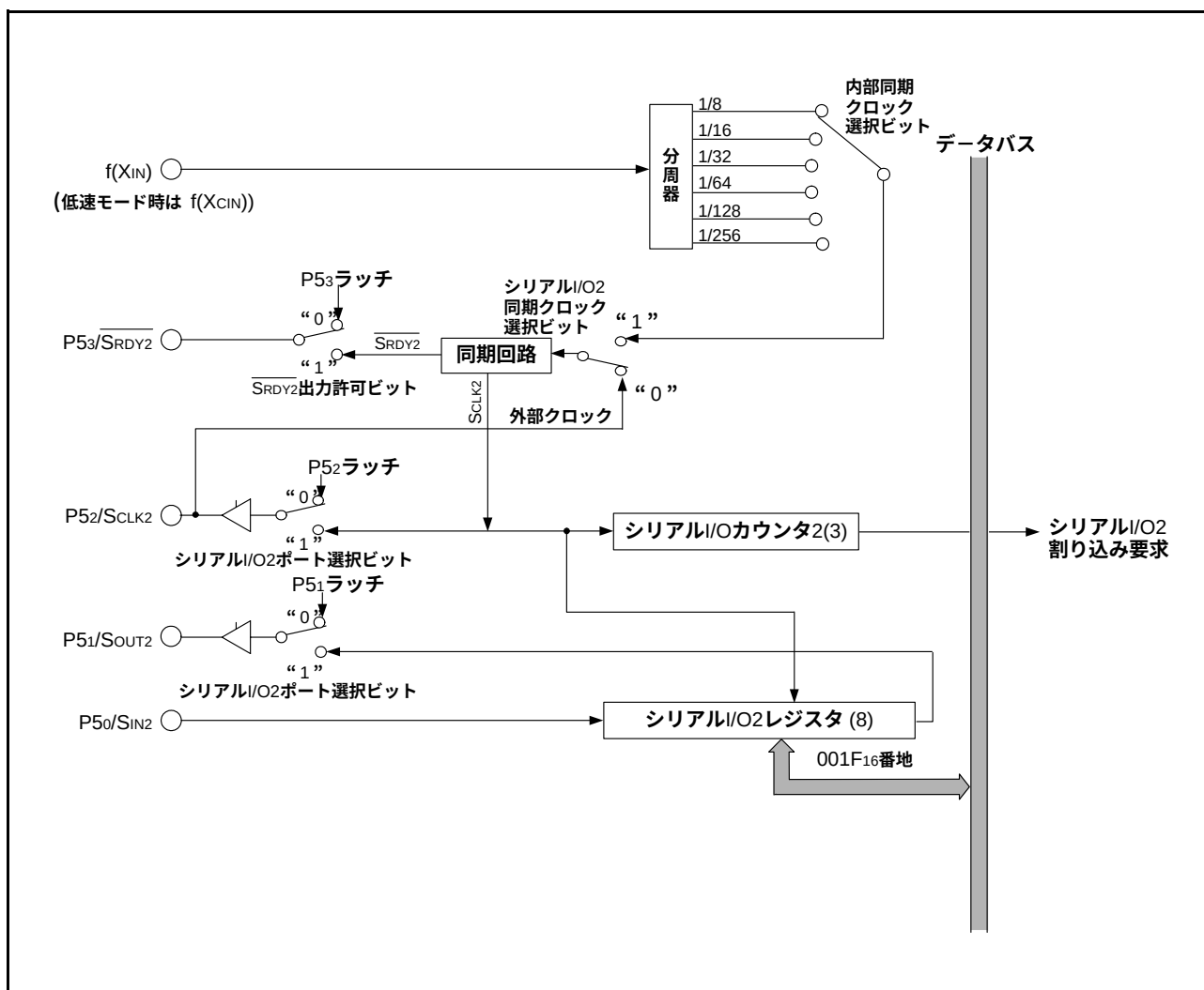
図42. シリアルI/O2ブロック図
