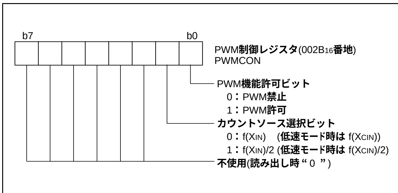
図51. PWM制御レジスタの構成
