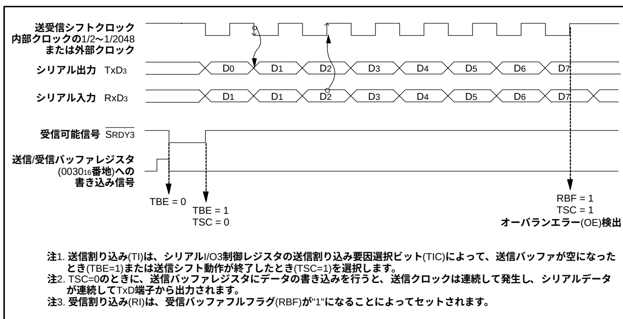
図45. クロック同期形シリアルI/O3動作図
