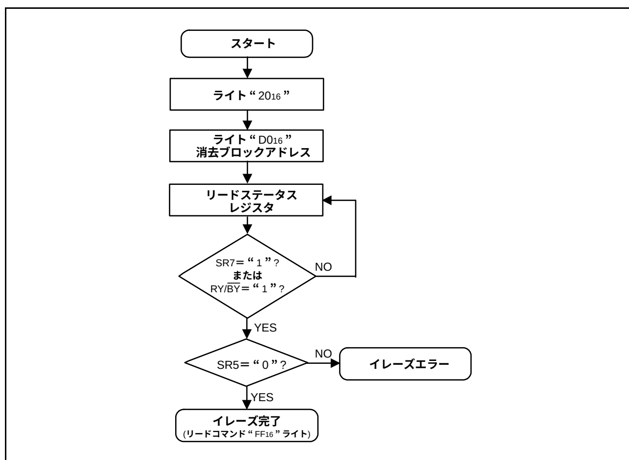
図 73. イレーズフローチャート
