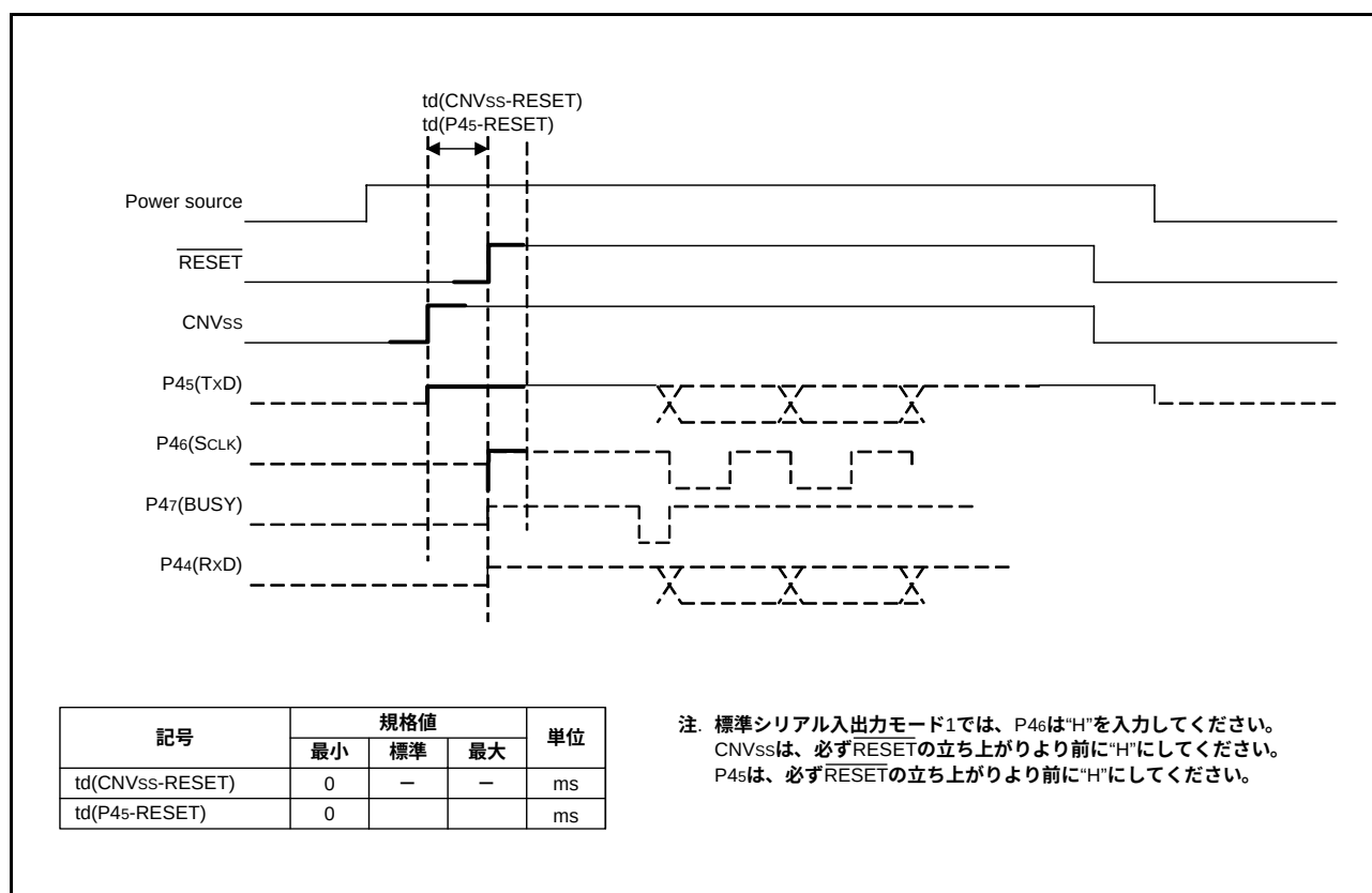
図83. 標準シリアル入出力モード1時の動作波形図
