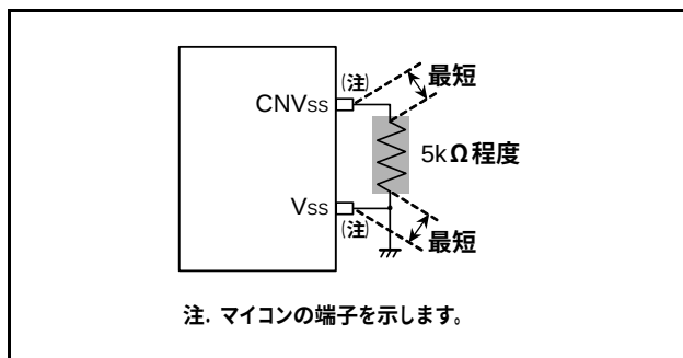
図 99. CNVss 端子の配線
