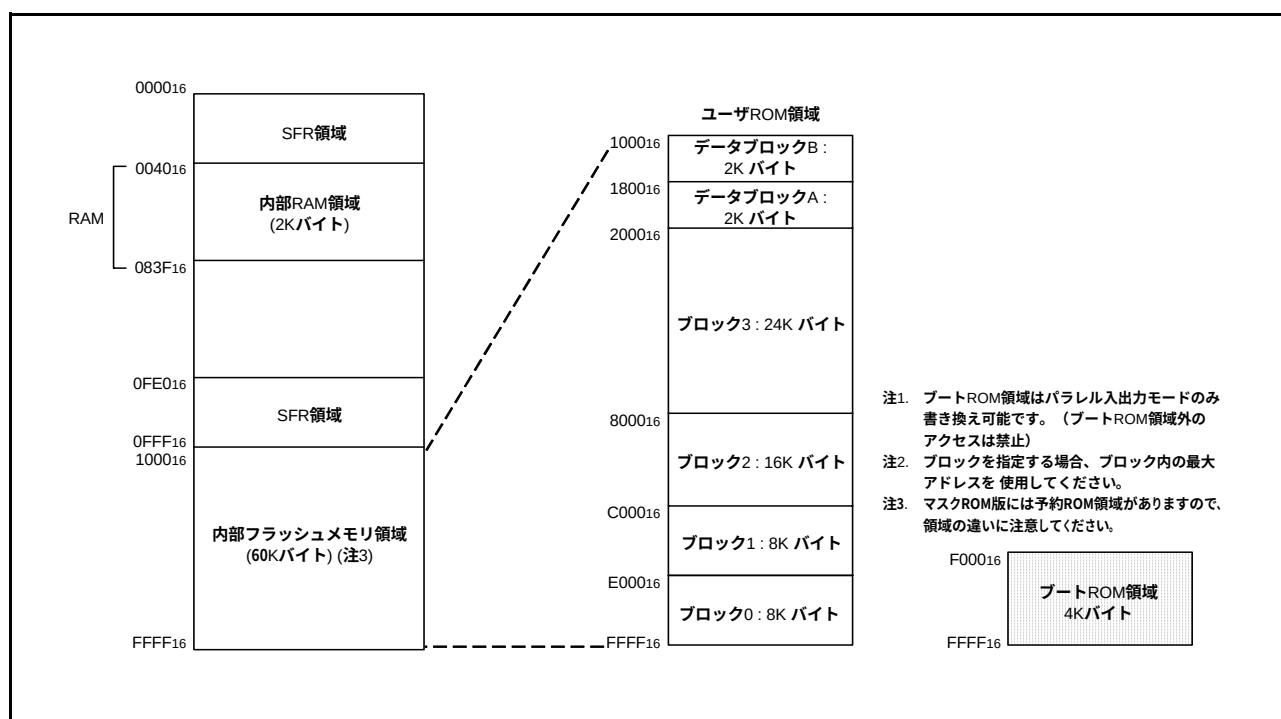
図67. 内蔵フラッシュメモリのブロック図
