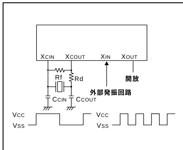
図64. 外部クロック入力回路
