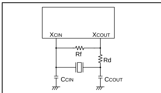
図98. 水晶発振外付け
