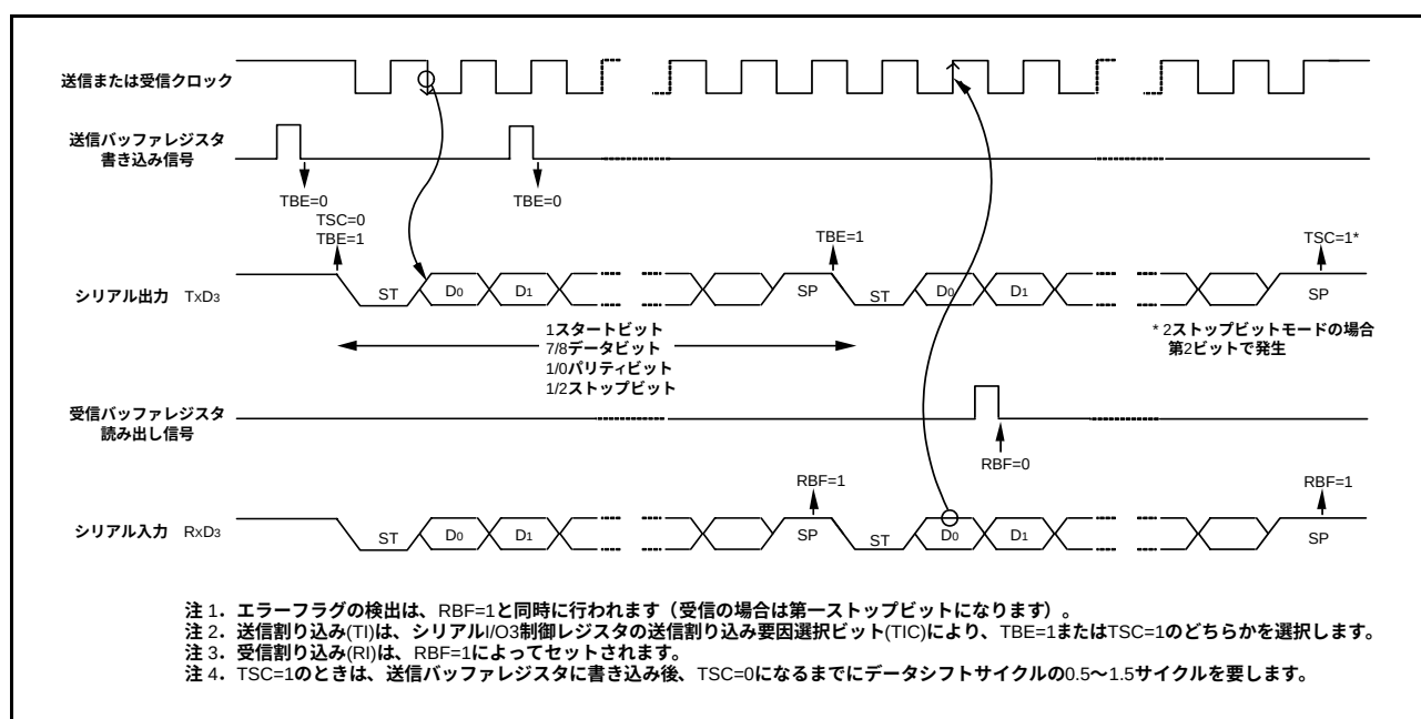
図47. UART形シリアルI/O3動作図
