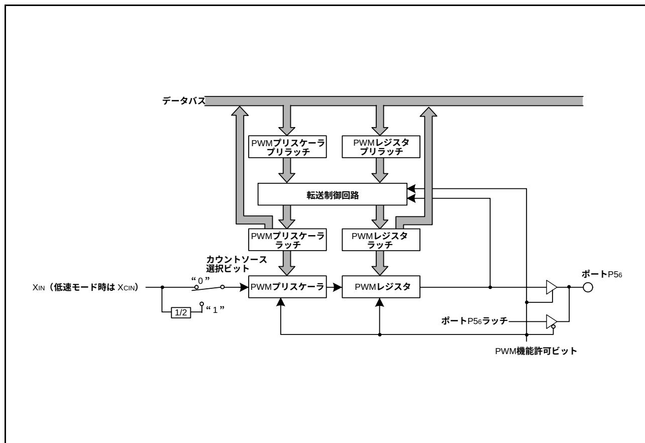
図50. PWMブロック図
