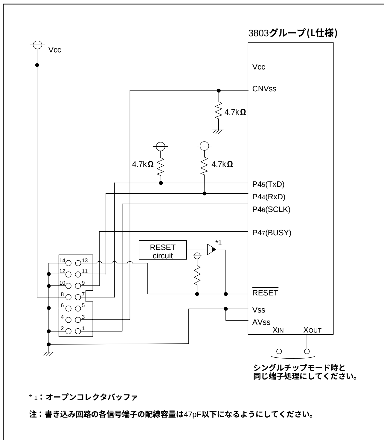
図86. E8プログラマ(標準シリアル入出力モード1)使用時の基板上の端子処理例
