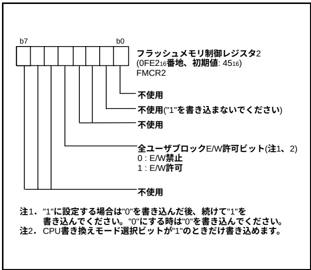
図70. フラッシュメモリ制御レジスタ2の構成
