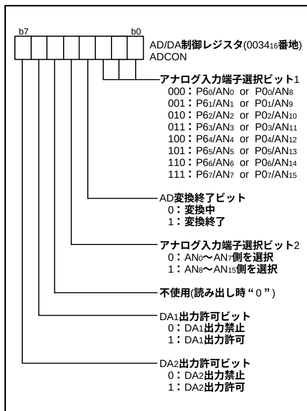
図53. AD/DA制御レジスタの構成
