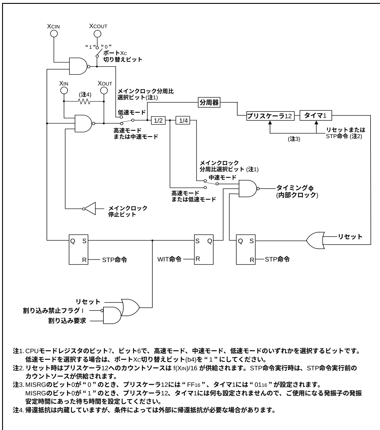
図65. システムクロック発生回路ブロック図 (シングルチップモード)
