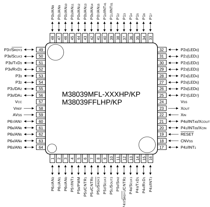
外形 PLQP0064KB-A (64P6Q-A) / PLQP0064GA-A (64P6U-A)
