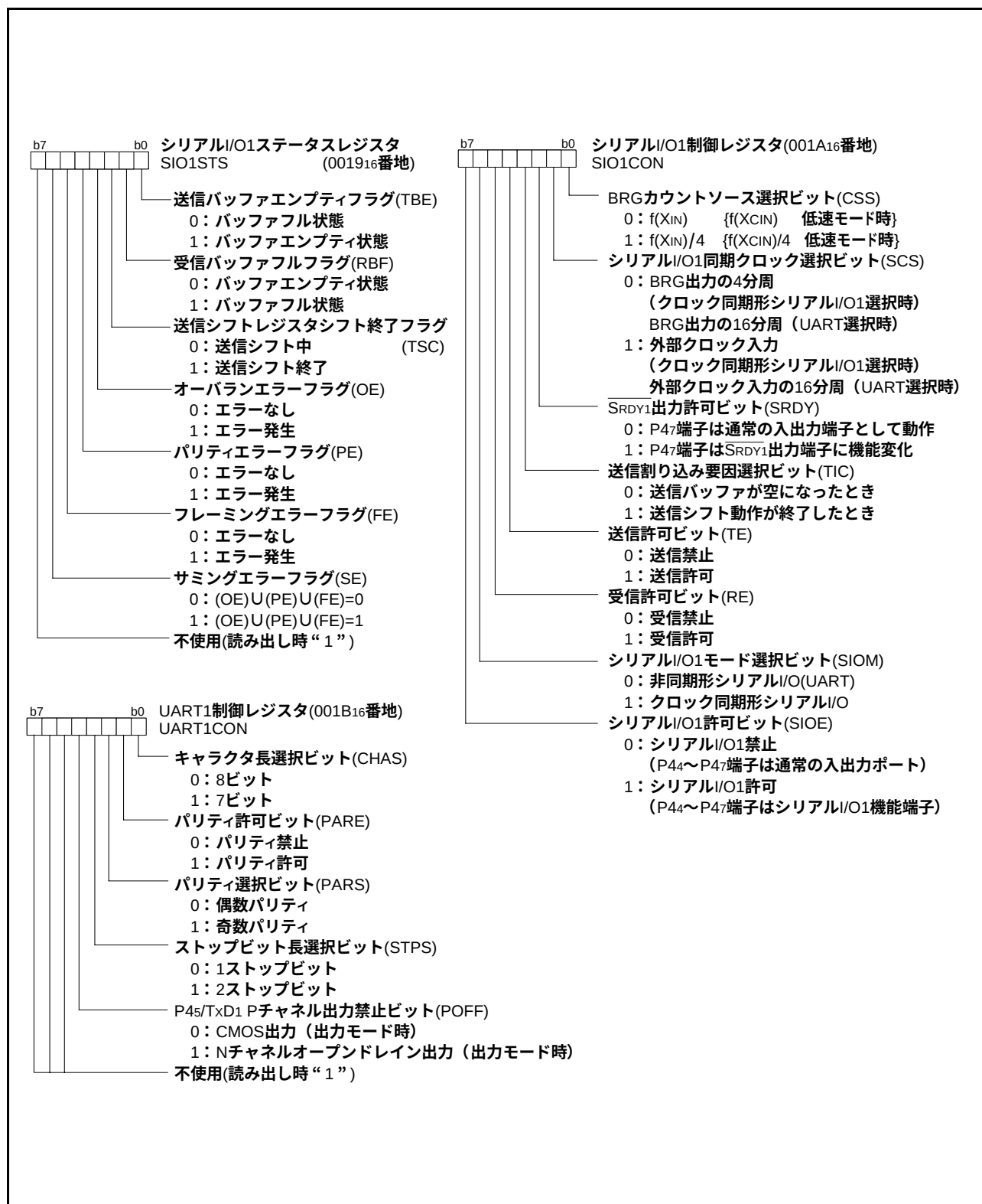
図40. シリアルI/O関係レジスタの構成
