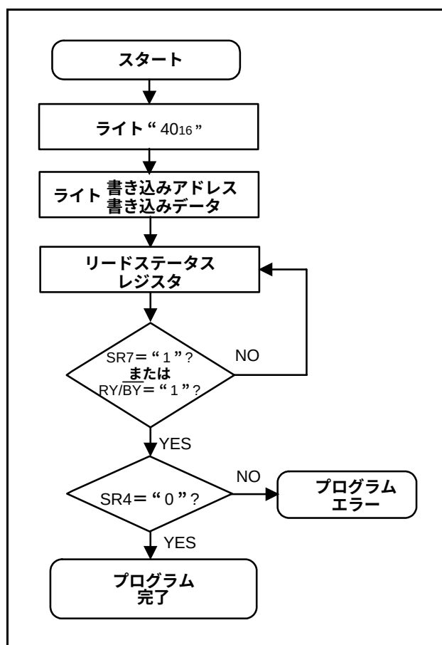
図72. プログラムフローチャート
