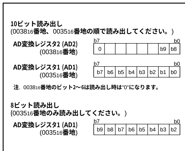
図54. 10ビットA/Dモードの読み出し構成
