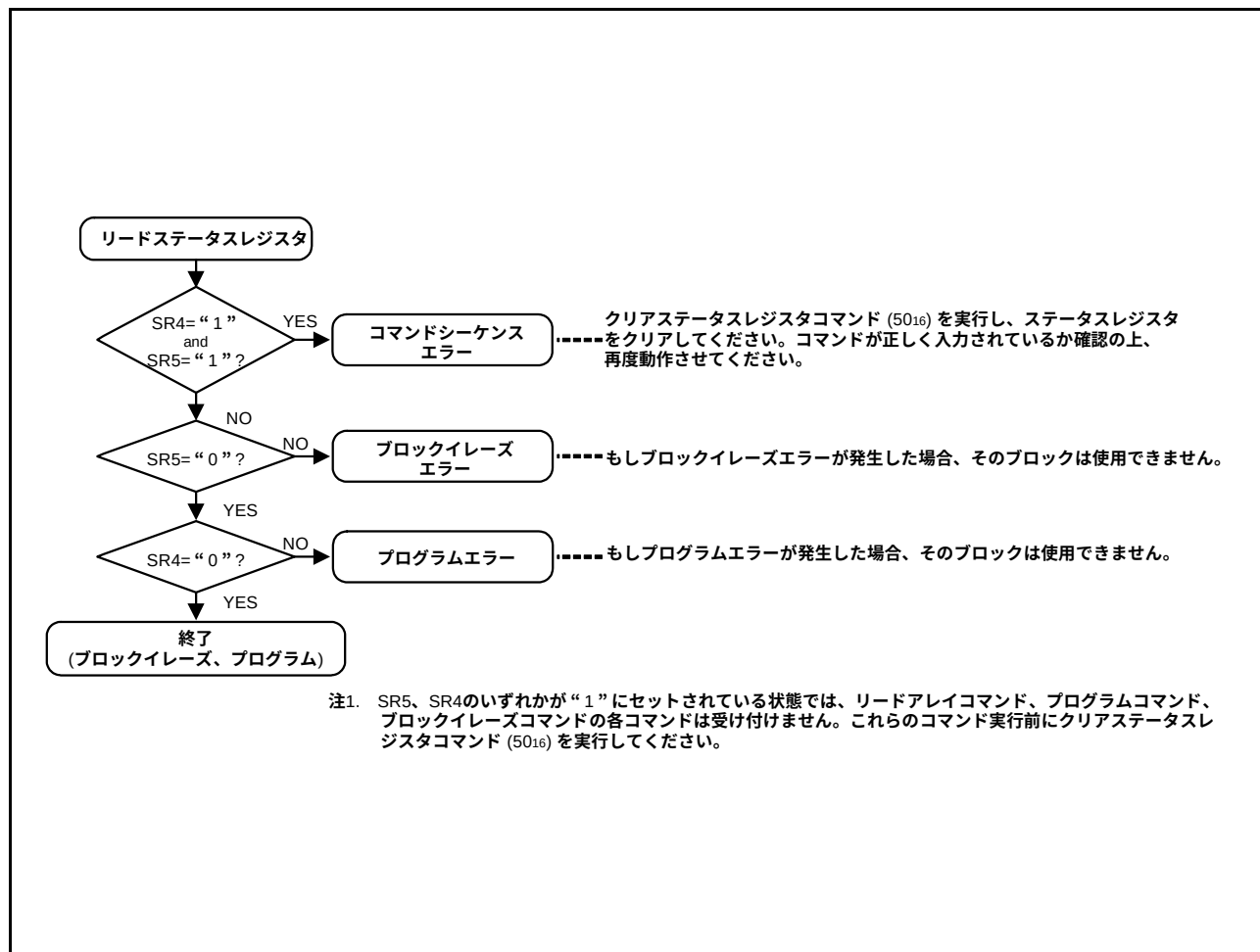
図74. フルステータスチェックフローチャートおよび各エラー発生時の対処方法
