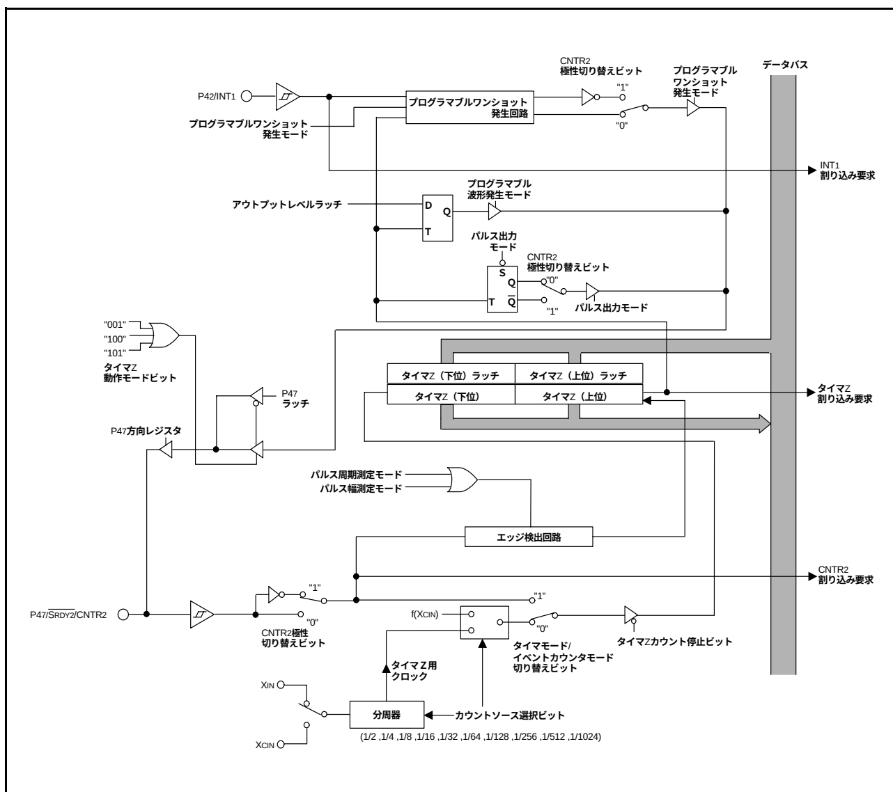
図28. タイマZのブロック図
