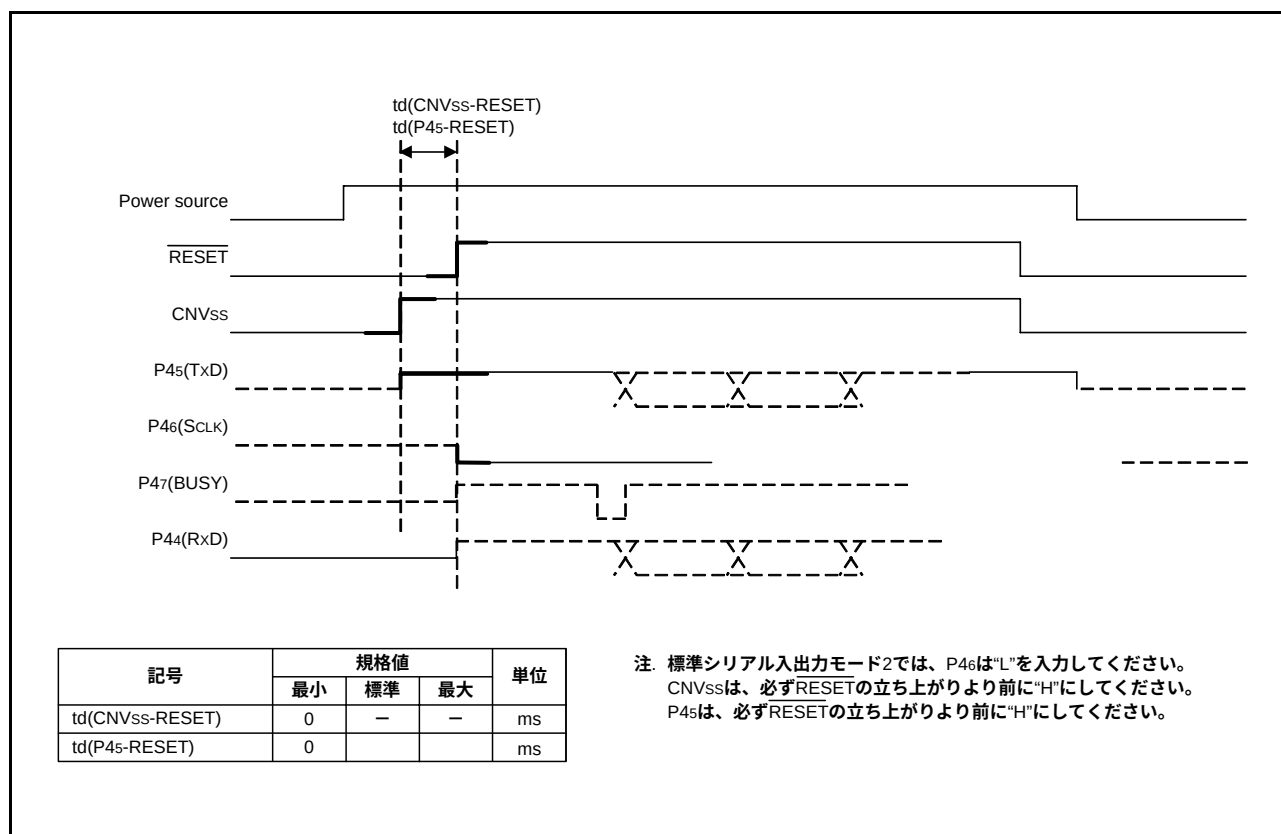
図84. 標準シリアル入出力モード2時の動作波形図
