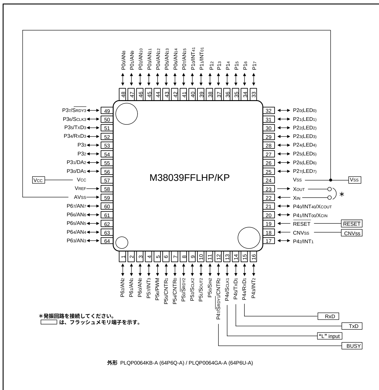
図 78. 標準シリアル入出力モード 2 時の端子結線図 (M38039FFLHP/KP)
