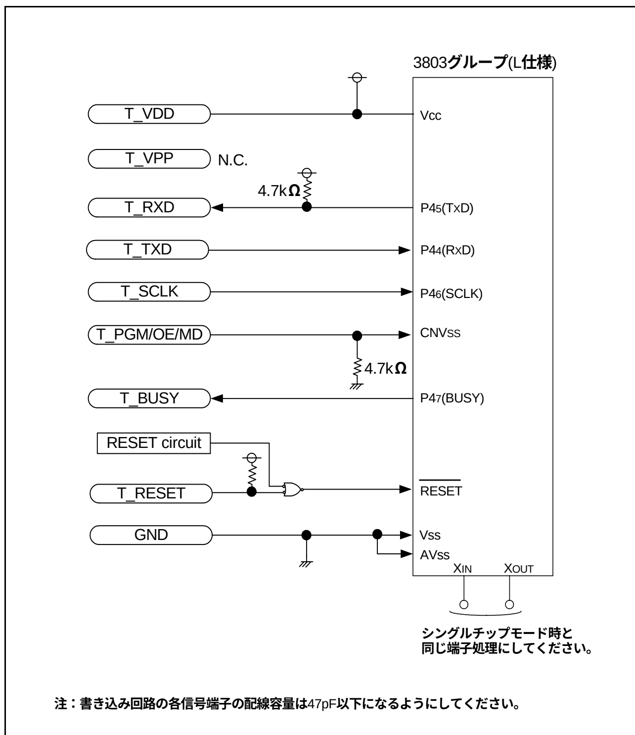
図85. 慧星電子システム製プログラマ(標準シリアル入出力モード1) 使用時の基板上の端子処理例
