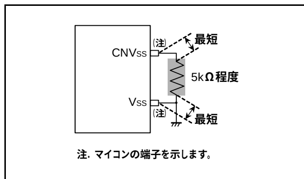
図94. CNVss端子の配線
