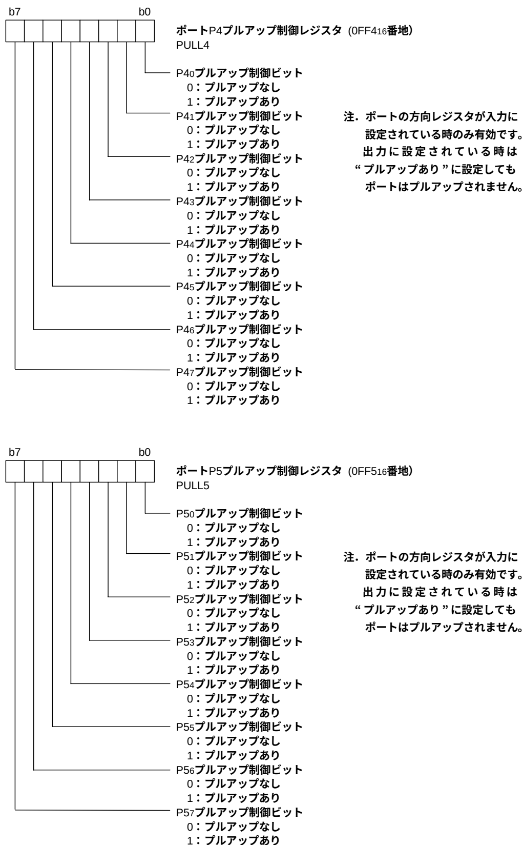
図18. ポートレジスタ構成図(3)
