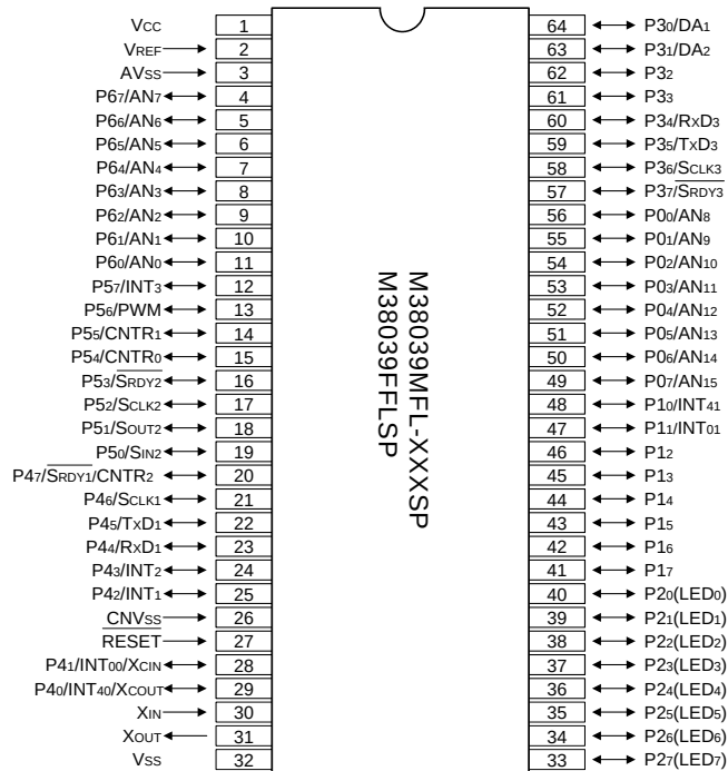
外形 PRDP0064BA-A (64P4B)
