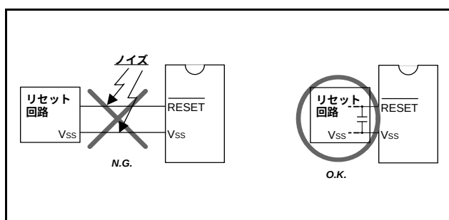
図90. リセット入力端子の配線
