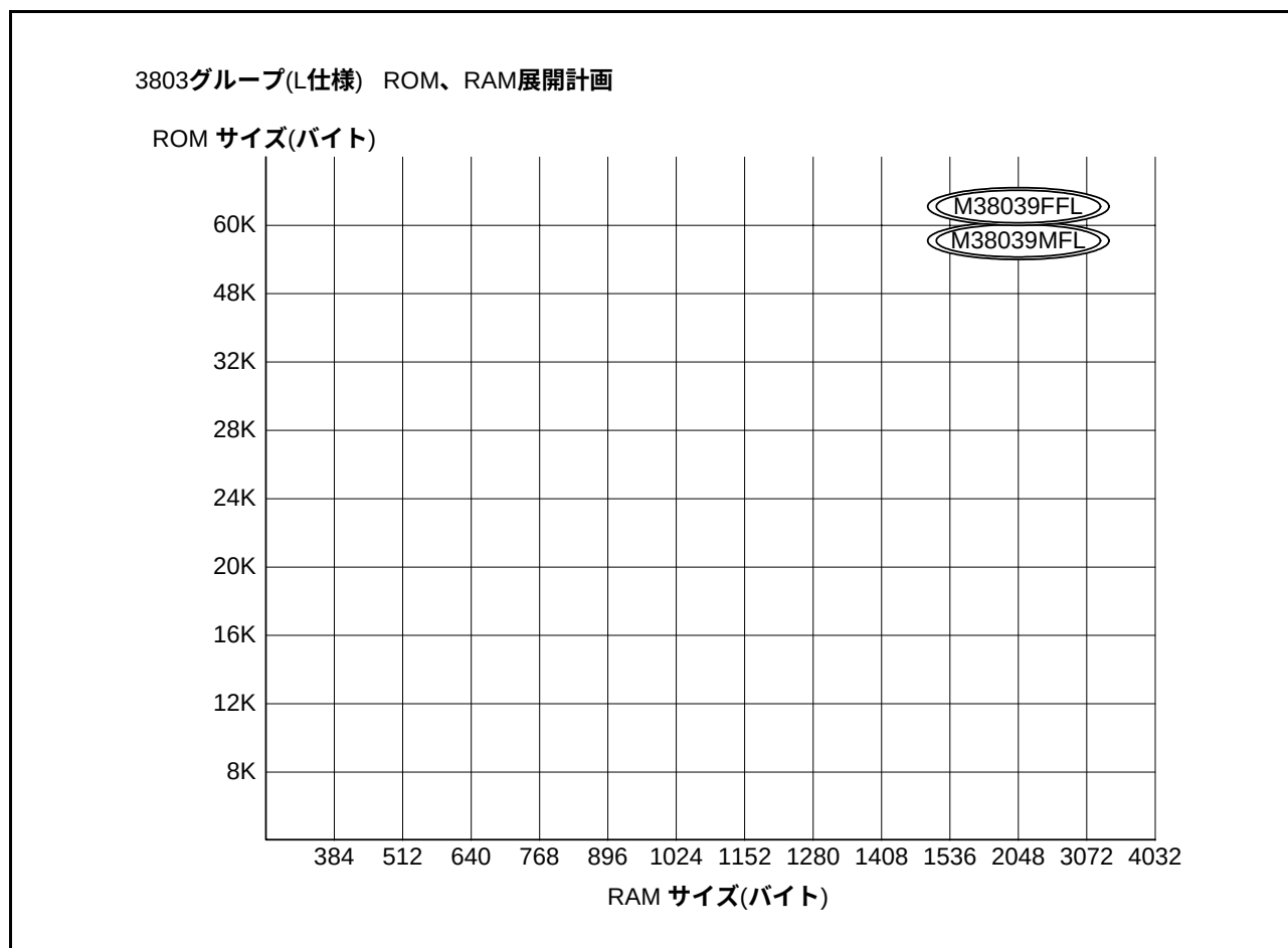
図6. ROMおよびRAM展開計画
