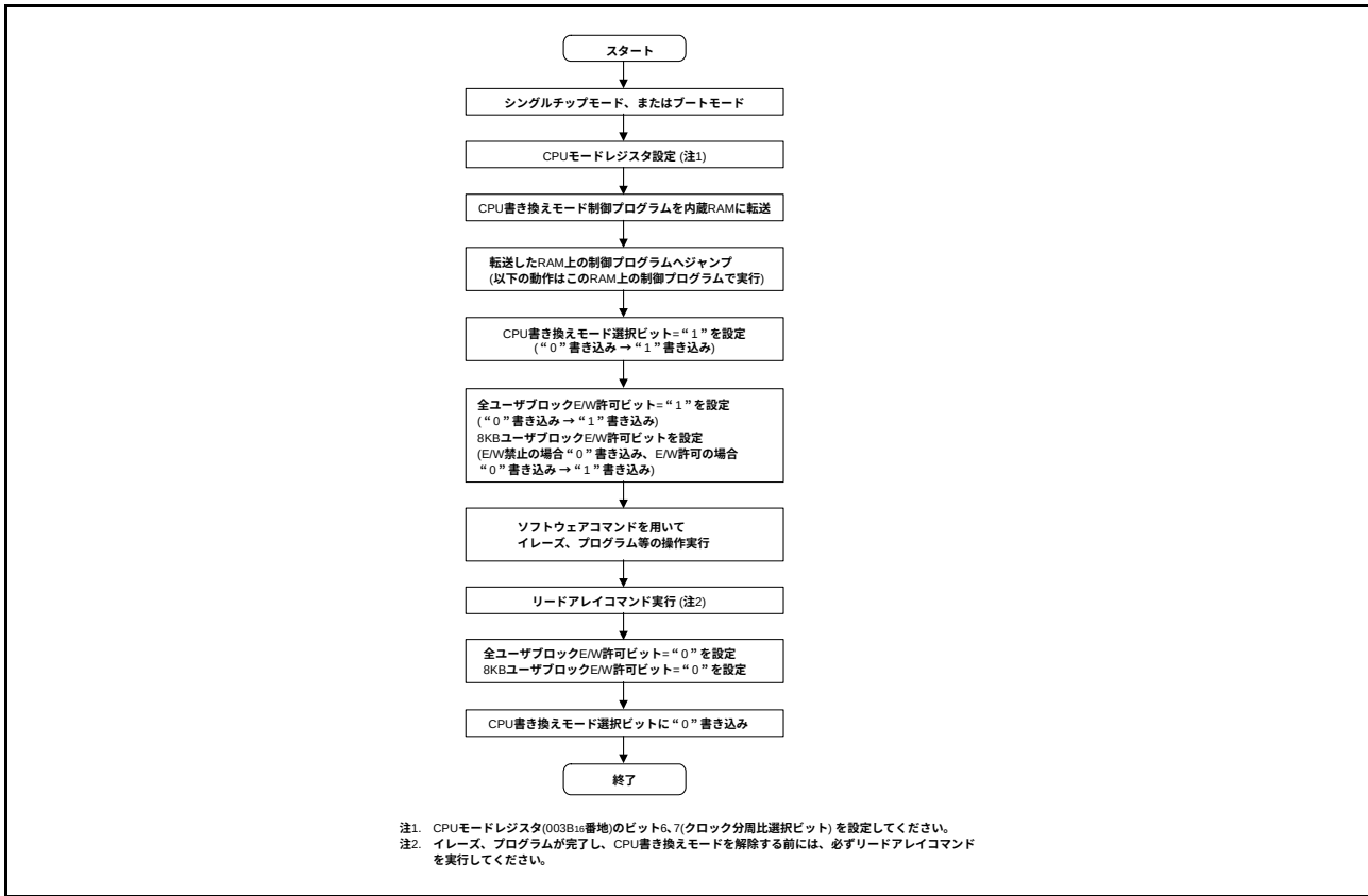
図71. CPU書き換えモードの設定/解除フローチャート
