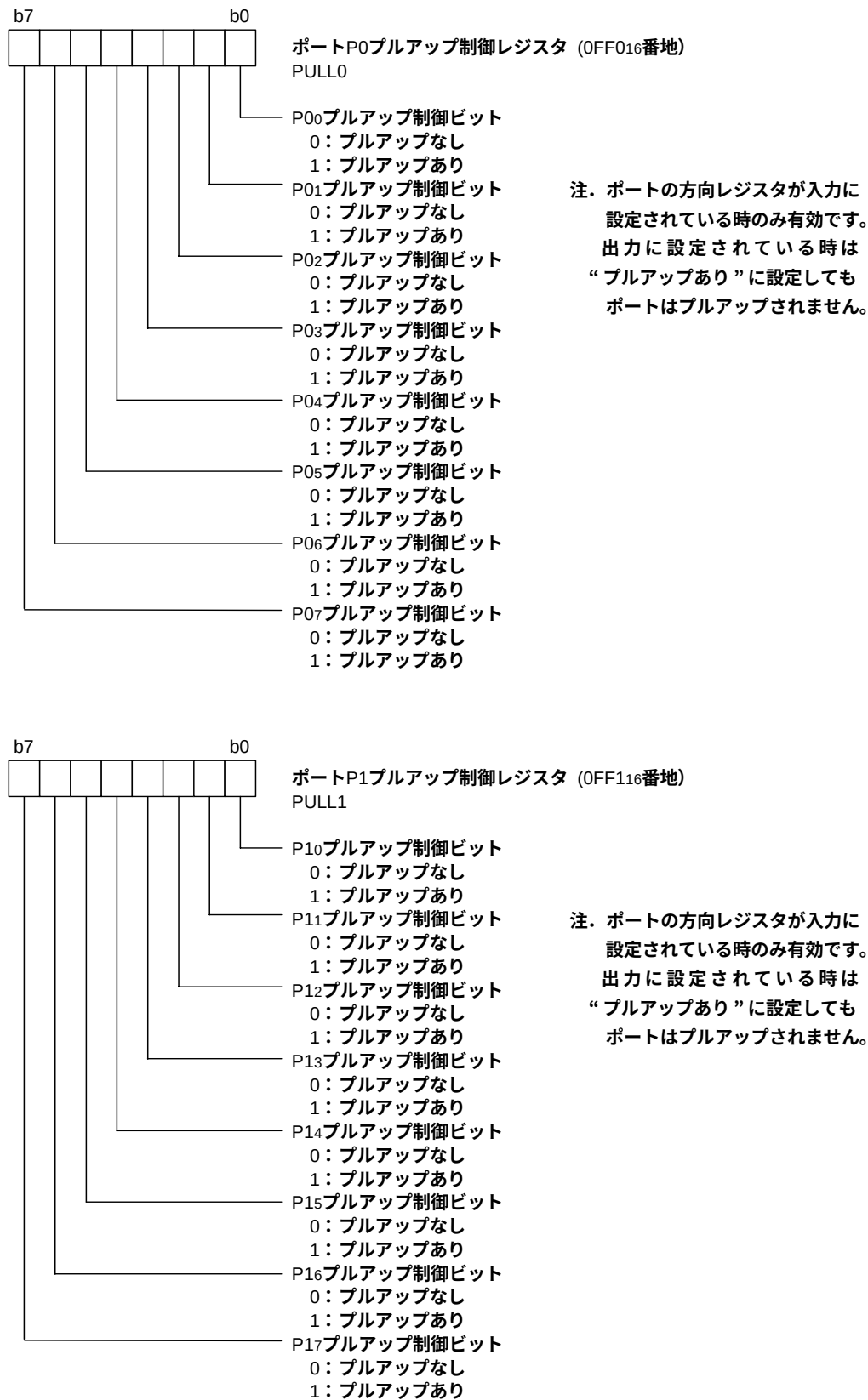
図16. ポートレジスタ構成図(1)
