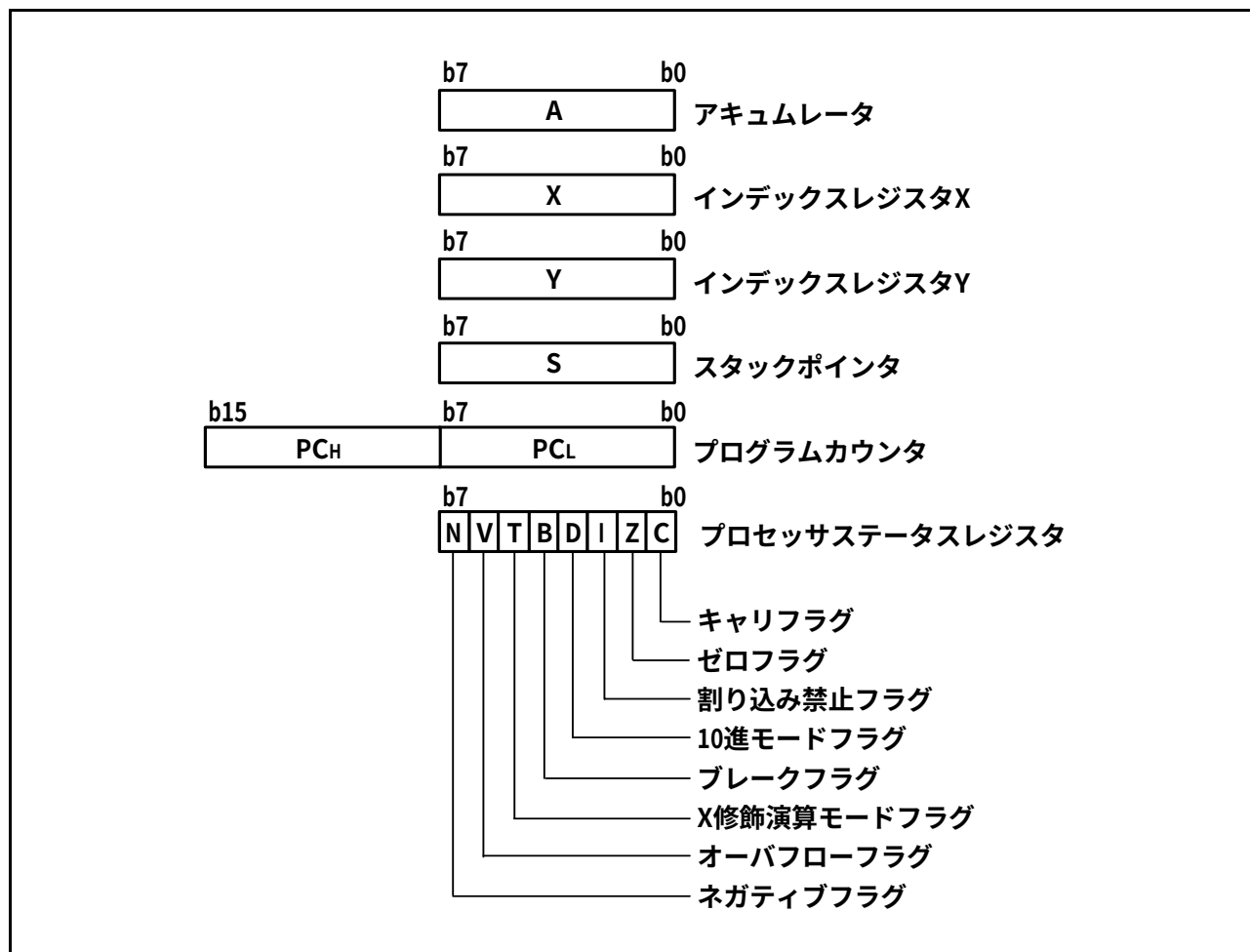
図7. 740ファミリCPUの構成
