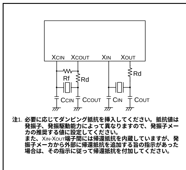
図63. セラミック共振子外付け回路
