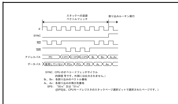
図23. 割り込みシーケンス
