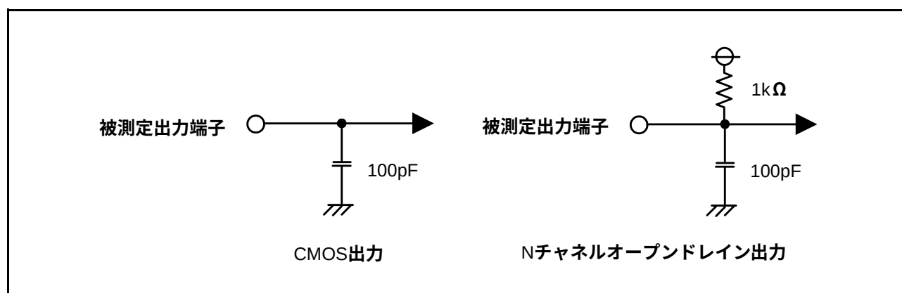
図100. 出力スイッチング特性測定回路図
