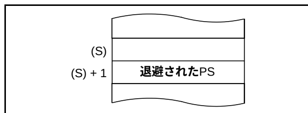
図88. PHP命令実行後のスタックメモリの内容
