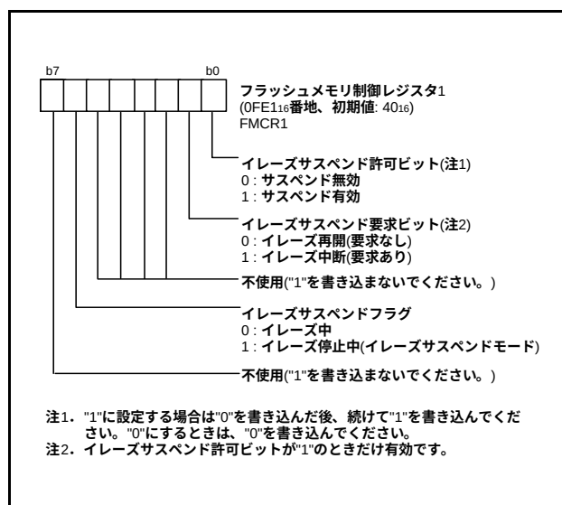
図69. フラッシュメモリ制御レジスタ1の構成
