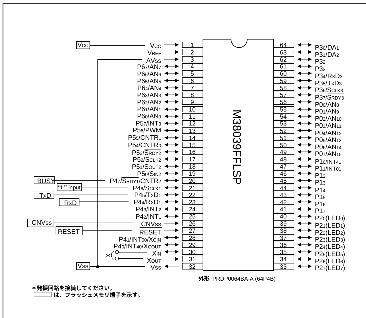
図80. 標準シリアル入出力モード2時の端子結線図 (M38039FFLSP)
