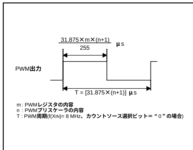
図49. PWM周期のタイミング図
