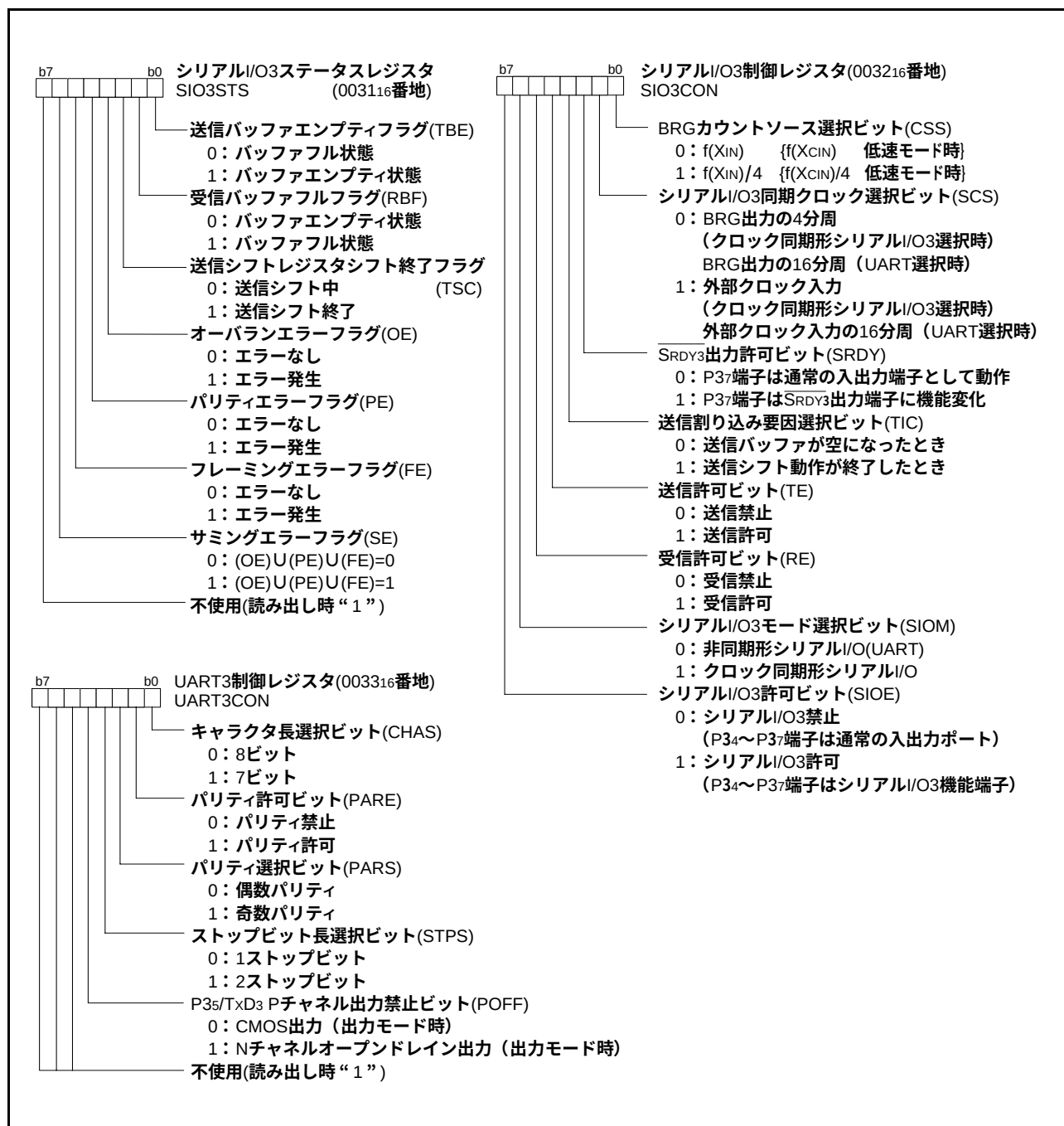
図48. シリアルI/O3関係レジスタの構成
