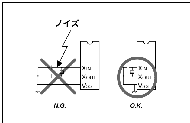
図91. クロック入出力端子の配線
