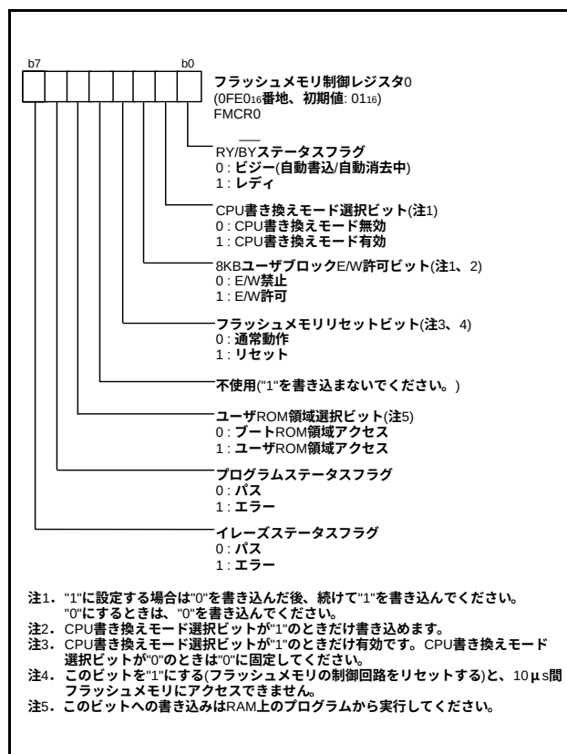
図68. フラッシュメモリ制御レジスタ0の構成
