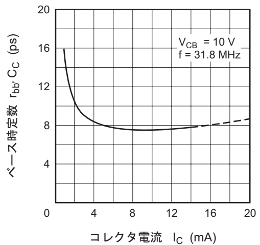
ベース時定数対コレクタ電流特性
