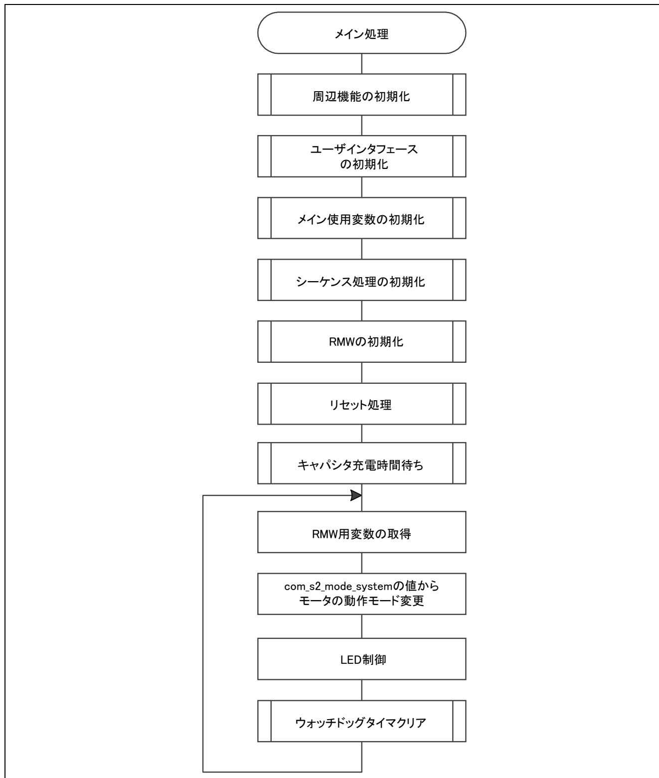
図 3-4 メイン処理
