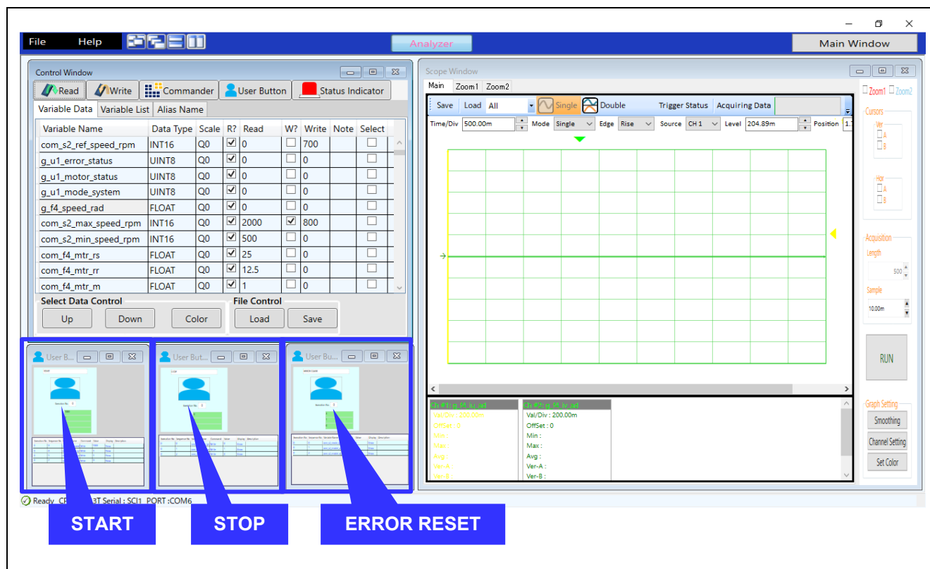
図 4-2 RMW 操作方法
