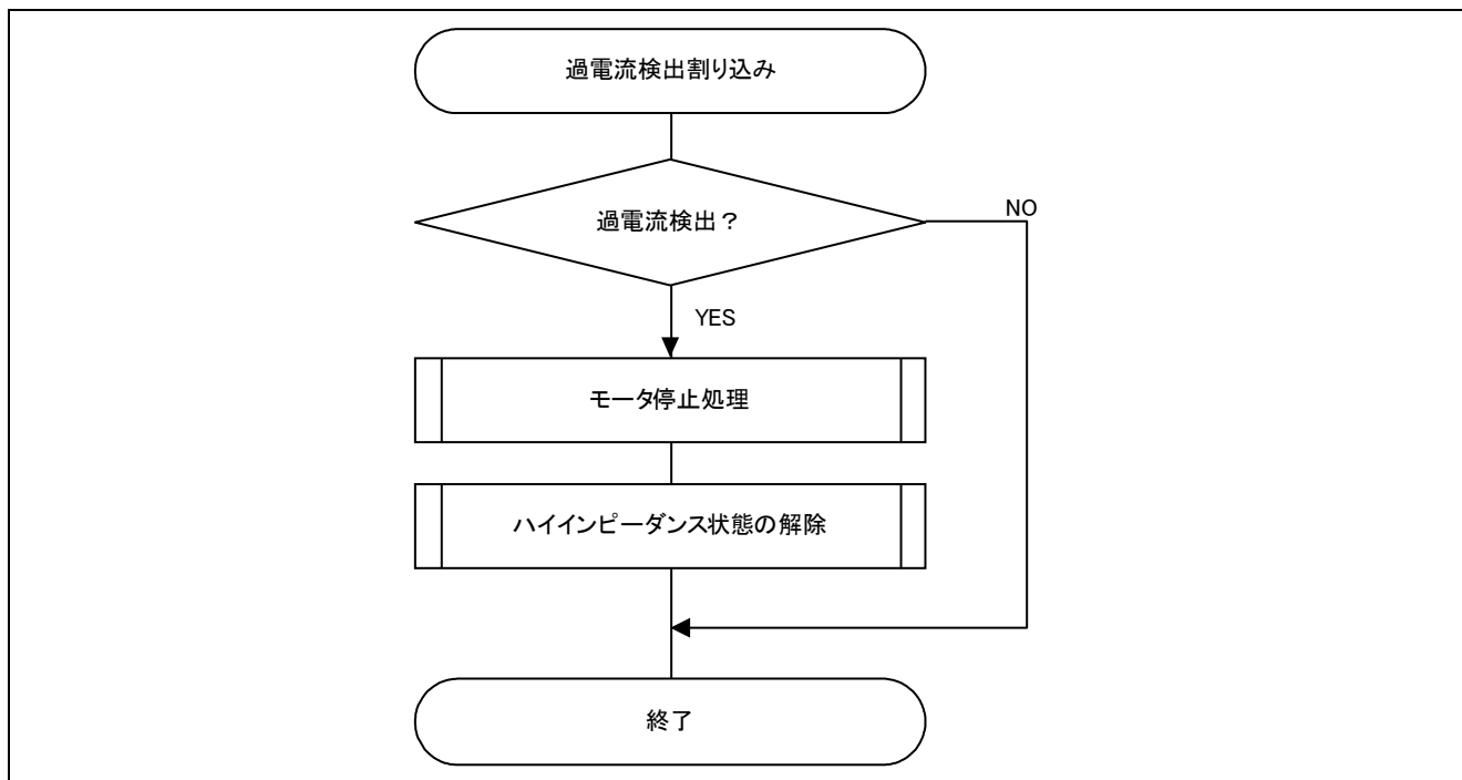
図 3-7 過電流検出割り込み処理
