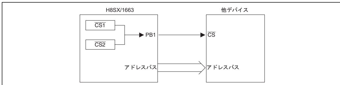
図 1 接続例
