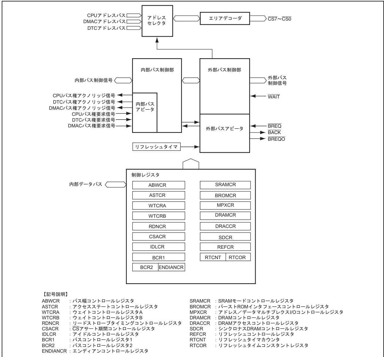
図2 バスコントローラブロック図
