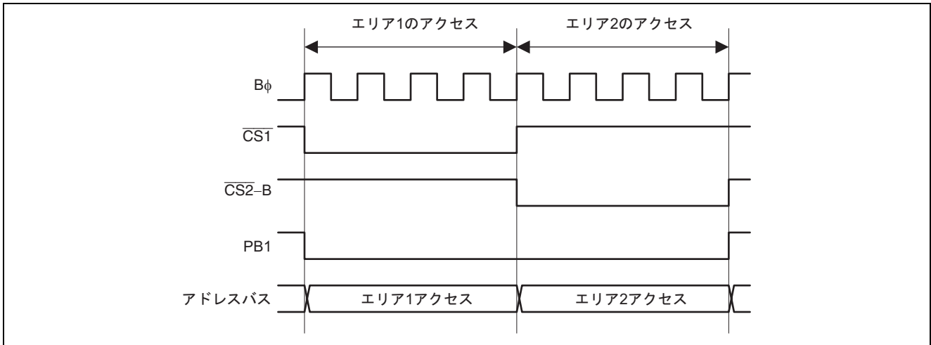
図 4 \overline{CS} を同一端子に出力したときのタイミング
