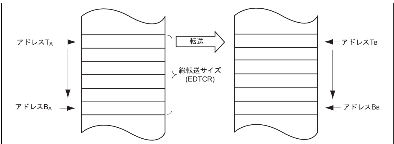
図 5 ノーマル転送モードの動作
