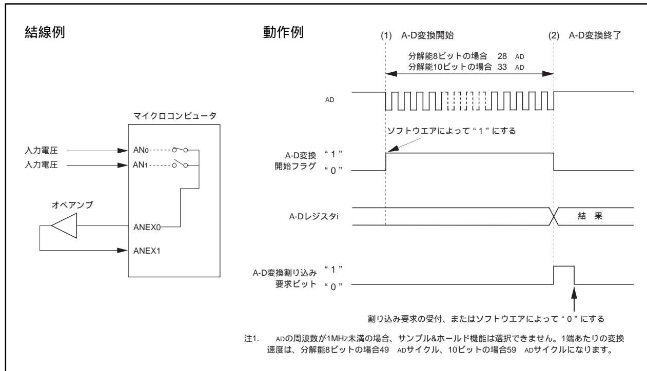
図1 単発モード、外部オペアンプ接続モード選択時の動作タイミング
