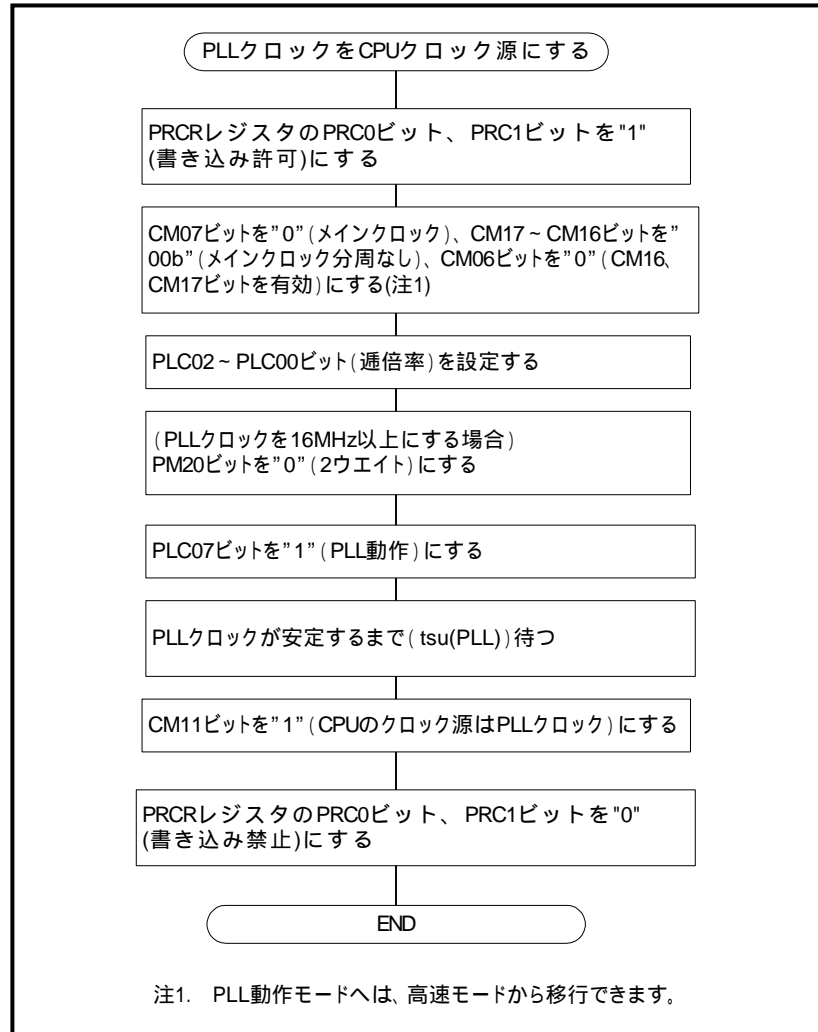
図 1 PLL クロックを CPU のクロック源にするフロー図
