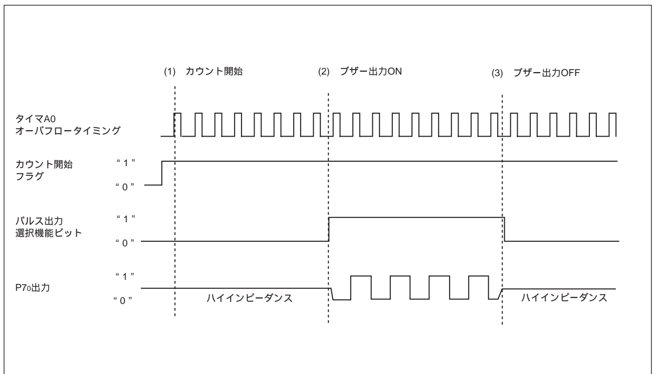
図2 ブザー出力の動作図
