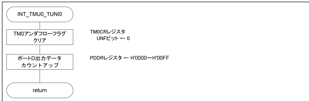
図5.3 INT_TMU0_TUNIO 関数
