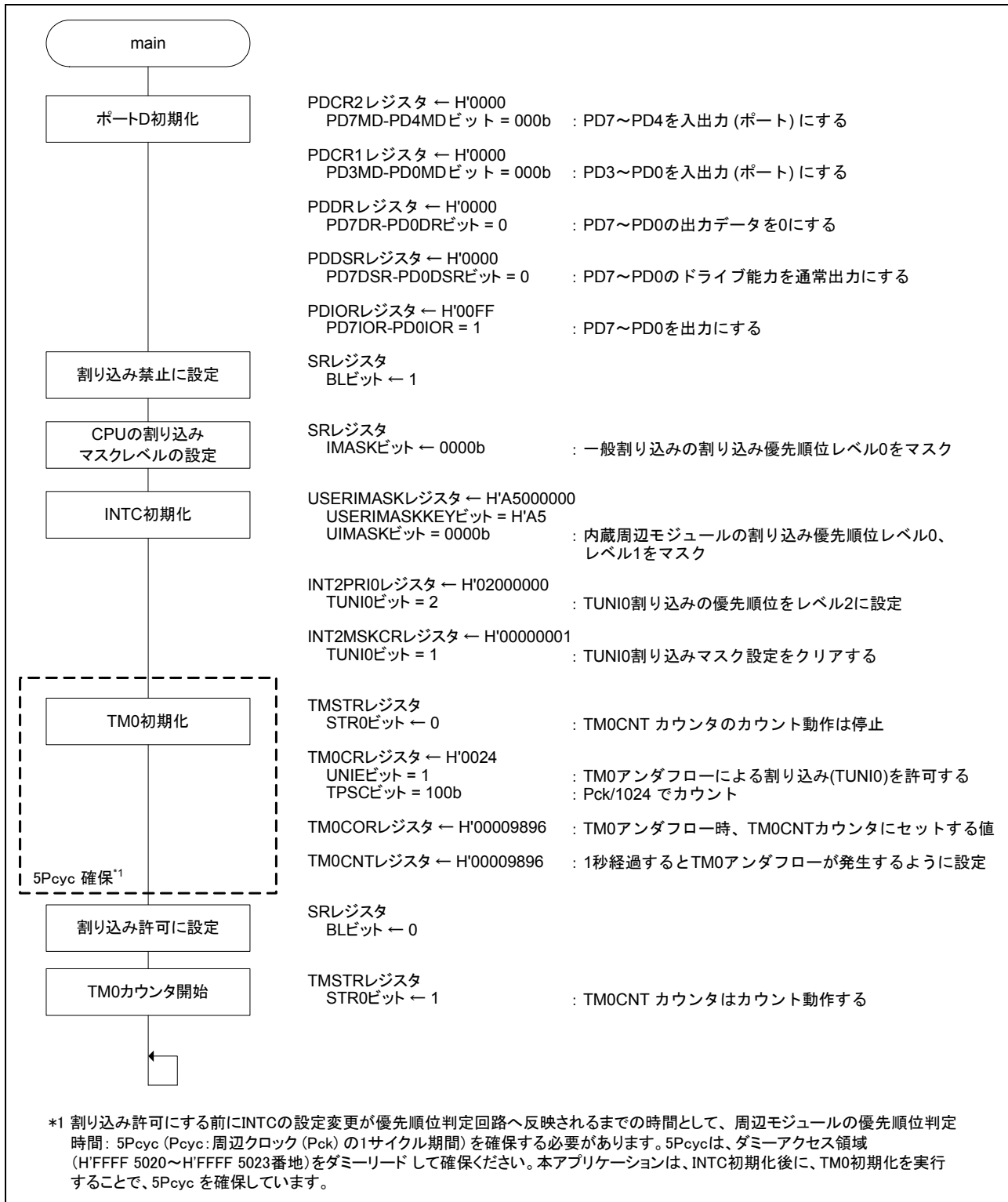
図5.2 main 関数
