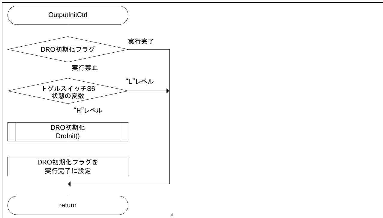
図5.7 OutputInitCtrl 処理
