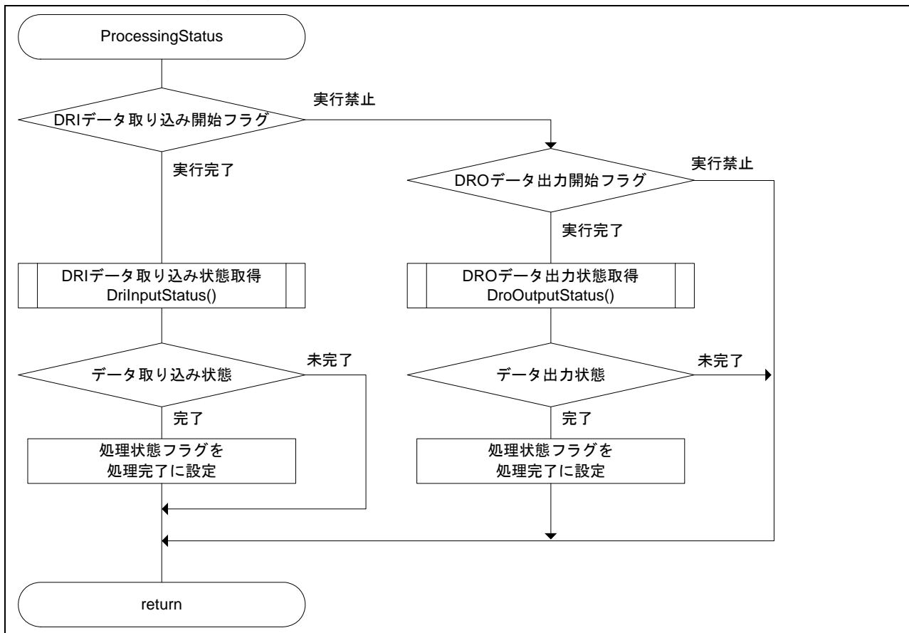
図5.11 ProcessingStatus 処理
