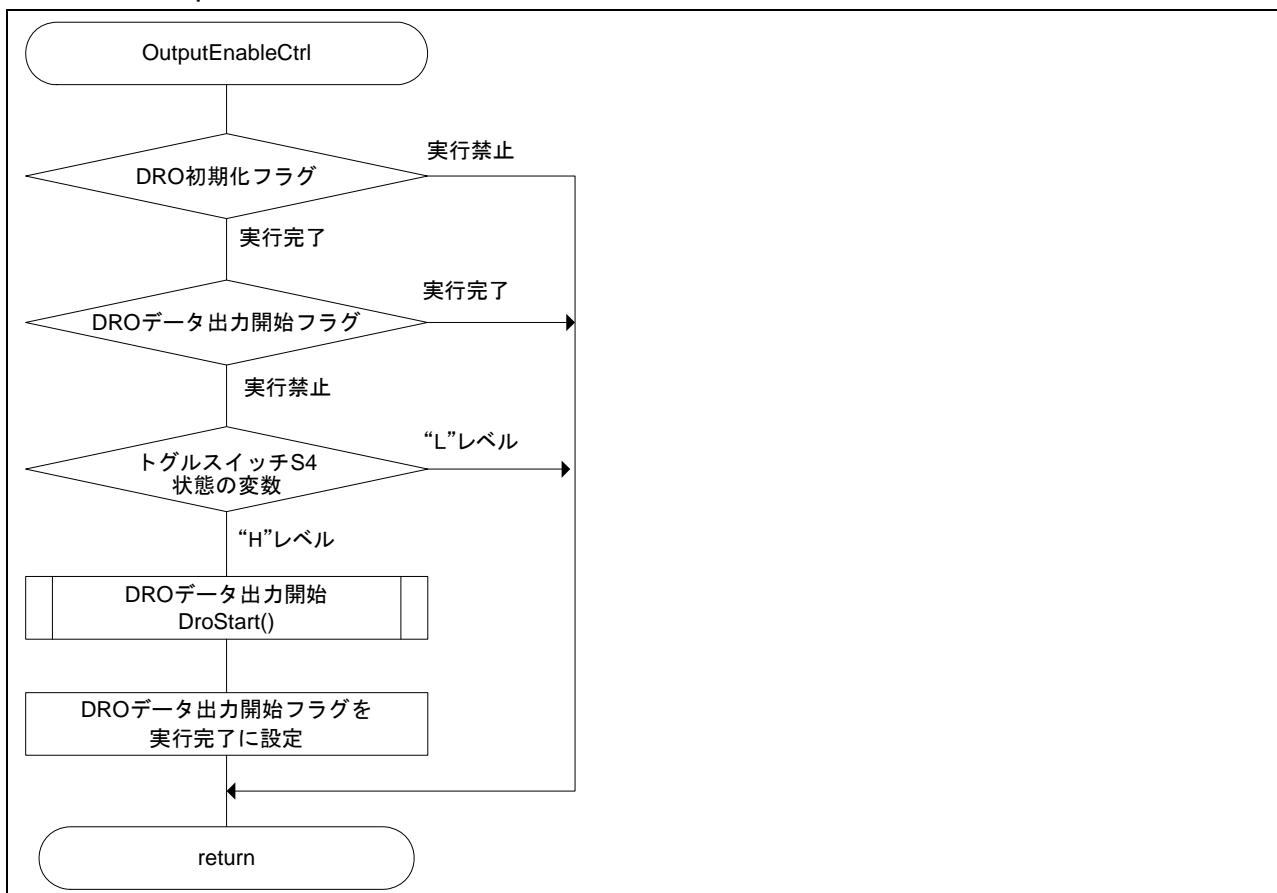
図5.8 OutputEnableCtrl 処理
