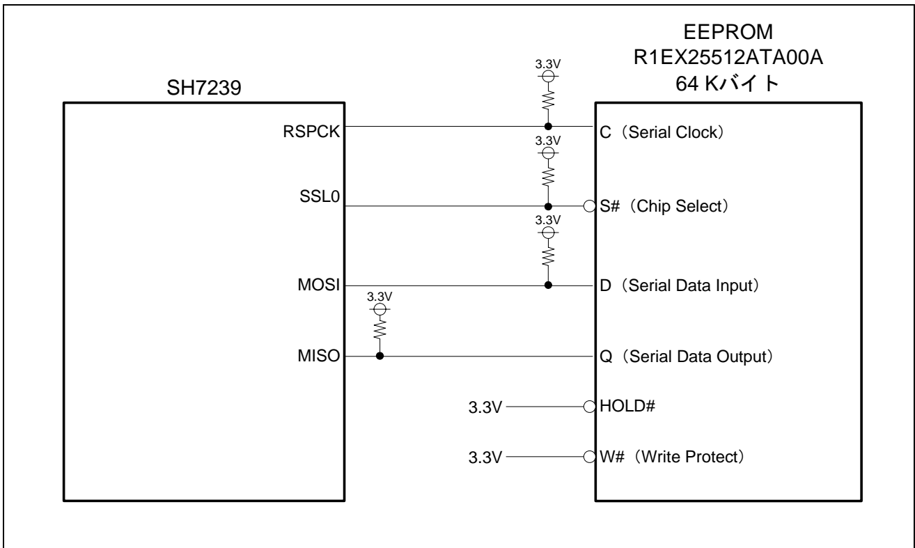
図1 EEPROM 接続回路例
